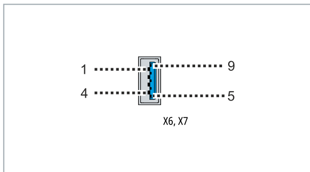
Abb. 6: USB-Schnittstellen Pin-Nummerierung
