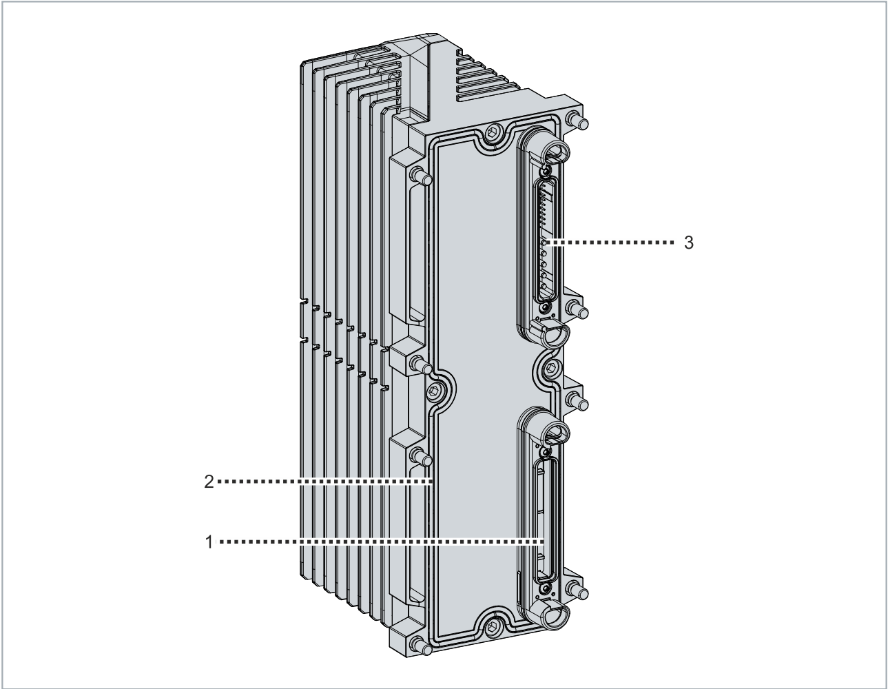
Abb. 2: Beispielaufbau eines IPC-Moduls MC6030-0080-2217, Rückansicht
