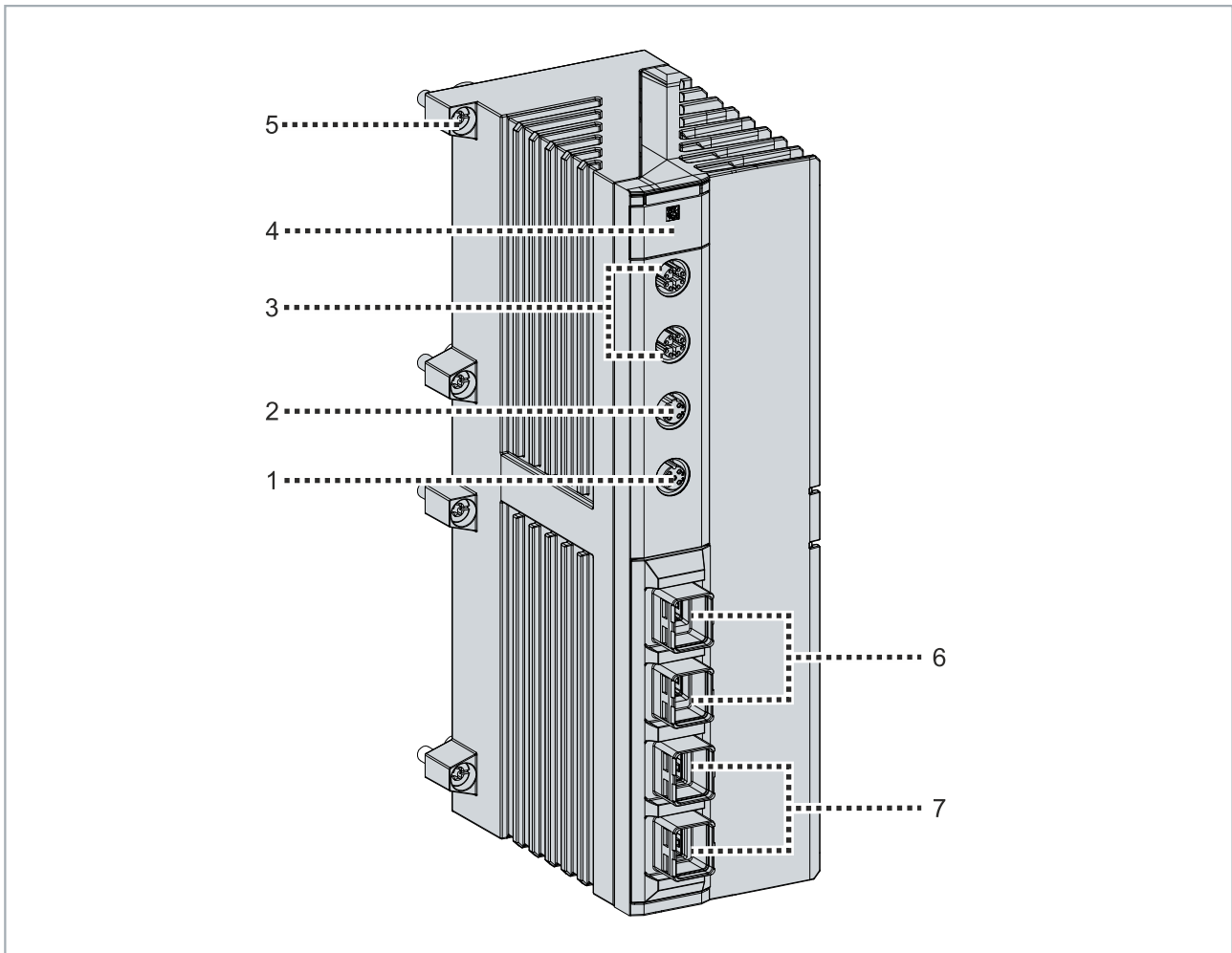
Abb. 1: Beispielaufbau eines IPC-Moduls MC6030-0080-2217, Frontansicht
