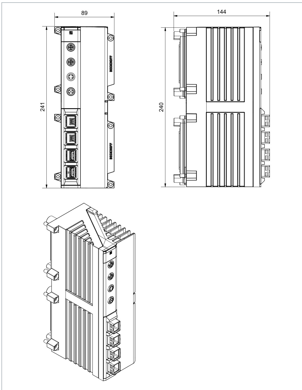
Abb. 4: MC6030-0080-2217 Abmessungen
