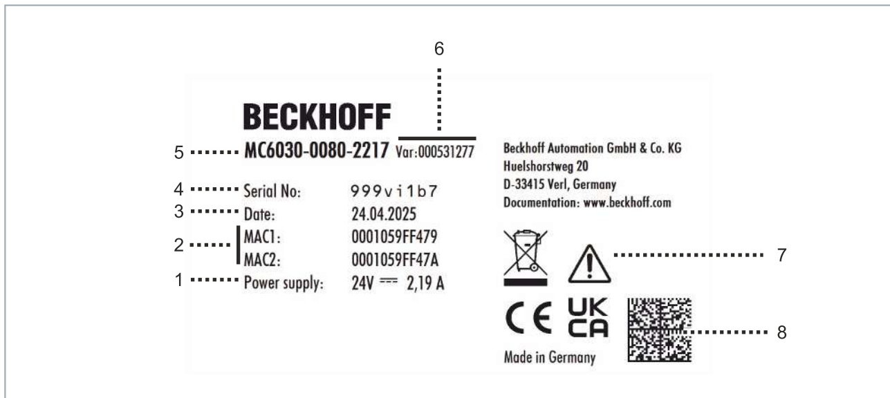
Abb. 3: Typenschild Beispielansicht.
