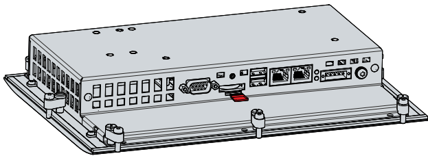
Abb. 19: CP6600_Austausch Speichermedium
