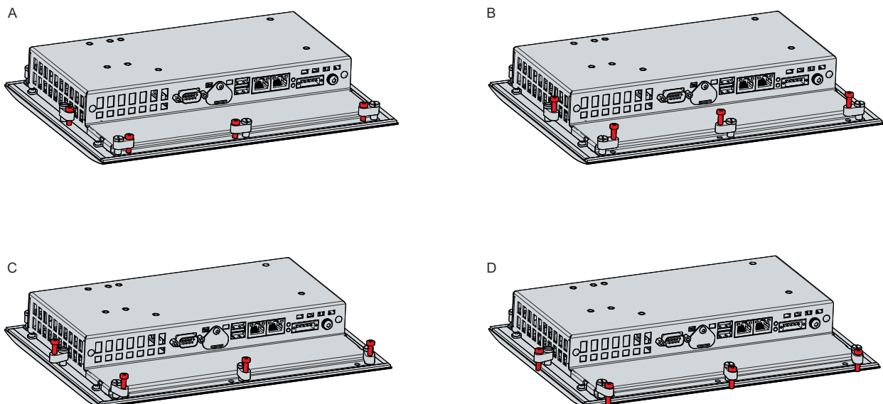
Abb. 12: CP6600_Schaltschrankeinbau
