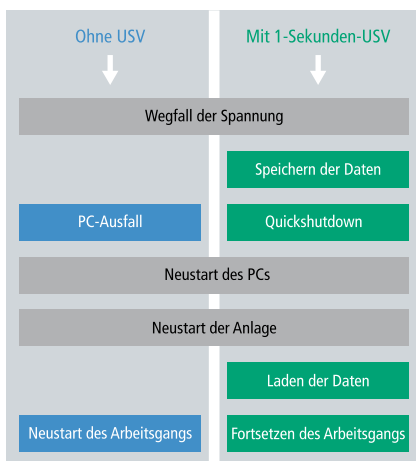
Abb. 9: Funktion USV
