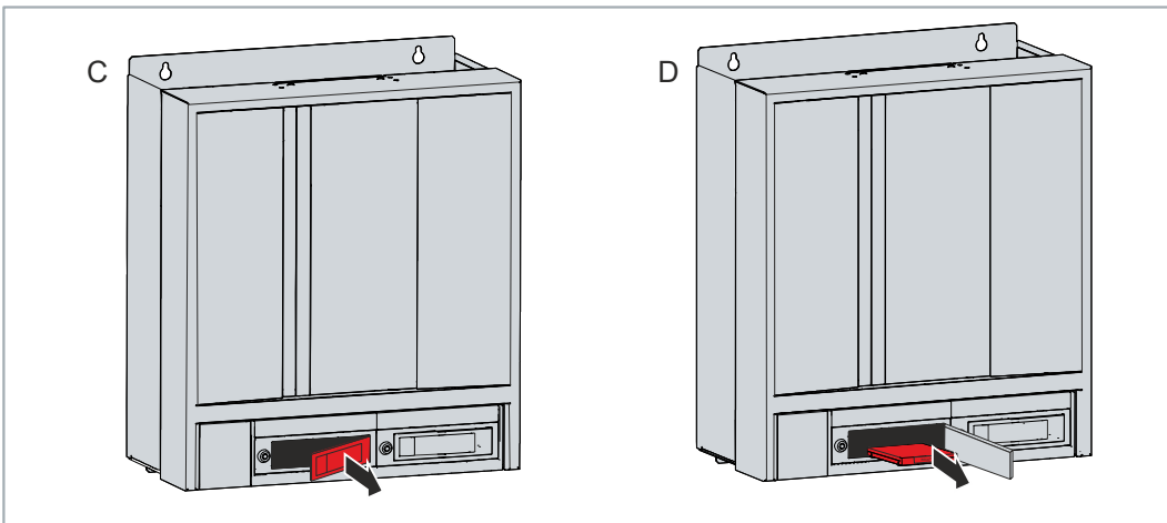
Abb. 34: Entnahme SSD
