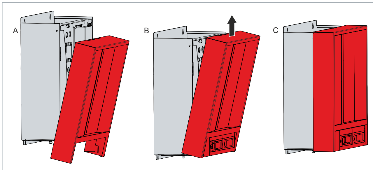
Abb. 29: Montage Gehäusedeckel
