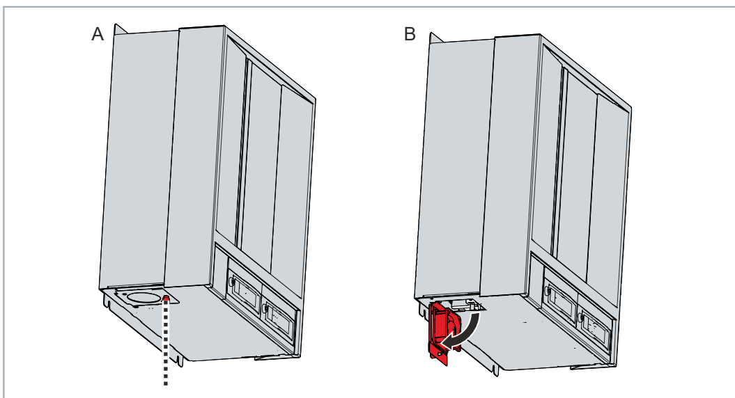
Abb. 35: Lösen Lüfterkassette
