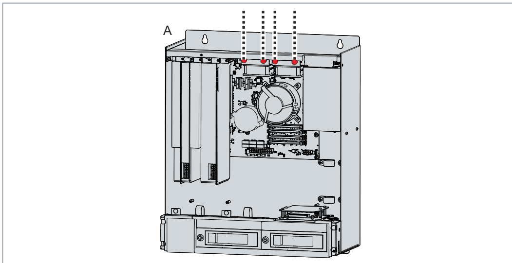
Abb. 37: Lösen Lüfterhalter
