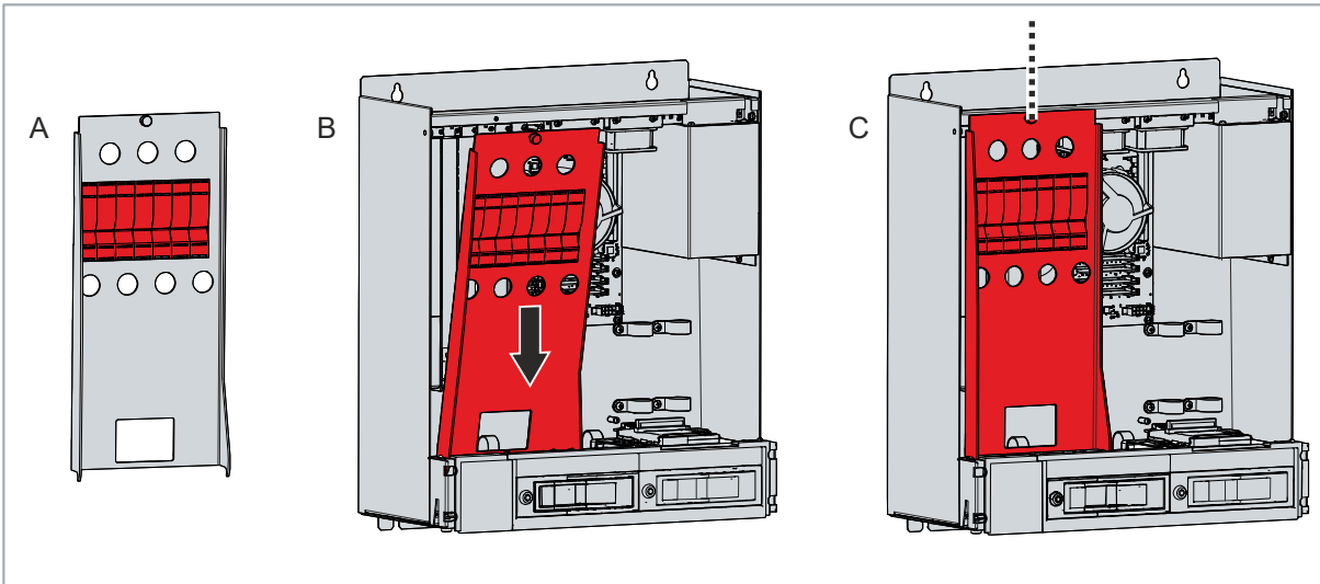
Abb. 27: Montage Kartenniederhalter
