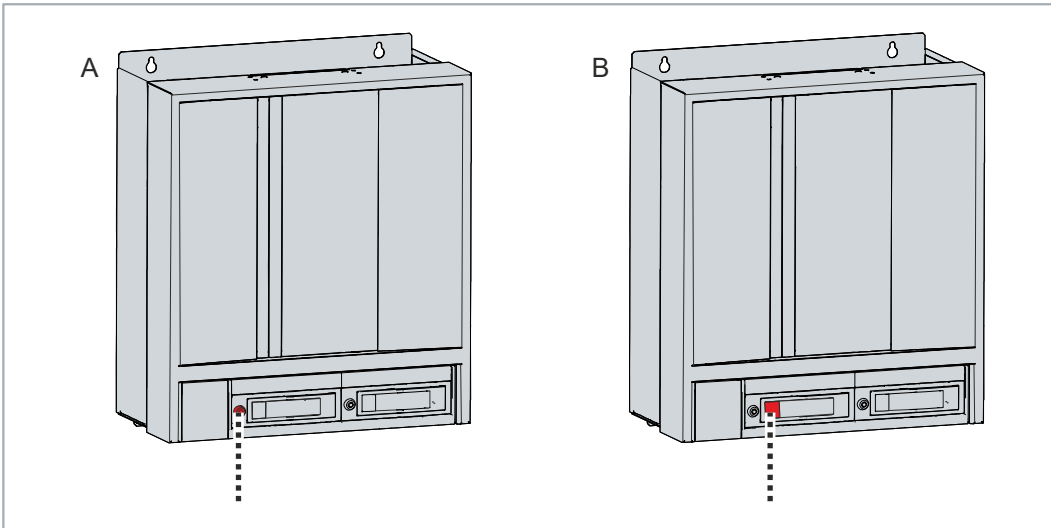
Abb. 33: Öffnen Wechselrahmen
