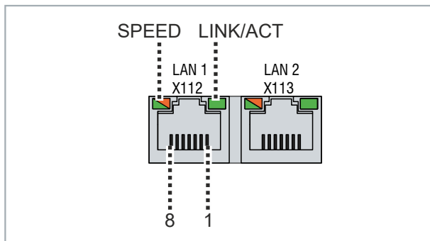
Abb. 8: Ethernet-Schnittstelle Pin-Nummerierung
