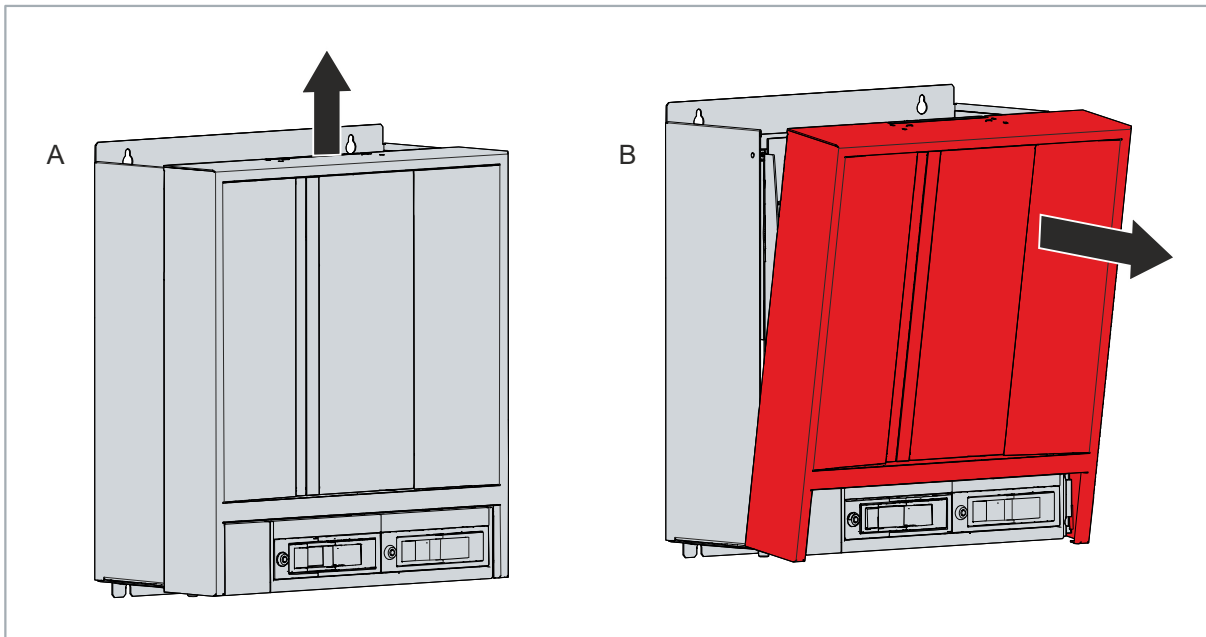
Abb. 25: Entriegelung Gehäusedeckel
