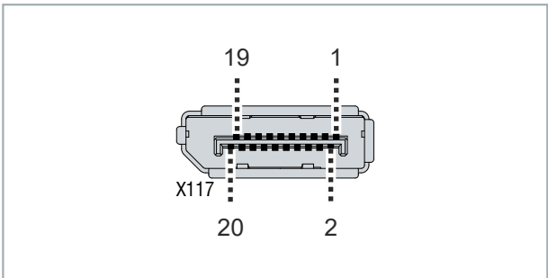
Abb. 6: DisplayPort Pin-Nummerierung
