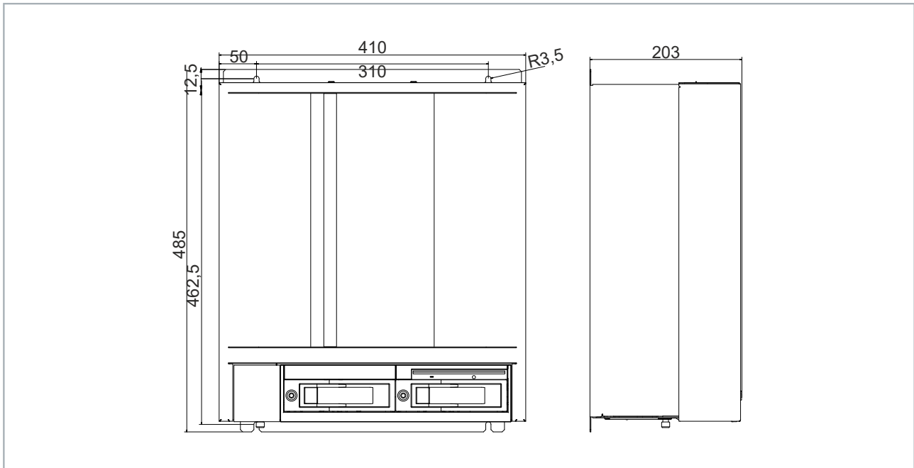
Abb. 14: Abmessungen
