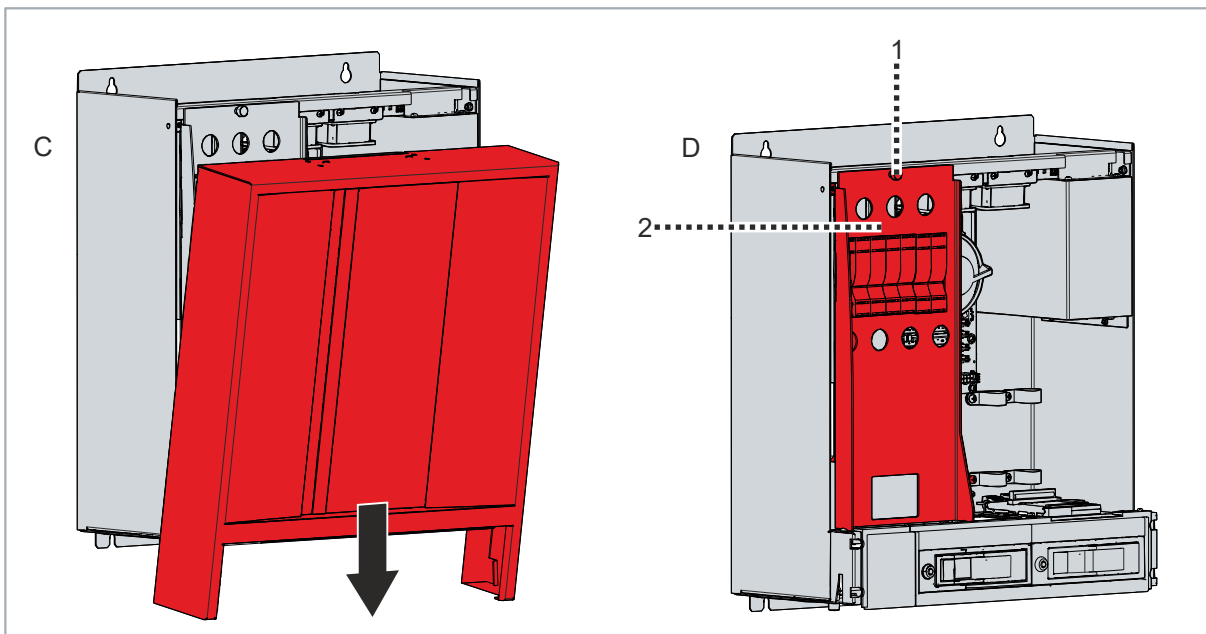
Abb. 26: Zugang Innenraum Gerät
