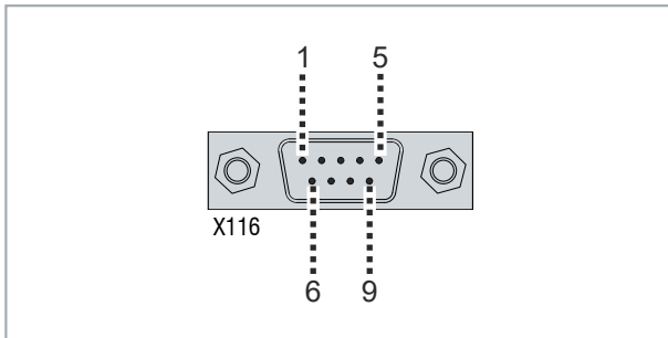
Abb. 5: RS232-Schnittstelle Pin-Nummerierung
