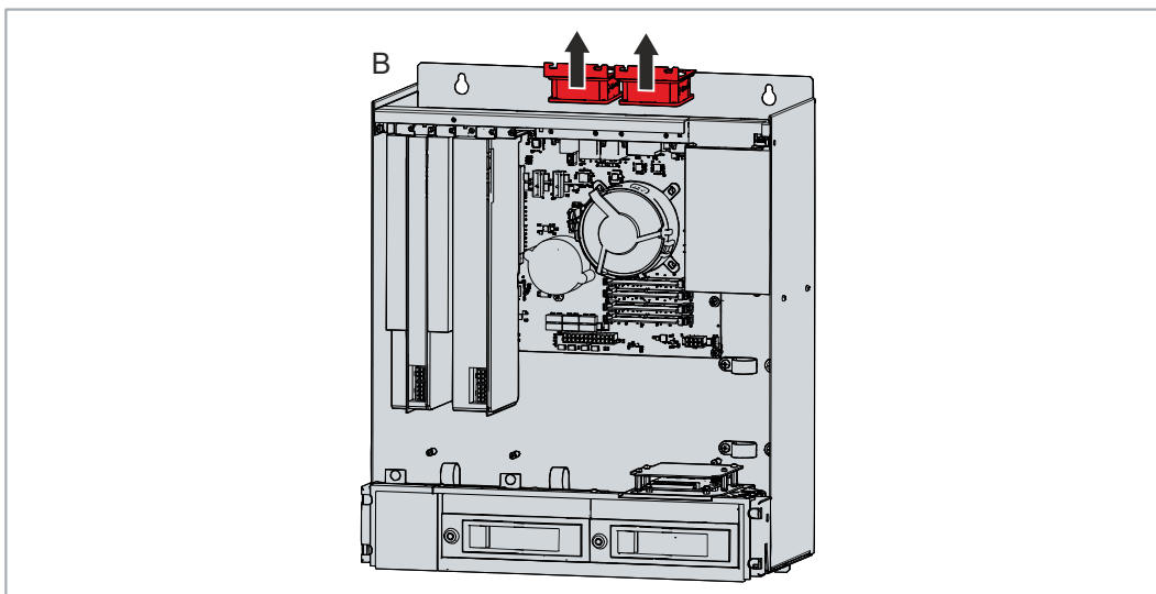
Abb. 38: Entfernen Lüfterhalter mit Lüfter
