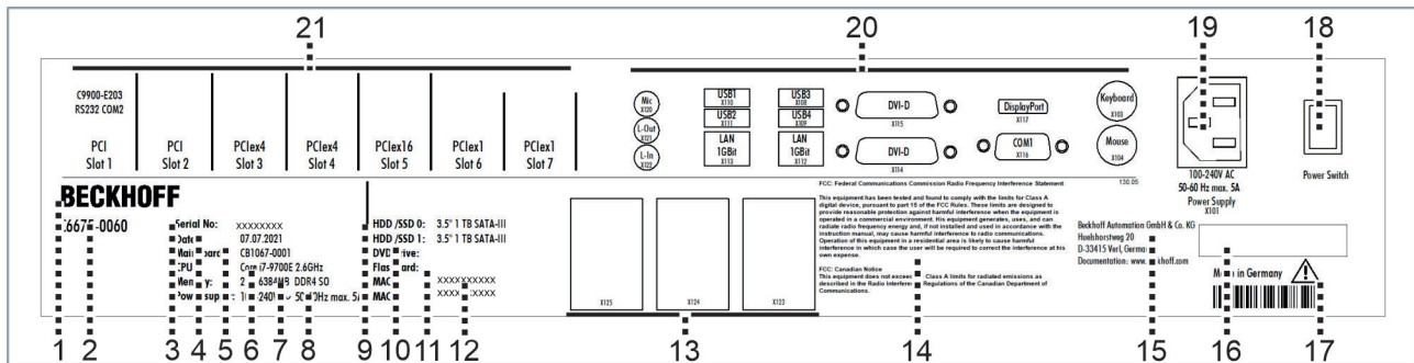
Abb. 12: Typenschild
