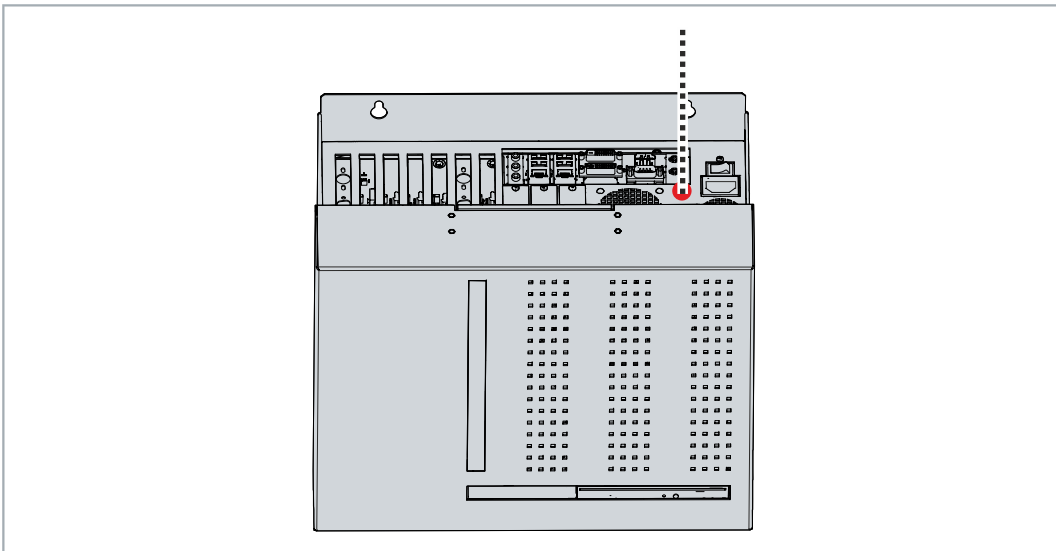
Abb. 18: Erdungsbolzen Funktionserdung
