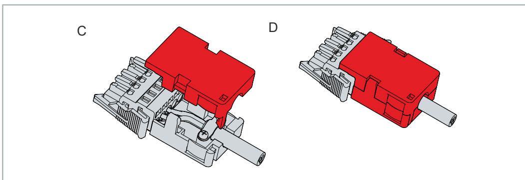
Abb. 22: Montage Oberteil Zugentlastungsgehäuse
