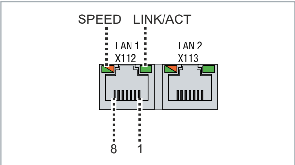
Abb. 10: Ethernet-Schnittstelle Pin-Nummerierung
