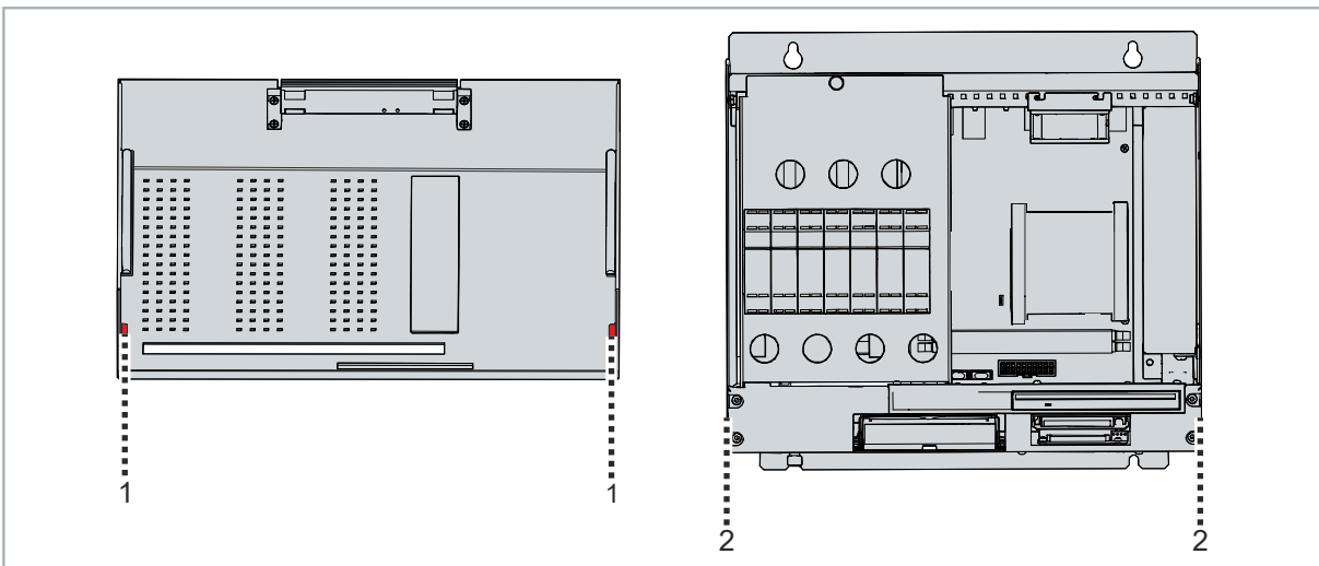
Abb. 35: Haken und Führungen
