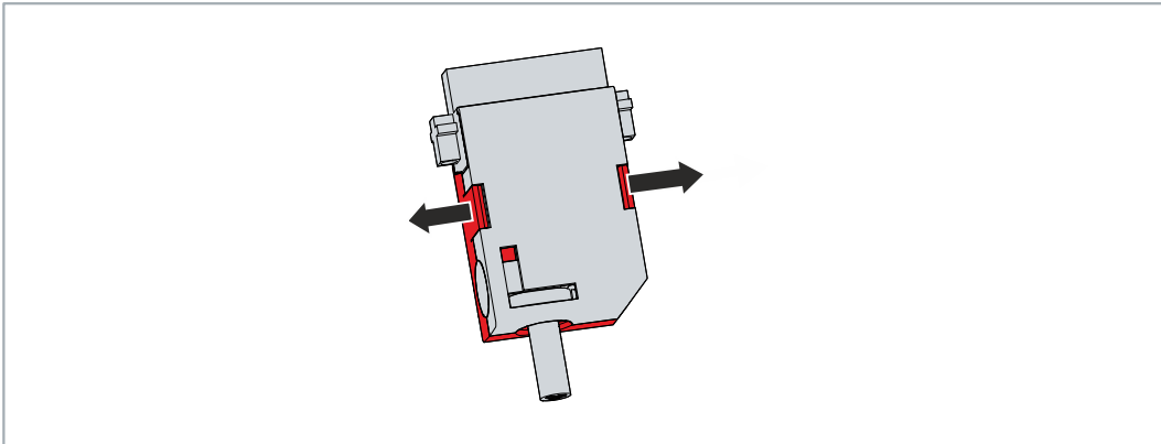
Abb. 23: Demontage Zugentlastungsgehäuse
