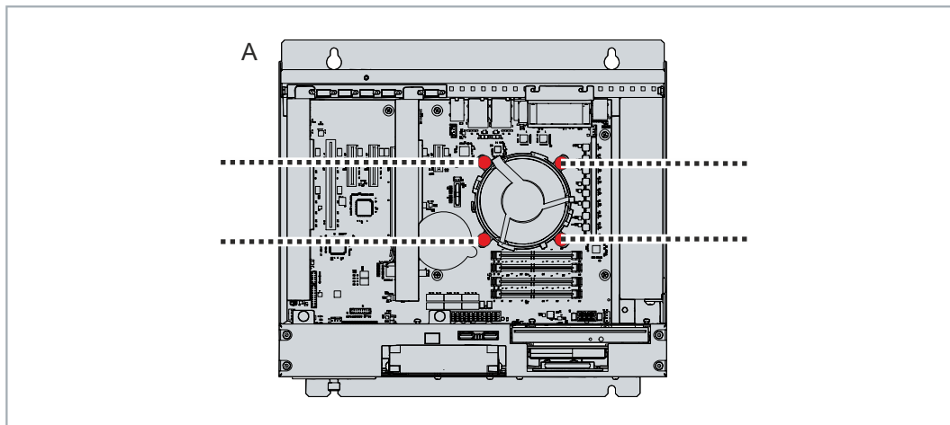
Abb. 43: Entriegelung CPU-Kühler
