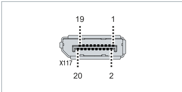
Abb. 8: DisplayPort Pin-Nummerierung
