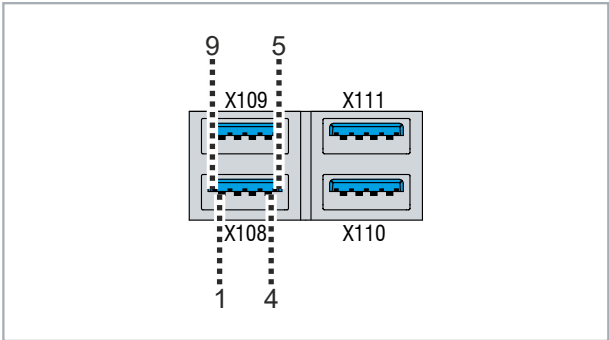
Abb. 11: USB-Schnittstelle Pin-Nummerierung
