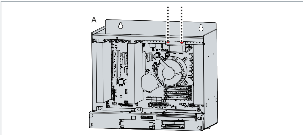
Abb. 41: Lösen Lüfterhalter
