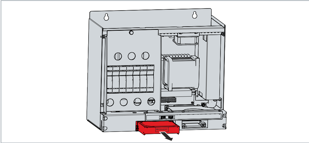
Abb. 38: Austausch Festplatte
