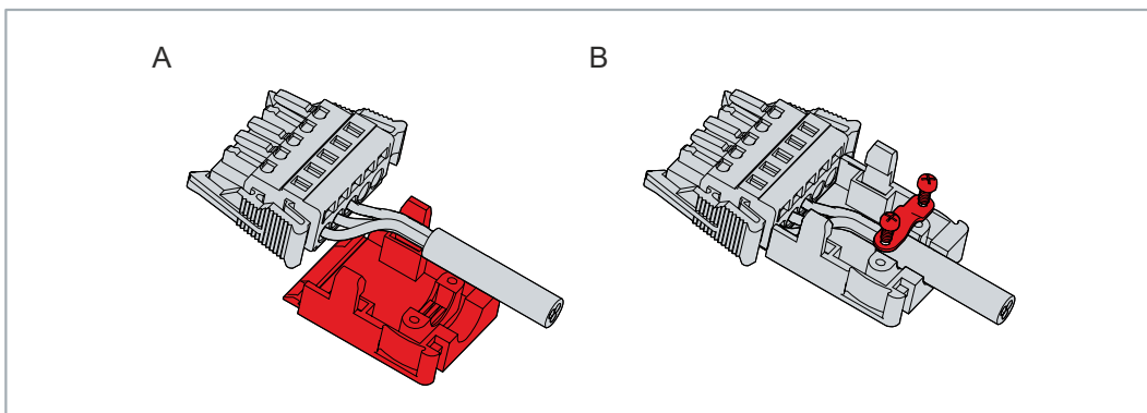
Abb. 21: Montage Zugentlastungsgehäuse
