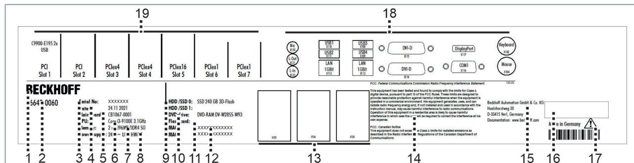
Abb. 14: Typenschild
