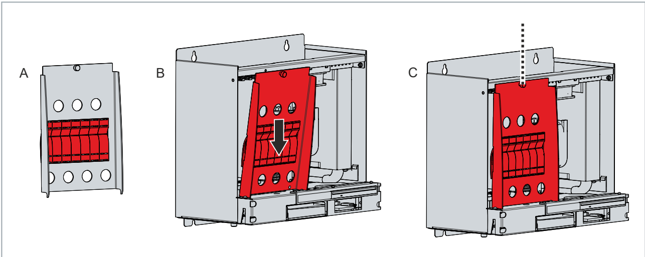
Abb. 34: Montage Kartenniederhalter
