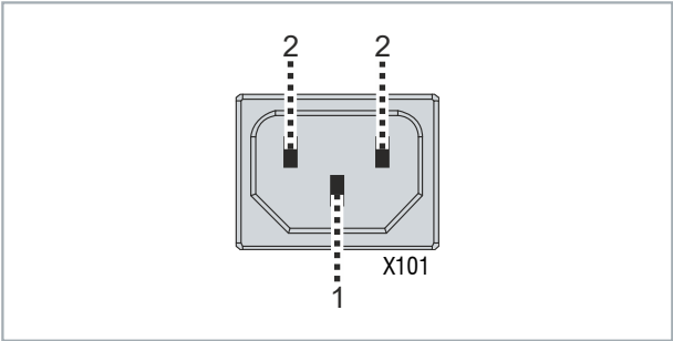
Abb. 3: Kaltgerätebuchse
