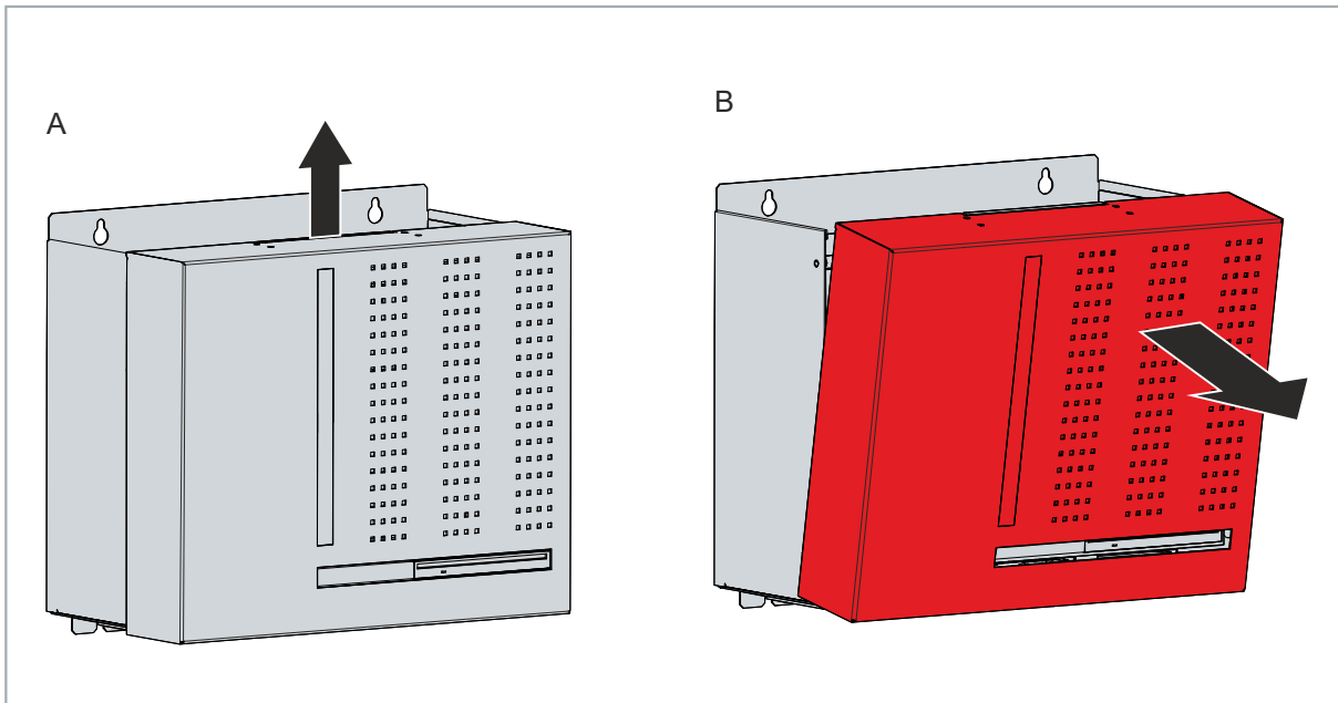
Abb. 32: Entriegelung Gehäusedeckel
