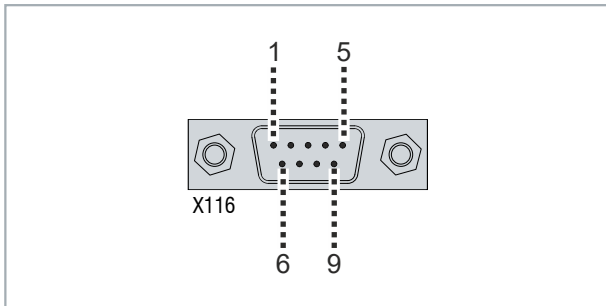
Abb. 7: RS232-Schnittstelle Pin-Nummerierung
