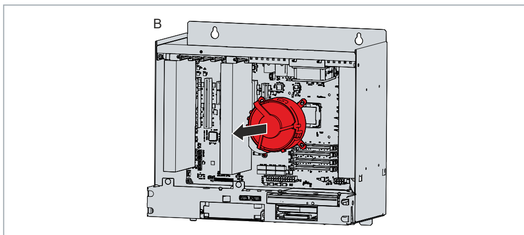
Abb. 44: Entnahme CPU-Kühler
