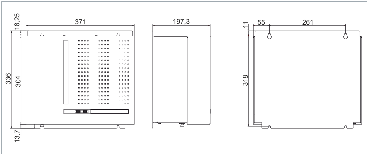
Abb. 16: Abmessungen
