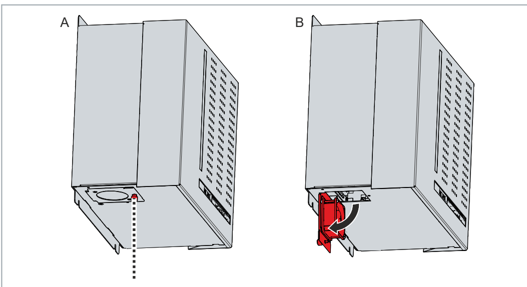
Abb. 39: Lösen Lüfterkassette
