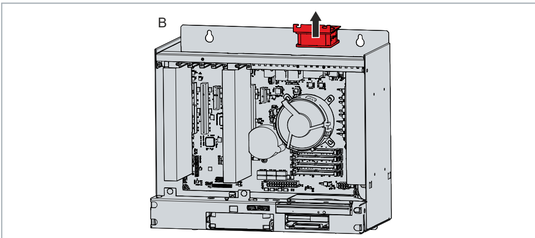
Abb. 42: Entfernen Lüfterhalter mit Lüfter
