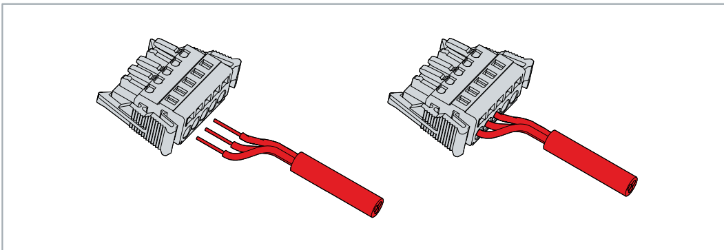
Abb. 20: Montage Versorgungsleitung
