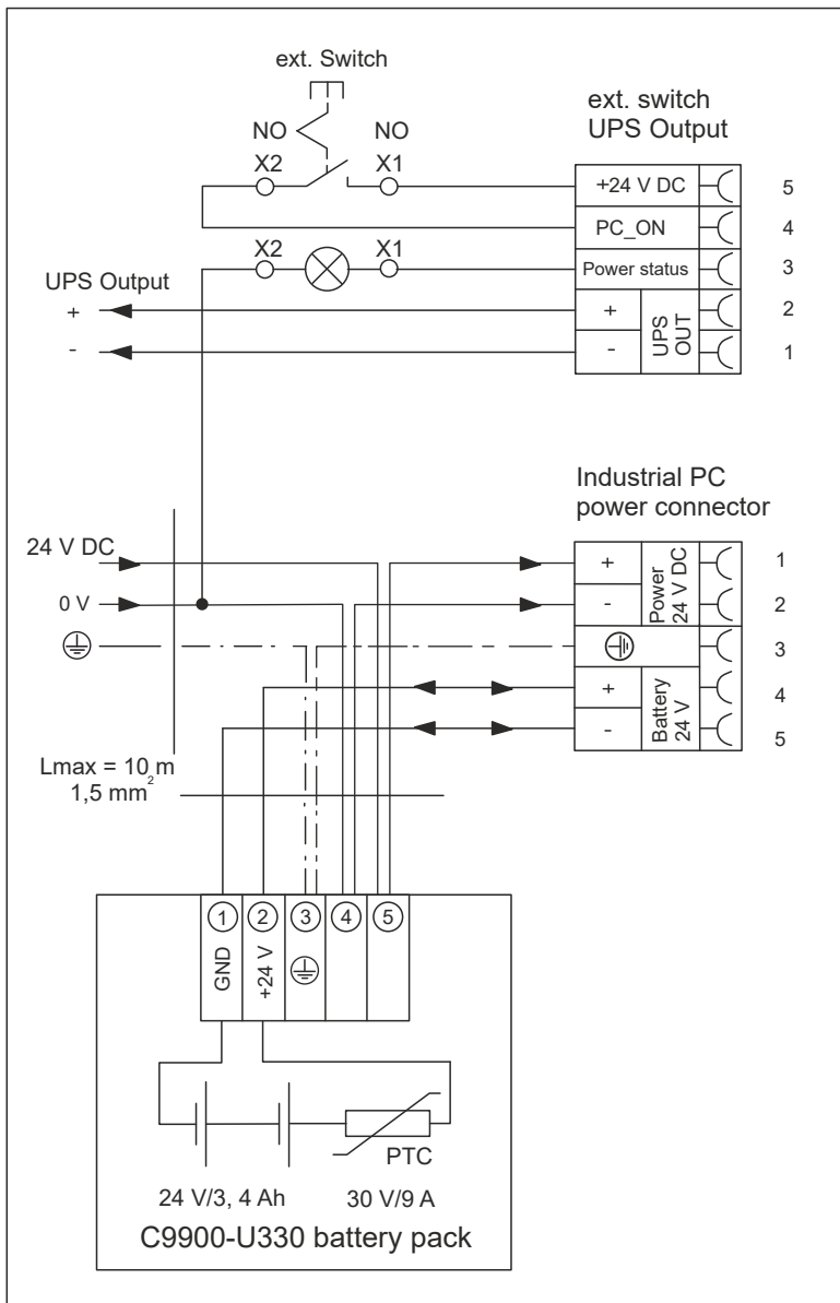
Abb. 19: Verdrahtungsplan
