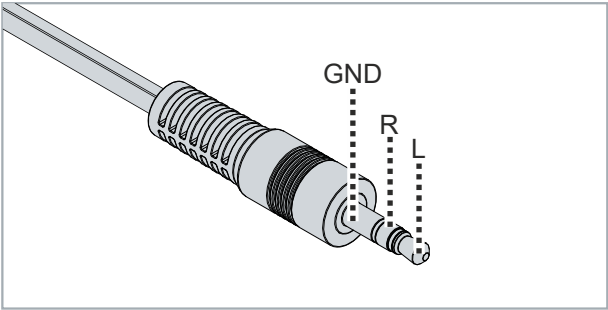
Abb. 13: Klinkenstecker Pinzuordnung
