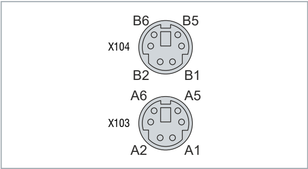
Abb. 6: PS/2-Maus und -Tastatur
