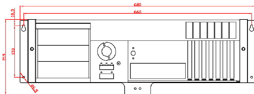
Frontansicht
