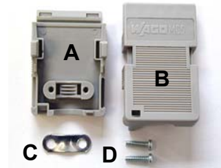
Zulentlastungsgehäuse
