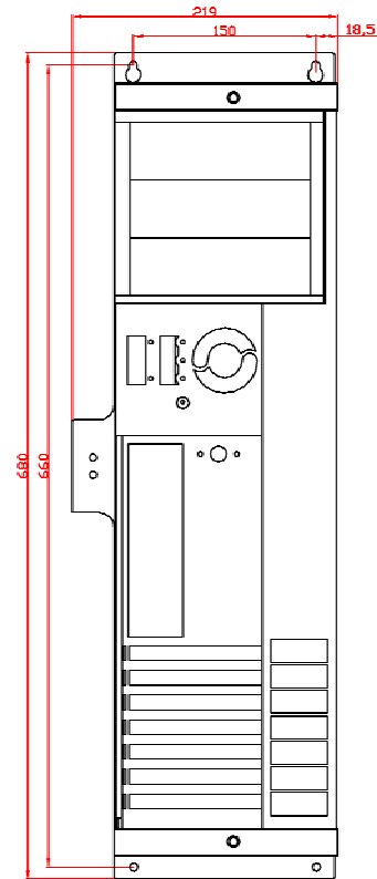
Frontansicht
