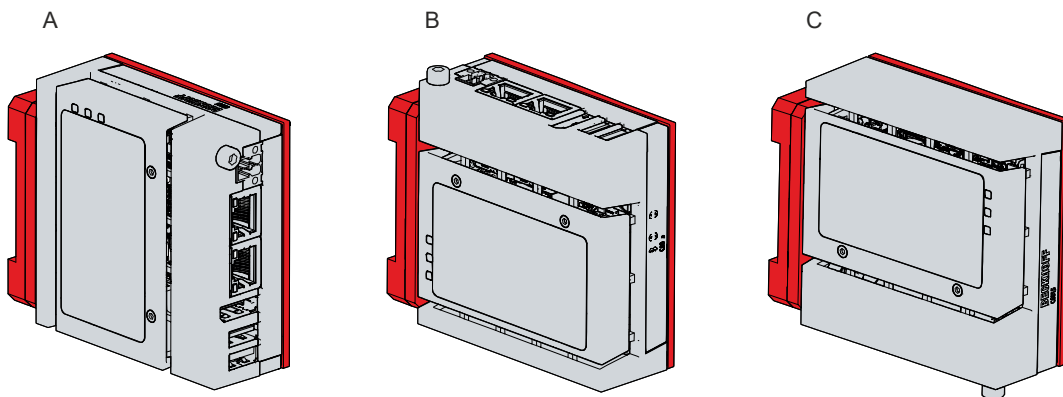
Abb. 11: Montageoptionen Montageplatte3
