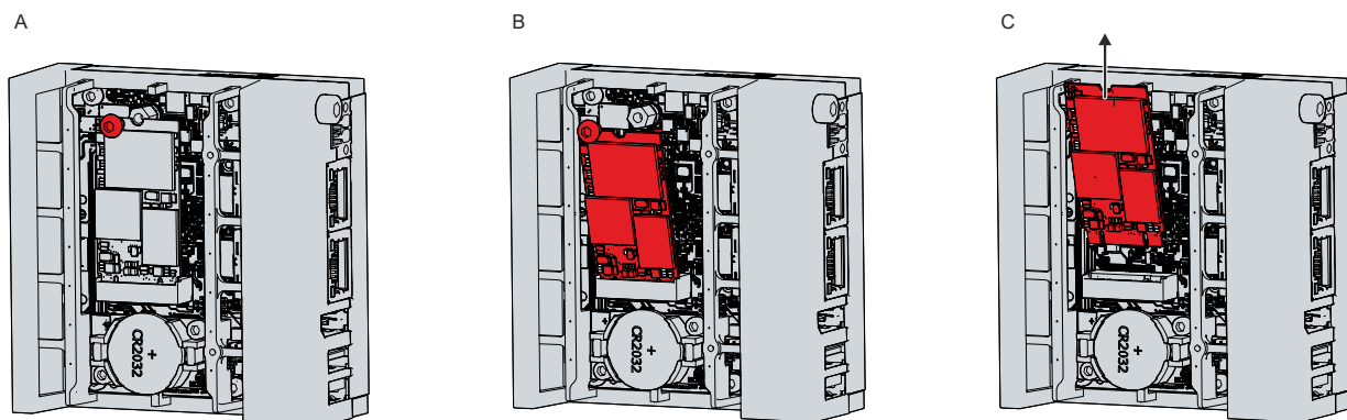
Abb. 27: Austausch Speichermedien
