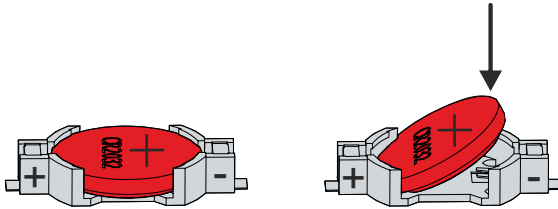
Abb. 26: Batteriewechsel
