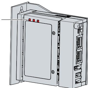
Abb. 6: Status-LEDs
