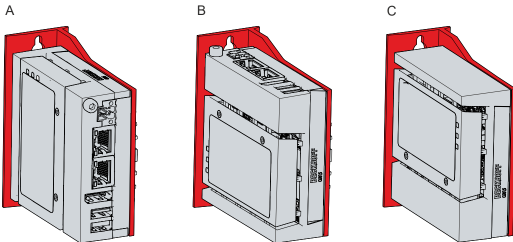
Abb. 9: Montageoptionen Montageplatte 1
