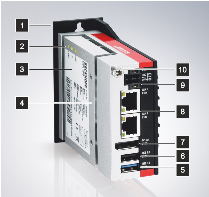
Abb. 1: Aufbau Grundausstattung
