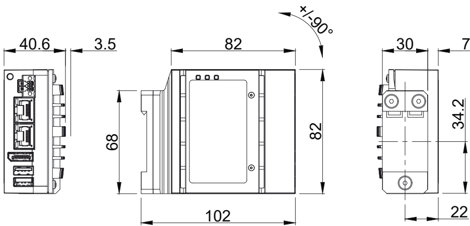
Abb. 14: Montageplatte Hutschienenadapter
