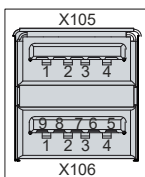
Abb. 4: USB-Schnittstelle Pin-Nummerierung
