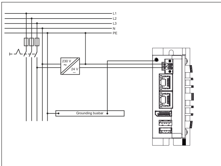
Abb. 18: Verdrahtungsbeispiel
