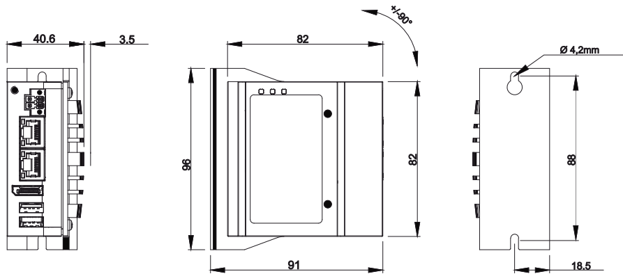
Abb. 12: Montageplatte Rückwand
