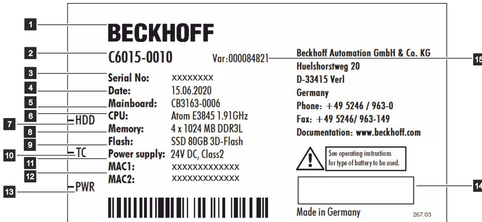
Abb. 7: Typenschild
