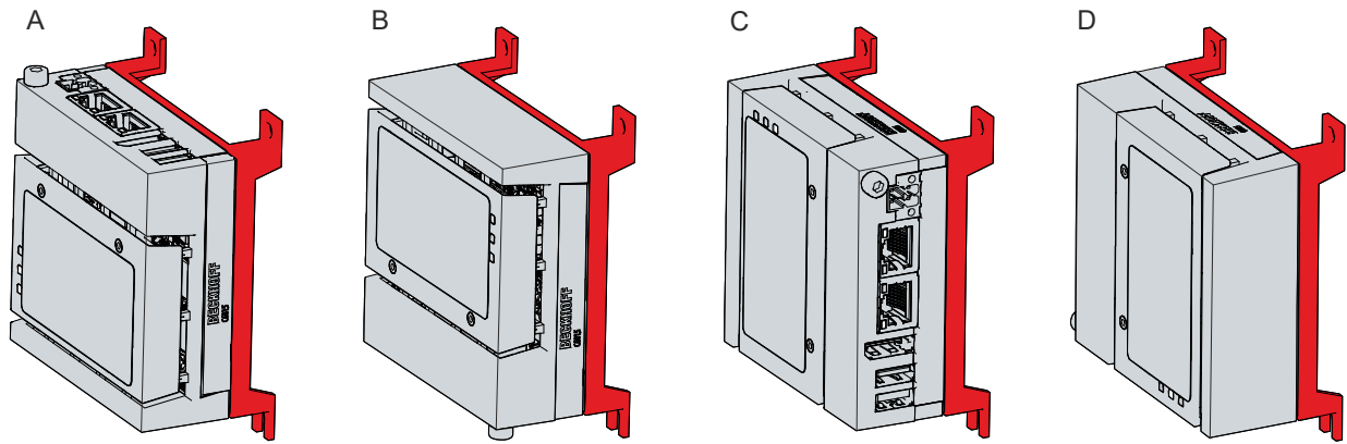
Abb. 10: Montageoptionen Montageplatte2
