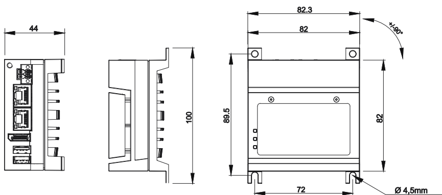
Abb. 13: Montageplatte Seitenwand
