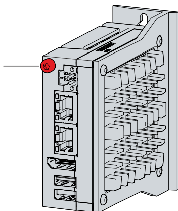
Abb. 19: Schutzleiteranschluss PE
