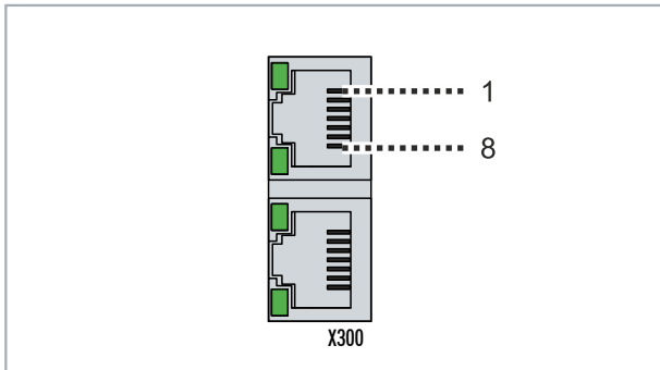
Abb. 14: EtherCAT-Master-Schnittstelle X300.
