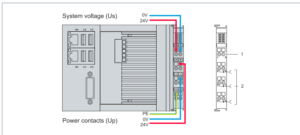
Abb. 23: Anschlüsse für Systemspannung (Us) und Powerkontakte (Up)
