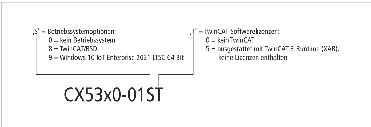
Abb. 3: Bezeichnungssystematik des Embedded-PCs CX53x0.
