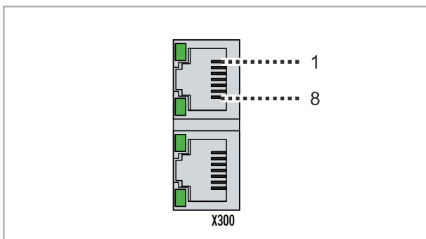
Abb. 15: EtherCAT-Slave-Schnittstelle X300.
