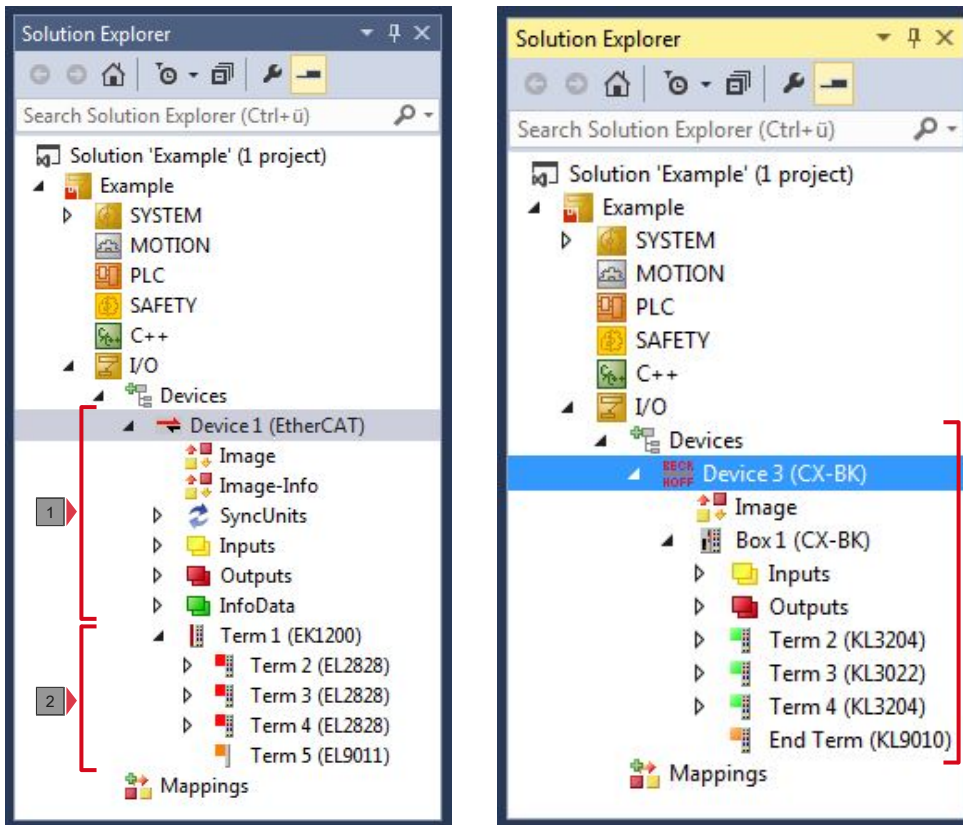
Abb. 27: Embedded-PC CX53x0 in der Strukturansicht von TwinCAT 3, mit angereihten EtherCAT-Klemmen (links) oder Busklemmen (rechts).
