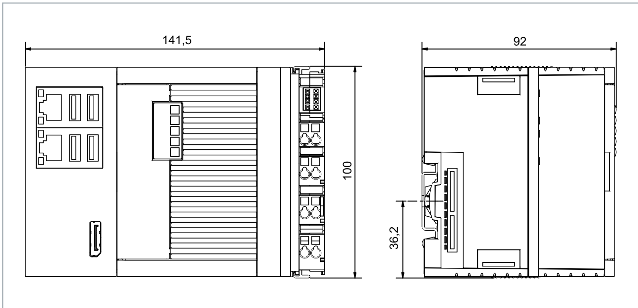
Abb. 19: Embedded-PC CX53x0, Abmessungen.
