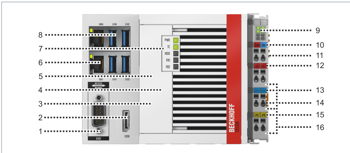
Abb. 1: Beispielaufbau eines Embedded-PCs CX5340.
