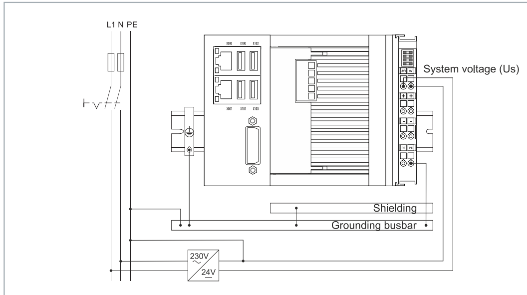
Abb. 24: Anschlussbeispiel mit einem CX52x0.
