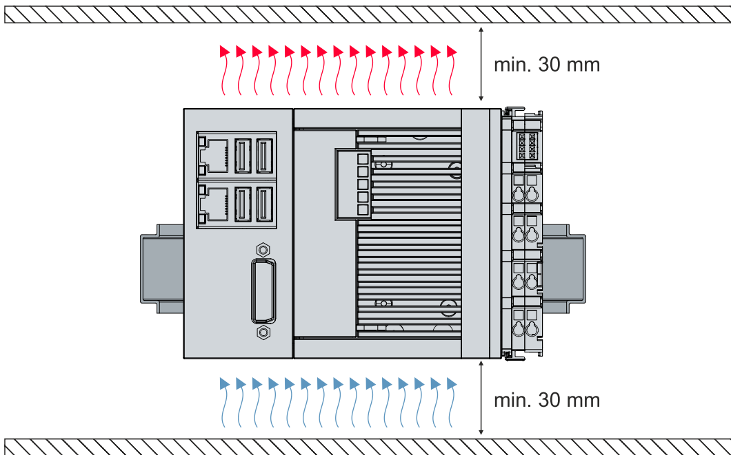
Abb. 20: Embedded-PC CX53x0, zulässige Einbaulage.
