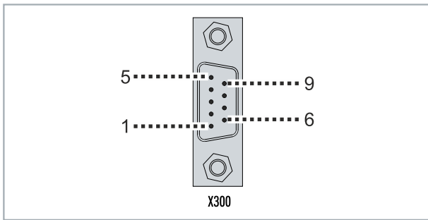
Abb. 12: RS232-Schnittstelle X300.
