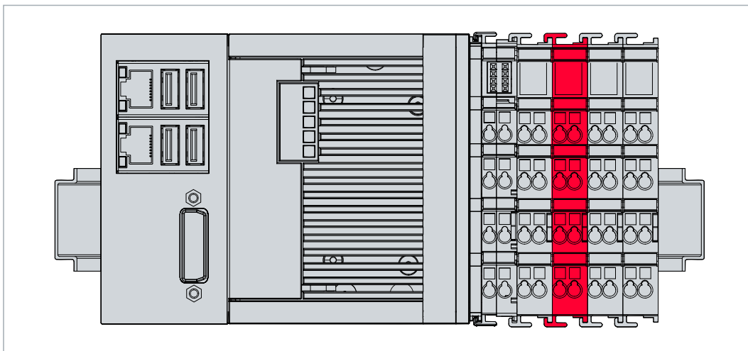
Abb. 22: Passive EtherCAT-Klemmen, zulässige Montage.
