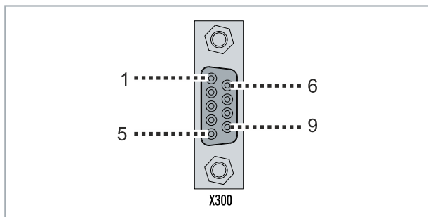
Abb. 13: RS485-Schnittstelle X300.
