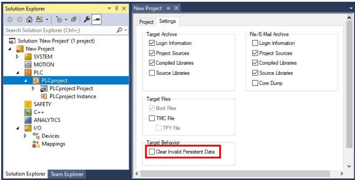
Abb. 29: Backup der persistenten Daten laden. Einstellungen unter TwinCAT 3.
