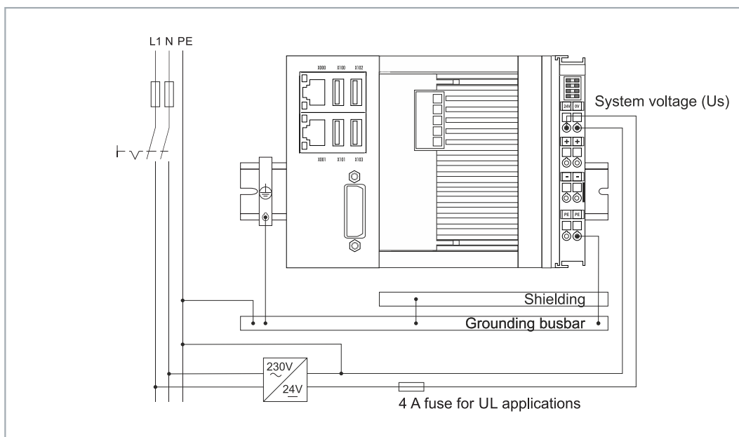
Abb. 26: Anschlussbeispiel für Bereiche mit speziellen UL-Anforderungen.
