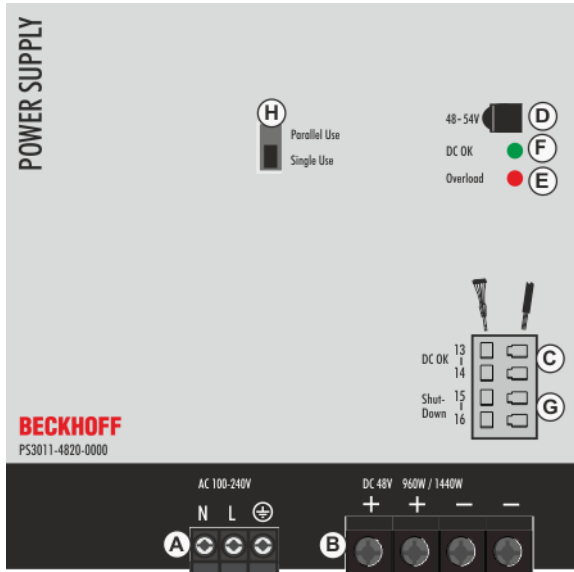
Fig. 16: Front PS3011-4820-0000
