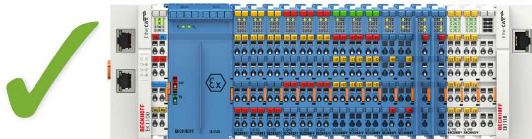
附图 8: 允许的安裝 - 不属于 ELX 系列的端子模块被放置在 ELX 端子模块网段的前后。由 ELX 端子模块网段开头的 ELX9560 和 ELX 端子模块网段末端的两个 ELX9410 隔离。
