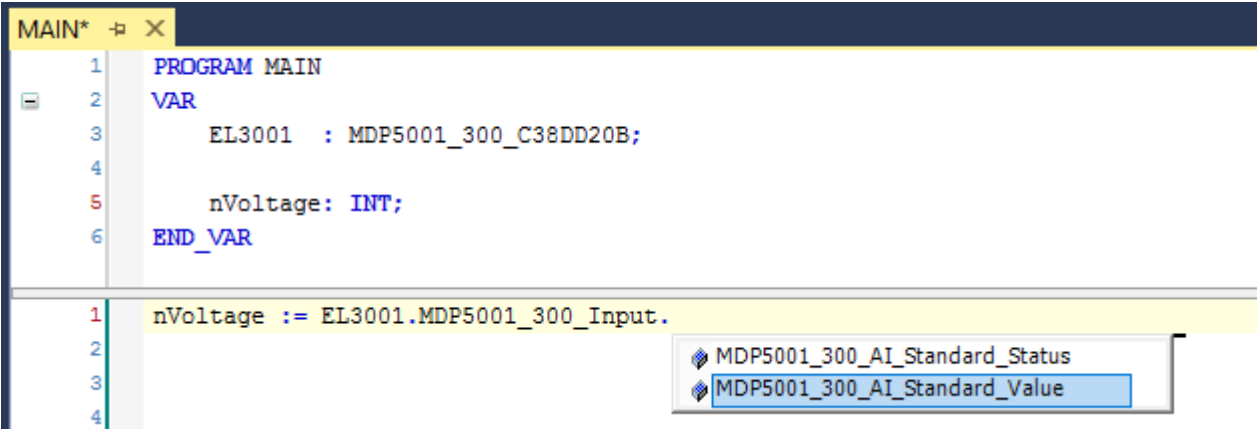
附图 82: 从过程数据的结构中读取一个变量
