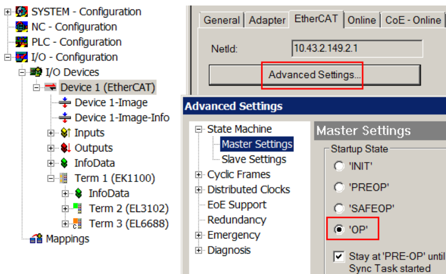
附图 145: 系统管理器的默认行为
