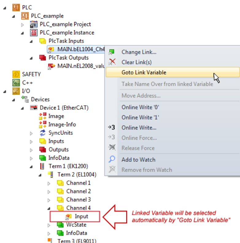
附图 78: 应用“转到链接变量”变量，以“MAIN.bEL1004_Ch4”为样本
