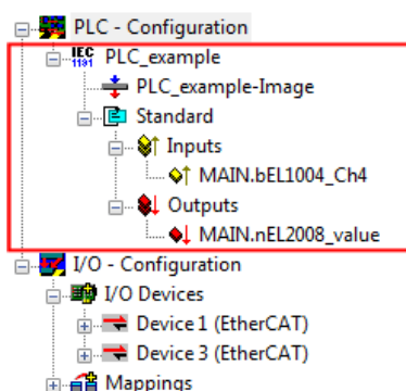
附图 54: 集成在系统管理器的PLC配置中的PLC项目
