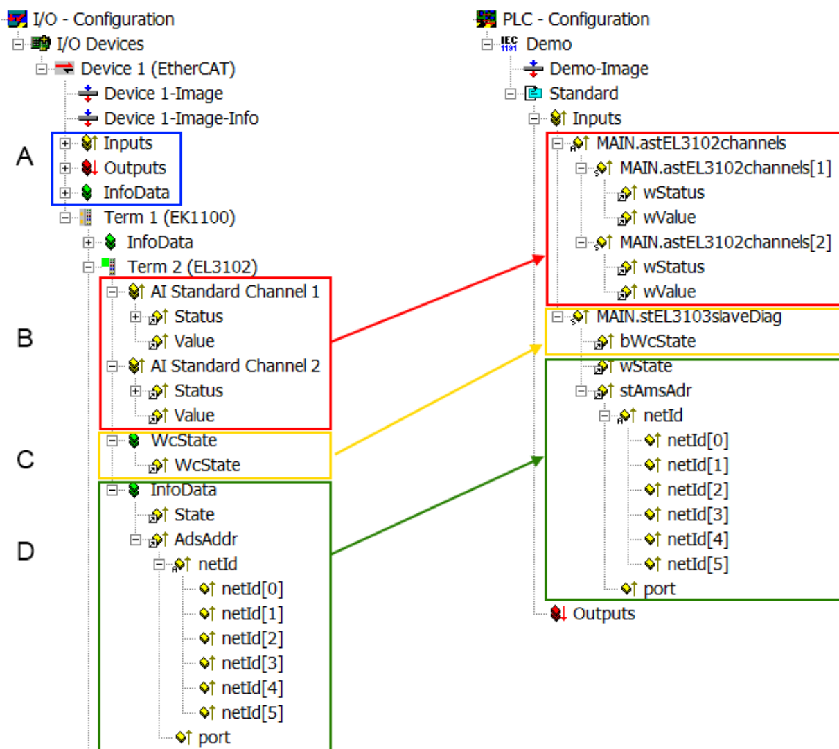
附图 142: PLC 中的 EtherCAT 从站基本诊断
