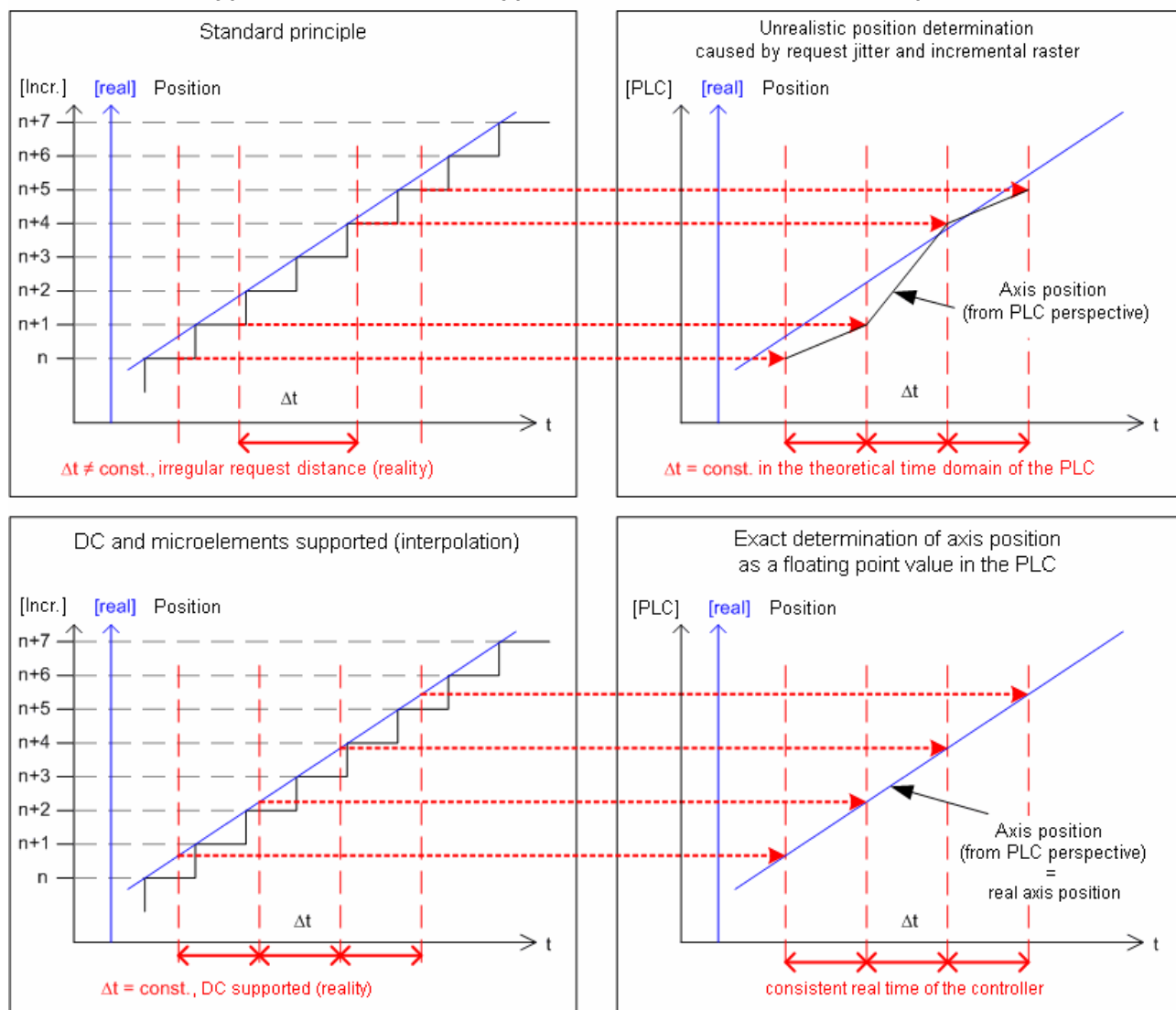
附图 32: 频率测量的原理
