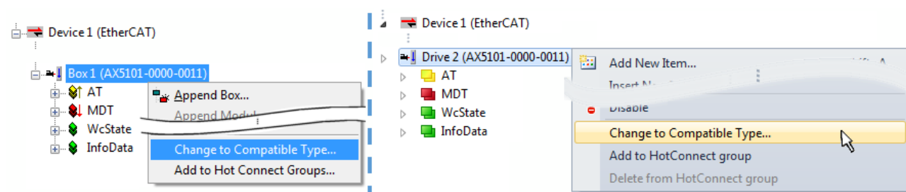
附图 129: 对话框“更改为兼容类型...”（左：TwinCAT 2；右：TwinCAT 3）
