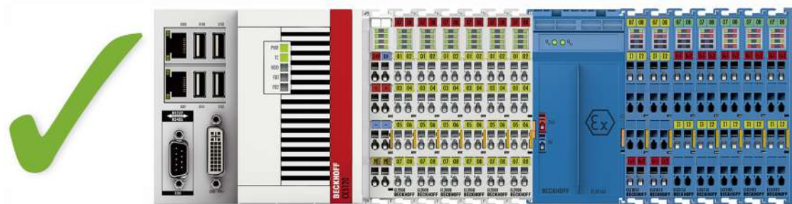
附图 7: ELX 端子模块的允许安装（右侧端子模块）。
