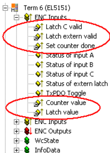
附图 156: 与 NC 任务相连的 EL5151 输入端
