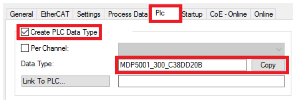
附图 79: 创建一个PLC数据类型
