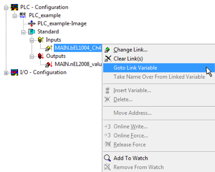
附图 58: 应用“转到链接变量”变量，以“MAIN.bEL1004_Ch4”为样本
