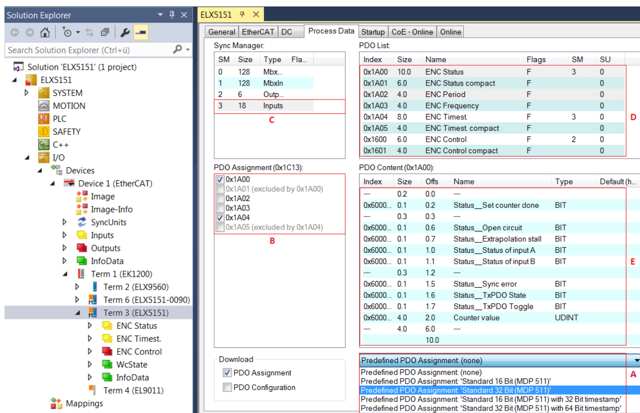
附图 27: ELX5151 - 选择对话框预定义的 PDO 分配
