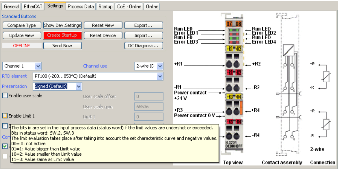
附图 144: EL3204 调试助手示例
