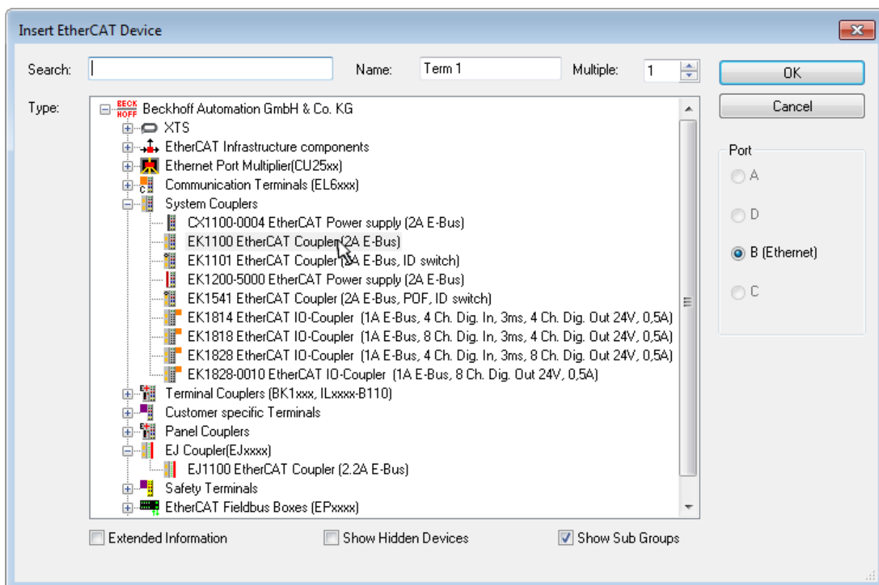
附图 105: 新EtherCAT设备的选择对话框
