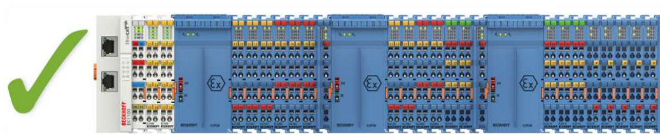
附图 10: 允许的安裝 - 由 ELX9560 提供多个再次供电电源，在每种情况下都有一个前端的 ELX9410。
