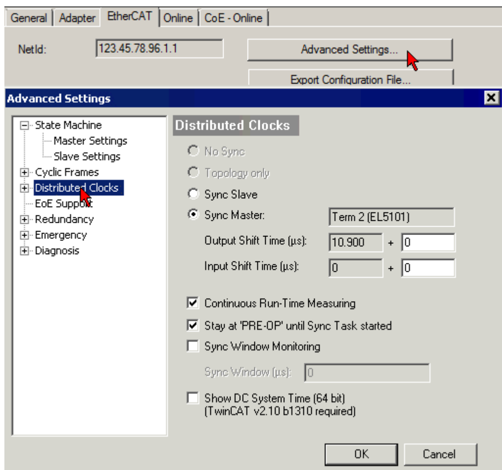
附图 159: EtherCAT 主站，高级设置，分布式时钟
