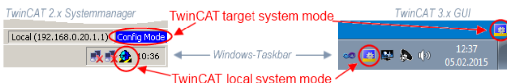
附图 110: 差异化的本地/目标系统（左：TwinCAT 2；右：TwinCAT 3）
