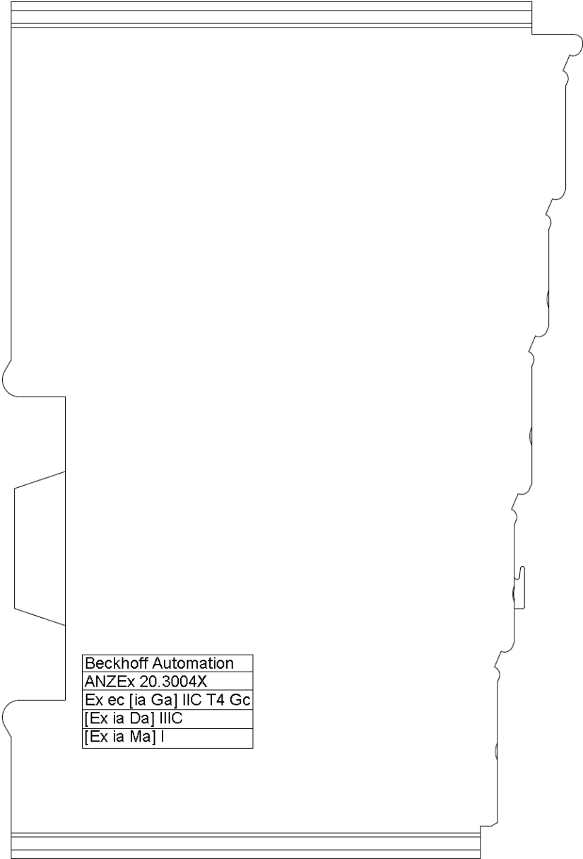
附图 4: ELX2002 带有 ANZEx 标识
