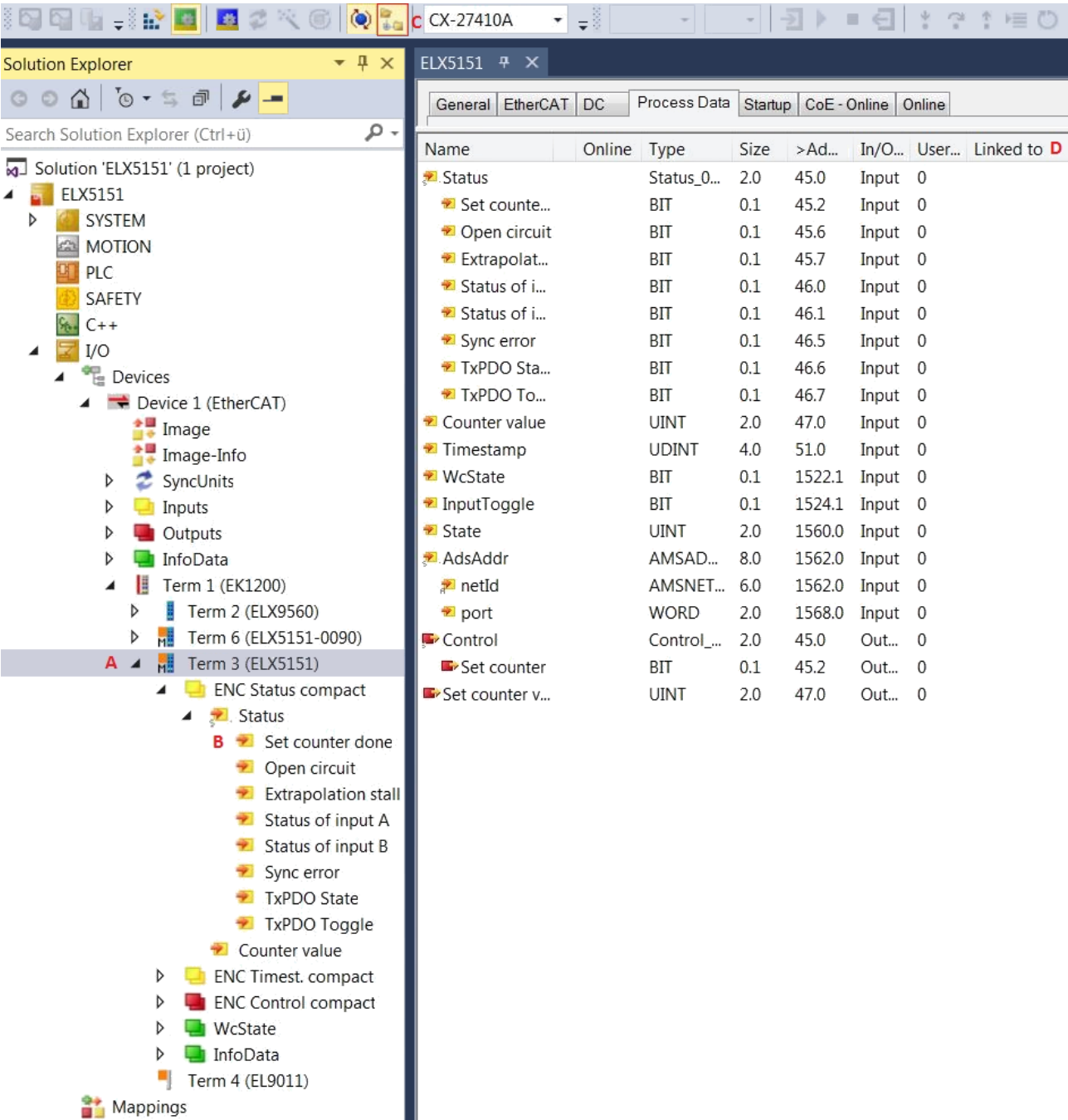
附图 24: ELX5151 - 在线显示过程数据和结构内容
