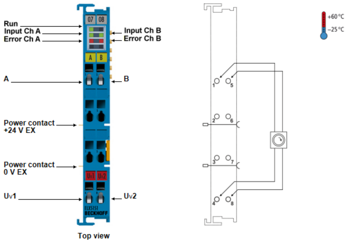
附图 22: ELX5151 - 触点分配
