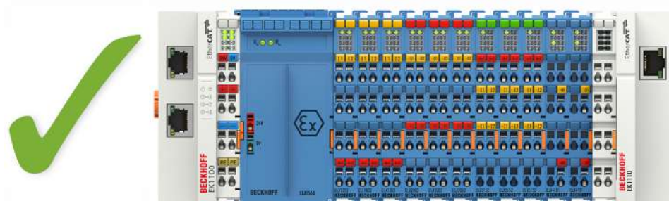
附图 9: 允许的安裝 - 不属于 ELX 系列的端子模块被放置在 ELX 端子模块网段的前后。由 ELX 端子模块网段开头的 ELX9560 和 ELX 端子模块网段末端的 EK1110 隔离。
