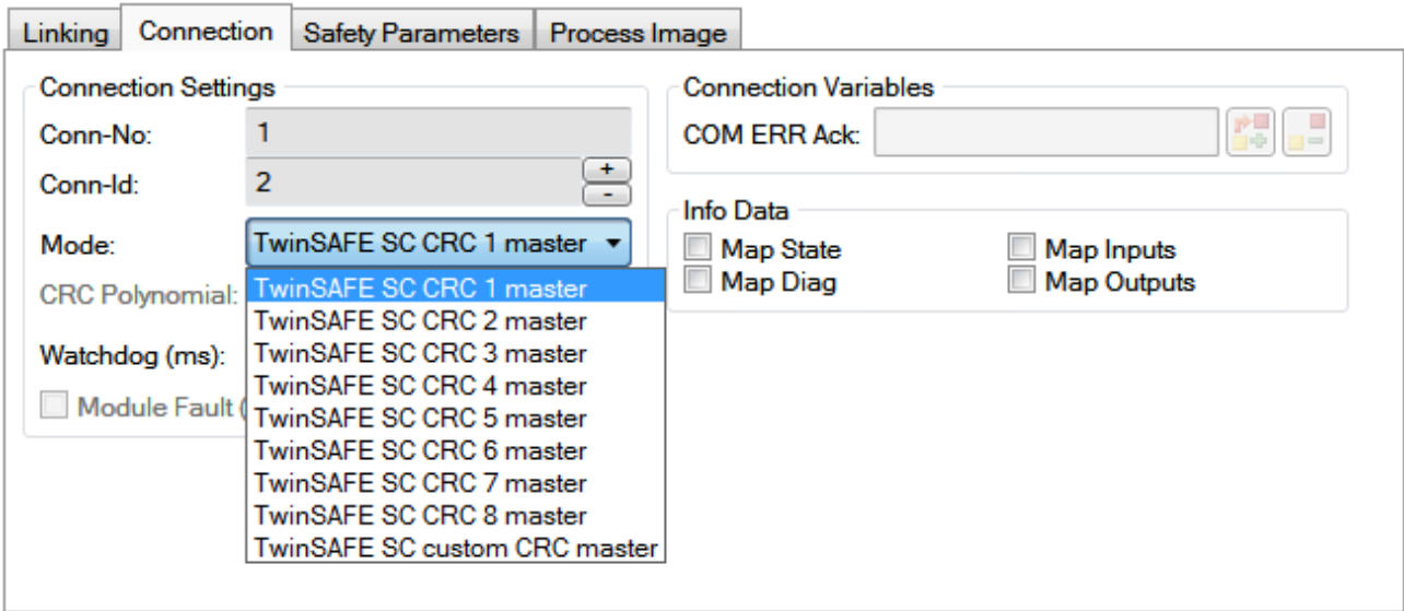
附图 37: 选择一个自由CRC
