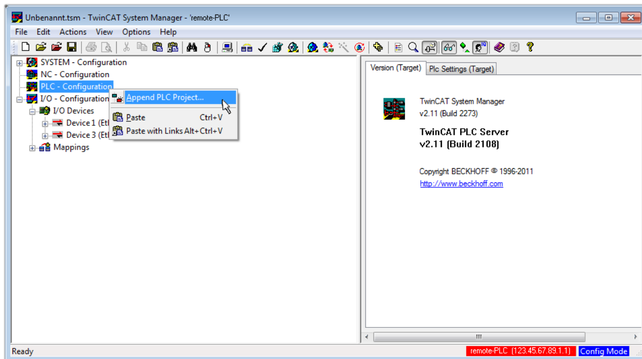
附图 53: 添加TwinCAT PLC控制项目
