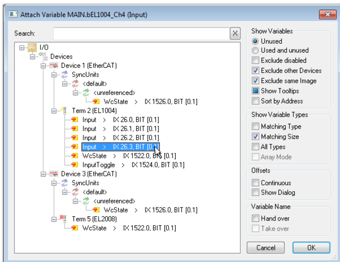
附图 76: 选择BOOL类型的PDO
