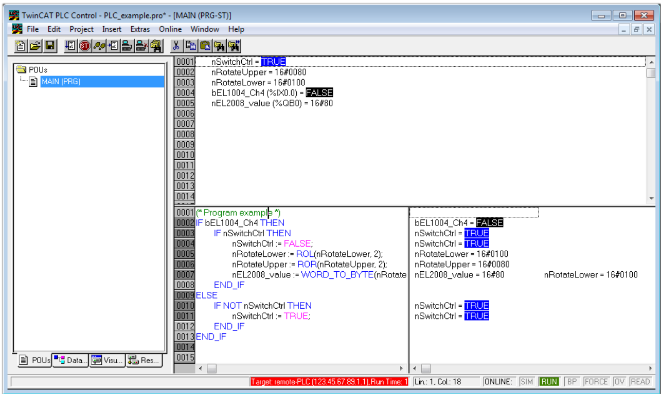
附图 60: PLC控制器登录，准备启动程序
