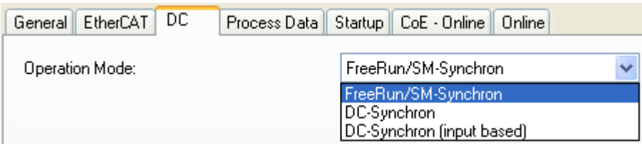
附图 25: DC 选项卡
