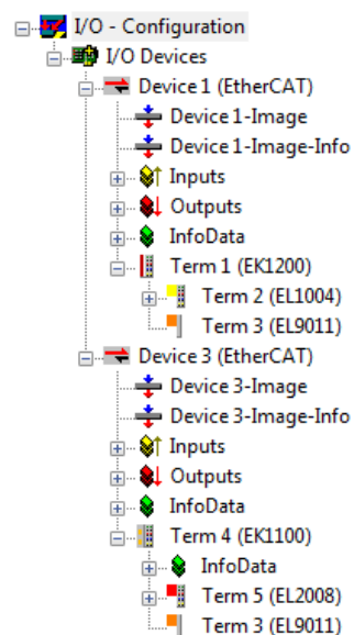
附图 49: TwinCAT 2系统管理器中的配置映射
