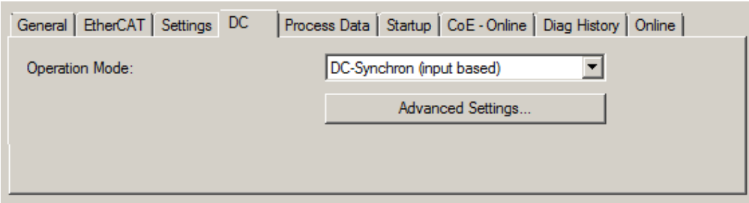
附图 140: “DC” 选项卡（分布时钟）
