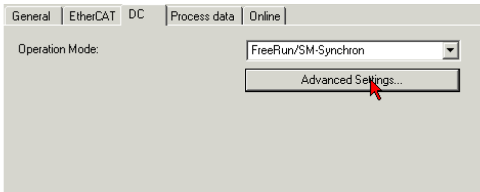
附图 157: DC 选项卡 (分布式时钟)
