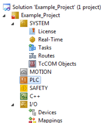
附图 63: 在项目文件夹资源管理器中新建TwinCAT3项目
