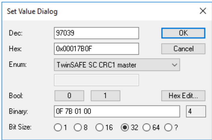
附图 41: 输入安全地址和CRC
