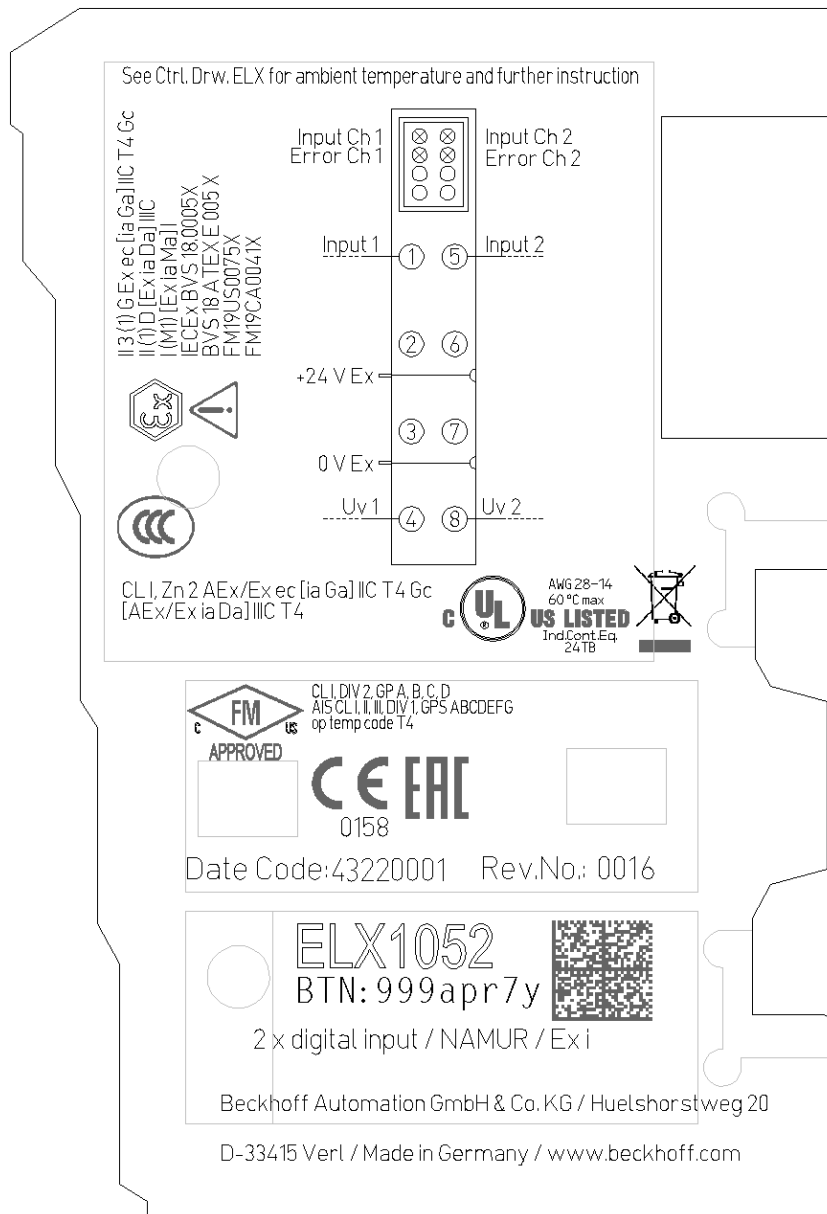
附图 1: ELX1052, 日期代码 43220001, BTN 999apr7y 和标识 für ATEX、IECEX 和 cFMus
