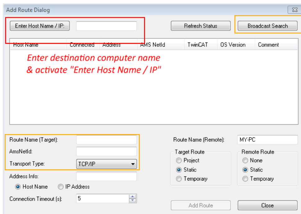
附图 65: 为TwinCAT系统管理器指定访问的PLC：选择目标系统
