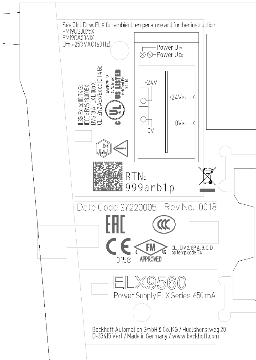
附图 2: ELX9560, 日期代码 37220005, BTN 999arb1p 和标识 für ATEX、IECEx 和 cFMus
