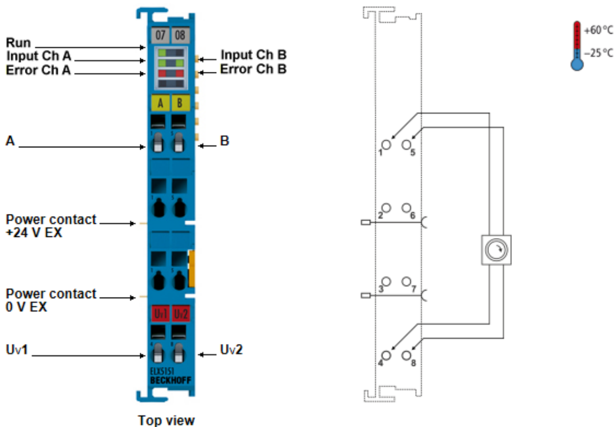
附图 6: ELX5151 - 单通道增量式编码器接口, NAMUR, 32 位, Ex i
