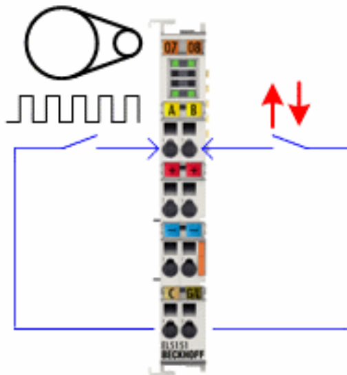
附图 31: ELX5151 - 计数器连接原理
