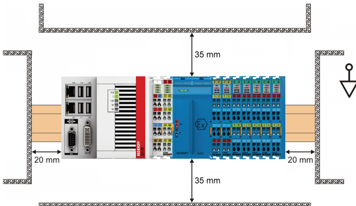
附图 16: 安装位置和最小距离
