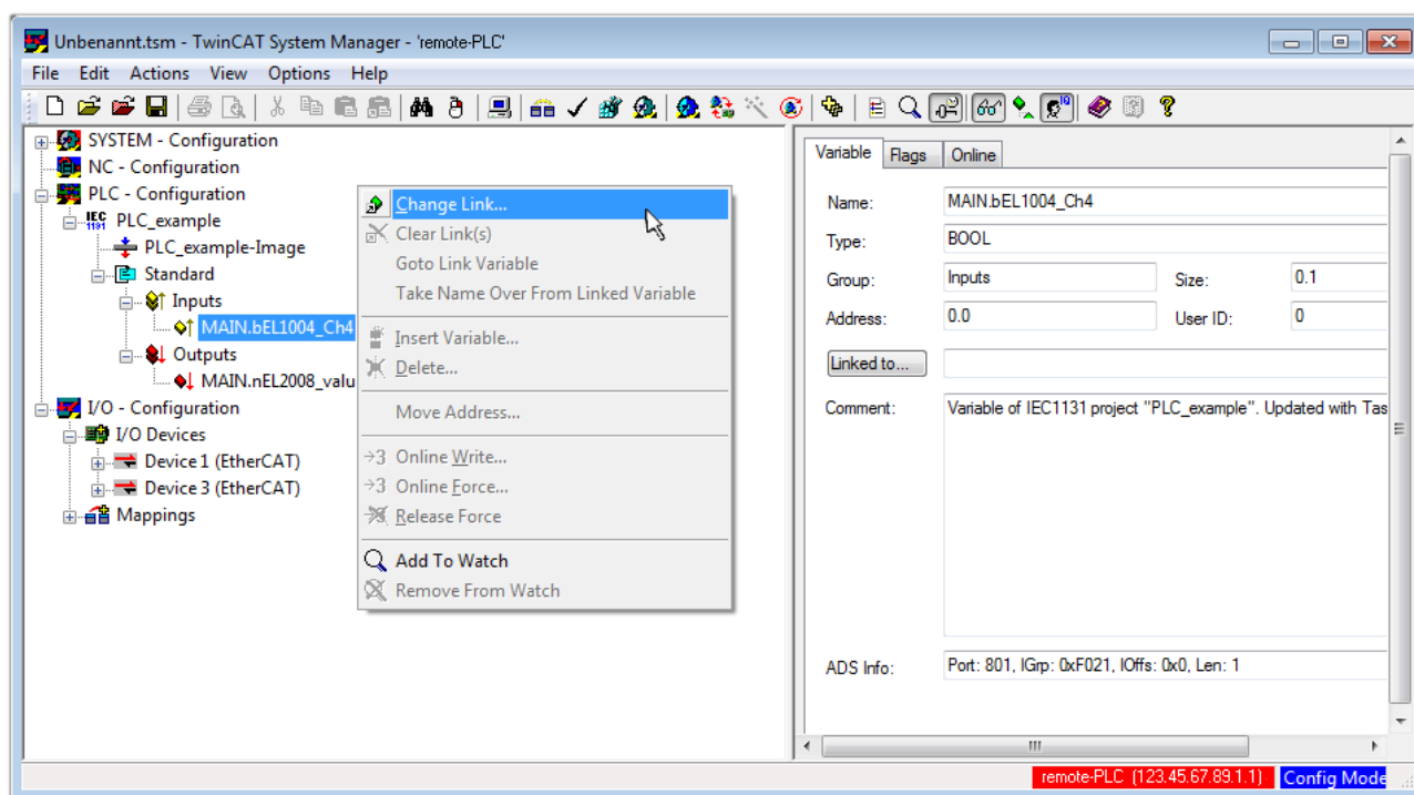
附图 55: 在PLC变量和过程对象之间建立联系
