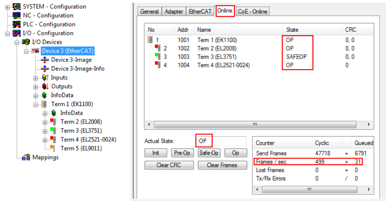
附图 123: 在线显示示例
