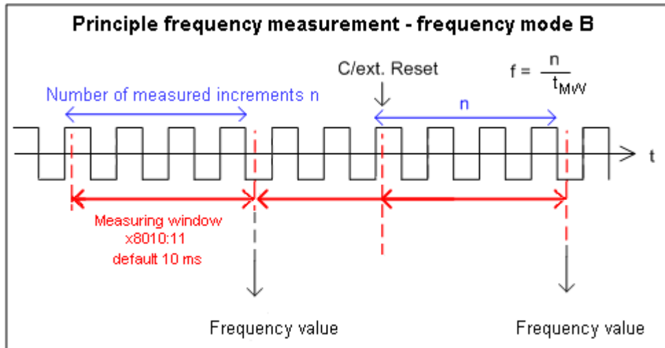
附图 30: 频率测量原理--频率模式 B
