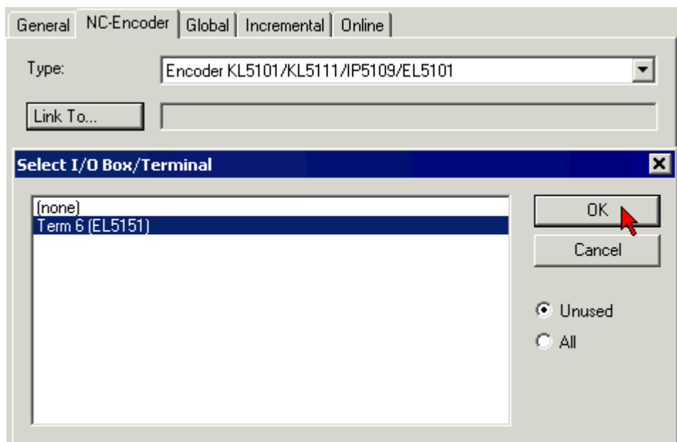
附图 155: 选择和确认一个编码器端子模块
