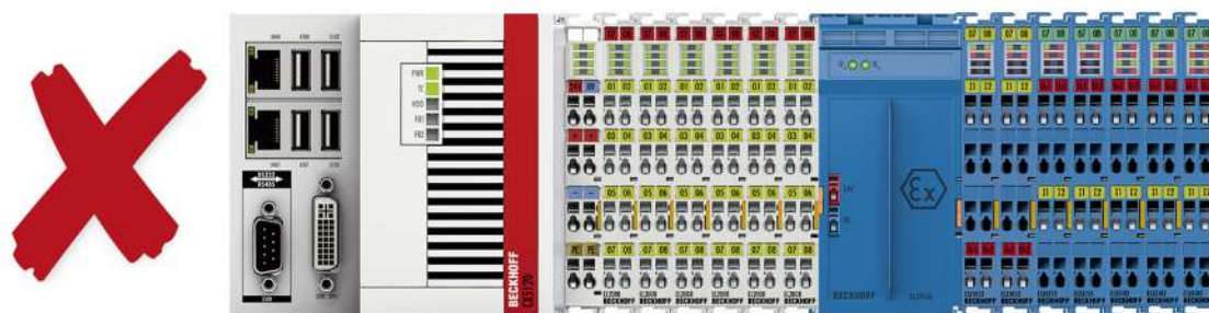
附图 15: 非法的安装 - 缺少 ELX9012 总线终端盖板。
