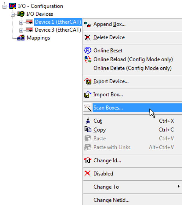
附图 50: 读取连接到设备的单个终端
