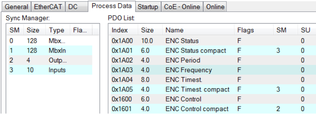
附图 26: ELX5151 - 参数化
