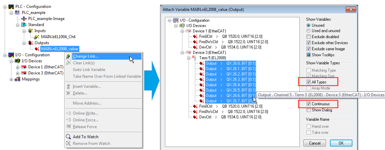
附图 57: 同时选择几个PDO: 激活“连续”和“所有类型”
