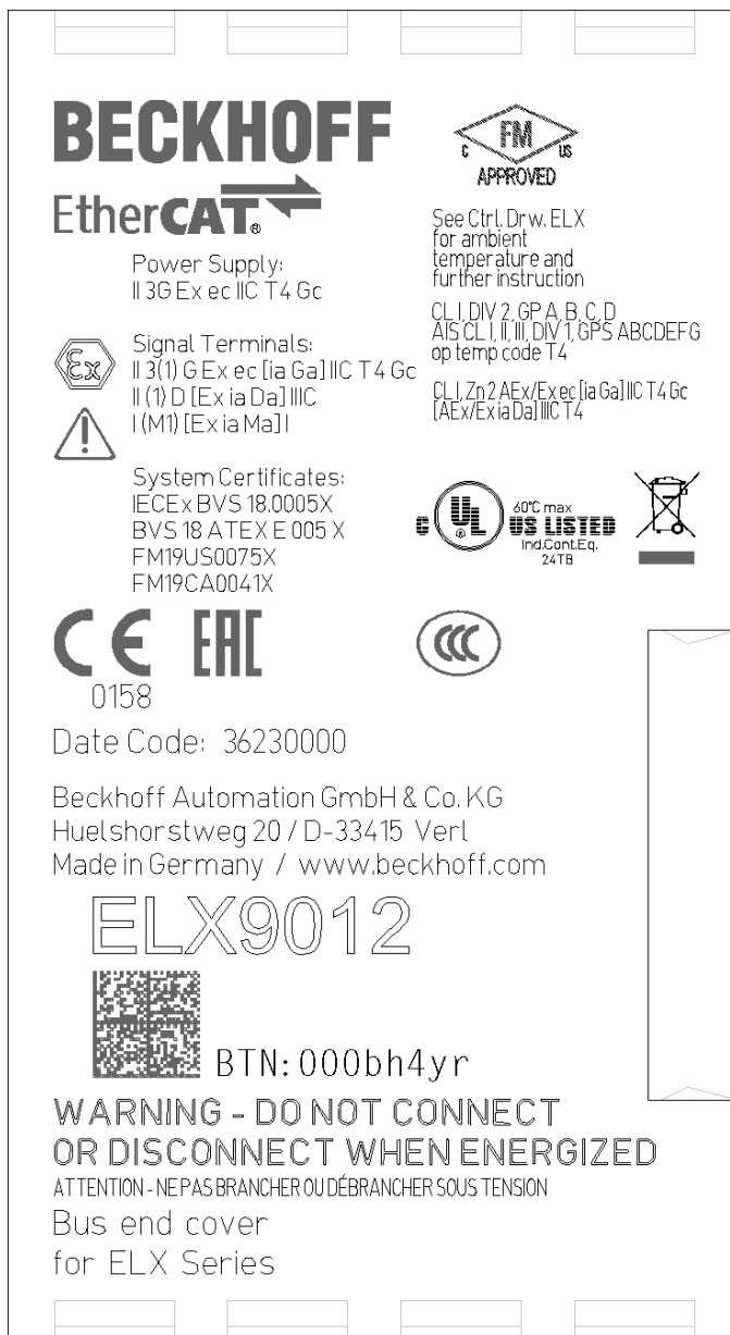
附图 3: ELX9012, 日期代码 36230000, BTN 000bh4yr 和标识 für ATEX、IECEX 和 cFMus
