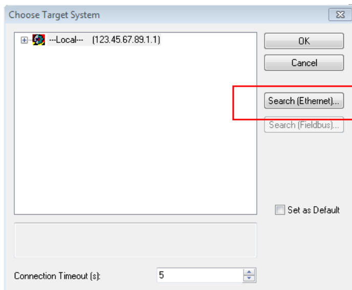
附图 45: 选择目标系统
