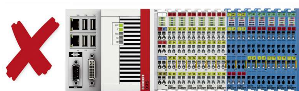
附图 12: 非法的安裝 - 缺少 ELX9560 电源端子模块。
