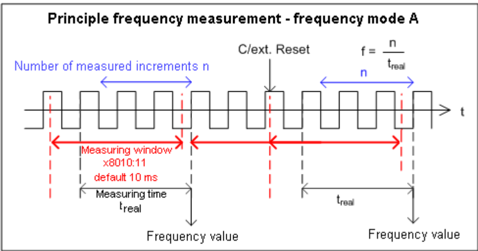
附图 29: 频率测量原理--频率模式 A
