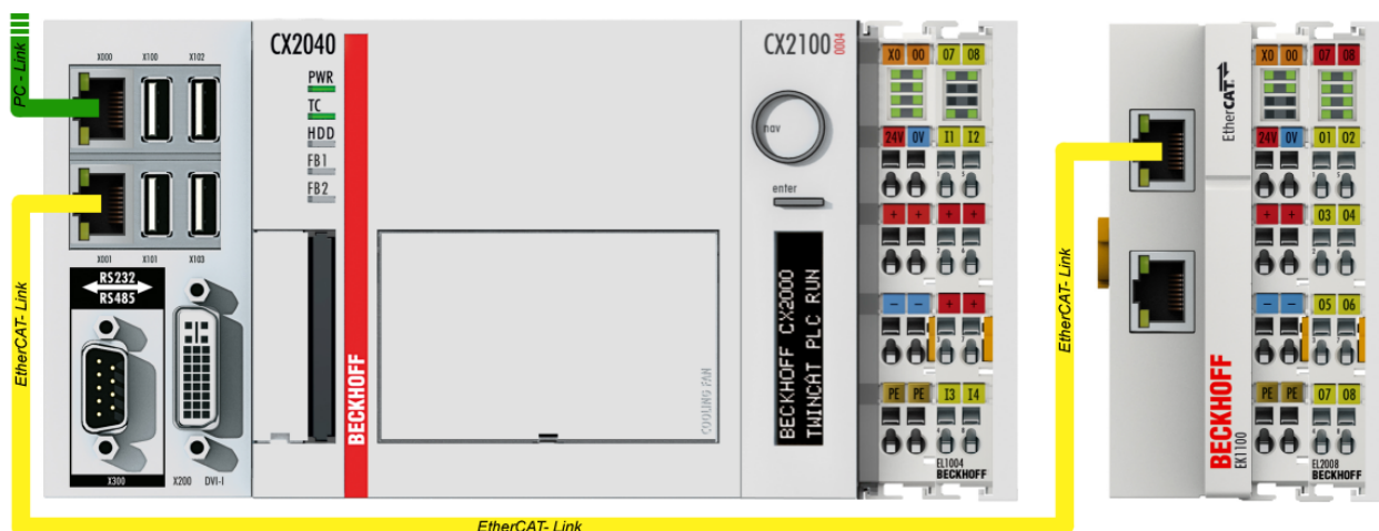
附图 43: 控制配置，带嵌入式电脑、输入（EL1004）和输出（EL2008）
