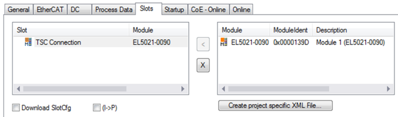
附图 33: 在组件下添加TwinSAFE SC过程数据，如EL5021-0090
