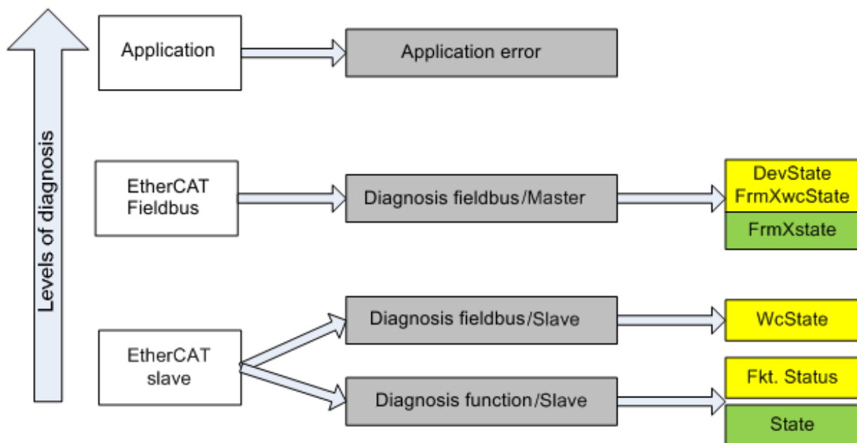
附图 141: 选择 EtherCAT 从站的诊断信息
