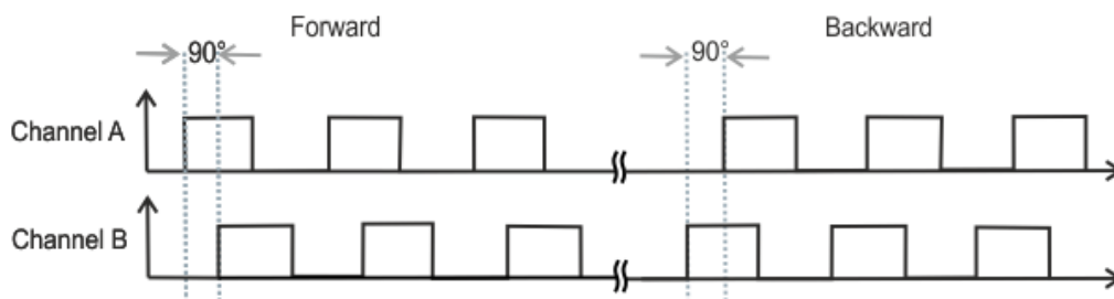
附图 23: 正交解码器
