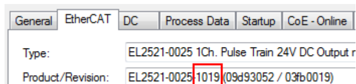
附图 116: 检测修订版本-1019 的 EtherCAT 端子
