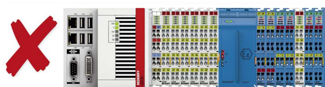
附图 13: 不允许的安裝 - ELX 端子模块网段中的端子模块不属于 ELX 系列
