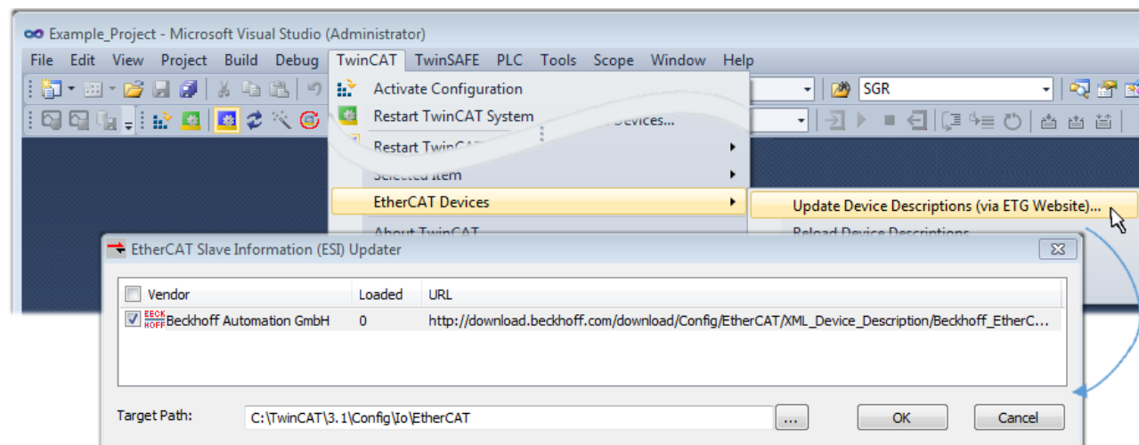
附图 99: 使用ESI Updater (TwinCAT 3)
