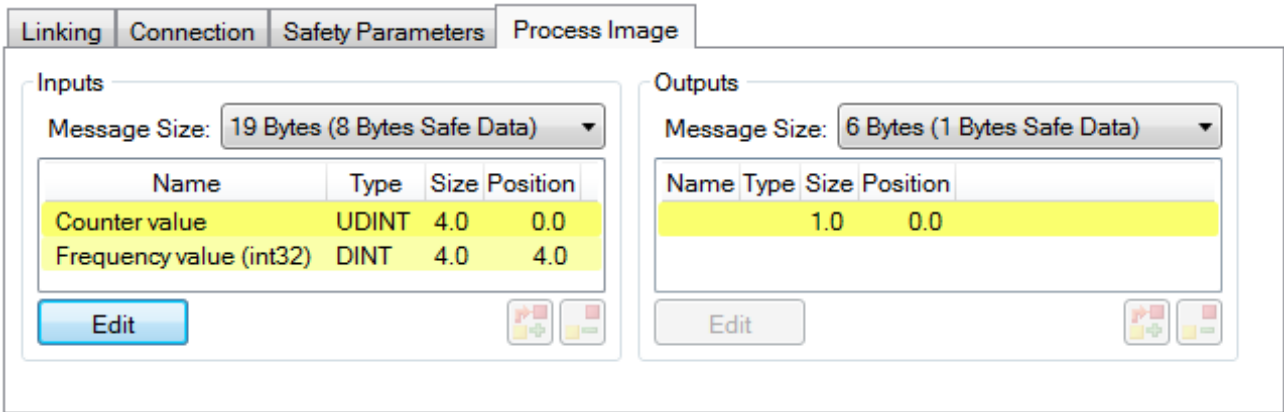
附图 38: 选择过程数据大小和过程数据
