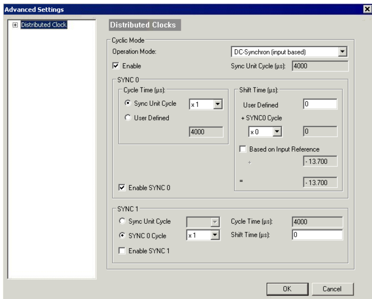
附图 158: ELX5151 - 高级设置，分布式时钟 (DC)
