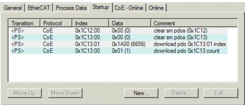
附图 136: “Startup (启动)” 选项卡
