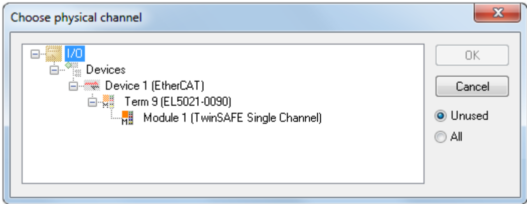
附图 36: 创建一个与TwinSAFE SC终端的连接
