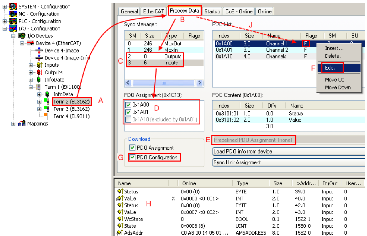
附图 135: 配置过程数据
