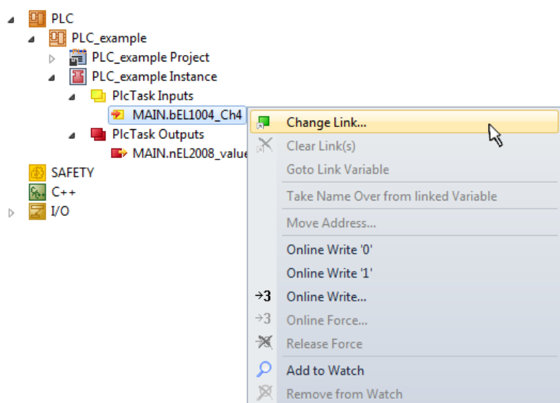
附图 75: 在PLC变量和过程对象之间建立联系
