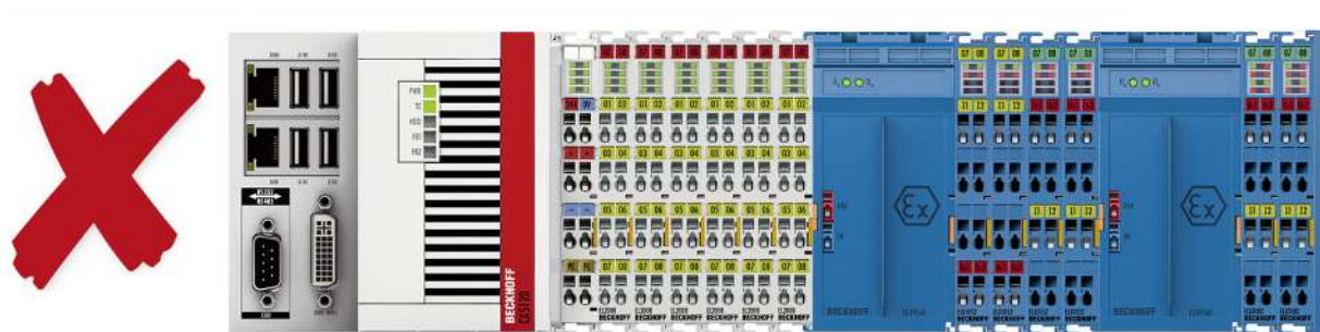
附图 14: 不允许的安装 - ELX 端子模块网段中的第二个 ELX9560 电源端子模块没有前端的 ELX9410。
