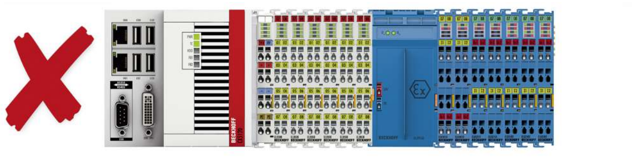
附图 12: 无效安排 - 缺少 ELX9012 总线端盖。
