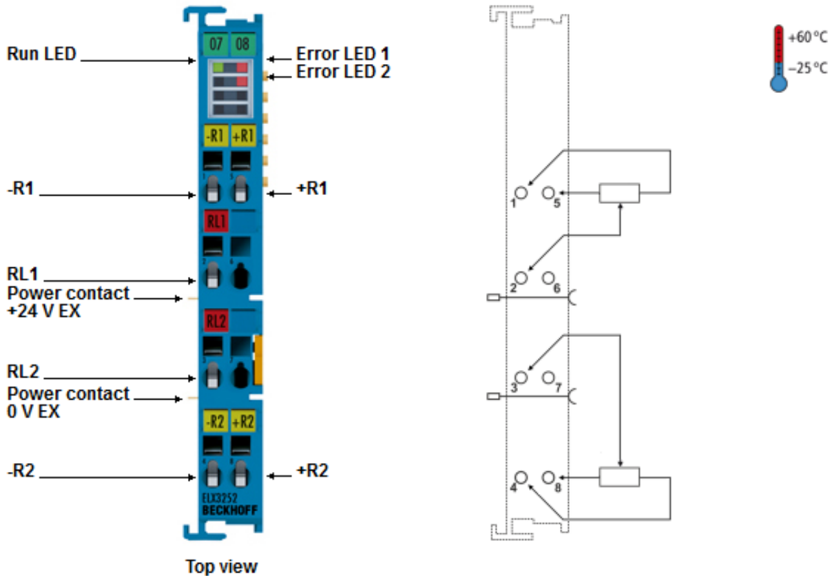
附图 19: ELX3252 - 触点分配
