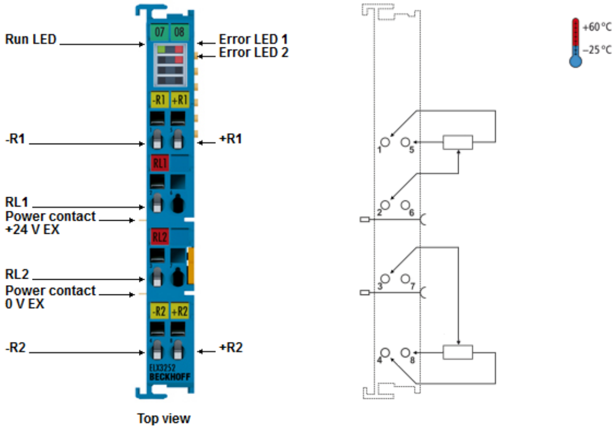
附图 4: ELX3252 - 用于电位计的双通道模拟量输入端子模块，16 位，Ex i
