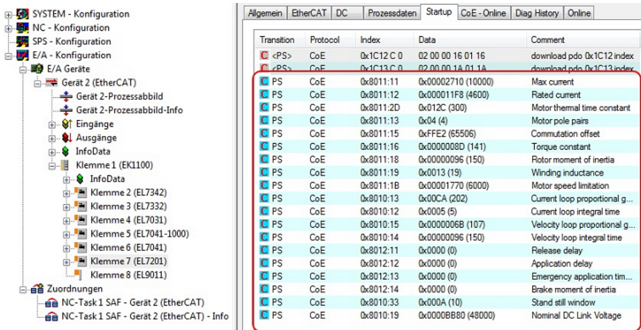
Abb. 113: CoE Parameterbild der Motor XML-Datei
