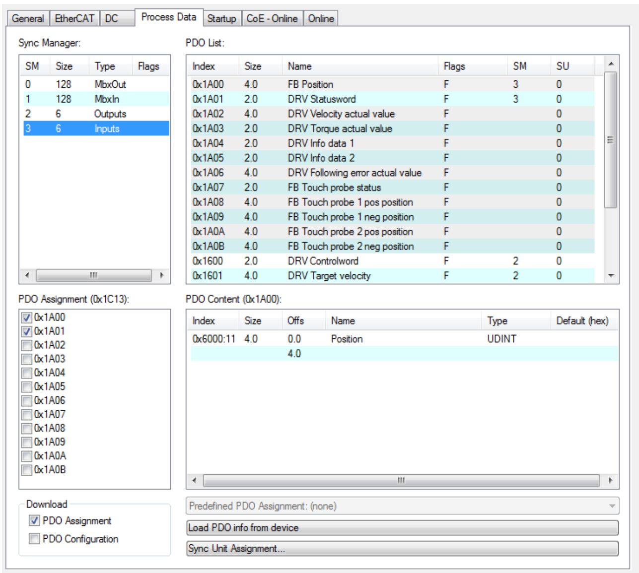
Abb. 161: Karteireiter Prozessdaten SM3, EL72x1-0010 (default)
