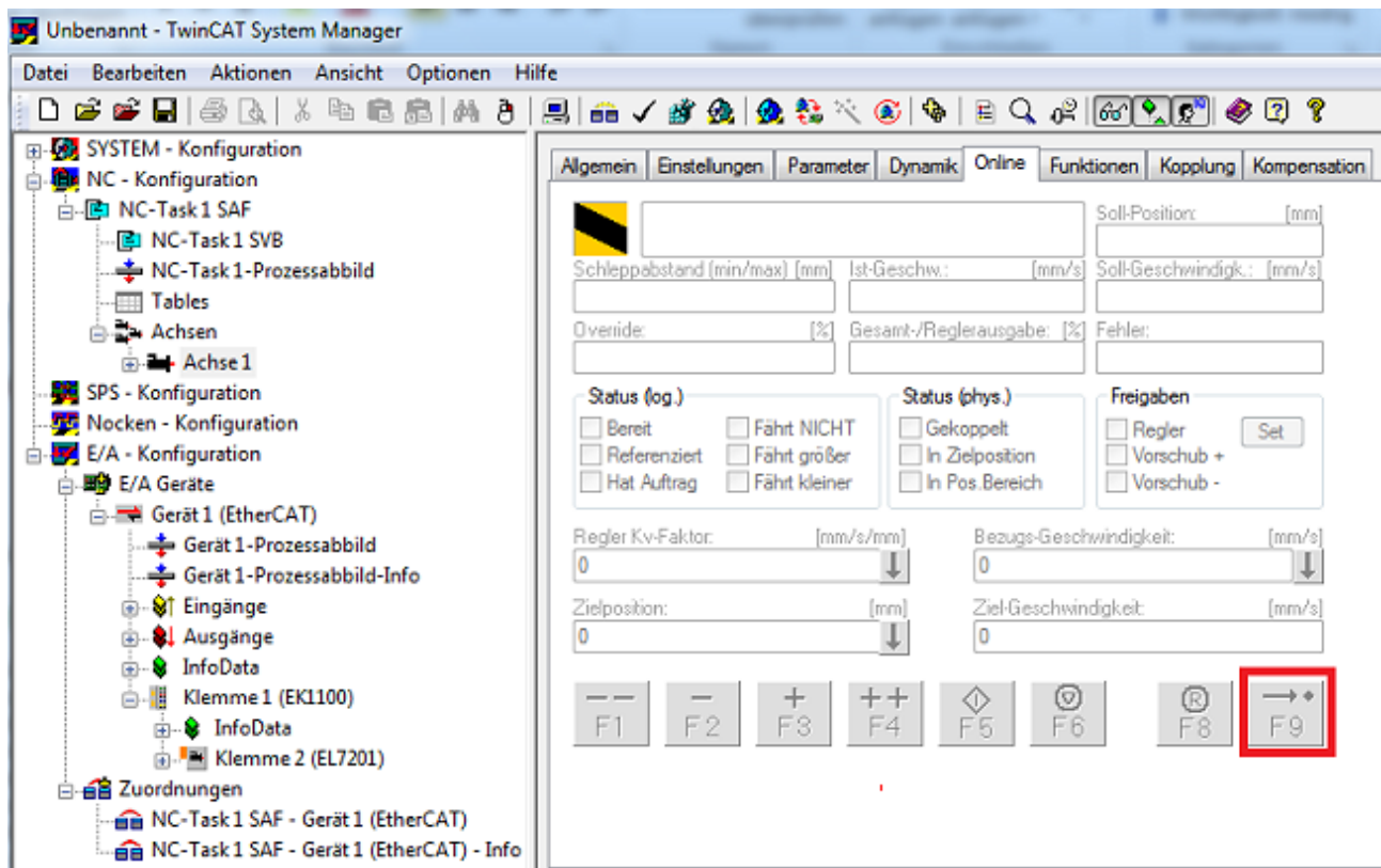
Abb. 126: Online-Homing in der NC
