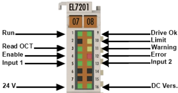
Abb. 33: EL7201-001x - LEDs
