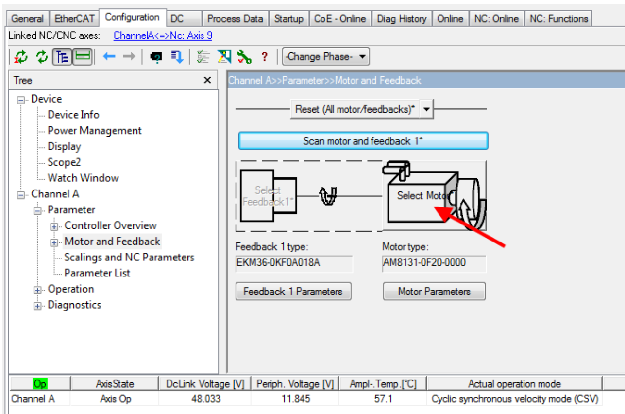
Abb. 105: Auswahl des angeschlossenen Motors
