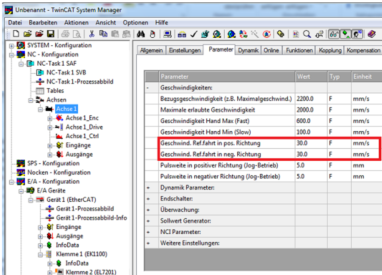
Abb. 130: Einstellung der Referenzgeschwindigkeit
