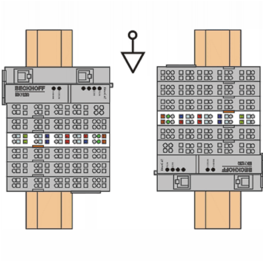
Abb. 27: Weitere Einbaulagen, Beispiel 1
