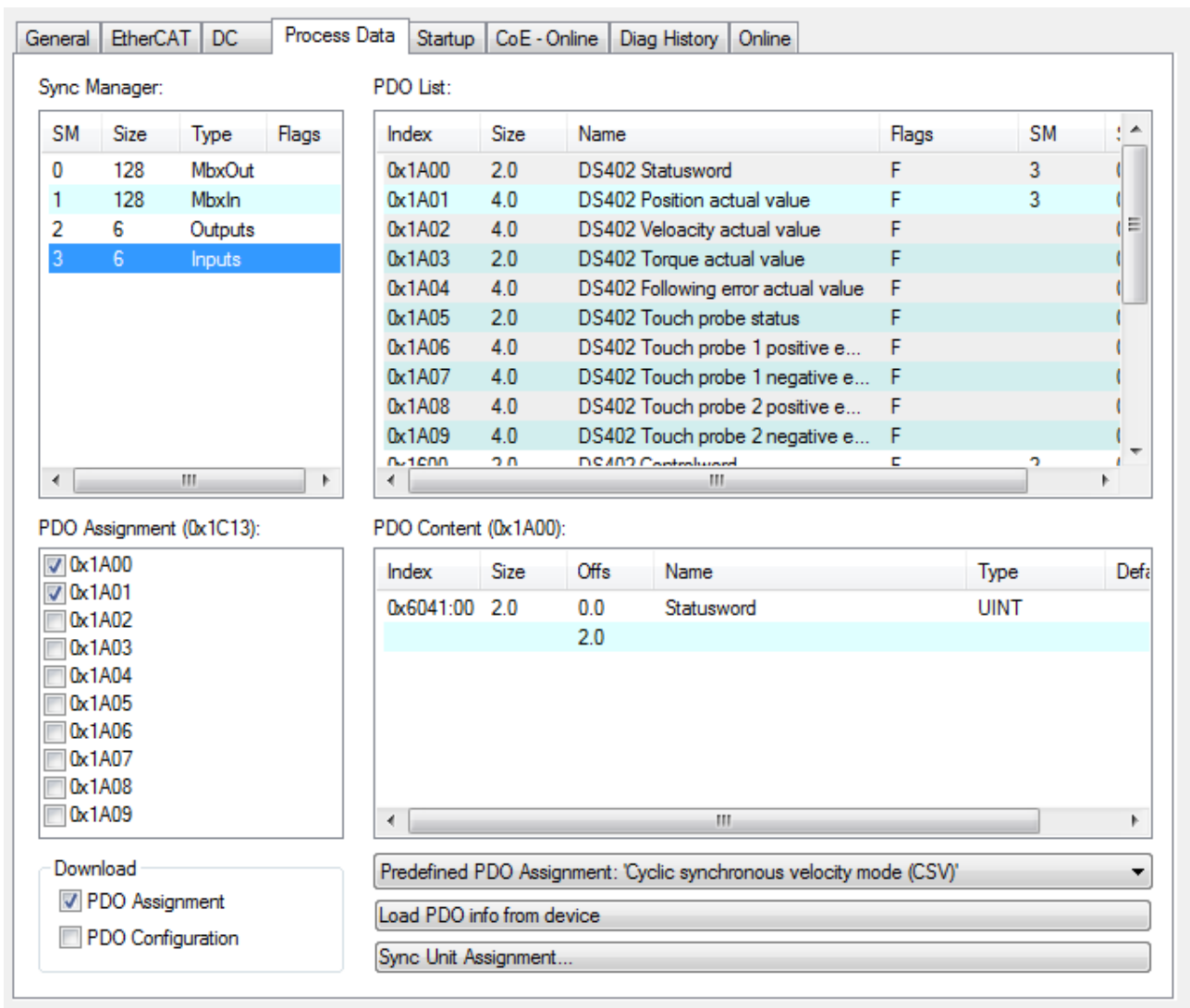
Abb. 164: Karteireiter Prozessdaten SM3, EL72x1-0010 (default)
