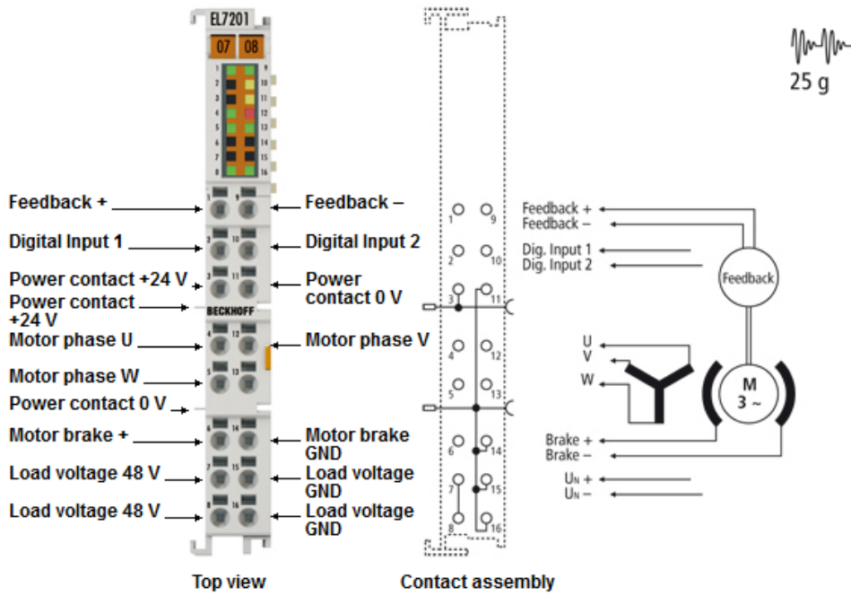
Abb. 4: EL7201-0010
