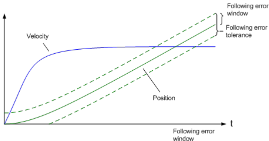
Abb. 159: Schleppfehler über die Zeit
