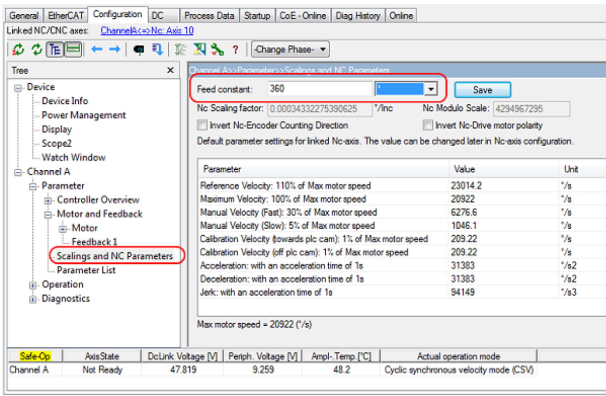
Abb. 108: Anpassung der Skalierung
