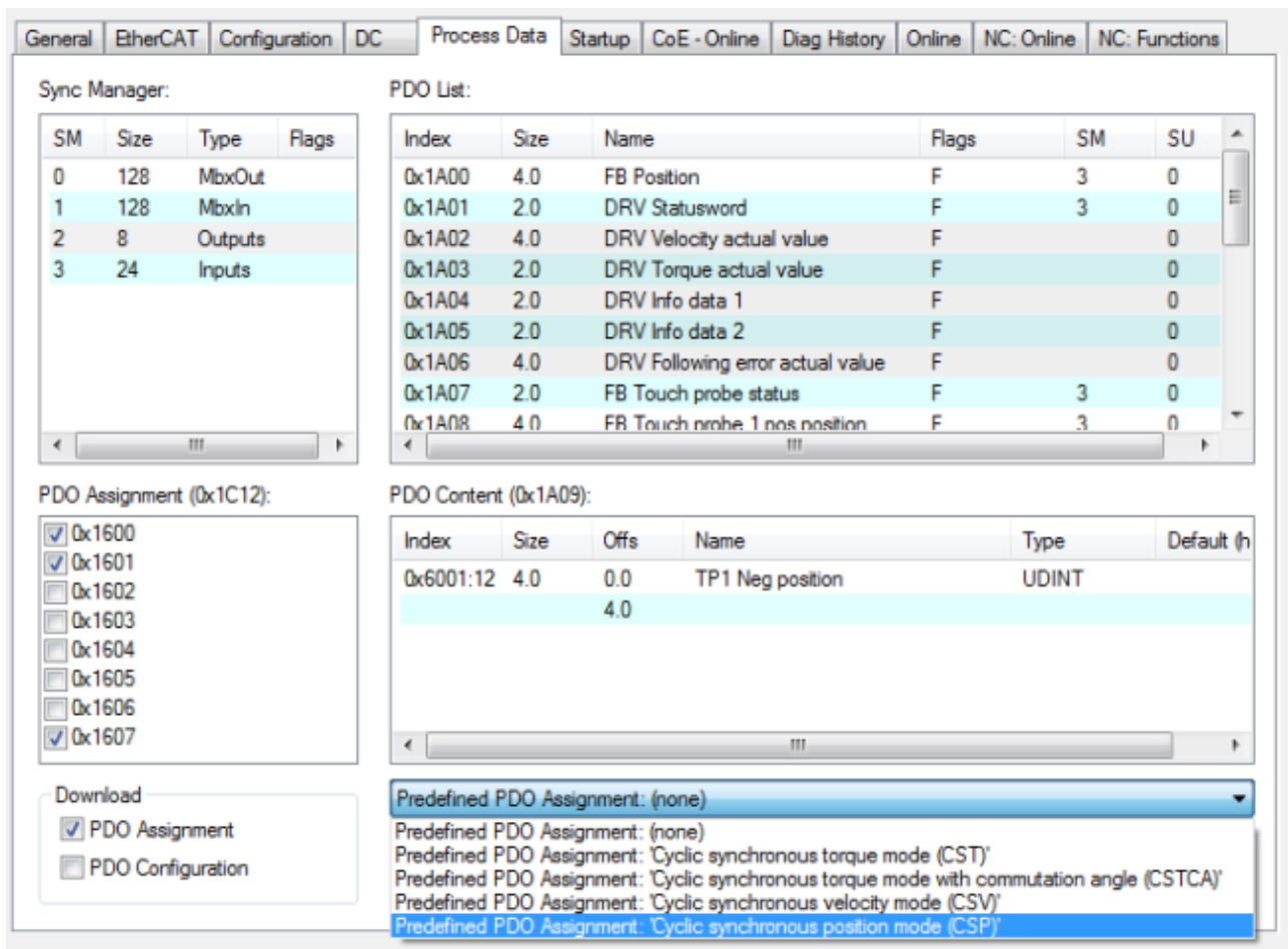
Abb. 155: Predefined PDO Assignment wählen
