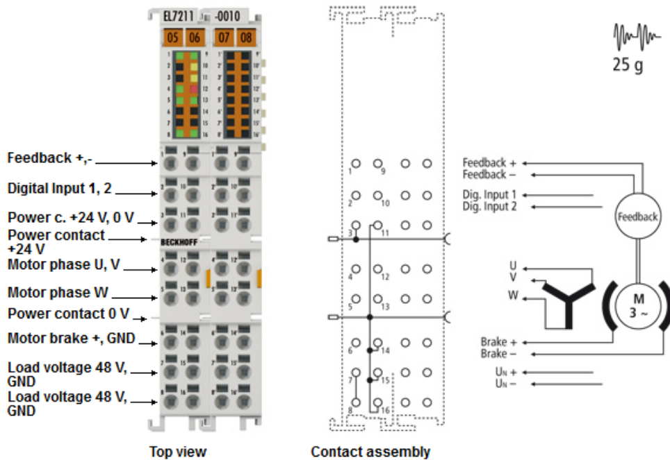
Abb. 36: EL7211-001x - Anschlussbelegung
