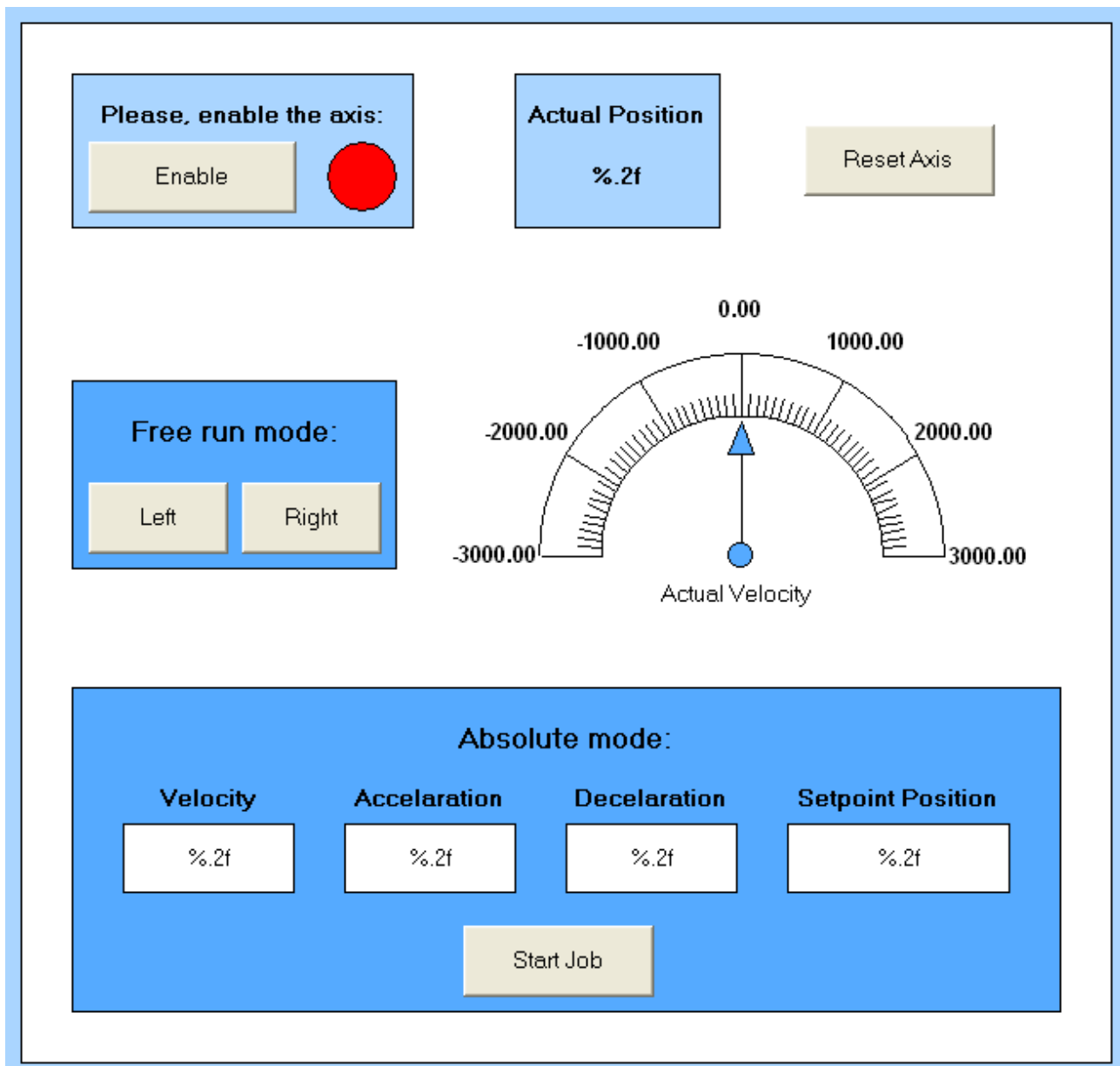
Abb. 122: Visualisierung
