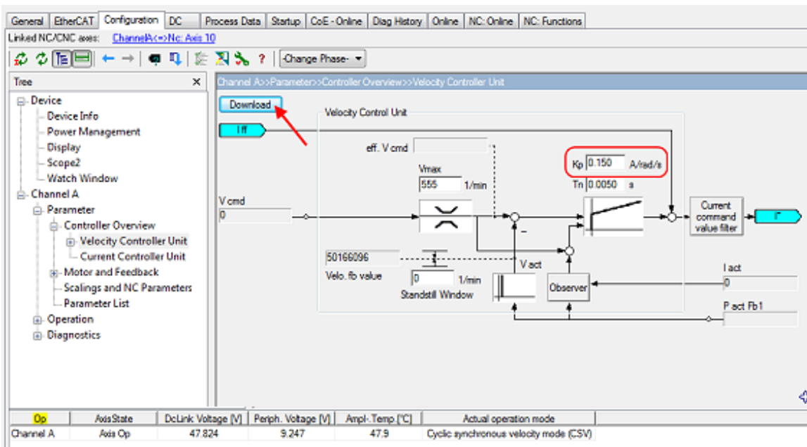
Abb. 110: Anpassung Kp
