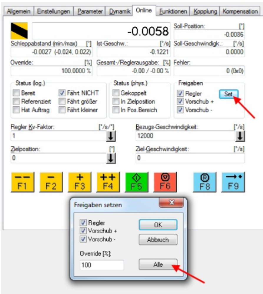
Abb. 140: Achse freigeben
