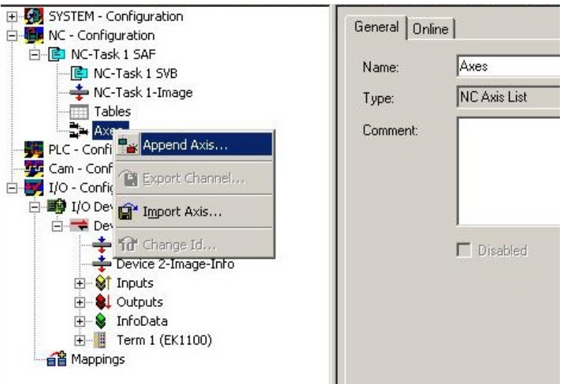
Abb. 98: Auswahl einer neuen Achse
