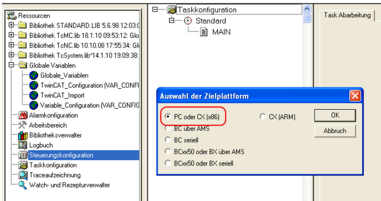
Abb. 115: Auswahl der Zielplattform
