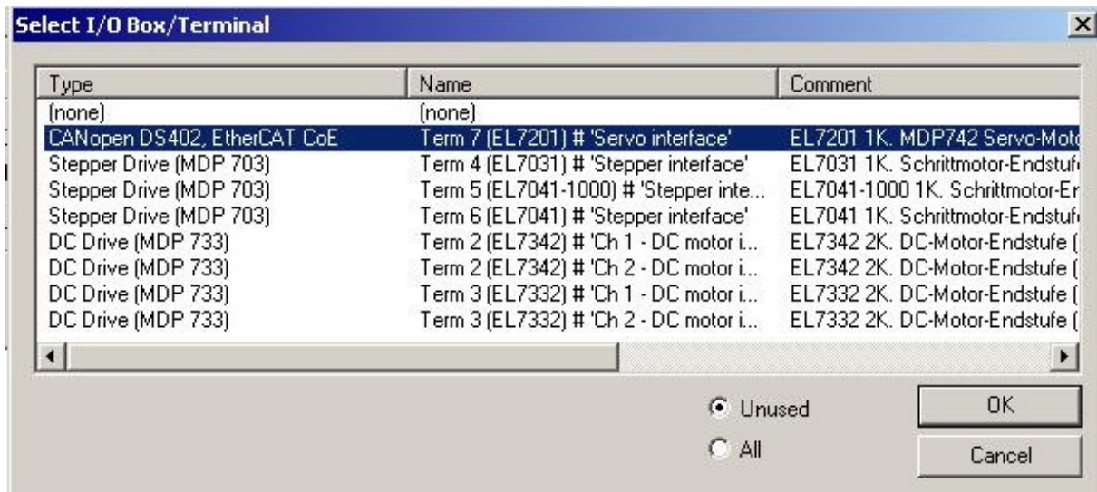
Abb. 101: Auswahl der richtigen Klemme
