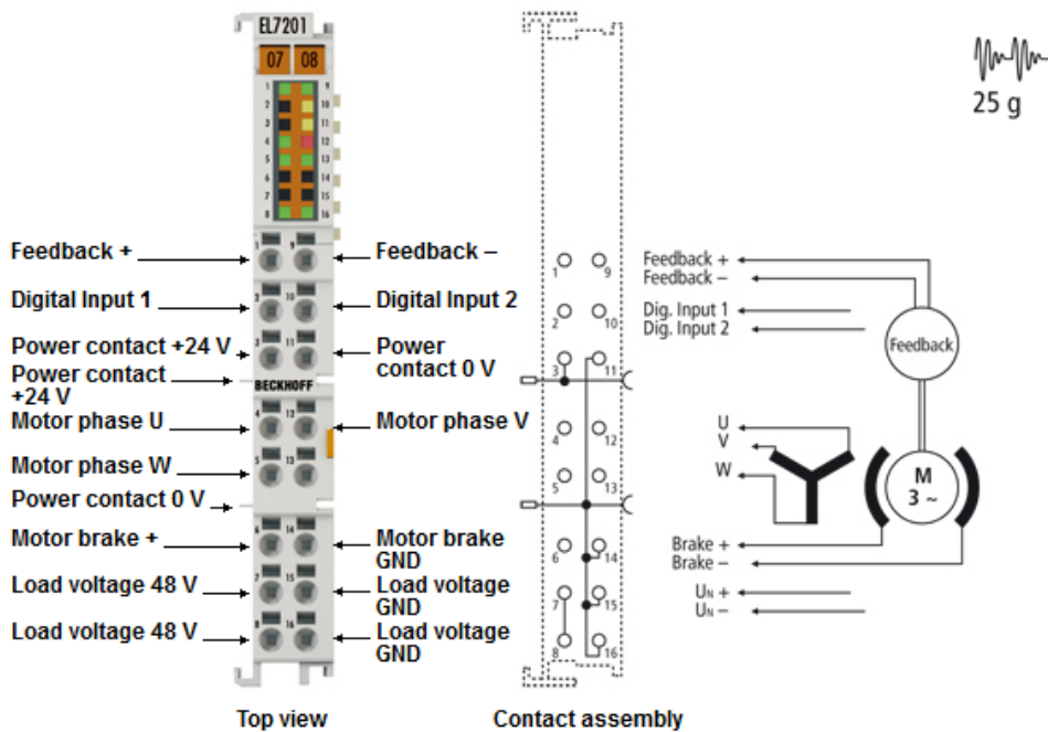
Abb. 34: EL7201-001x - Anschlussbelegung
