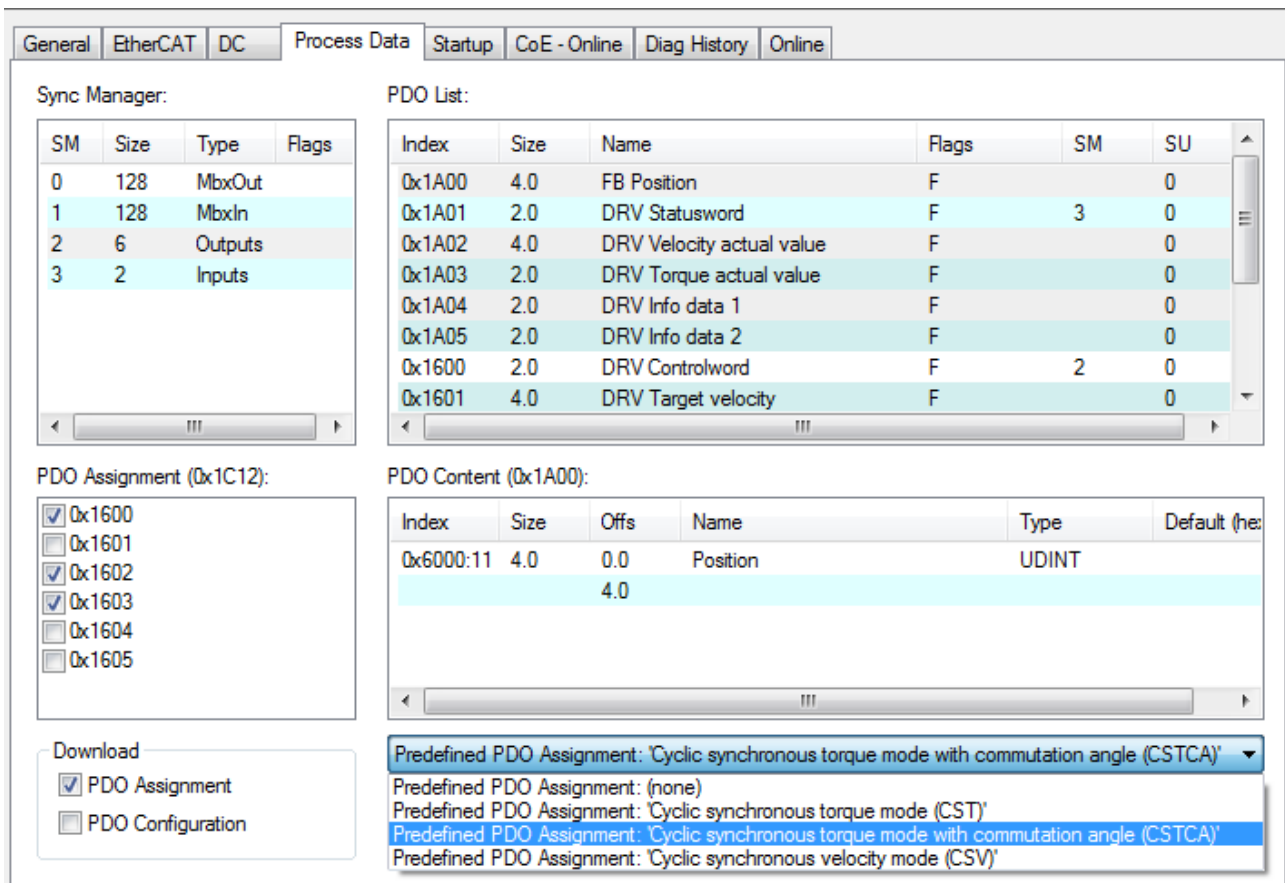
Abb. 151: Predefined PDO Assignment wählen
