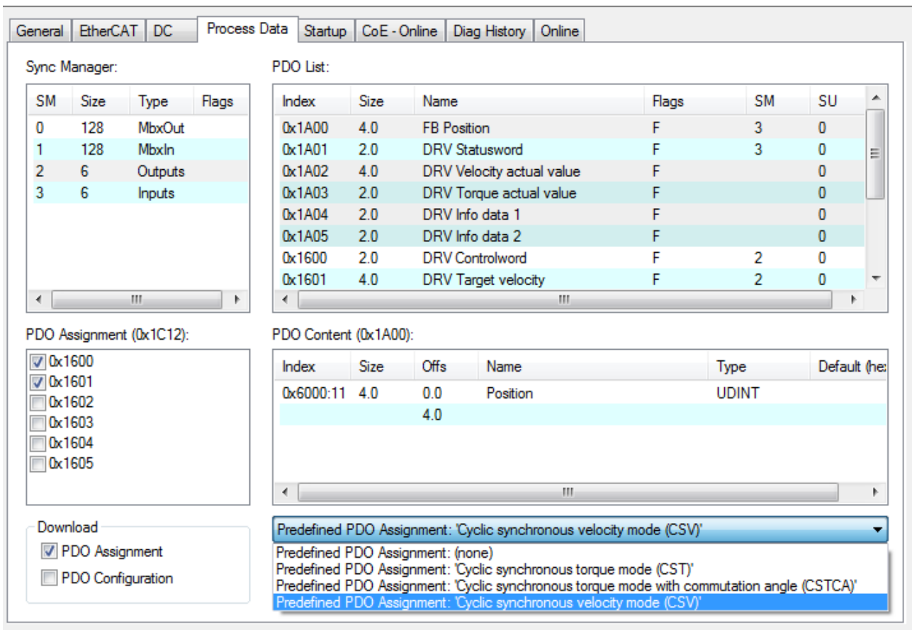
Abb. 143: Predefined PDO Assignment wählen
