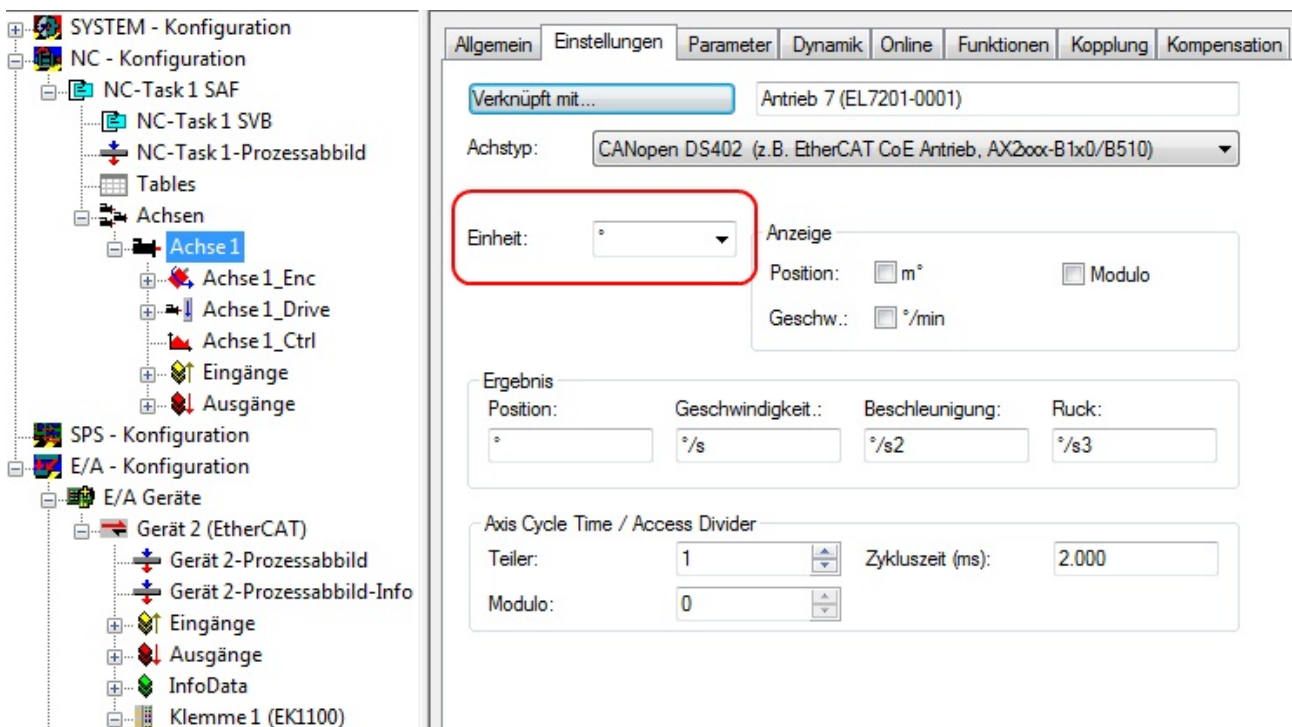
Abb. 133: Definition der Einheit
