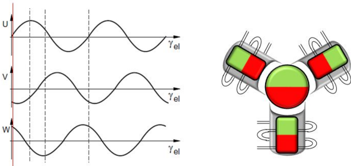
Abb. 6: Drei um 120^\circ verschobenen Spulen eines Synchronmotors
