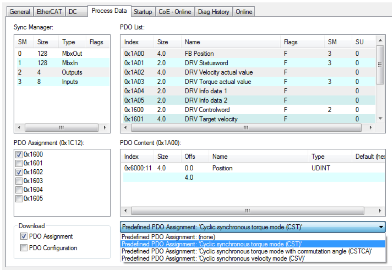
Abb. 147: Predefined PDO Assignment wählen
