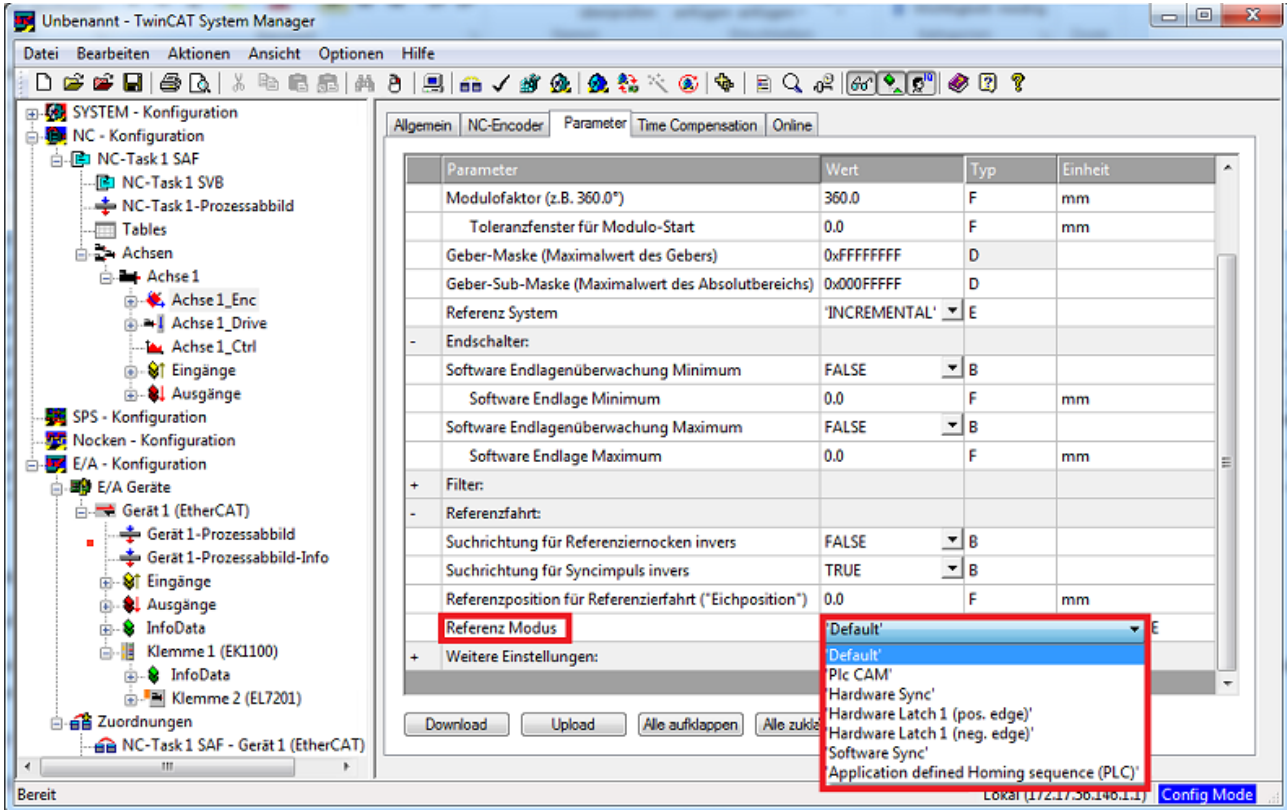
Abb. 129: Auswahl der Referenz Modi in der NC
