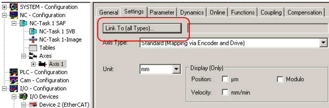
Abb. 100: Verknüpfung der Achse mit der Klemme
