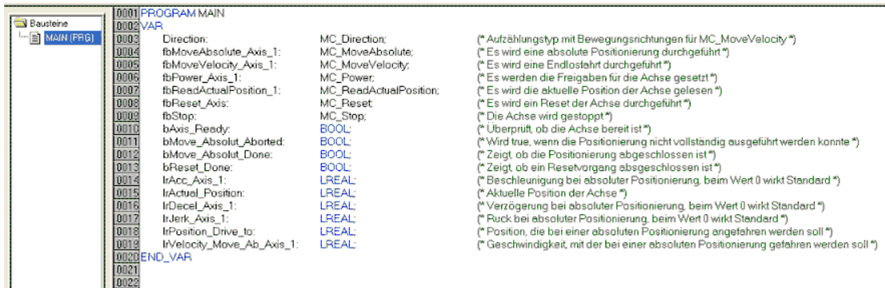
Abb. 120: Lokale Variablen
