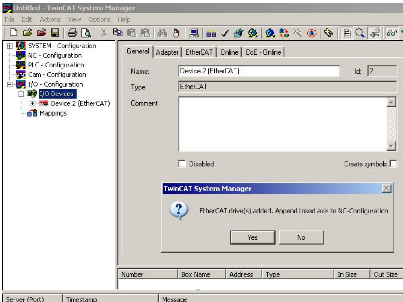
Abb. 96: Achse erkannt
