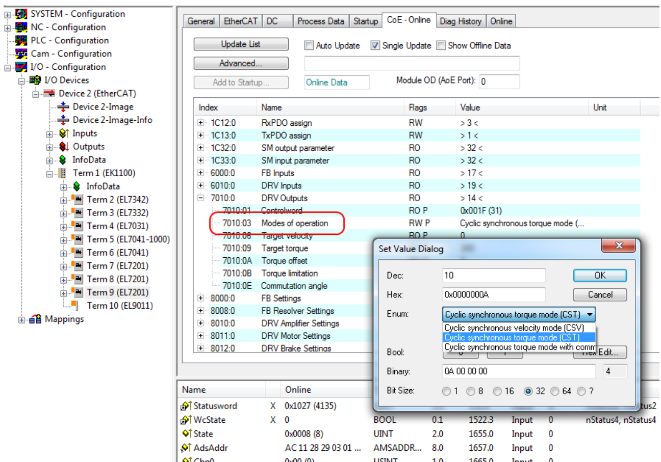
Abb. 146: Auswahl Betriebsart
