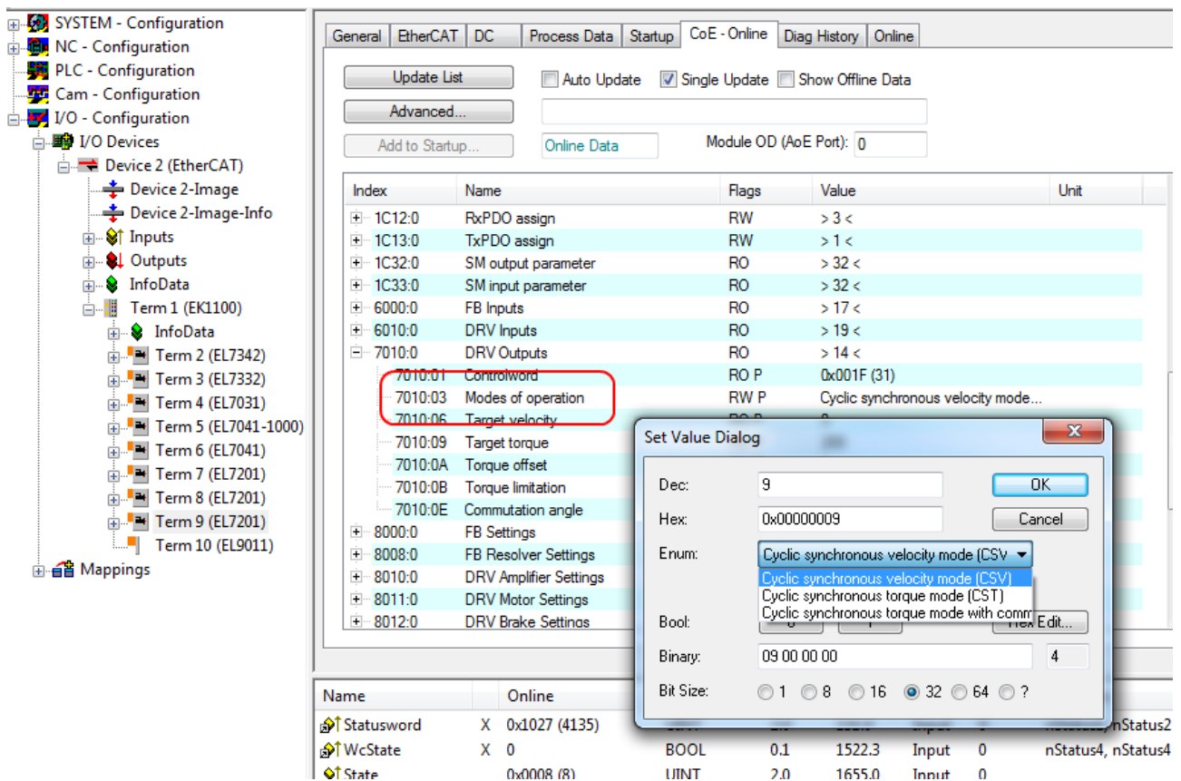
Abb. 142: Auswahl Betriebsart
