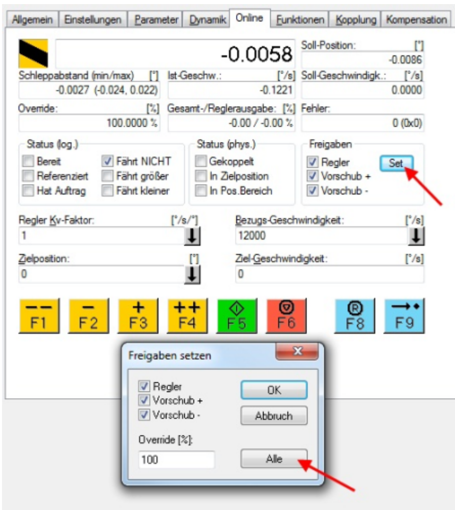
Abb. 156: Freigaben setzen
