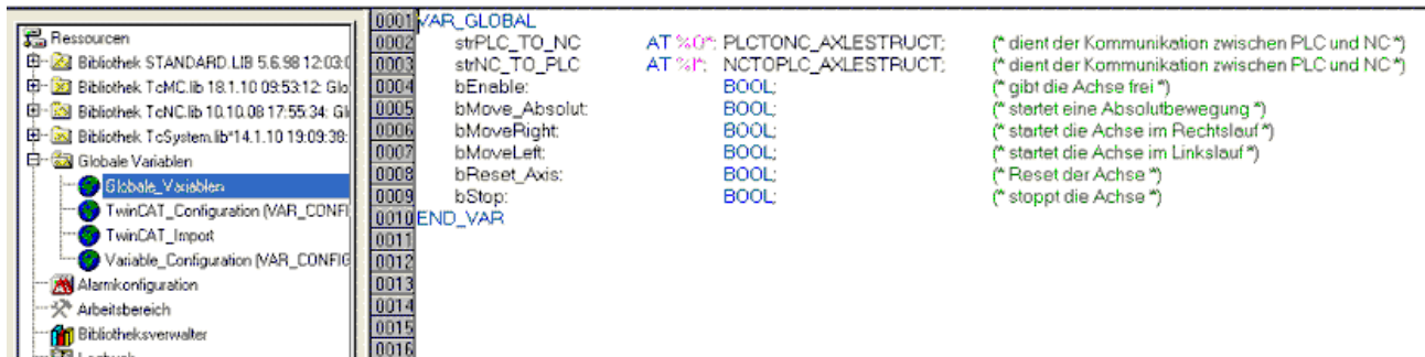
Abb. 119: Globale Variablen
