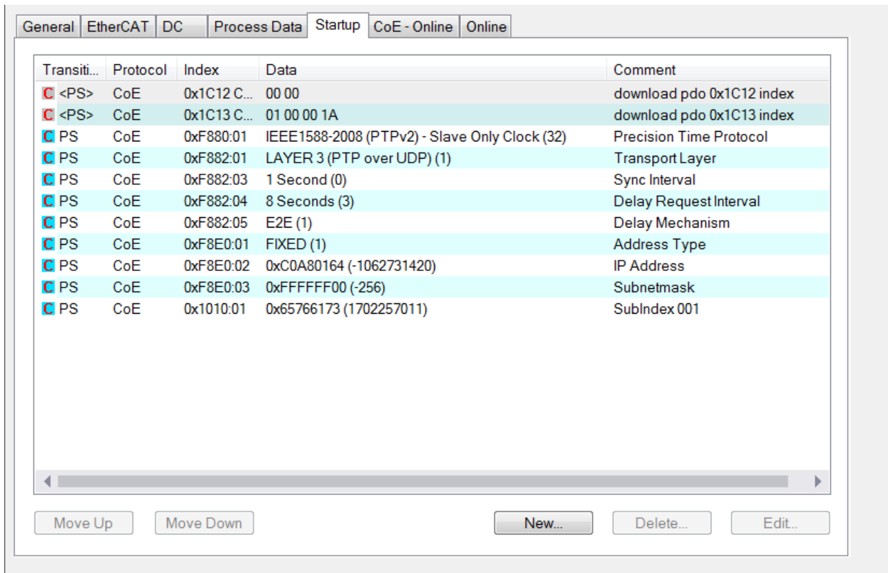
Abb. 84: StartUp-Liste
