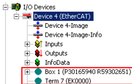
Abb. 58: Fehlerhafte Erkennung
