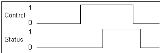
Abb. 137: Zyklischer Betrieb mit Handshake
