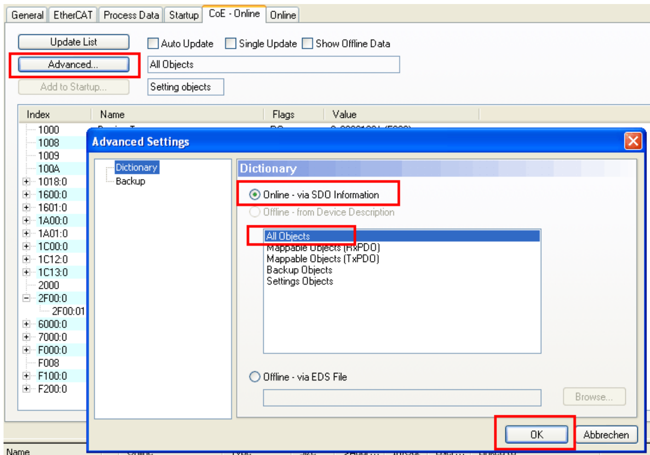
Abb. 143: Vollständiger Reload des CoE-Verzeichnisses
