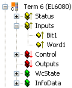
Abb. 136: Unzulässige Konfiguration bis TwinCAT b2.10 b1330
