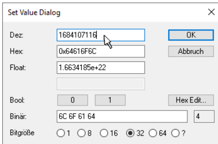
Abb. 159: Eingabe des Restore-Wertes im Set Value Dialog
