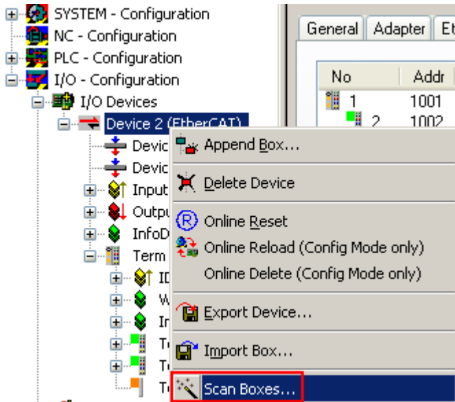
Abb. 147: Rechtsklick auf das EtherCAT-Gerät bewirkt das Scannen des unterlagerten Feldes
