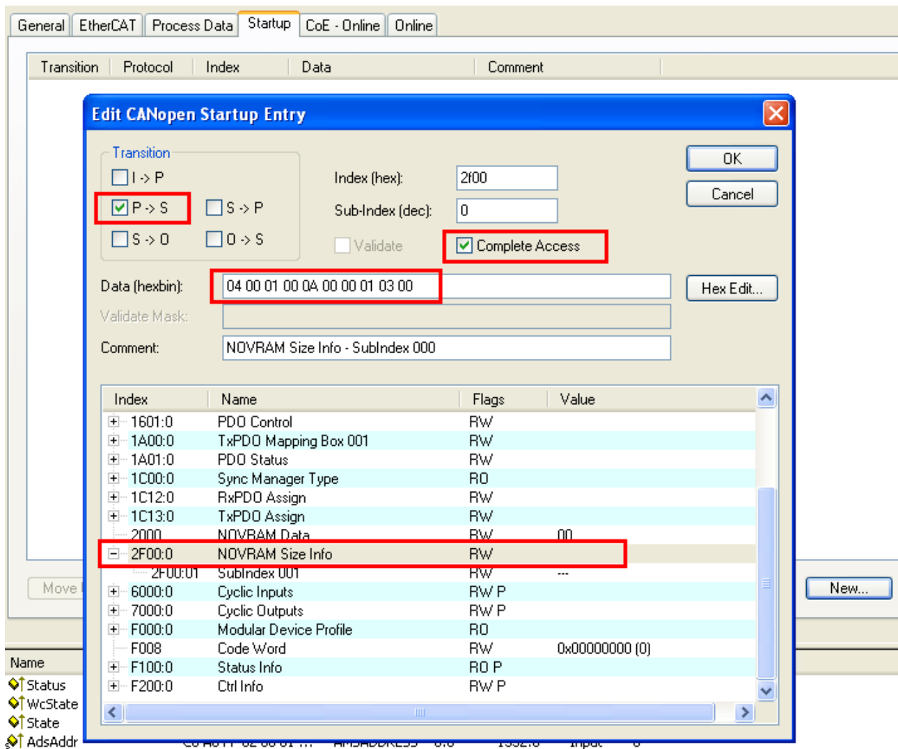
Abb. 140: Definition des StartUp-Eintrages
