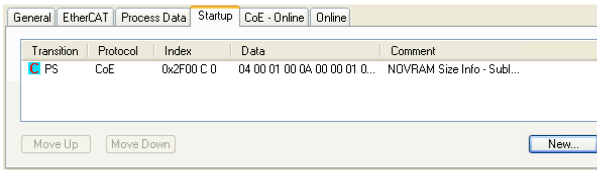
Abb. 141: Neuer StartUp-Eintrag der EL6080
