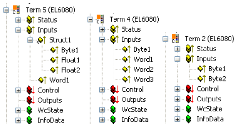
Abb. 135: Zulässige Konfiguration
