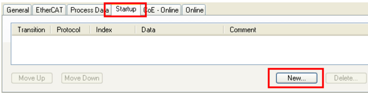
Abb. 139: Hinzufügen eines neuen StartUp-Eintrages
