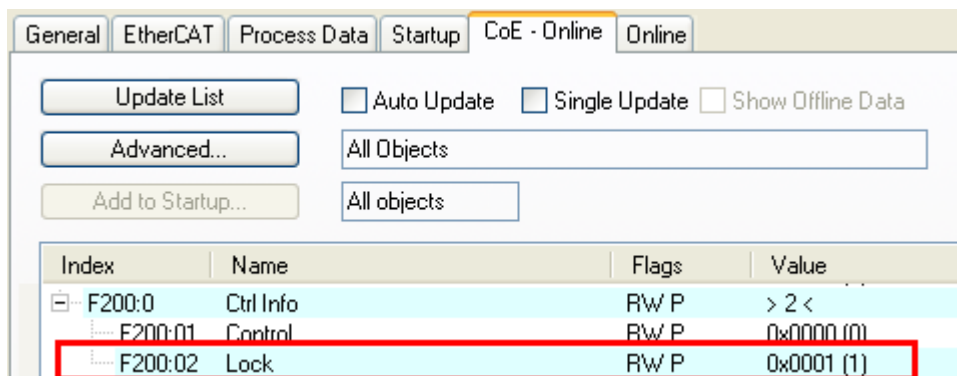
Abb. 145: Lock im CoE
