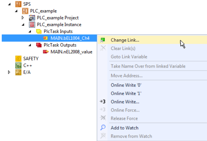
Abb. 57: Erstellen der Verknüpfungen PLC-Variablen zu Prozessobjekten
