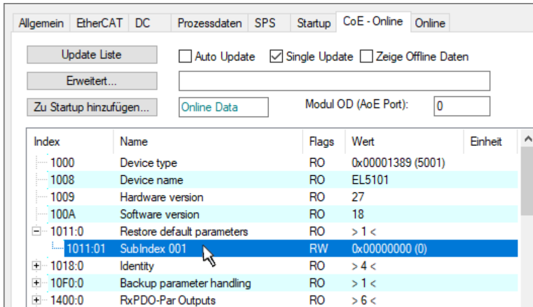
Abb. 158: Auswahl des PDO Restore default parameters
