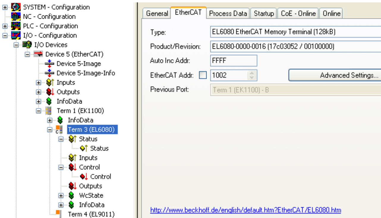
Abb. 133: Default Prozessabbild der EL6080 nach dem Einfügen
