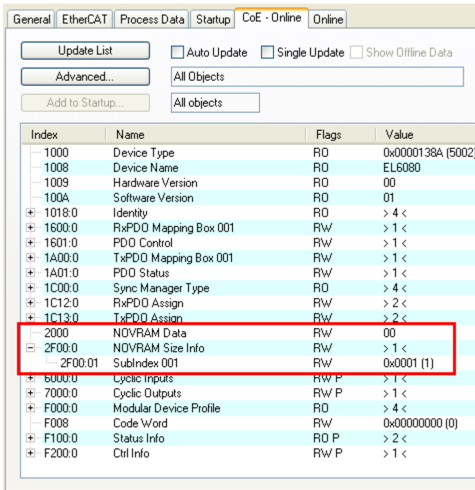
Abb. 138: Beliebiger Startzustand der EL6080
