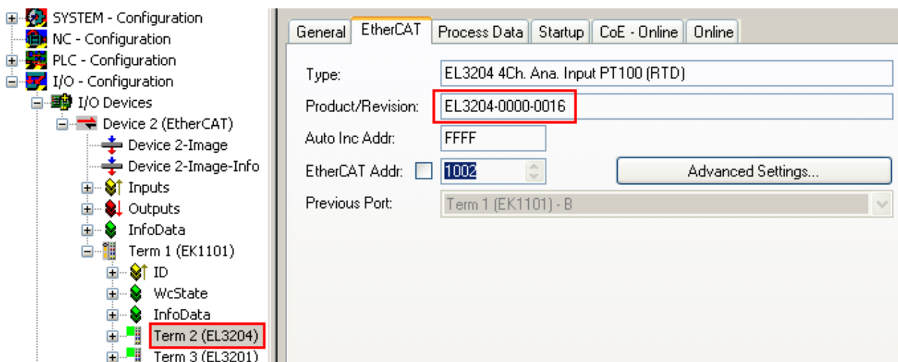
Abb. 146: Geräteerkennung aus Name EL3204-0000 und Revision -0016
