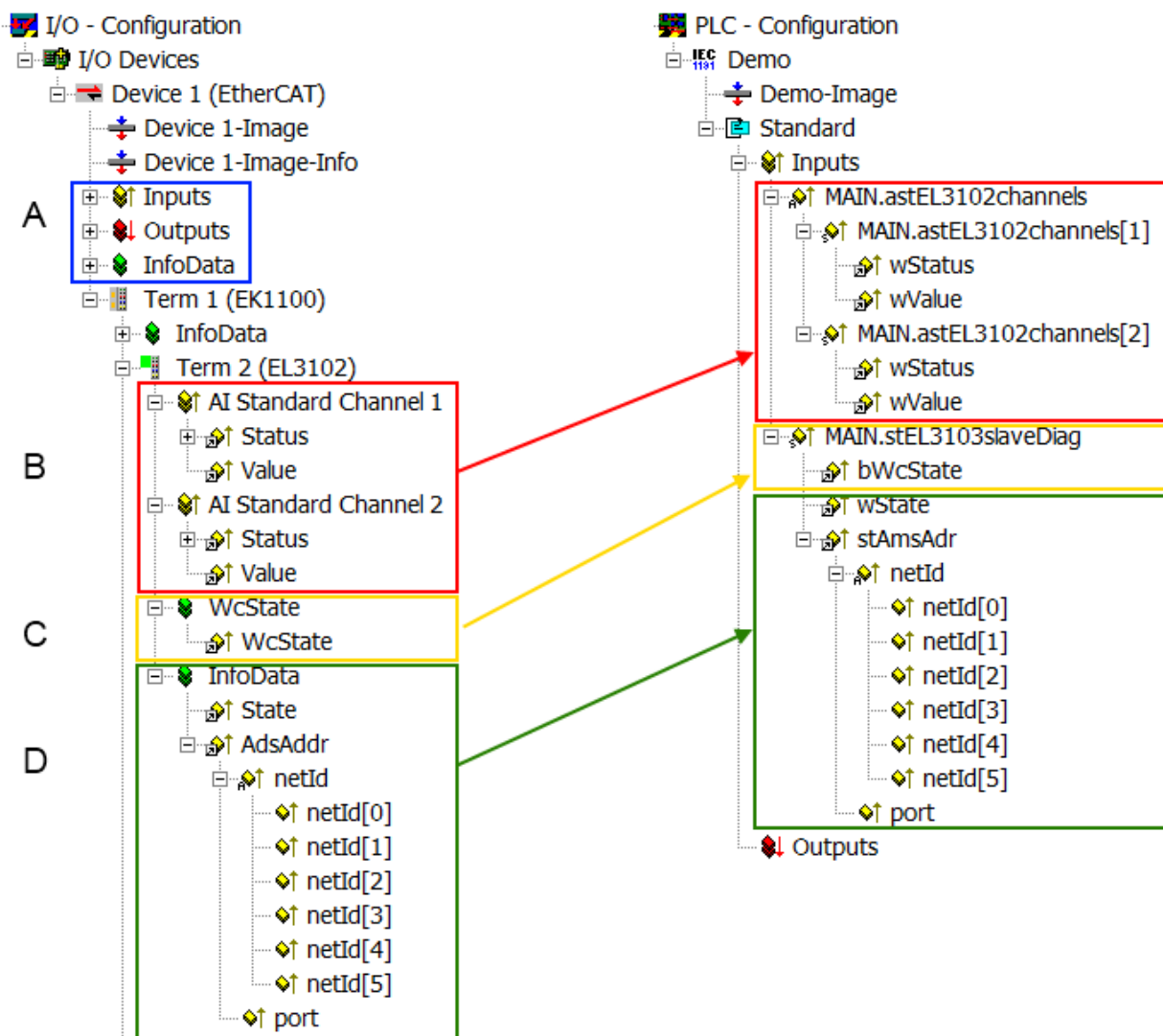
附图 127: PLC 中的 EtherCAT 从站基本诊断
