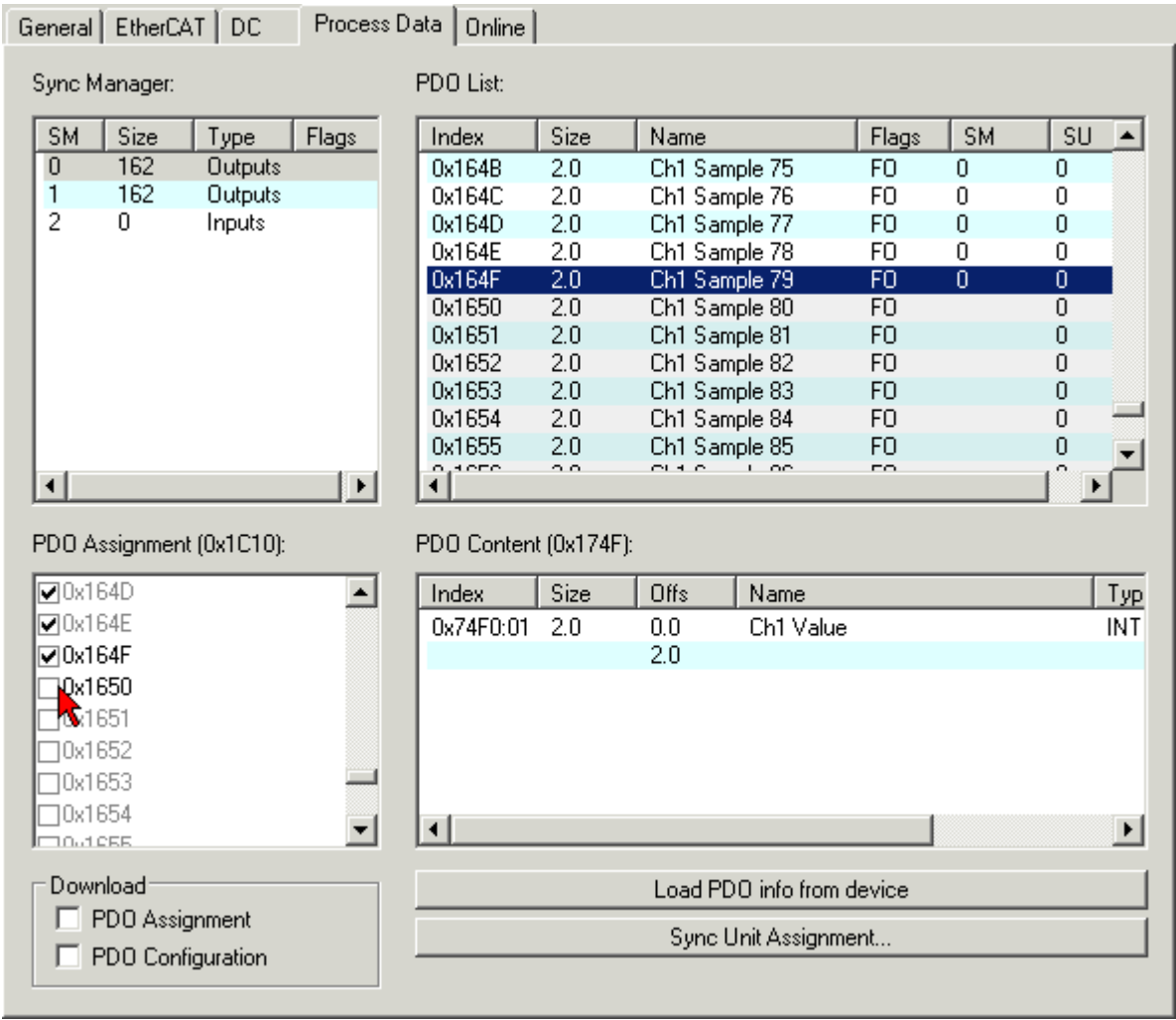
附图 187: Process Data（过程数据）选项卡，SM0 中过程数据的适配调整
