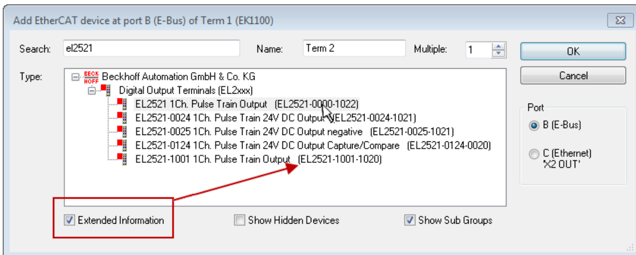
附图 91: 显示设备版本
