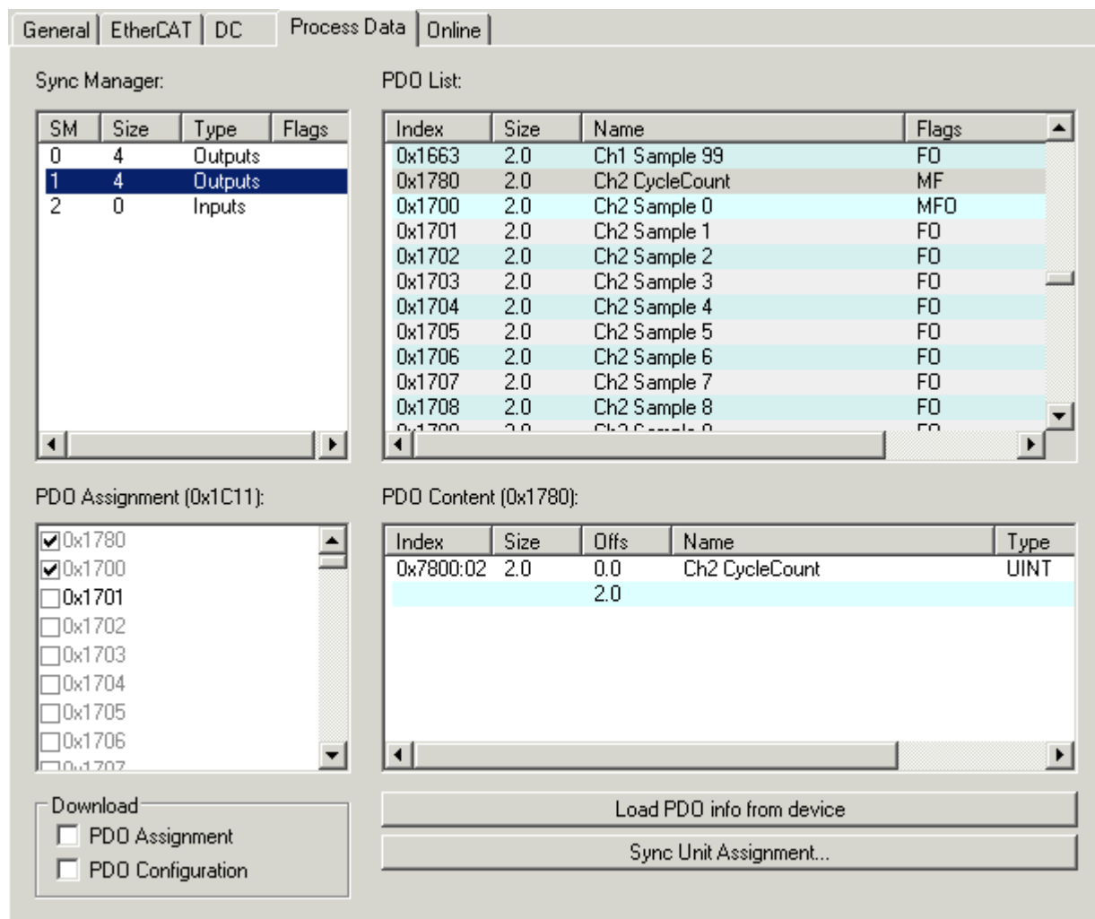
附图 176: Process Data (过程数据) 选项卡 SM1, EL47xx
