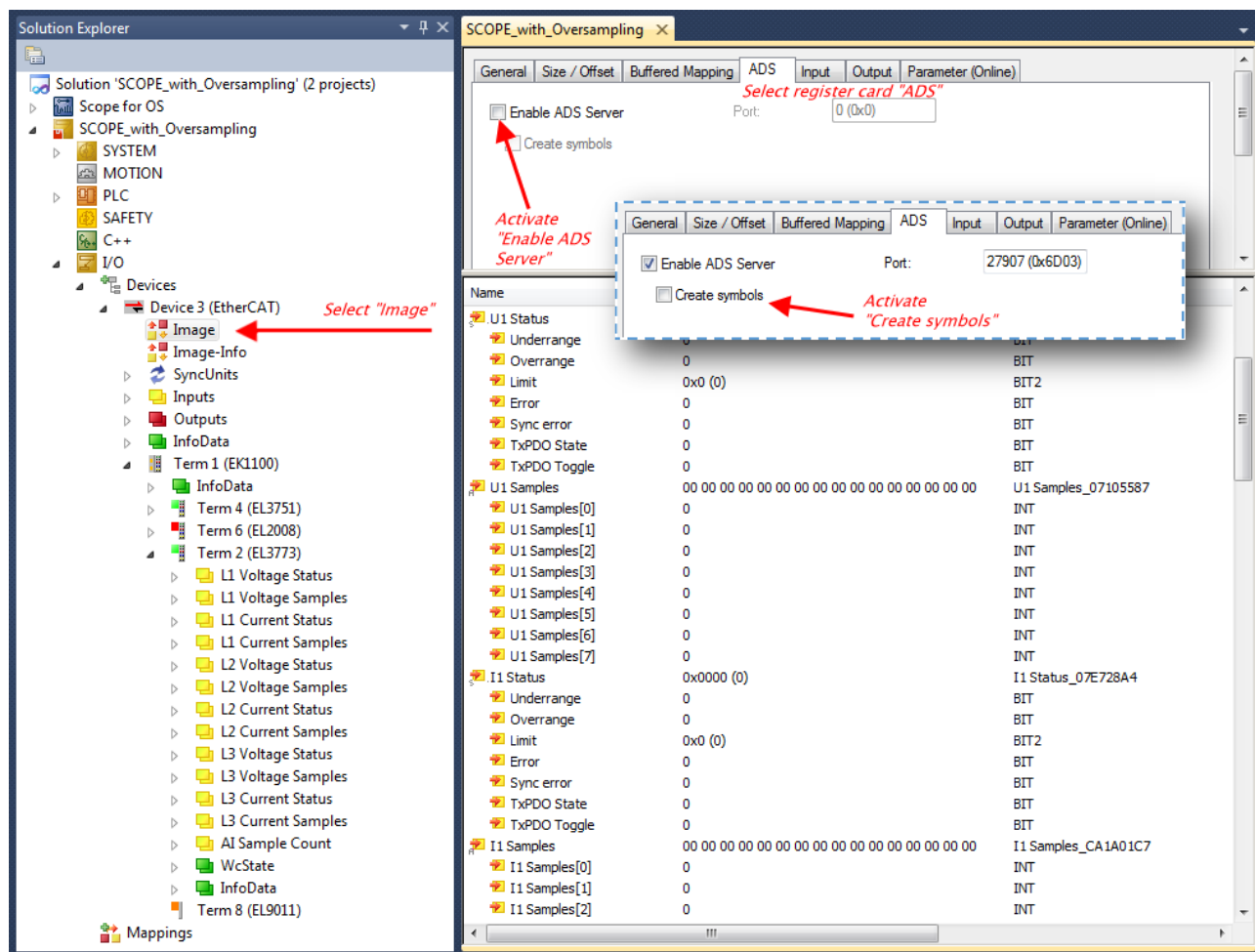
附图 146: 激活 EtherCAT 设备（TwinCAT 3）的 ADS 服务器
