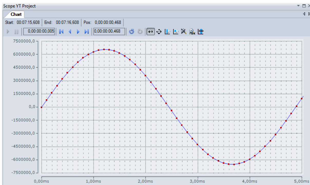
附图 145: 以 1 ms 测量周期时间进行 10 倍超采样记录正弦信号的示例
