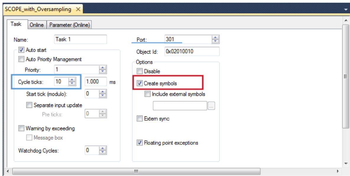
附图 139: 务必激活任务属性“Create symbols”（生成符号）
