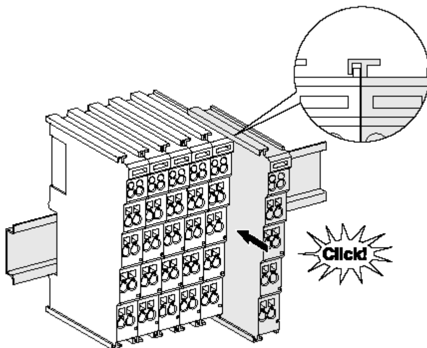
附图 9: 安装在安装轨道上
