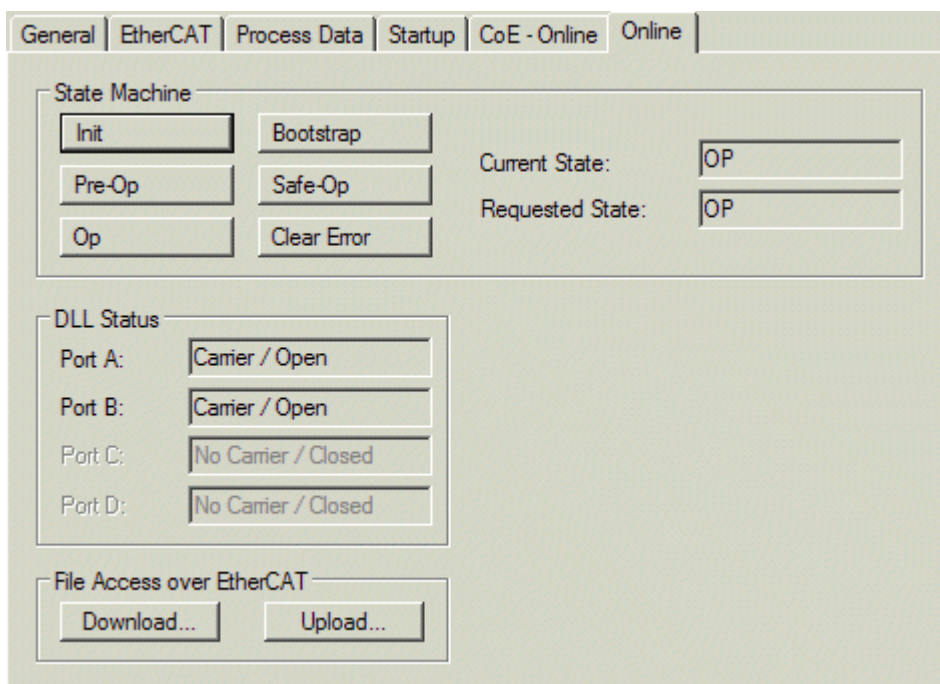
附图 124: “Online (在线)” 选项卡
