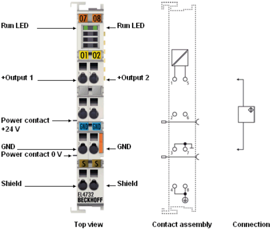
附图 24: EL4732 连接
