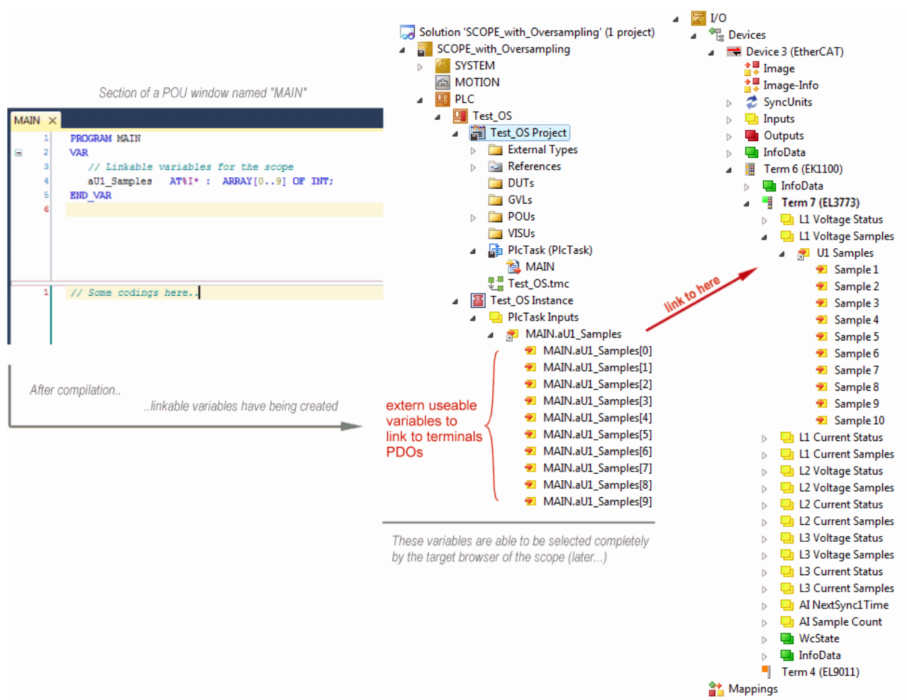
附图 137: 所创建的 PLC 数组变量（“aUI_Samples”）与 EL3773 的超采样 PDO 进行链接的表示
