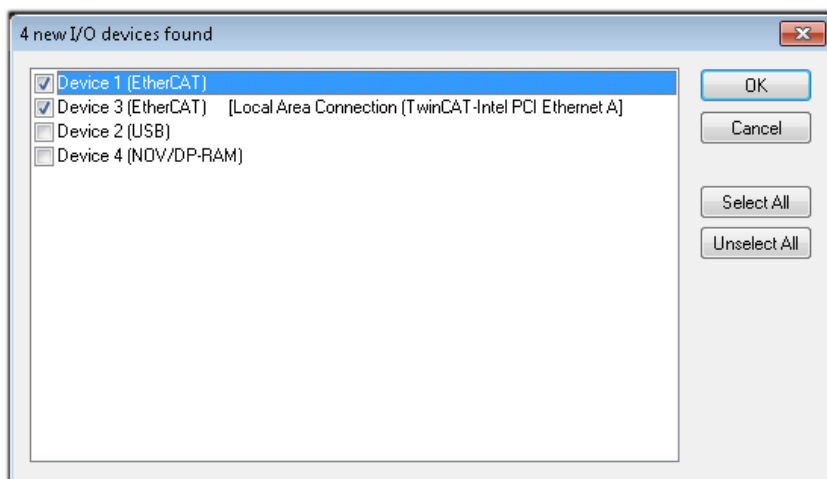
附图 31: 自动检测 I/O 设备：选择要集成的设备
