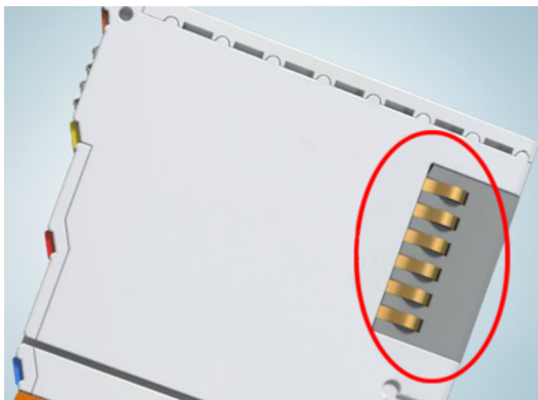
附图 8: 倍福 I/O 组件的弹簧触点
