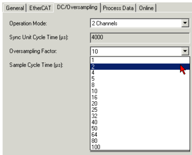
附图 180: DC 选项卡，示例设置为超采样系数 2，TwinCAT 2.11
