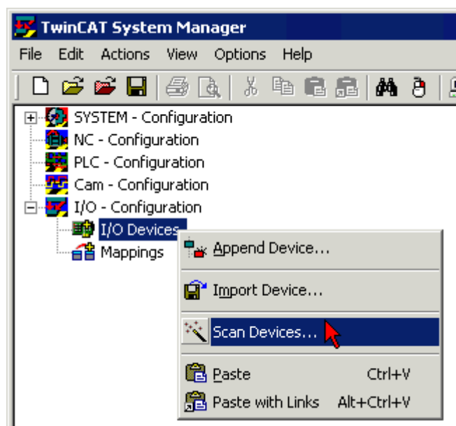
附图 164: 在 EtherCAT 配置中进行扫描（I/O Devices（I/O 设备）->右击->Scan Devices...（扫描设备...））
