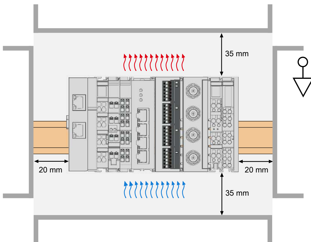
附图 16: 标准安装位置的建议最小距离
