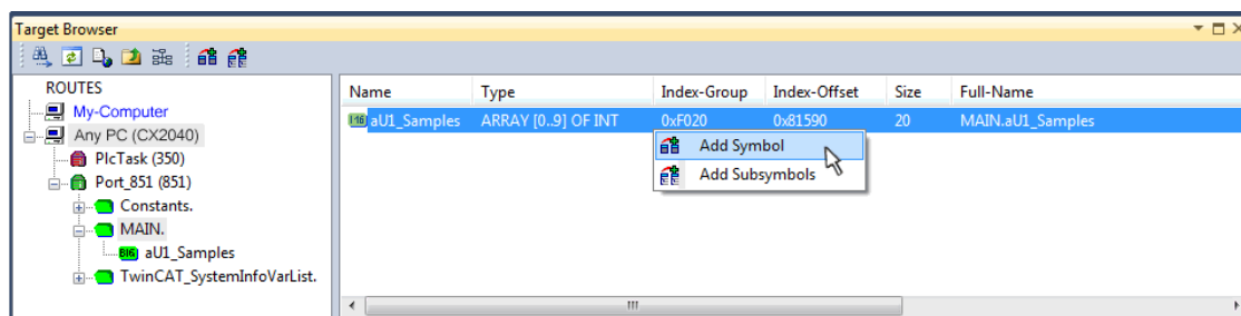
附图 144: 在 Solution Explorer（解决方案资源管理器）的示波器项目中，将变量“aUI_Samples”添加到“axis”（轴）下方
