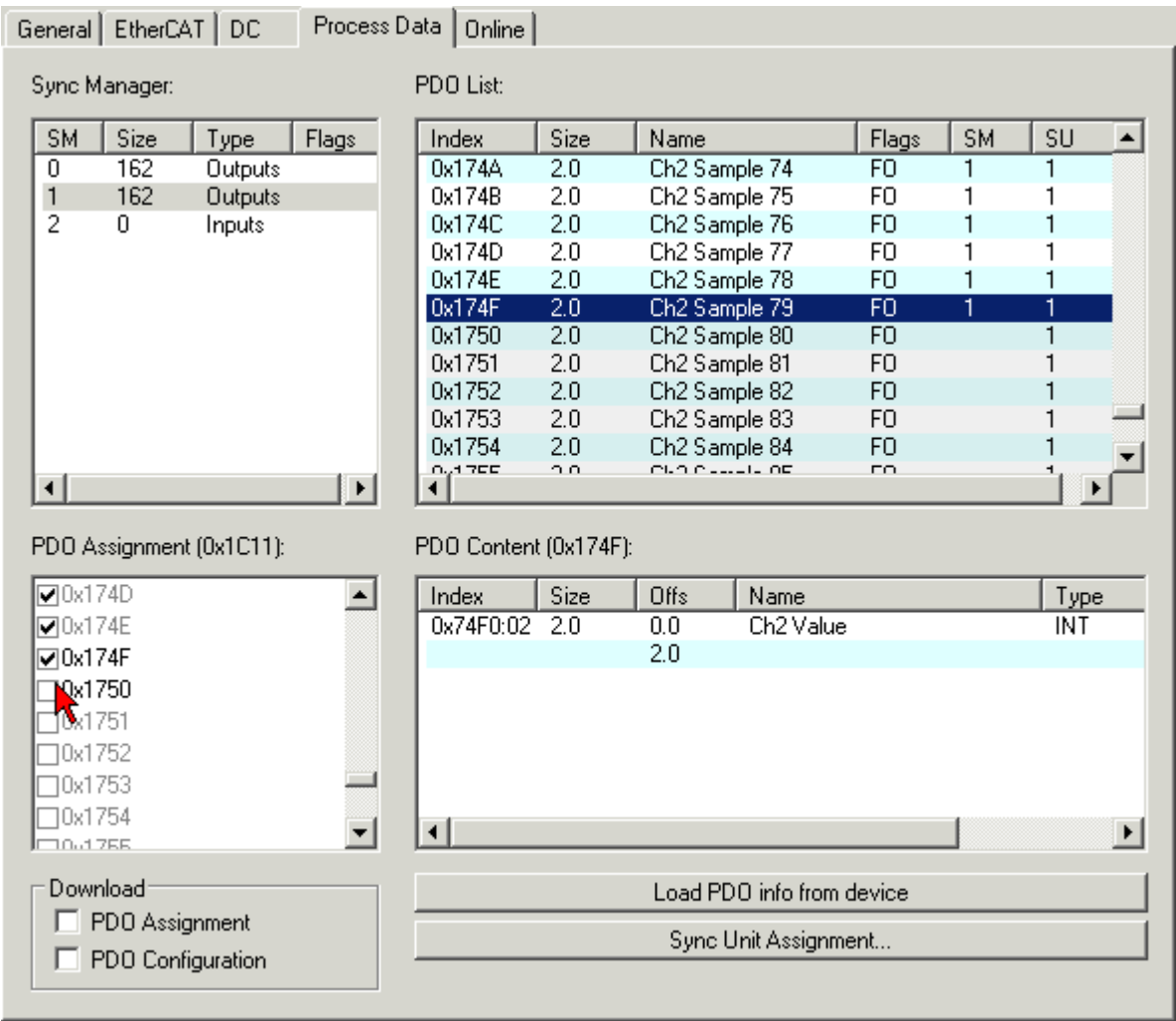
附图 188: Process Data（过程数据）选项卡，SM1 中过程数据的适配调整
