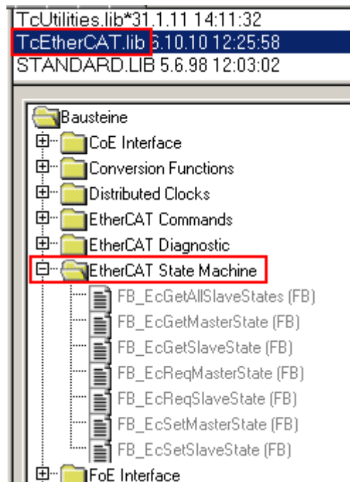
附图 132: PLC 功能块
