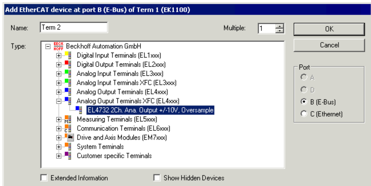
附图 170: 选择 EL4732 端子模块
