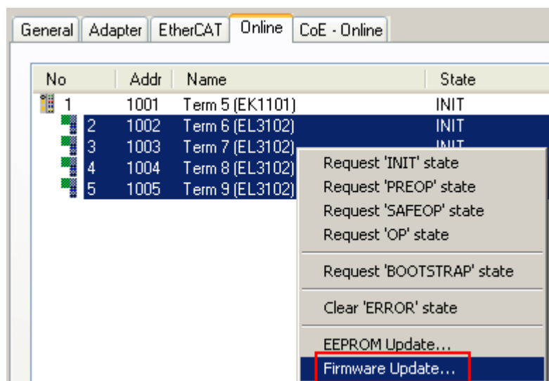
附图 201: 多重选择和固件更新
