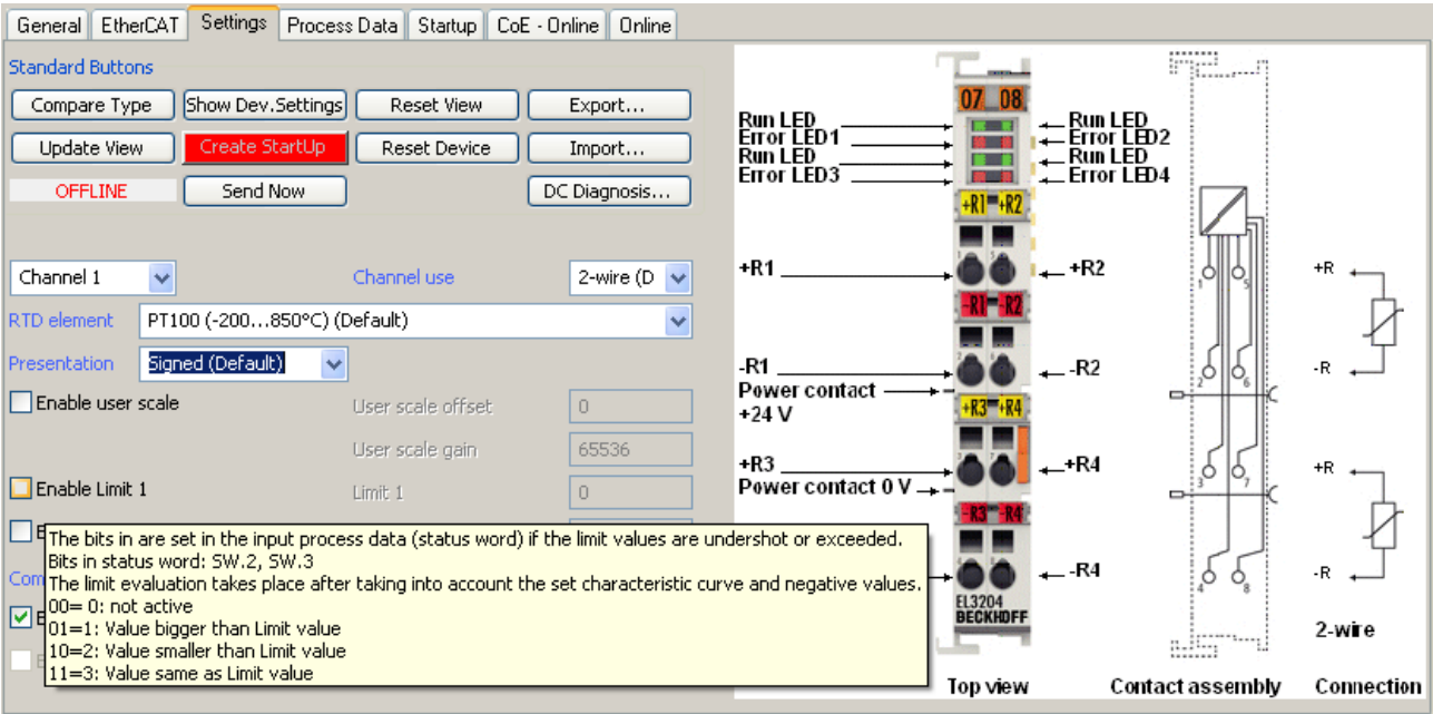
附图 129: EL3204 调试助手示例
