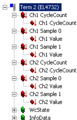
附图 181: TwinCAT 树型结构，示例设置为双通道、2 倍超采样
