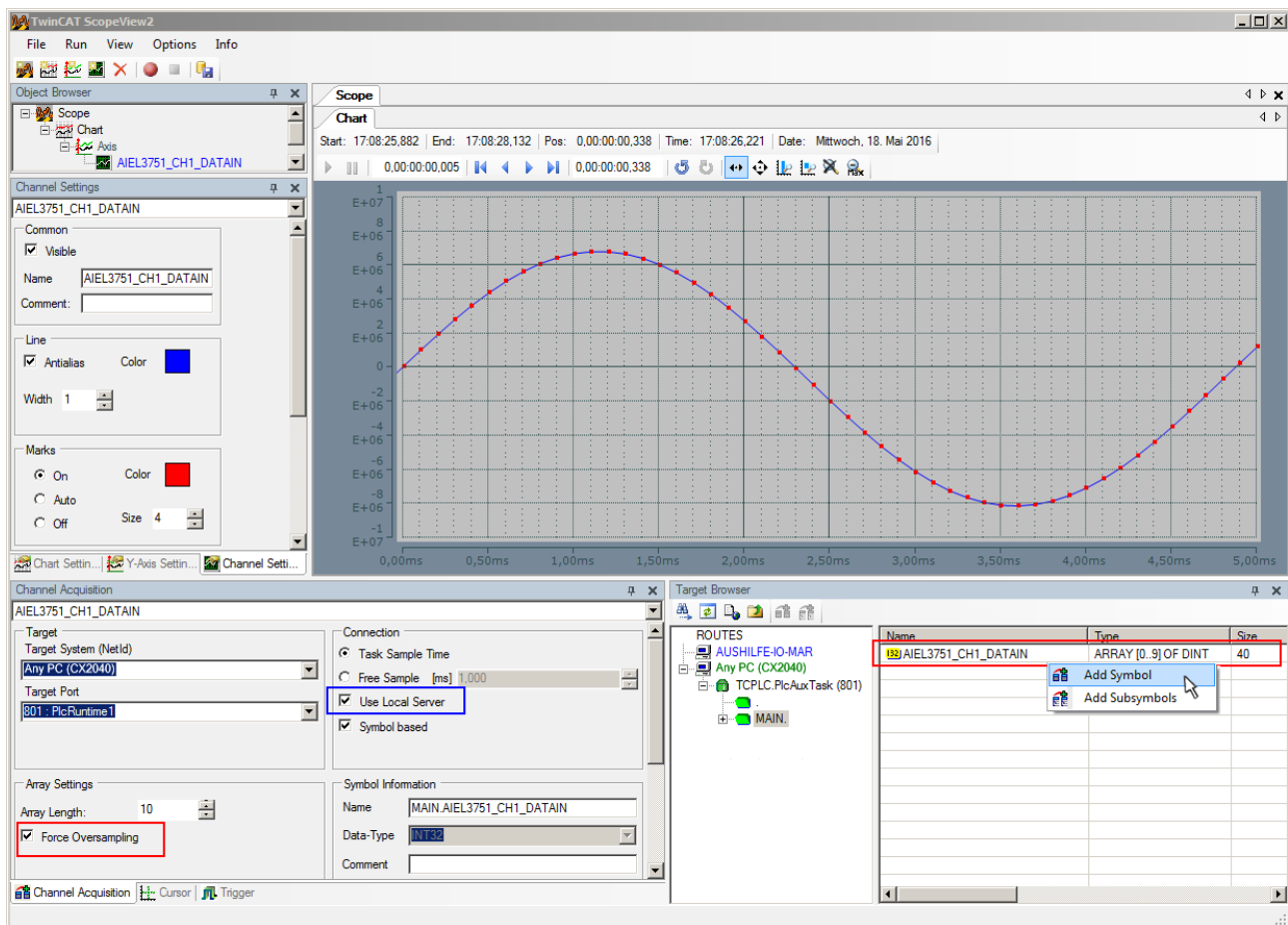
附图 160: Scope2 中 EL3751 的 10 倍超采样变量示意图
