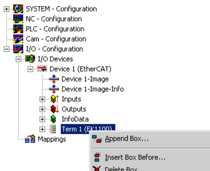
附图 169: 添加新对话框（Device（设备）-&gt;右击-&gt;Append Box...（添加对话框...））
