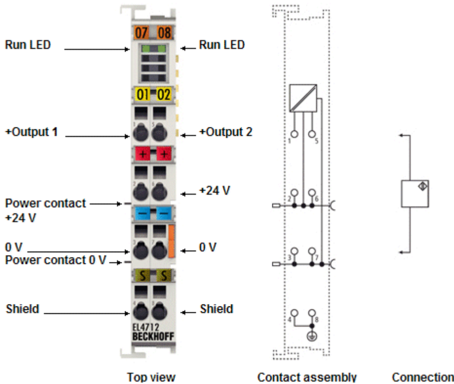
附图 23: EL4712 连接
