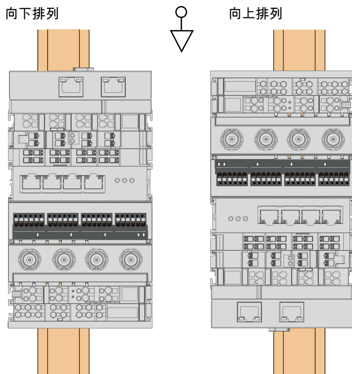
附图 17: 垂直安装位置，向下排列（左）/向上排列（右）
