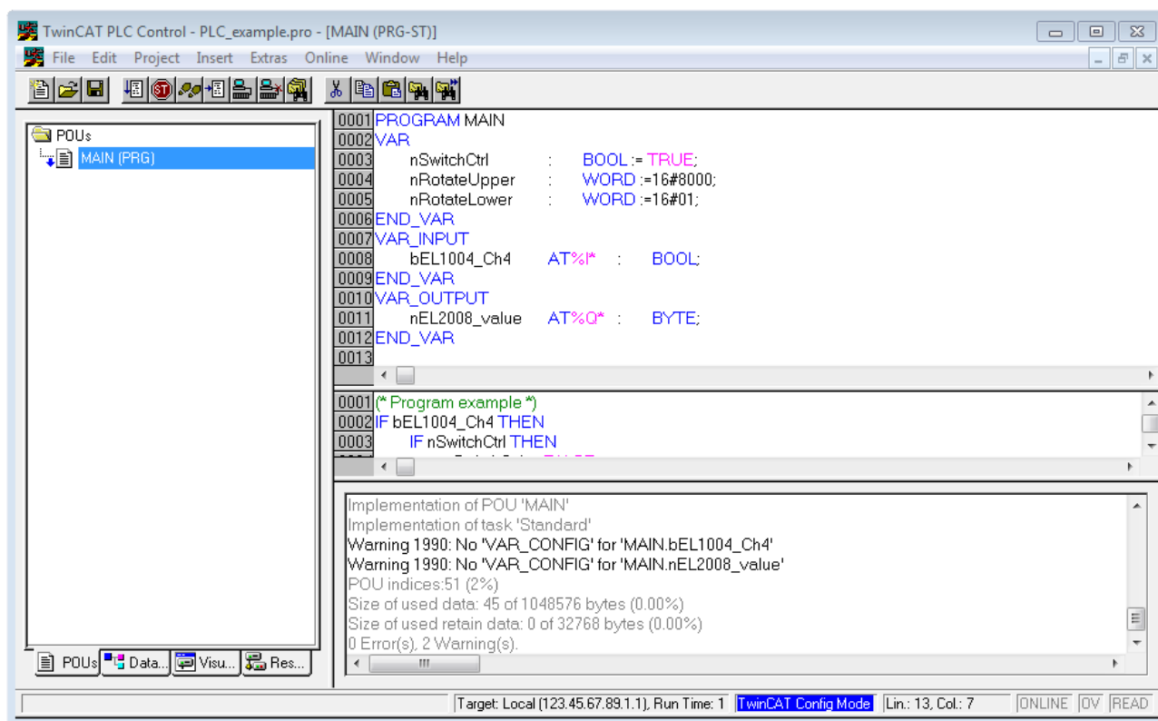
附图 35: 示例程序编译后，包含未分配地址的变量
