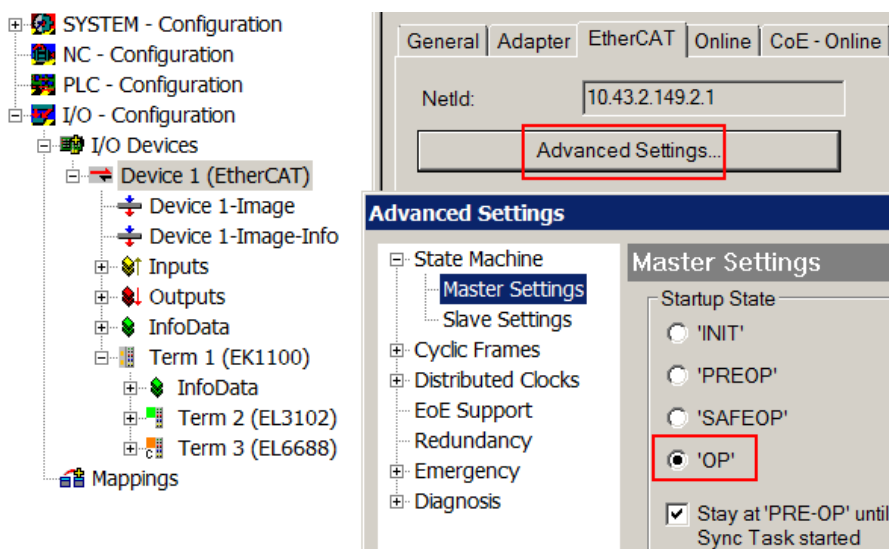
附图 130: System Manager 的默认行为
