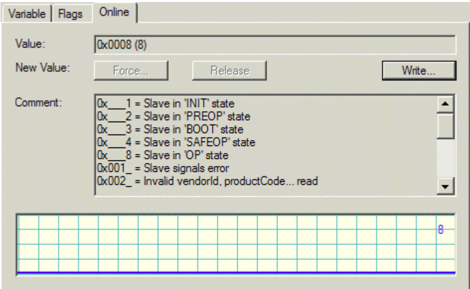
附图 174: InfoData, 状态, Online（在线）选项卡
