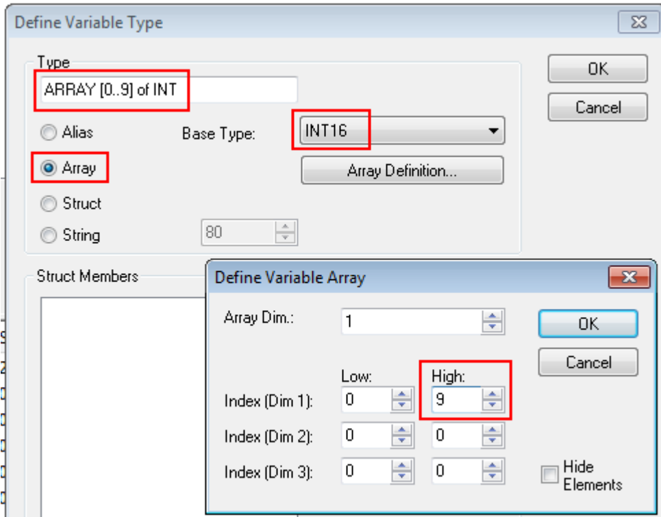
附图 151: 变量类型的定义
