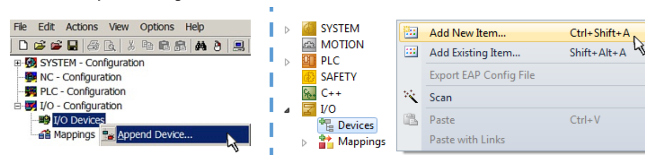
附图 85: 添加 EtherCAT 设备（左：TwinCAT 2；右：TwinCAT 3）
