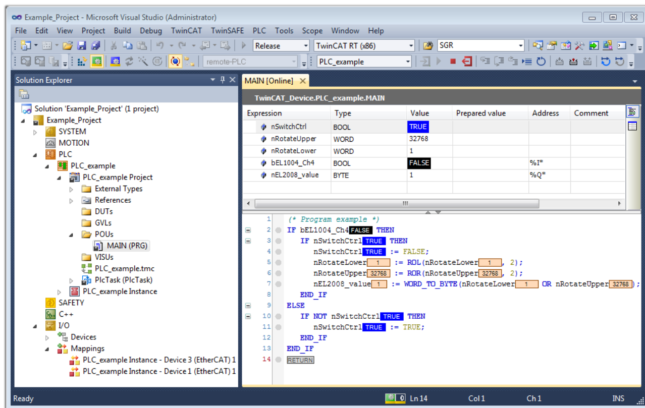
附图 66: TwinCAT 3 开发环境 (VS shell)：Login 后，程序已运行
