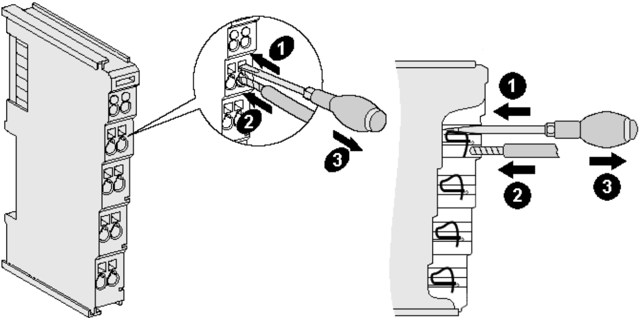
附图 15: 在一个接线点上连接线缆
