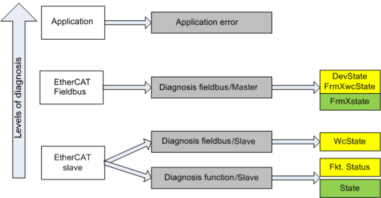
附图 126: 选择 EtherCAT 从站的诊断信息
