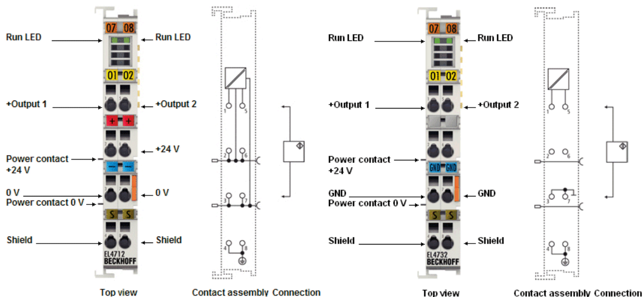
附图 4: EL4712, EL4732
