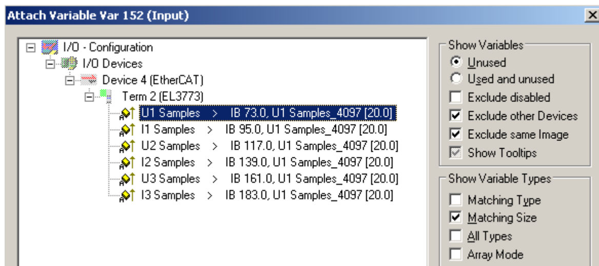
附图 154: 超采样端子模块的数组变量
