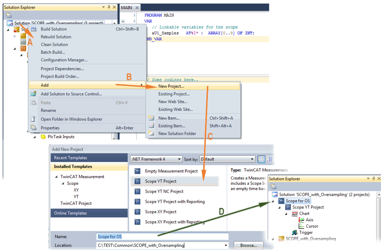
附图 136: 将 Scope 项目添加到现有项目中
