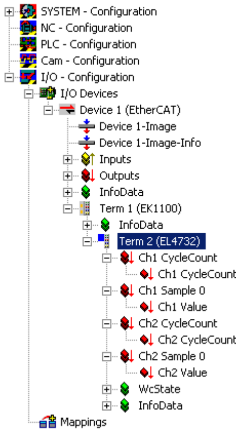
附图 172: TwinCAT 树型结构 EL4732
