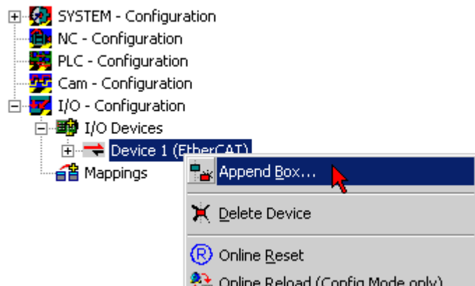
附图 167: 添加新对话框 (Device (设备) -> 右击 -> Append Box... (添加对话框...))
