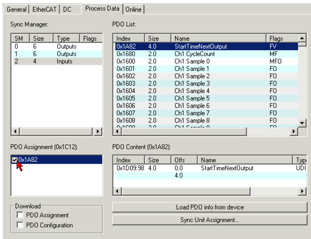
附图 182: Process Data（过程数据）选项卡，激活索引 0x1A82，条目“StartTimeNextOutput”
