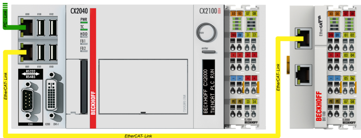
附图 26: 系统配置，含嵌入式控制器、输入（EL1004）和输出（EL2008）
