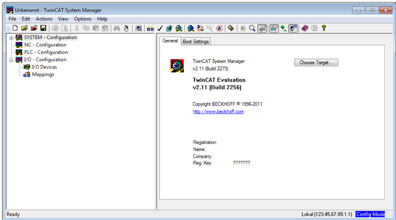
附图 27: TwinCAT 2 的初始用户界面
