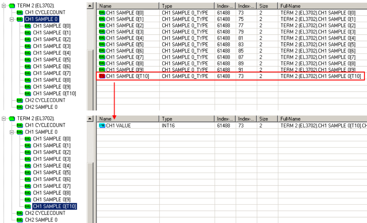
附图 163: Scope2 中自动计算的数组变量（红色）
