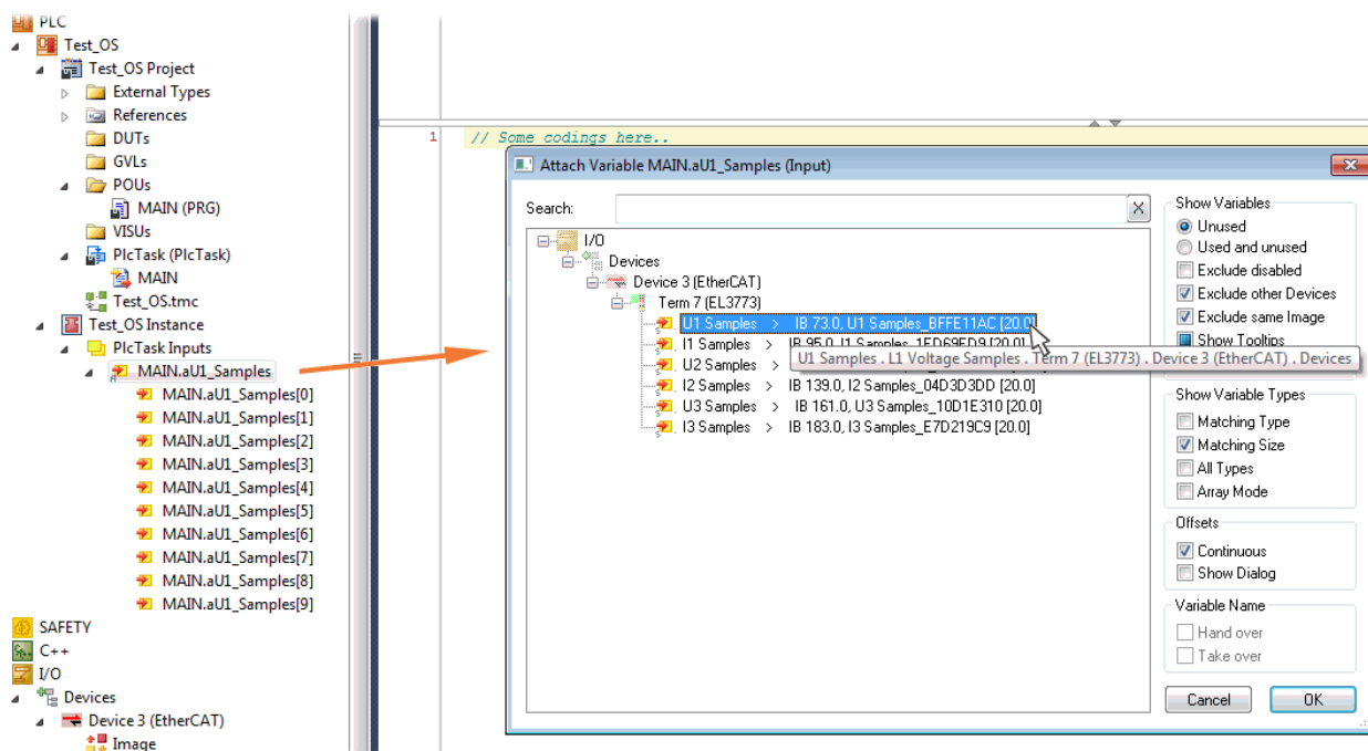
附图 142: 选择 EL3773 PDO “L1 Voltage Samples”（L1 电压采样），以创建与 PLC 数组变量“aUI_Samples”的链接
