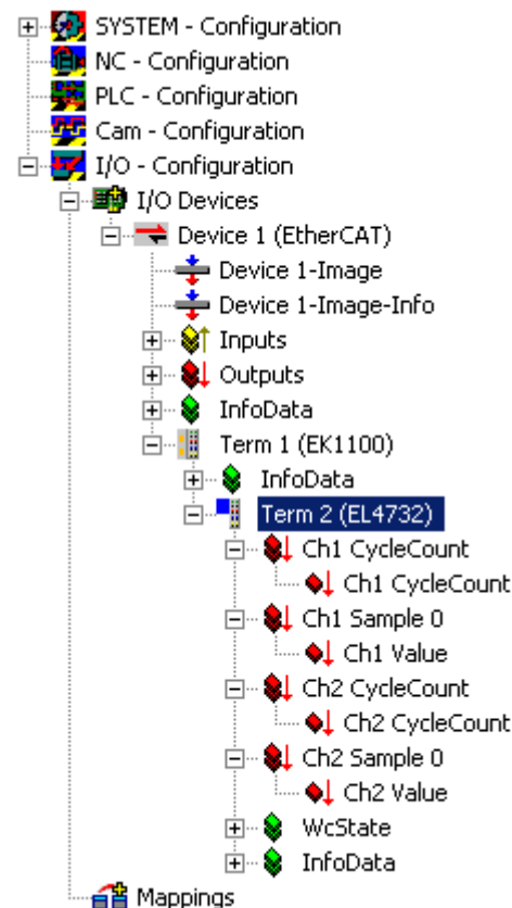
附图 171: TwinCAT 树型结构中的端子模块
