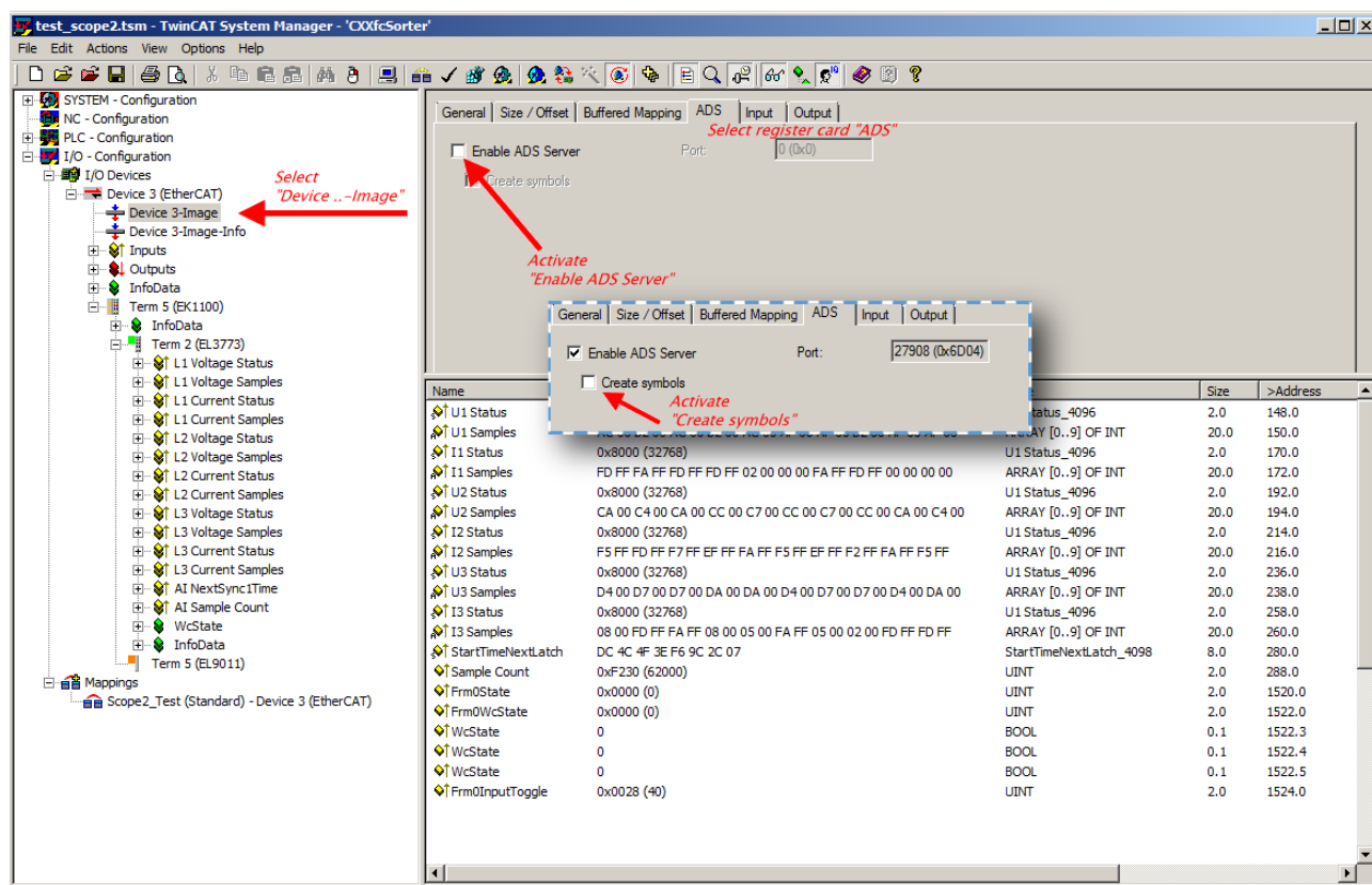
附图 161: 激活 EtherCAT 设备 (TwinCAT 2) 的 ADS 服务器
