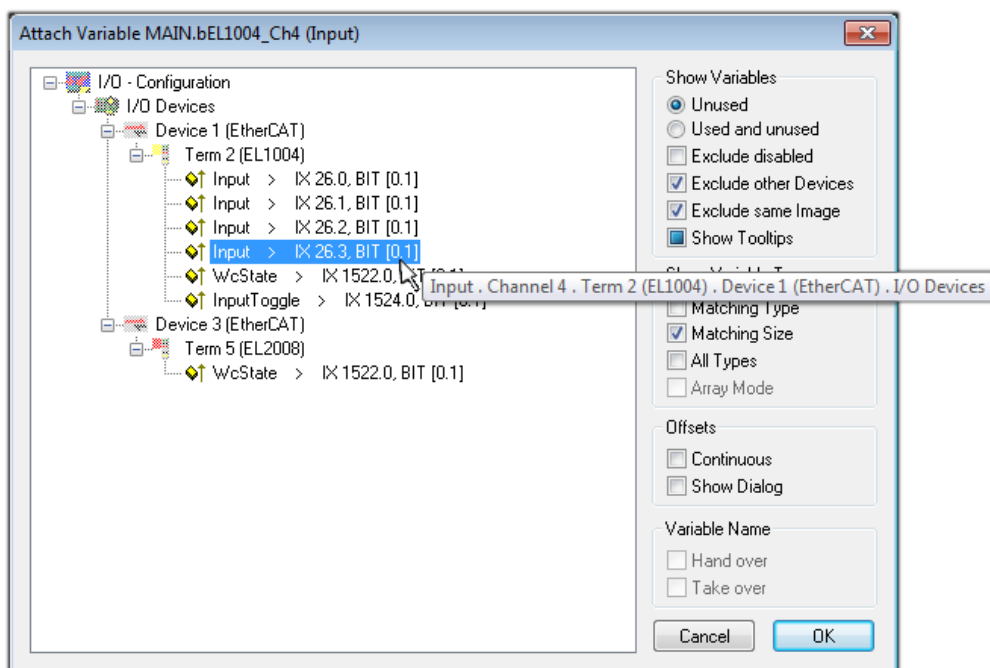
附图 39: 选择 BOOL 类型的 PDO
