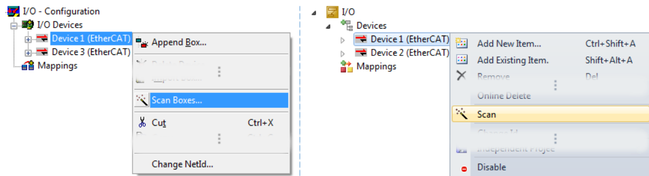
附图 103: 手动扫描特定 EtherCAT 主站上的设备（左：TwinCAT 2；右：TwinCAT 3）
