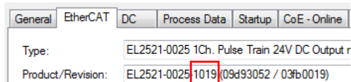
附图 101: 检测修订版本 1019 的 EtherCAT 端子模块
