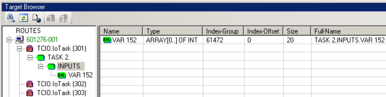
附图 156: 导航至数组 VAR152 的变量浏览器
