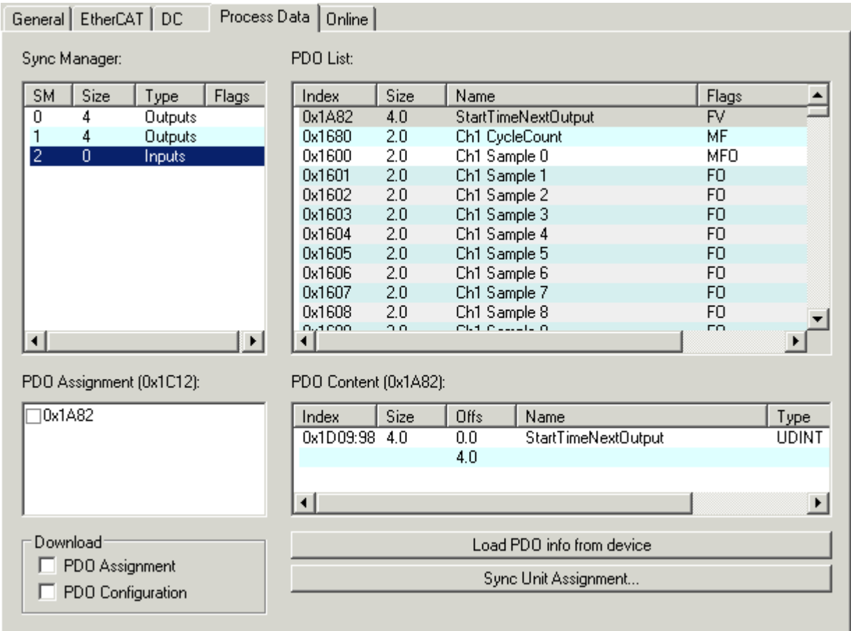
附图 177: Process Data（过程数据）选项卡 SM2，EL47xx
