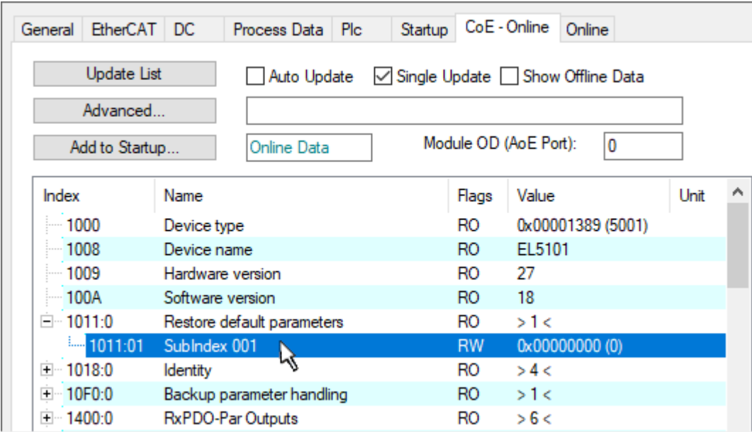
附图 202: 选择 Restore default parameters
