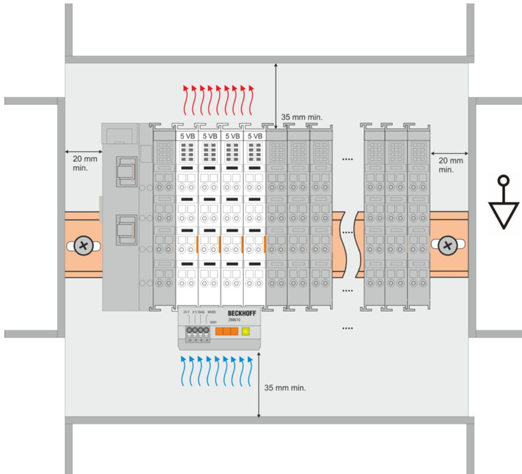
附图 19: 以水平安装位置为例，带风扇运行的建议最小距离
