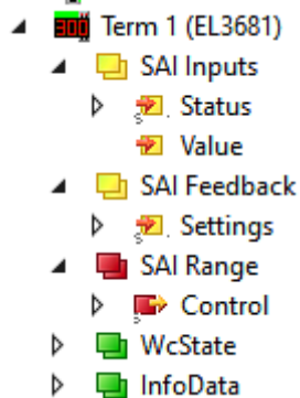
Abb. 136: EL3681 im TwinCAT-Baum
