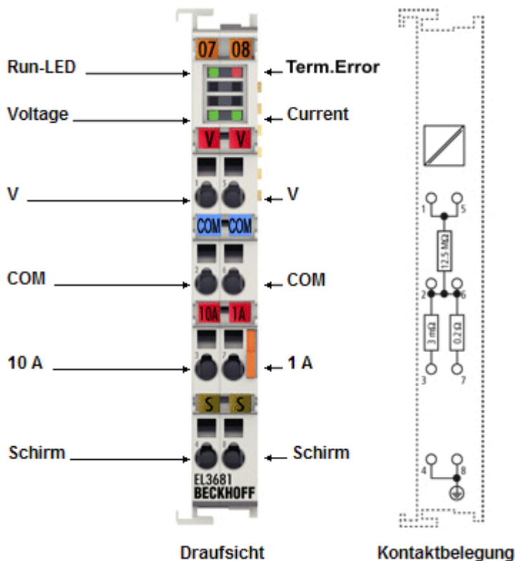
Abb. 26: EL3681 Anschlussbelegung
