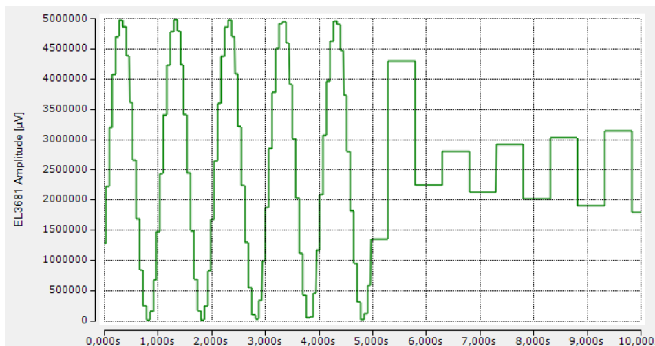
Abb. 145: Sinus-Signal, 0/5 V, 1 Hz
