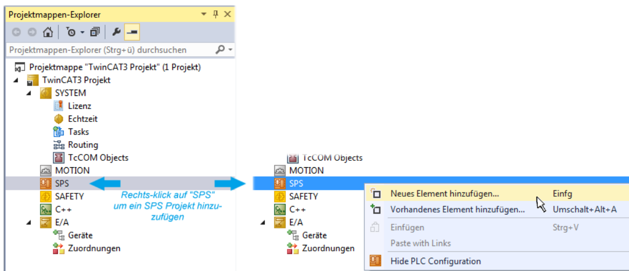
Abb. 55: Einfügen der Programmierumgebung in „SPS“
