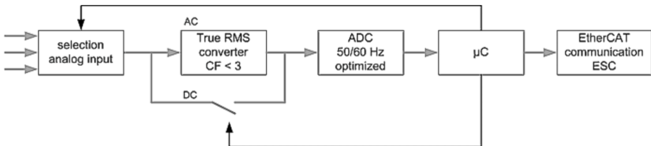
Abb. 5: Datenfluss EL3681
