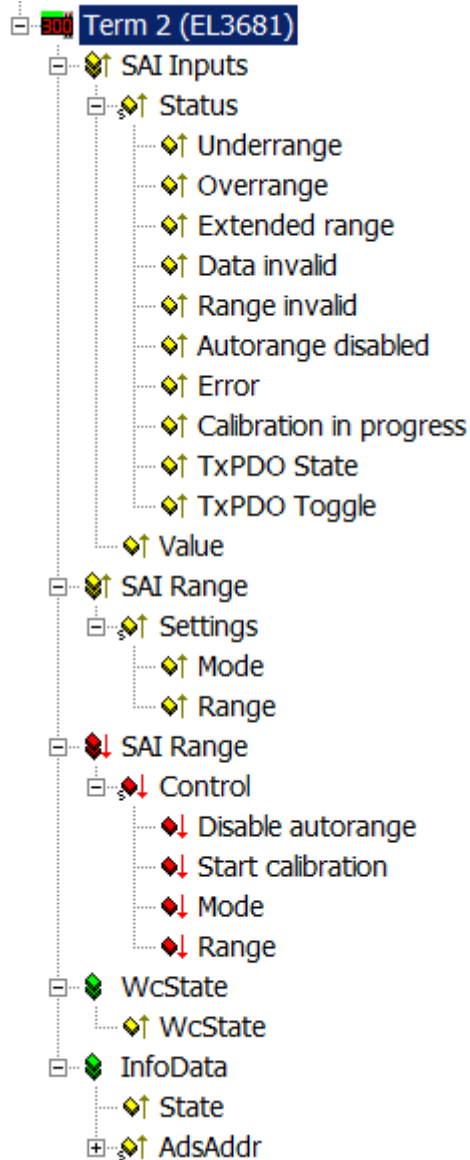
Abb. 147: Default-Prozessabbild EL3681
