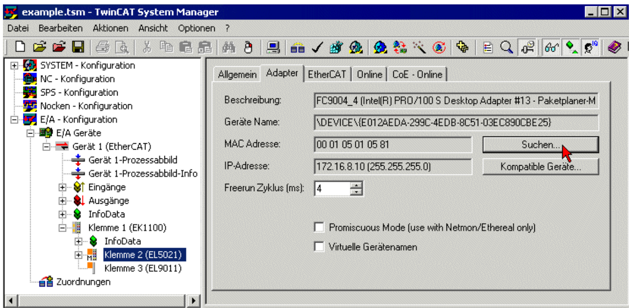
Abb. 151: Suchen des Ethernet-Adapters
