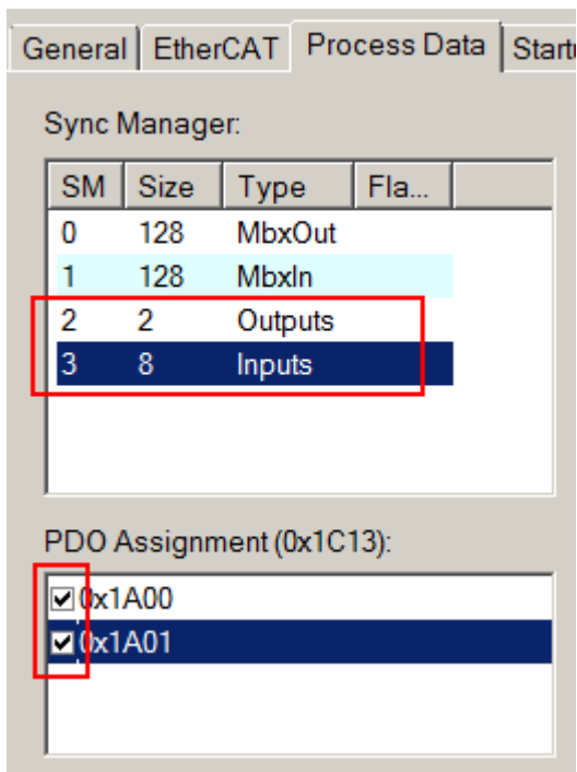
Abb. 148: PDO-Auswahl TwinCAT System Manager
