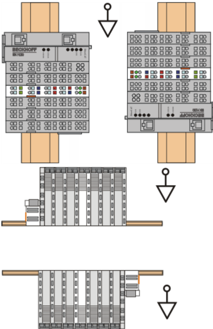
Abb. 102: Weitere Einbaulagen
