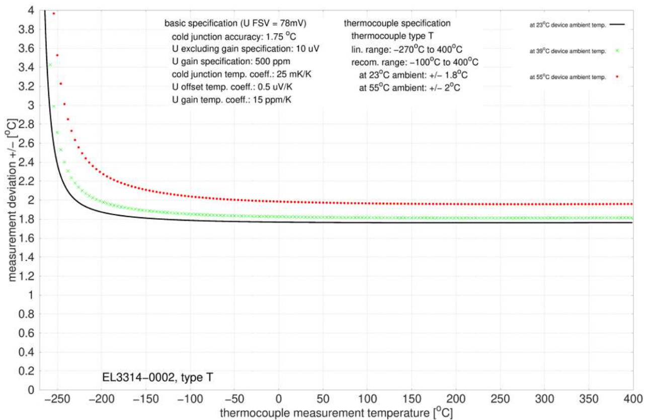
Abb. 74: EL3314-0002 und EL3314-0092 (entspricht EL3314-0002), Typ T
