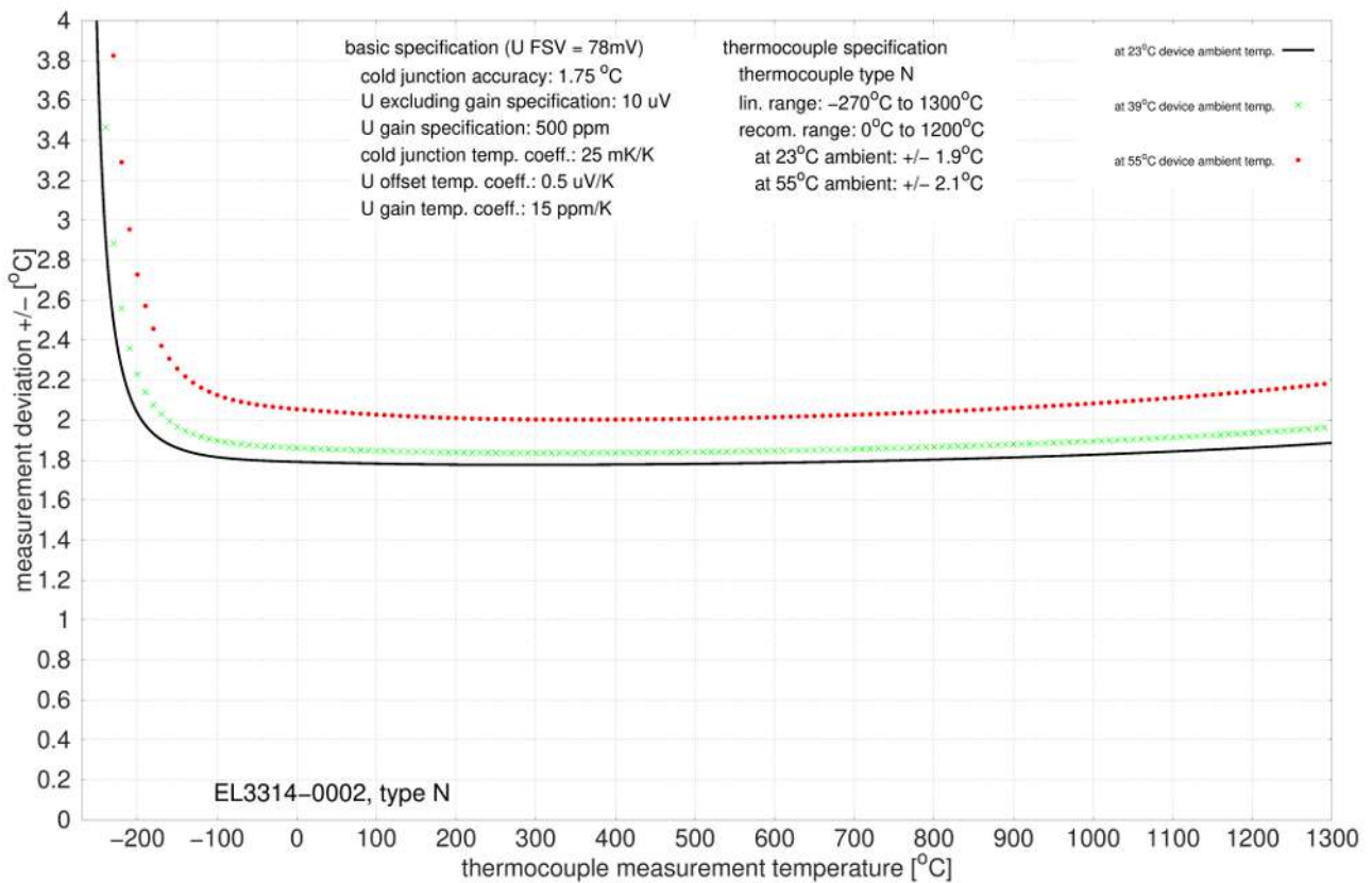
Abb. 71: EL3314-0002 und EL3314-0092 (entspricht EL3314-0002), Typ N
