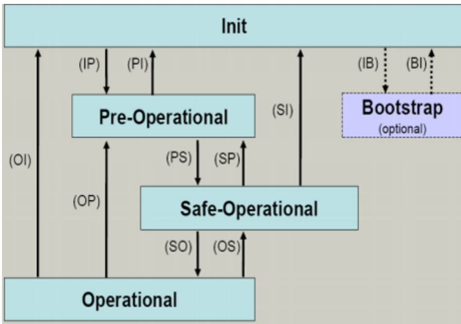
Abb. 85: Zustände der EtherCAT State Machine
