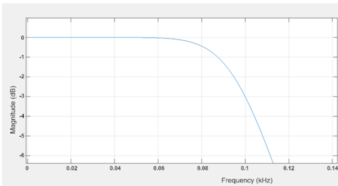
Abb. 225: Beispiel IIR Tiefpass 100Hz
