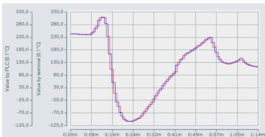
Abb. 241: Blau: Temperaturwerte aus der PLC-Berechnung; Rot: PDO-Werte im Temperaturmessbereich
