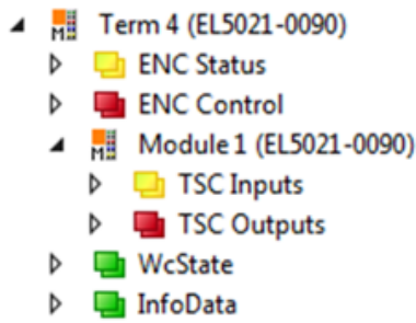
Abb. 233: Prozessdaten TwinSAFE SC Komponente, Beispiel EL5021-0090
