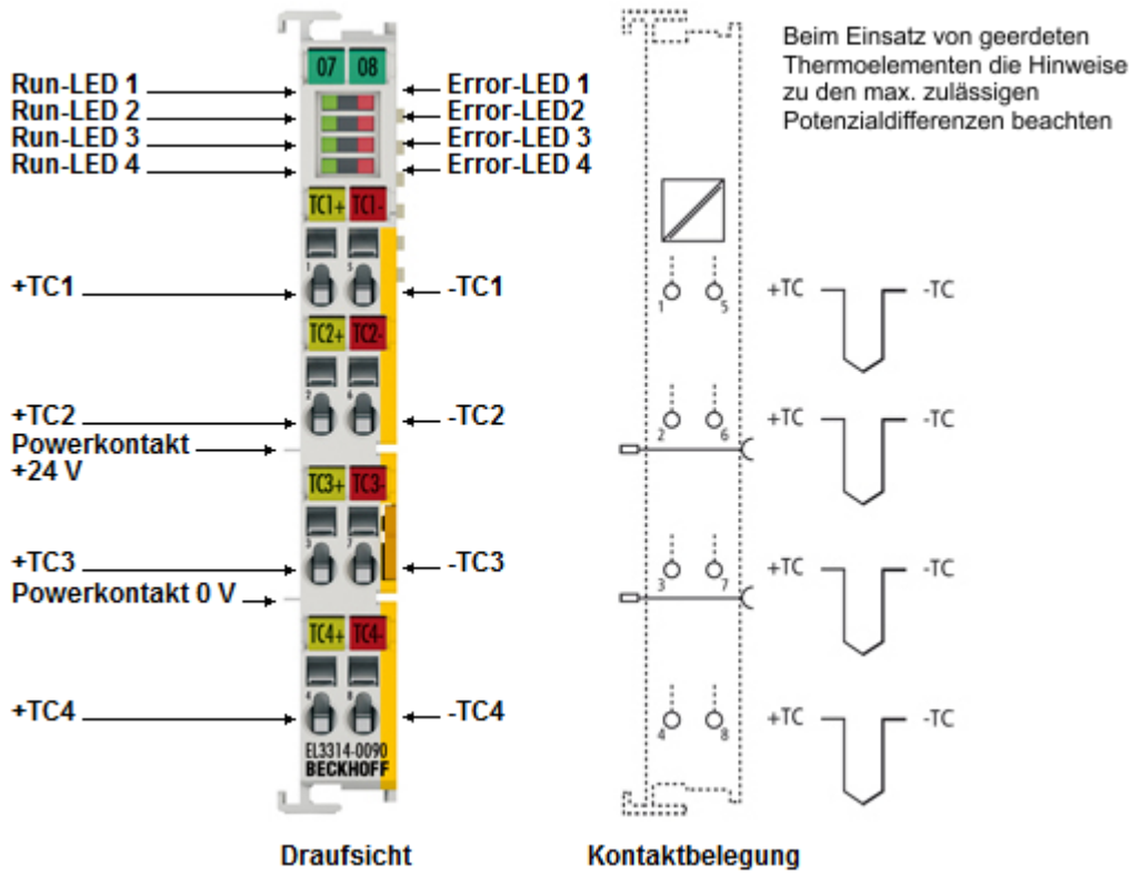
Abb. 63: EL3314-0090
