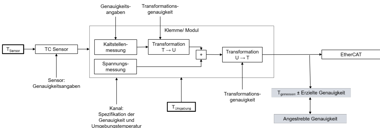
Abb. 80: Verkettung der Unsicherheiten in der Temperaturmessung mit Thermoelementen
