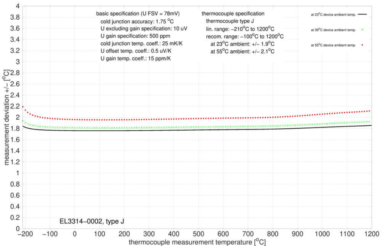
Abb. 68: EL3314-0002 und EL3314-0092 (entspricht EL3314-0002), Typ J
