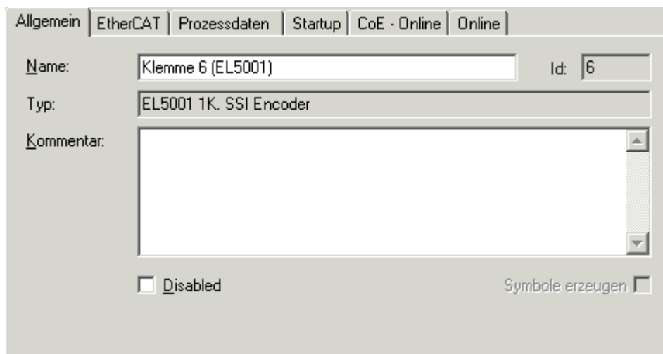
Abb. 194: Karteireiter „Allgemein“
