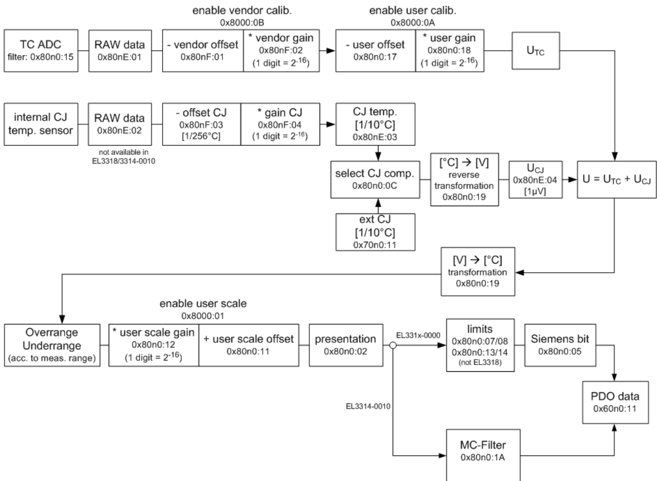
Abb. 215: EL33xx Dataflow
