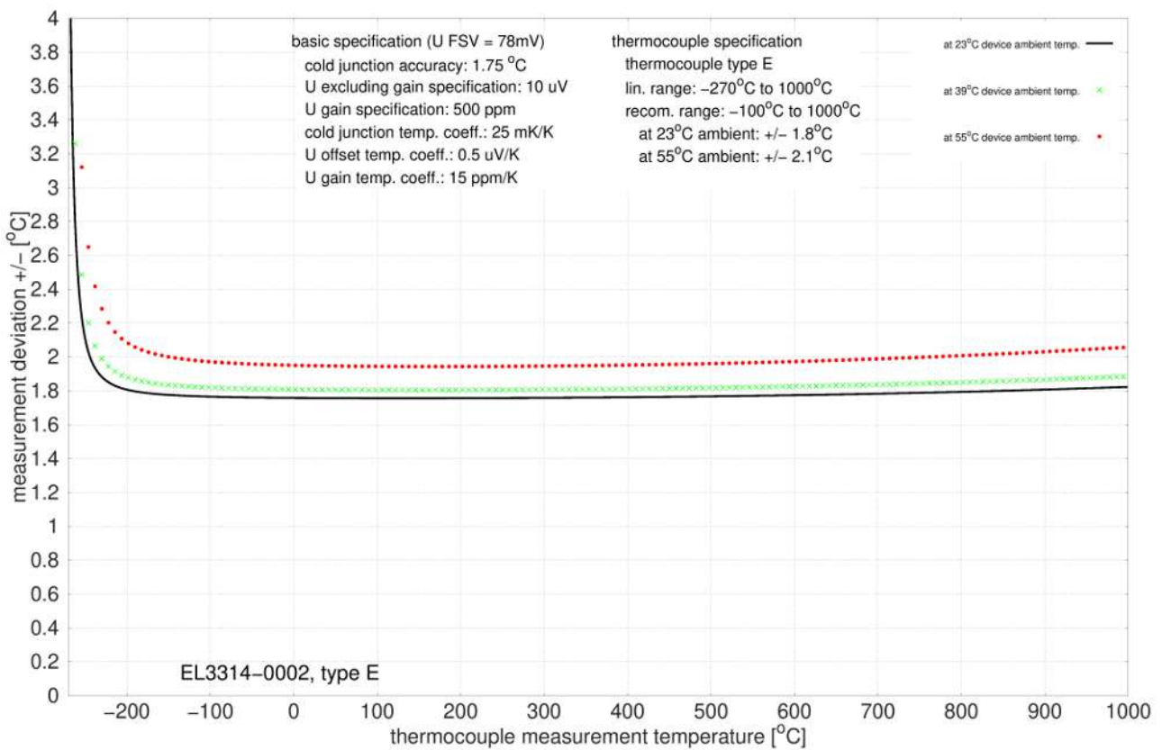
Abb. 13: EL3314-0002 und EL3314-0092 (entspricht EL3314-0002), Typ E
