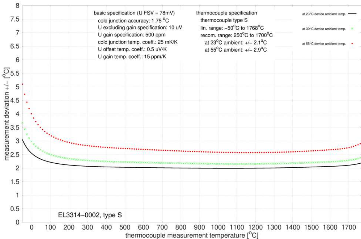
Abb. 19: EL3314-0002 und EL3314-0092 (entspricht EL3314-0002), Typ S
