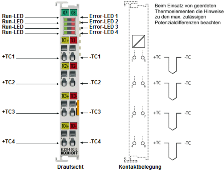
Abb. 61: EL3314-0030 (EL3314-0010)
