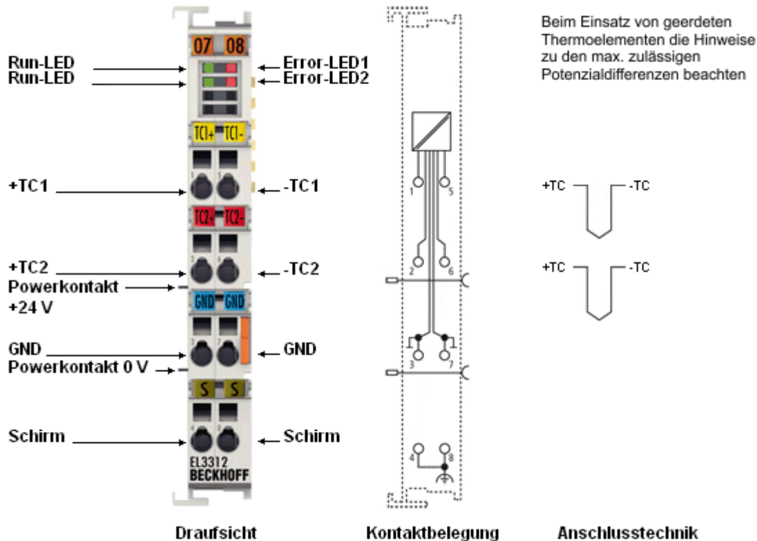
Abb. 6: EL3312
