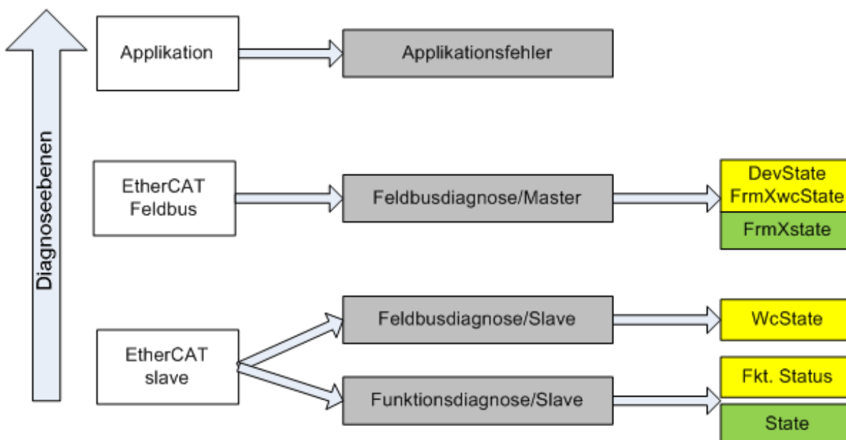
Abb. 203: Auswahl an Diagnoseinformationen eines EtherCAT Slave
