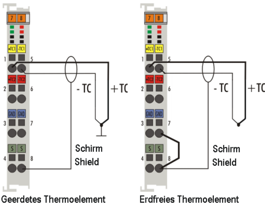
Abb. 98: Anschlussstechniken geerdetes - und erdfreies Thermoelement
