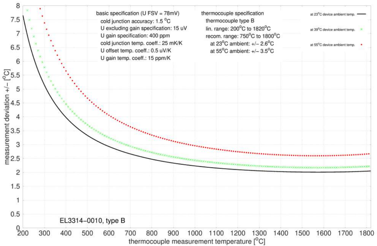
Abb. 37: EL3314-0010, EL3314-0020 und EL3314-0030 (entsprechen EL3314-0010), Typ B
