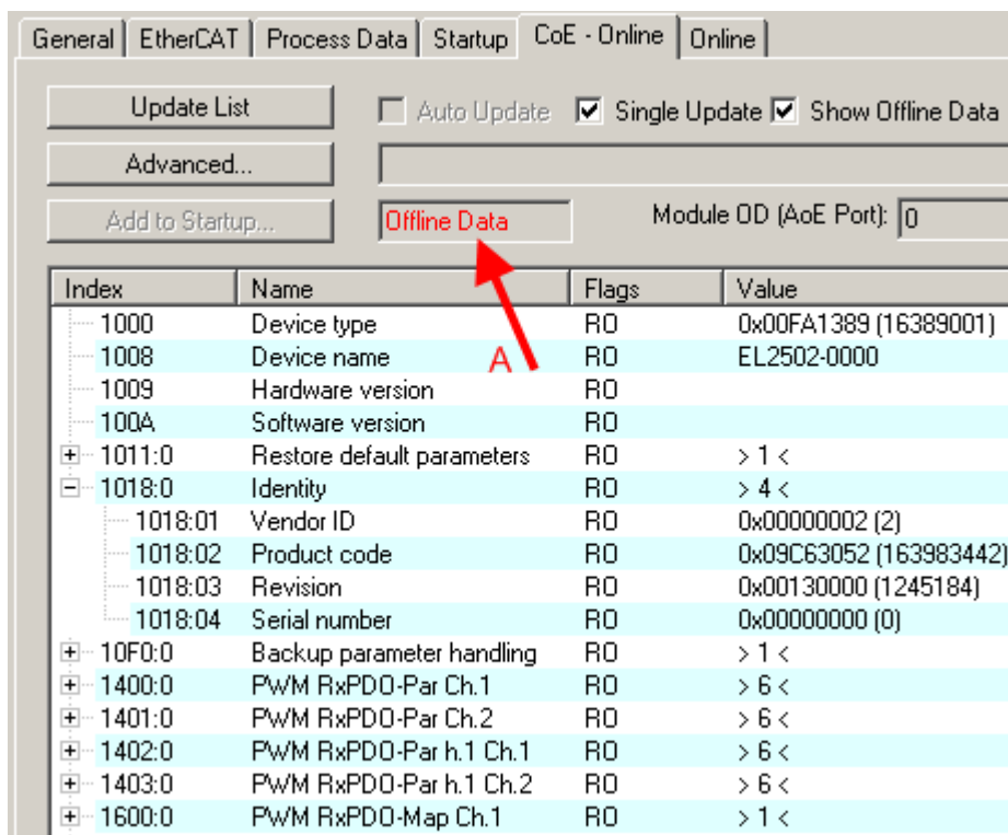
Abb. 88: Offline-Verzeichnis
