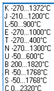
Abb. 223: Auswahlmöglichkeiten Transformation
