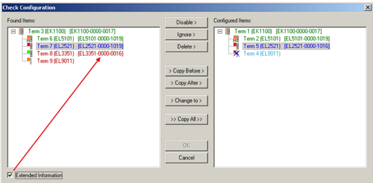
Abb. 188: Korrekturdialog
