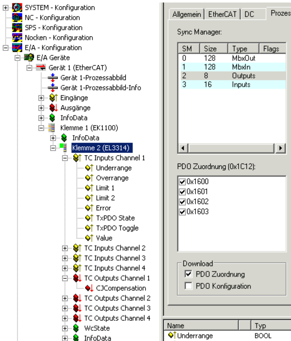
Abb. 81: Prozessdaten der EL3314
