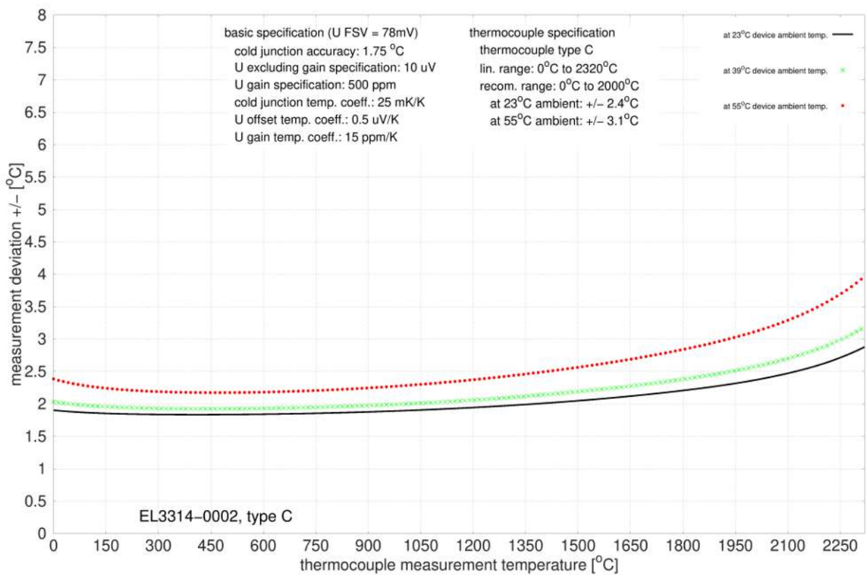
Abb. 12: EL3314-0002 und EL3314-0092 (entspricht EL3314-0002), Typ C
