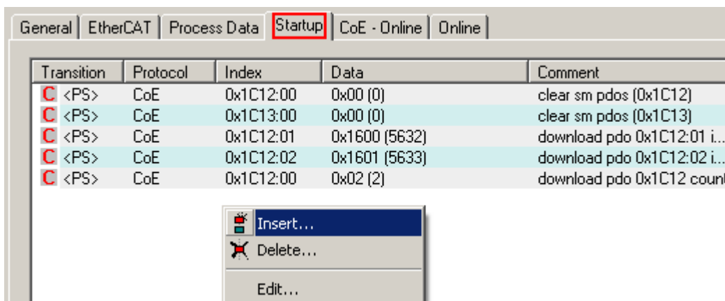
Abb. 87: StartUp-Liste im TwinCAT System Manager
