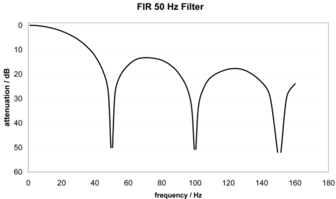
Abb. 226: Beispiel Notchfilter/Kerbfilter
