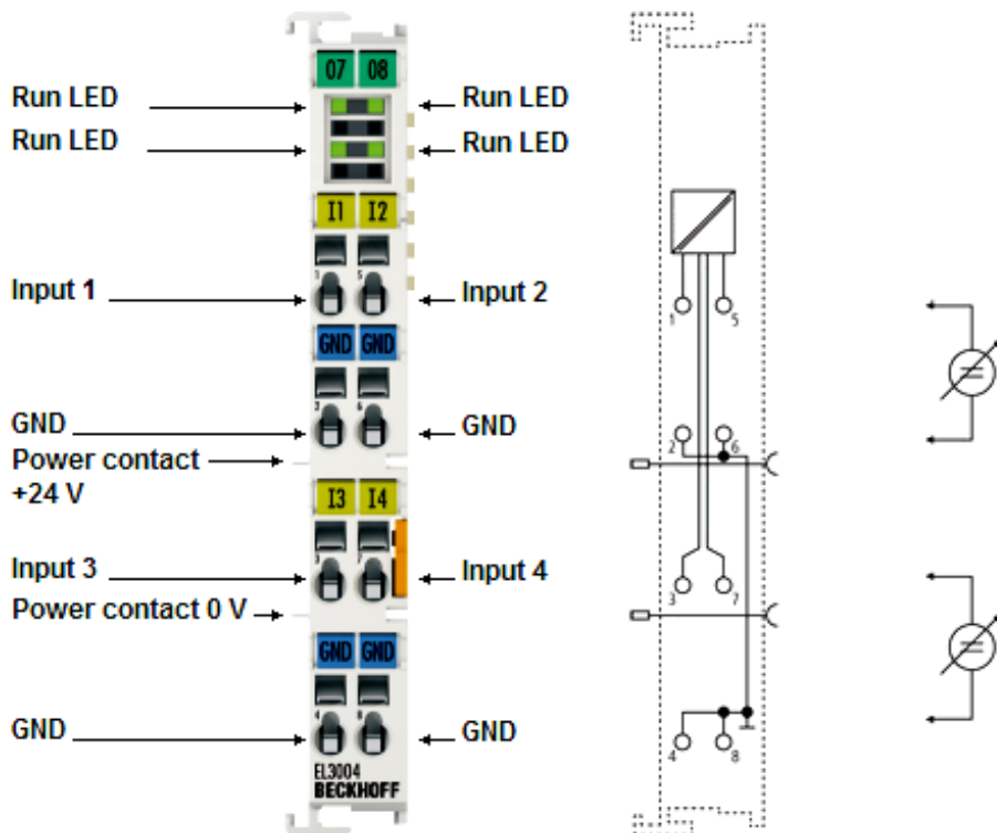
附图 8: EL3004
