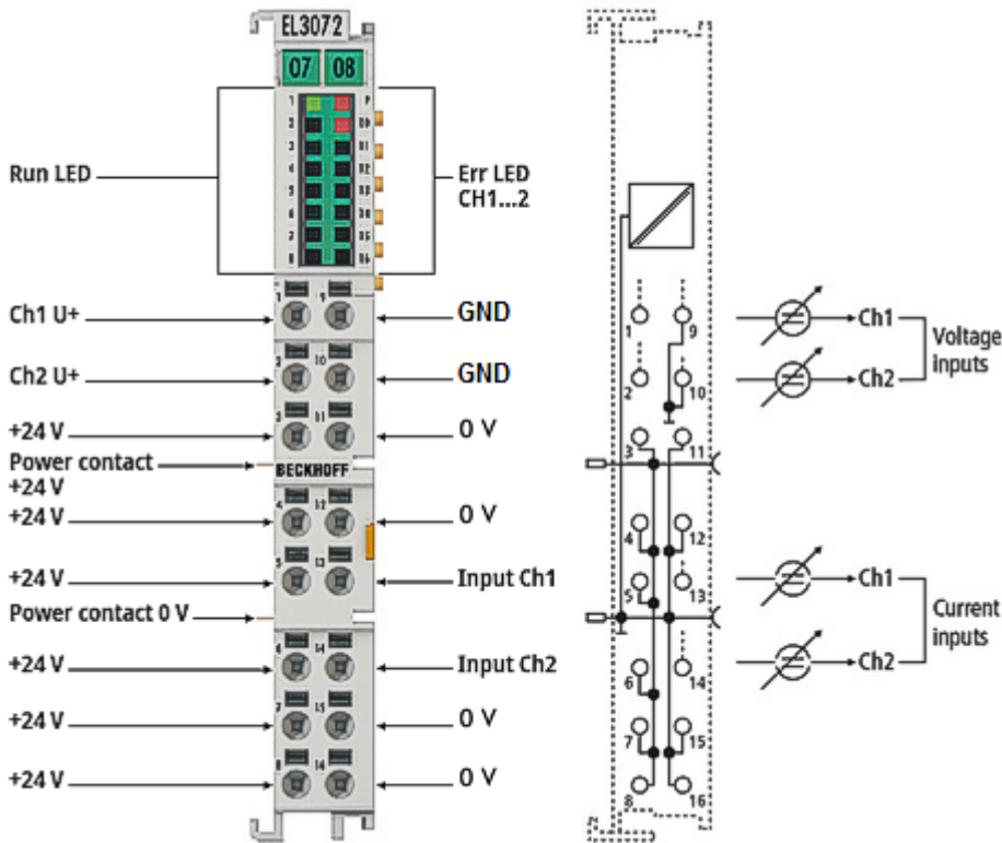
附图 50: EL3072
