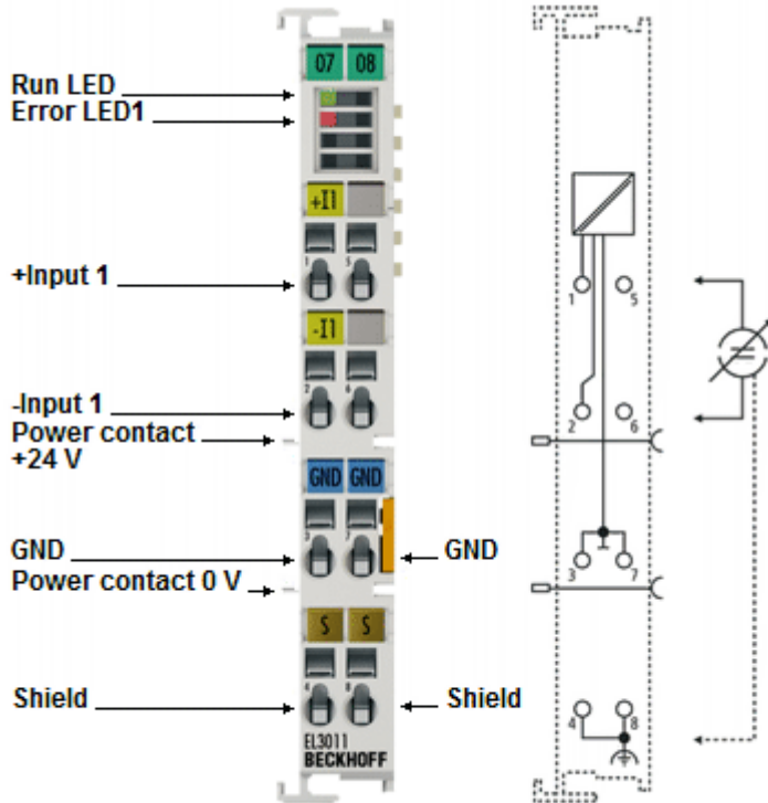
附图 12: EL3011
