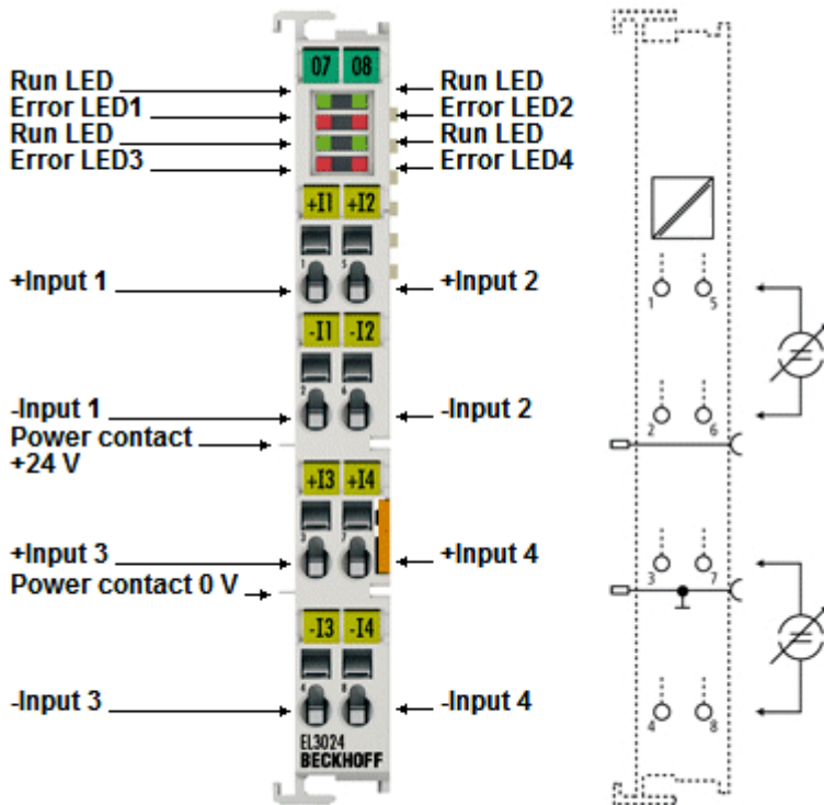
附图 22: EL3024
