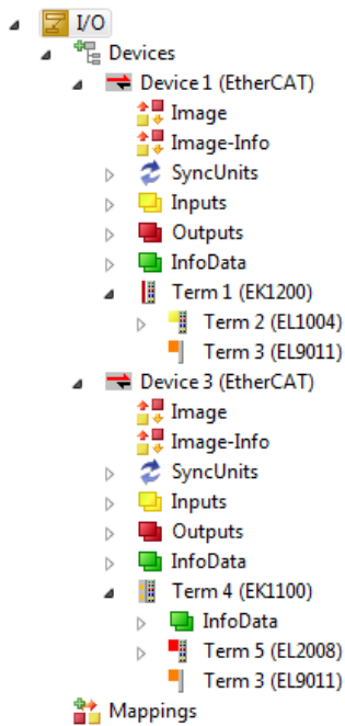
附图 99: 在集成于 VS shell 的TwinCAT 3 环境中配置映射
