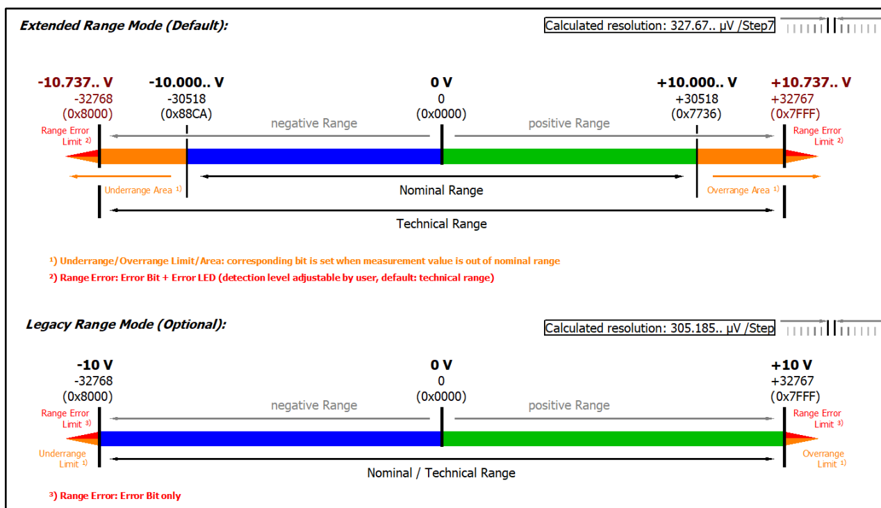
附图 200: EL3072、EL3074; 量程 -10...+10 V
