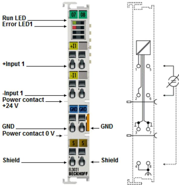
附图 19: EL3021 RUN 和 ERROR LED
