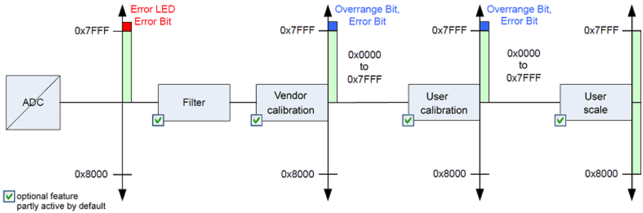
附图 197: 带校准计算的数据流 - EL301x、EL304x
