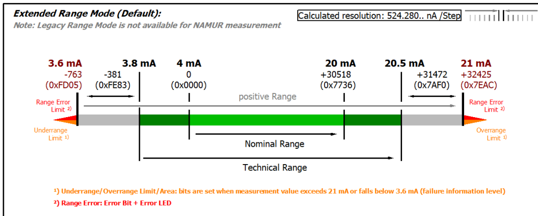
附图 205: EL3072、EL3074; 量程 4...20 mA (NAMUR NE43)
