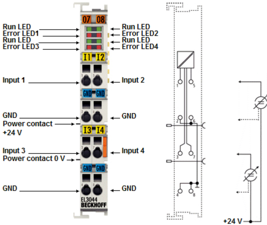
附图 29: EL3044 RUN 和 ERROR LED
