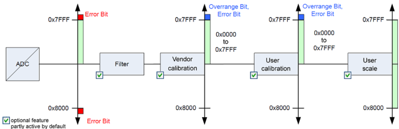
附图 199: 带校准计算的数据流 - EL306x
