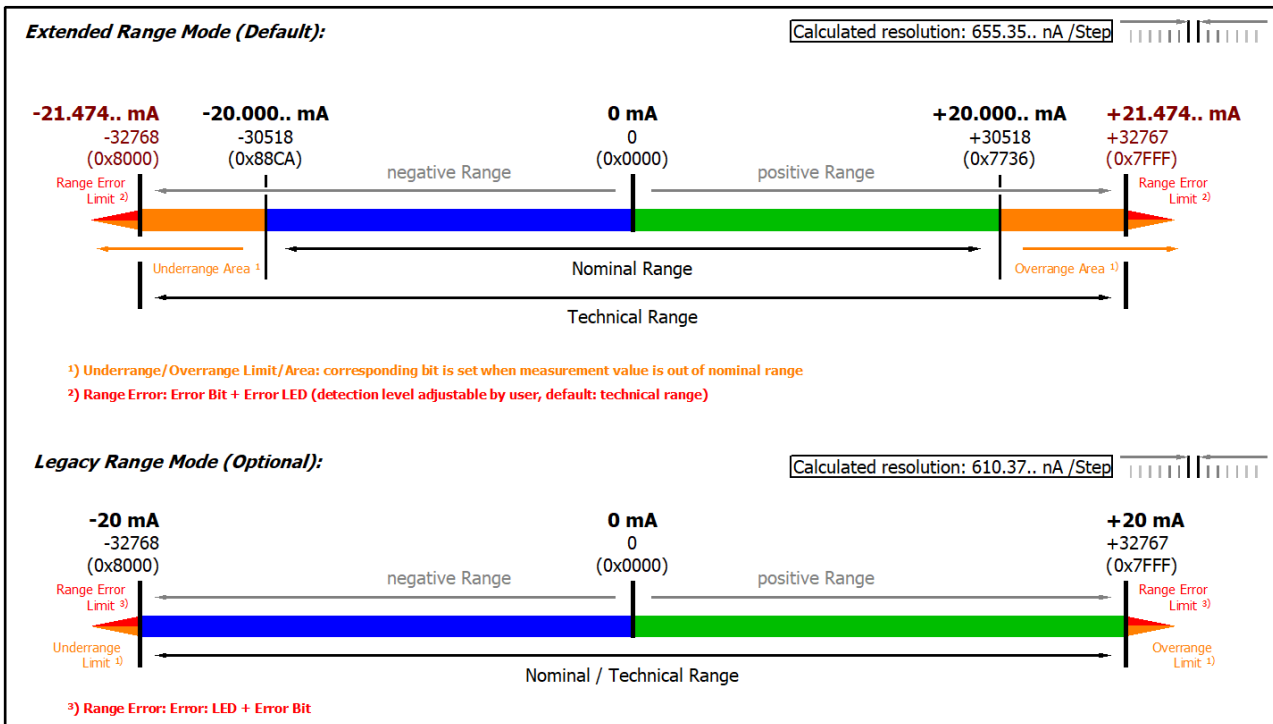
附图 202: EL3072、EL3074; 量程 -20...+20 mA
