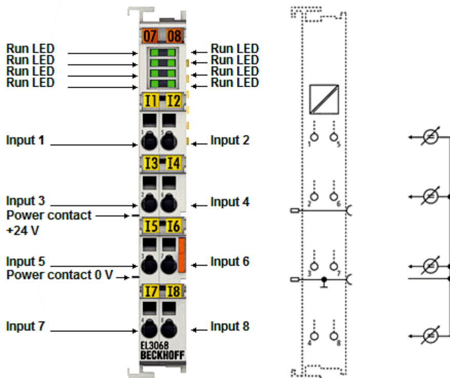
附图 48: EL3068
