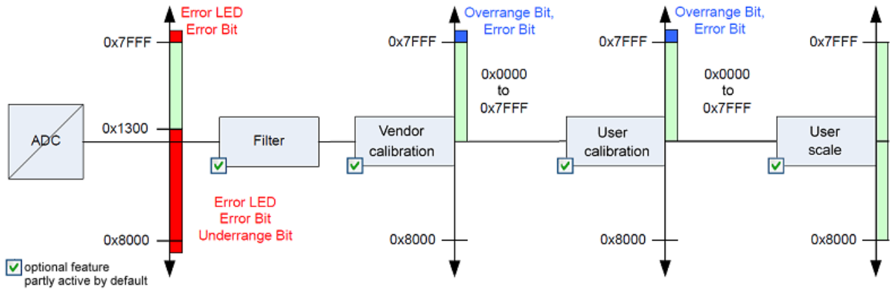
附图 198: 带校准计算的数据流 - EL302x、EL305x
