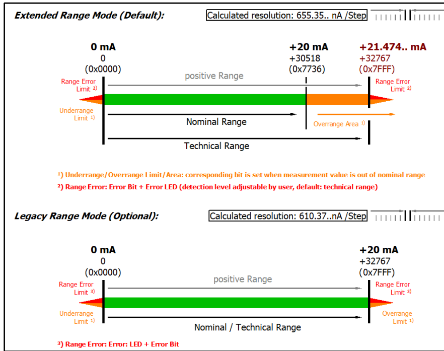
附图 203: EL3072、EL3074; 量程 0...20 mA
