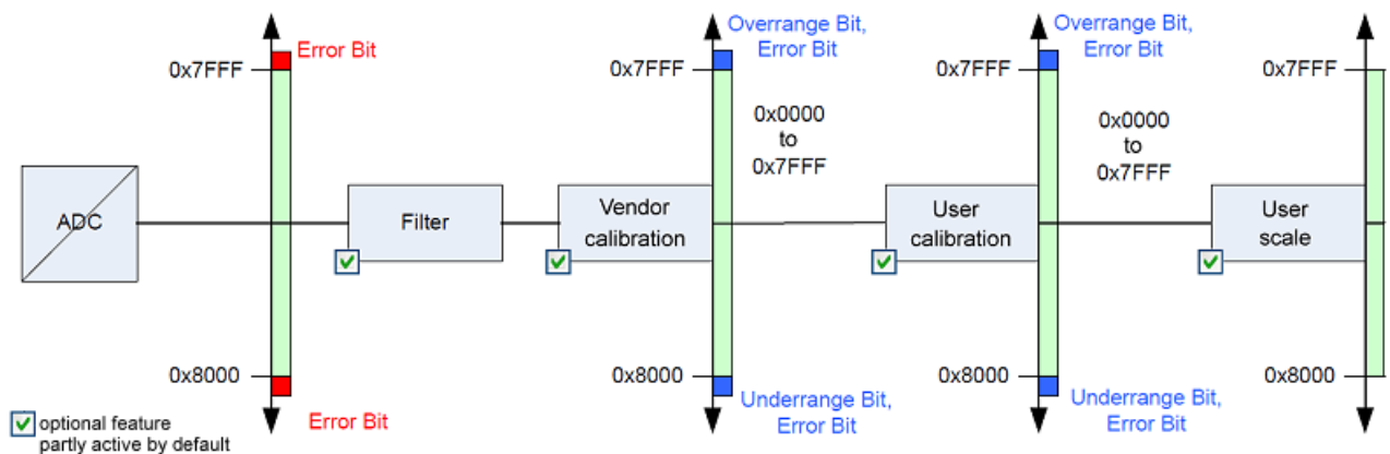
附图 196: 带校准计算的数据流 - EL300x
