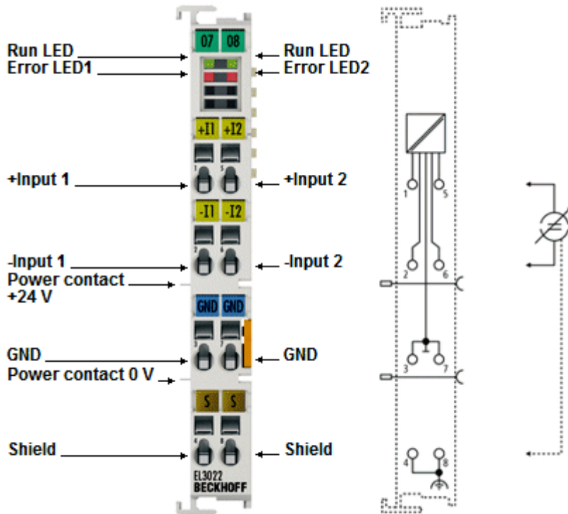
附图 20: EL3022
