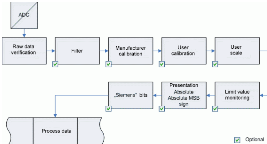
附图 195: EL30xx 数据流
