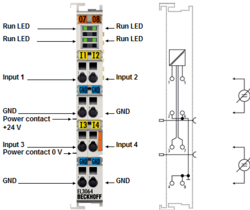
附图 46: EL3064
