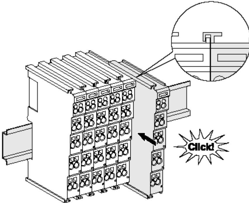
附图 62：安装在安装轨道上
