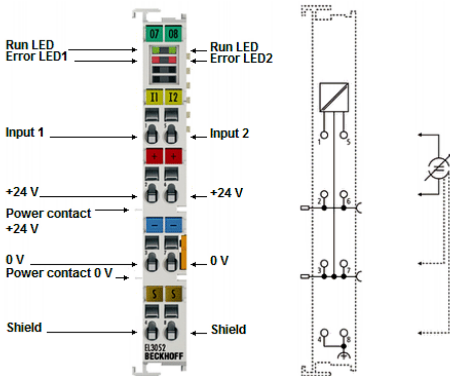
附图 35: EL3052 RUN 和 ERROR LED
