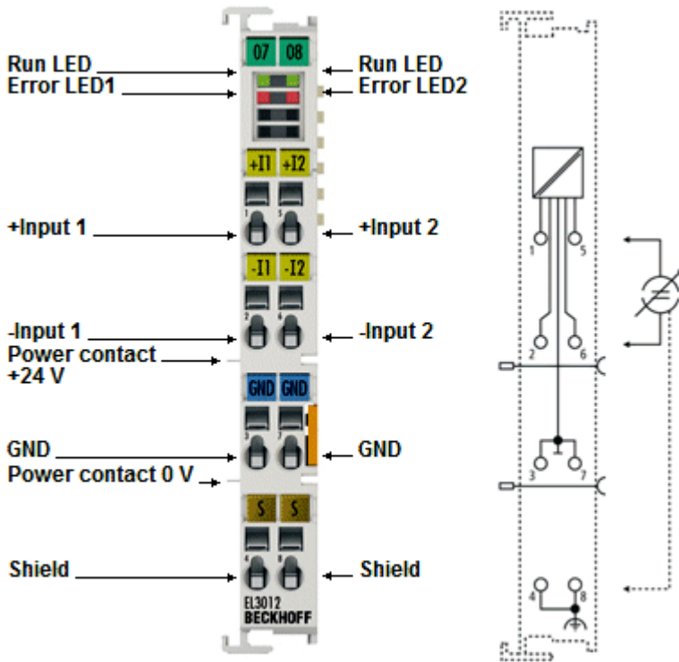
附图 15: EL3012 RUN 和 ERROR LED
