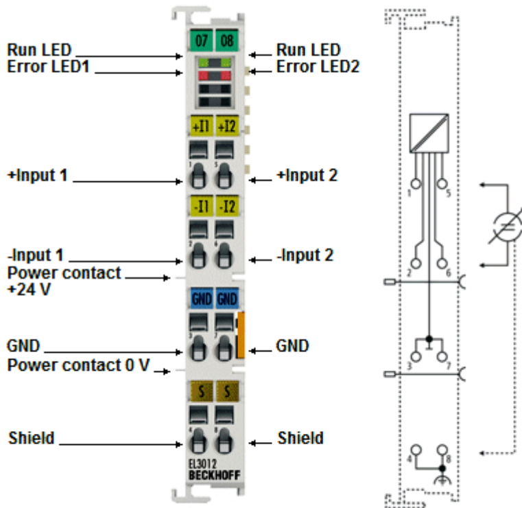
附图 14: EL3012
