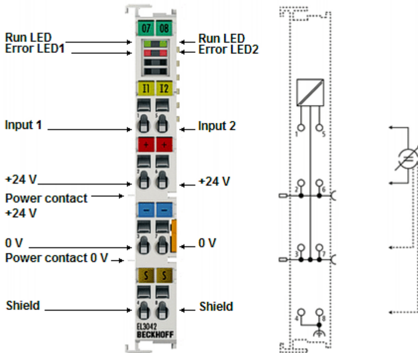
附图 26: EL3042
