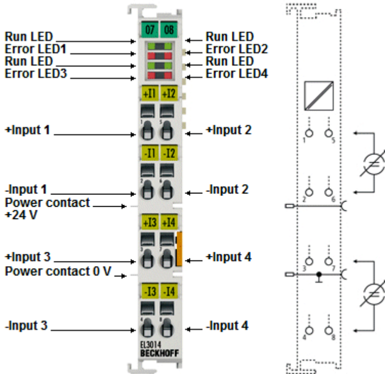
附图 17: EL3014 RUN 和 ERROR LED
