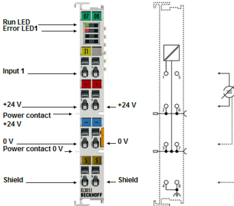
附图 32: EL3051
