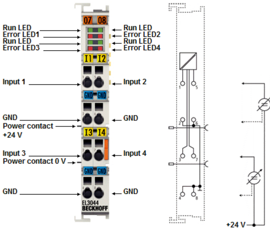
附图 28: EL3044
