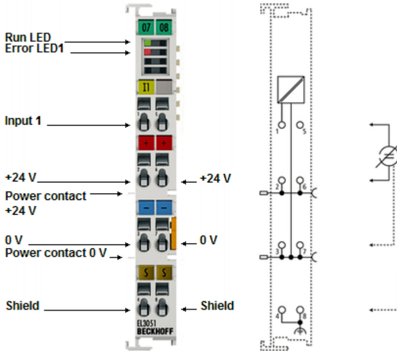
附图 33: EL3051 RUN 和 ERROR LED
