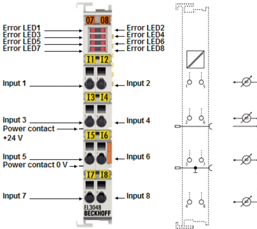
附图 30: EL3048
