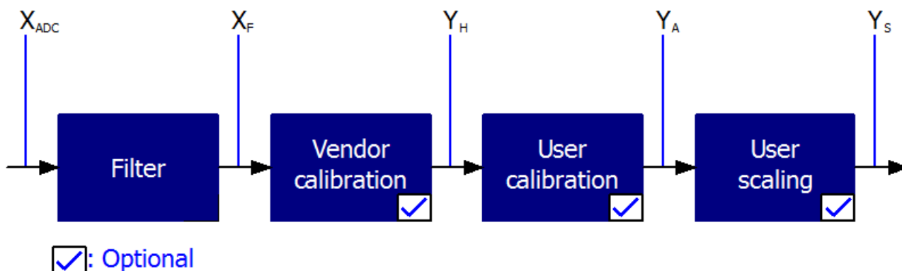
附图 206: 过程数据的计算
