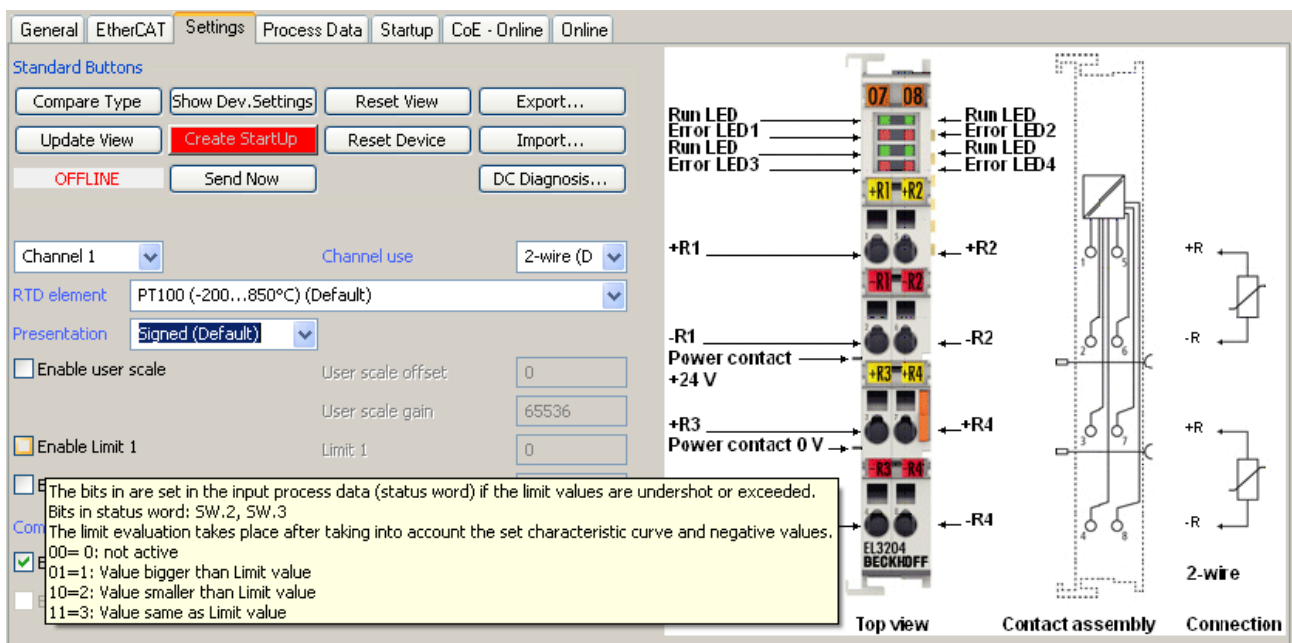
附图 176: EL3204 调试助手示例
