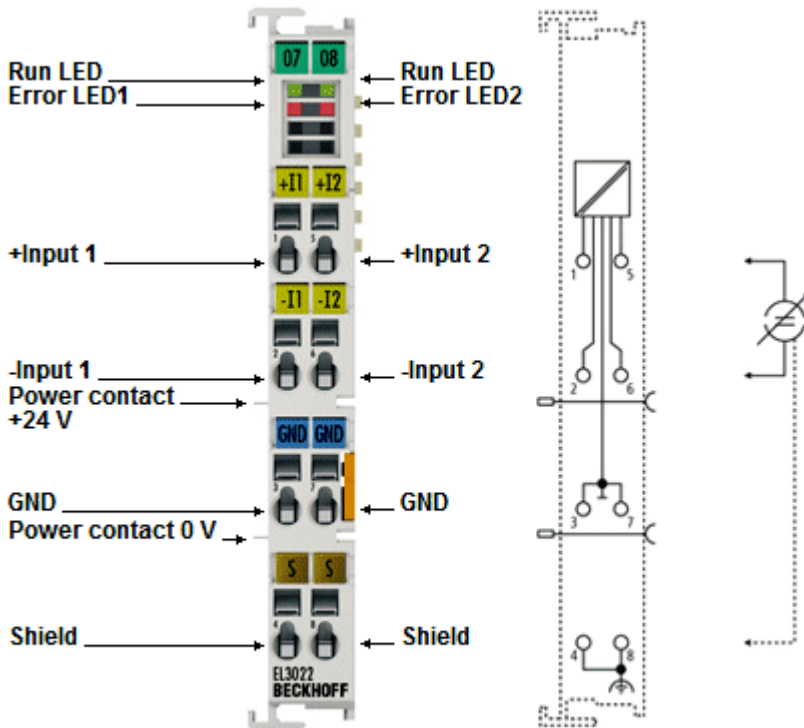
附图 21: EL3022 RUN 和 ERROR LED
