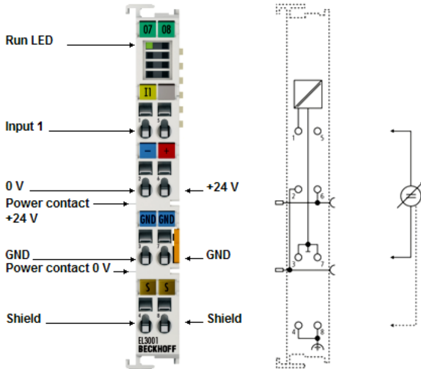
附图 4: EL3001
