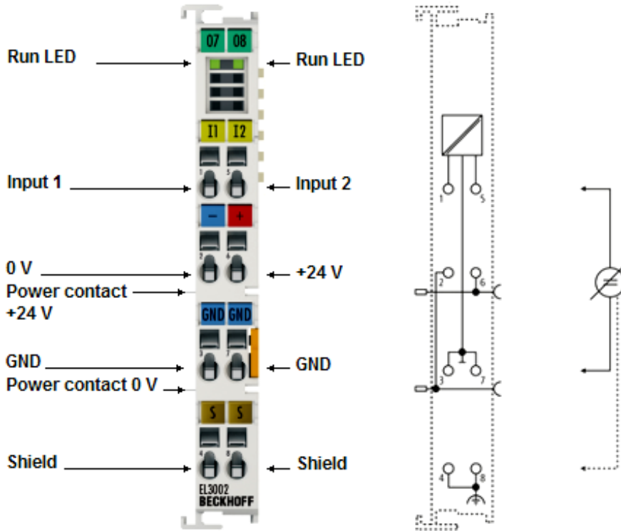
附图 7: EL3002 LED 和连接
