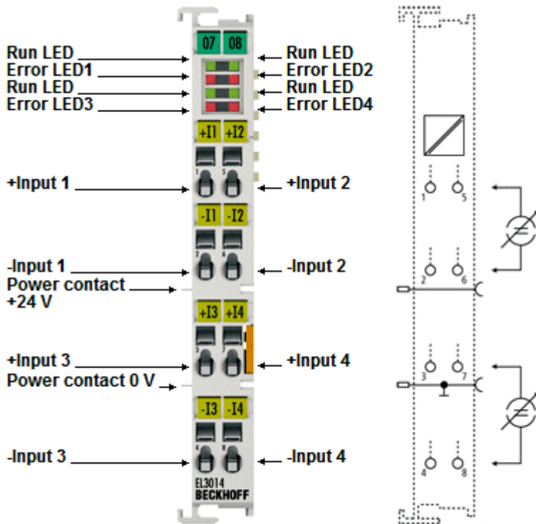
附图 16: EL3014
