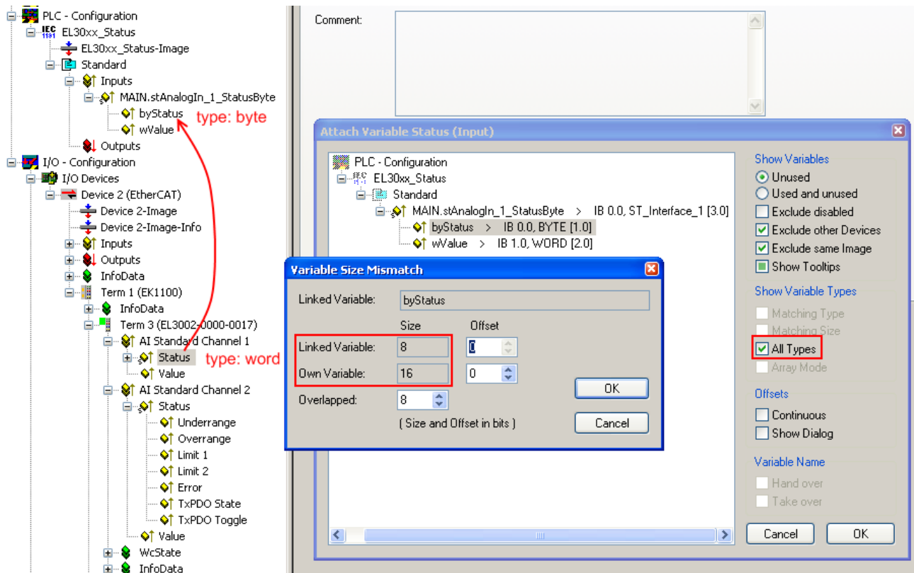
附图 190: 将 EL31xx/EL30xx 的 4 字节接口连接到项目中已有的 3 字节接口
