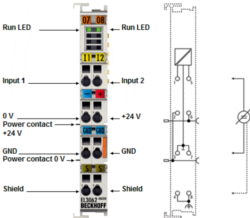
附图 44: EL3062-0030
