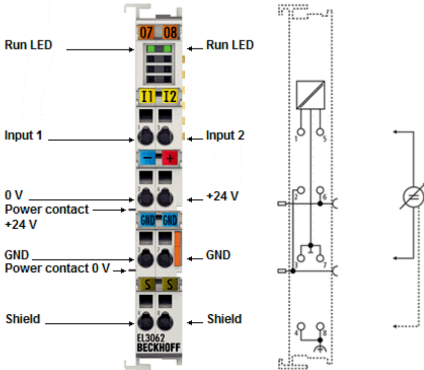
附图 42: EL3062
