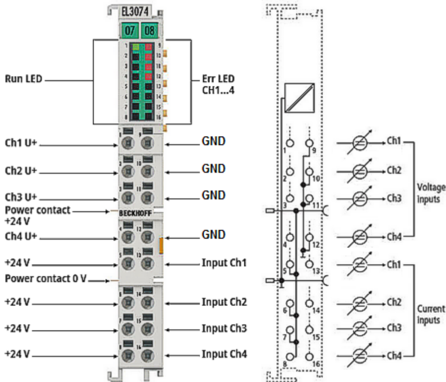
附图 52: EL3074
