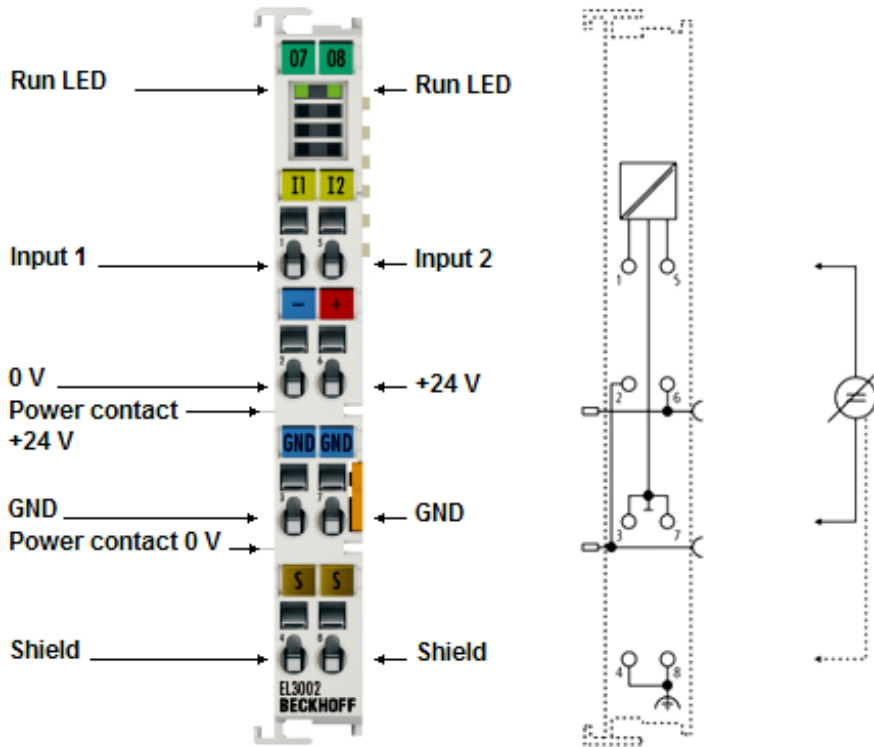
附图 6: EL3002
