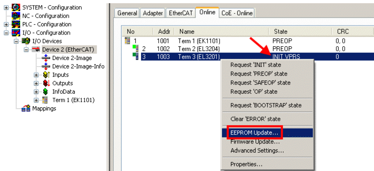
Abb. 138: EEPROM Update
