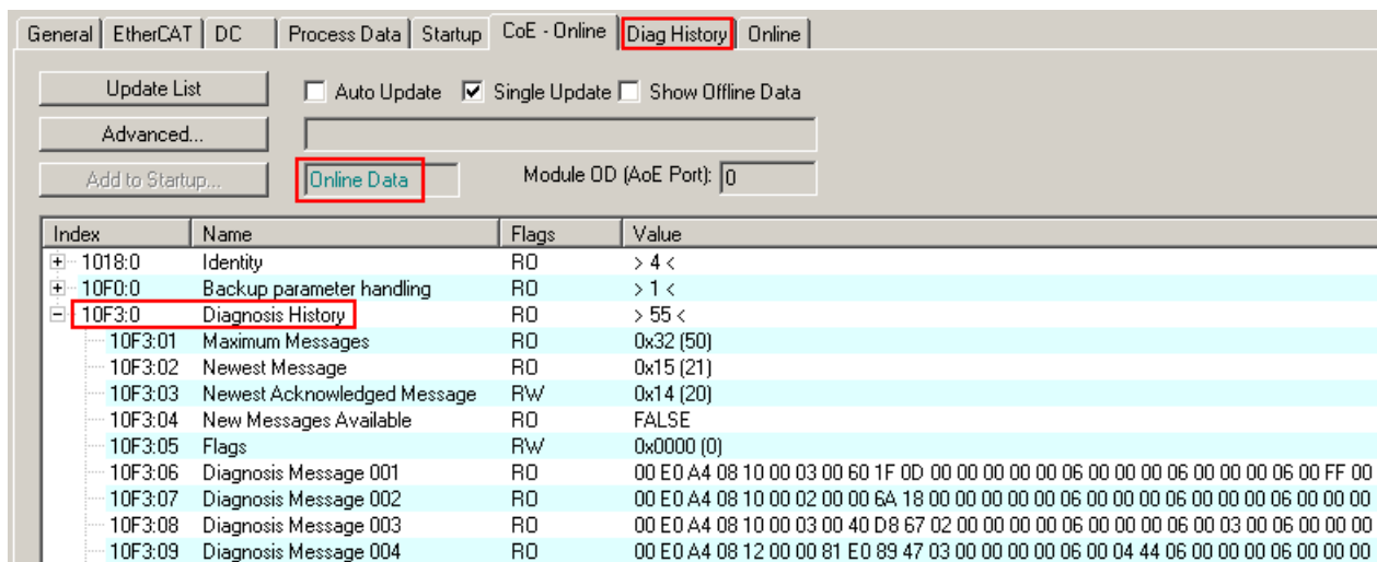
Abb. 141: DiagMessages im CoE
