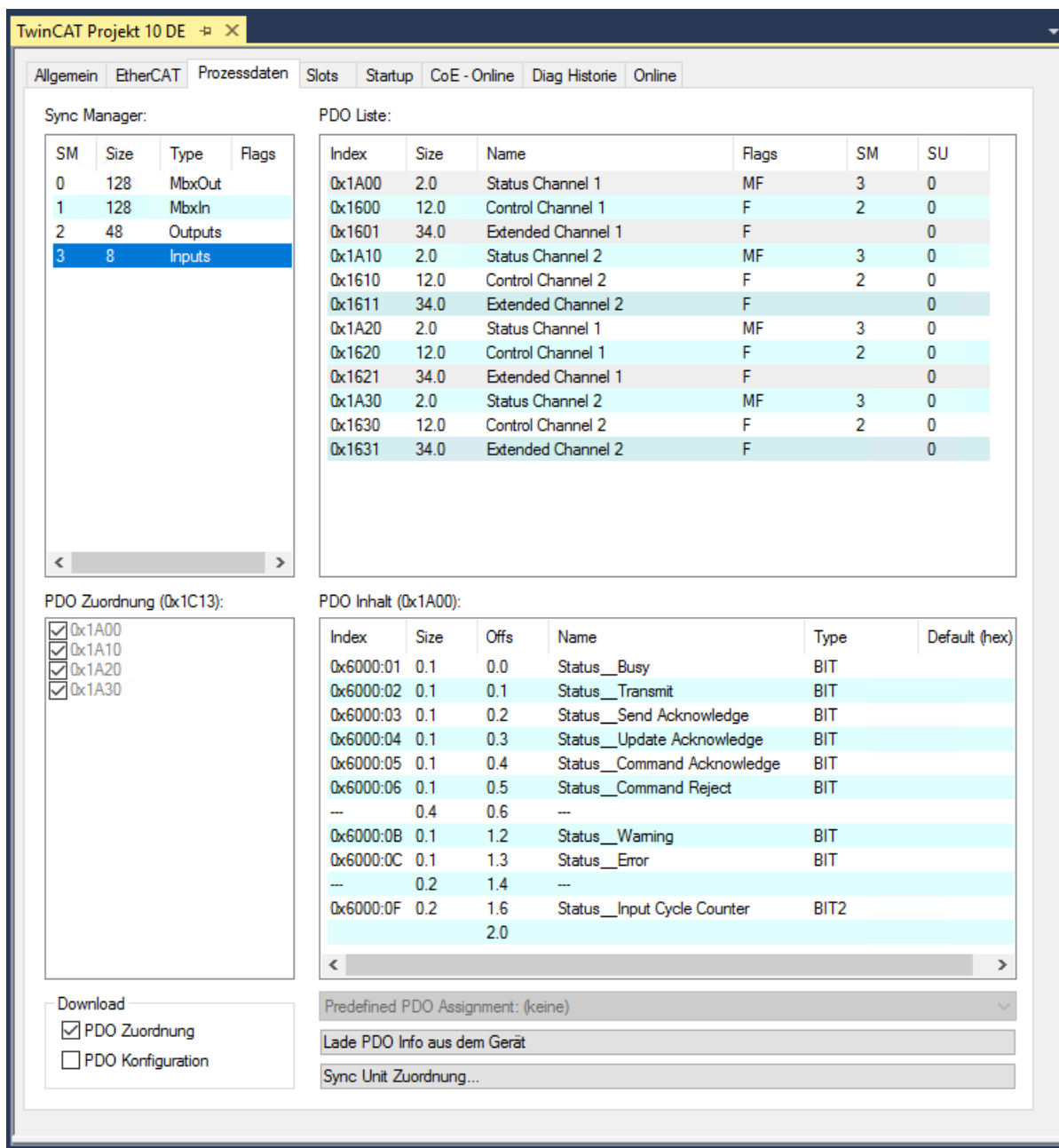
Abb. 139: EL2574 – Prozessdaten Input SyncManager (SM3)
