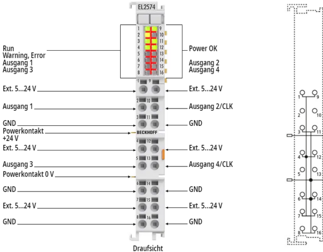
Abb. 4: EL2574 Anschlussbelegung
