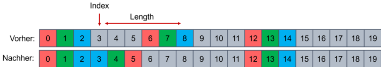
Abb. 134: Beispiel Kommando 0x07 „Reverse“
