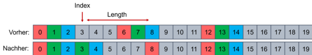
Abb. 133: Beispiel Kommando 0x06 „Rotate Right“
