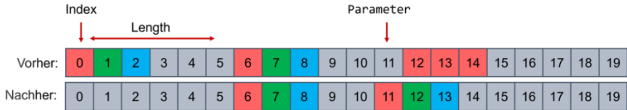
Abb. 132: Beispiel Kommando 0x04 „Move“
