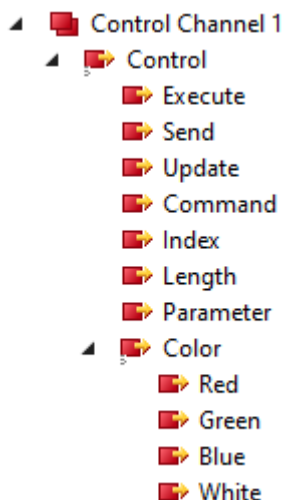
Abb. 128: EL2574 - Default - Prozessdatenanzeige im TwinCAT-Baum „Control Channel 1“
