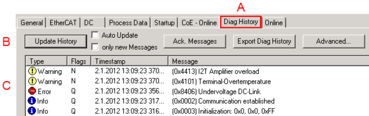
Abb. 142: Implementierung DiagMessage-System im TwinCAT System Manager
