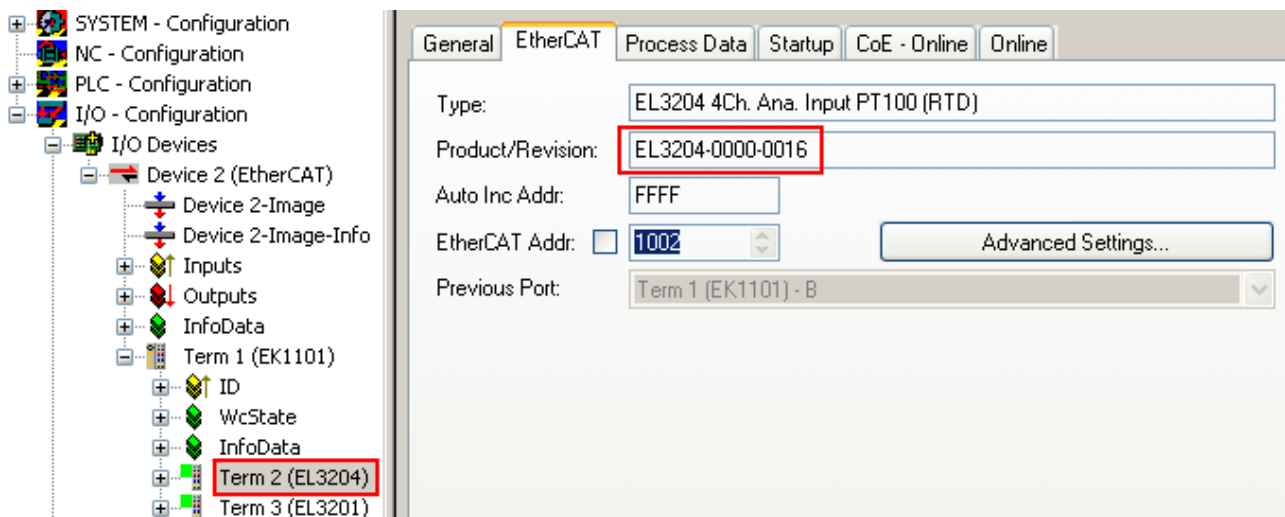
Abb. 153: Geräteerkennung aus Name EL3204-0000 und Revision -0016
