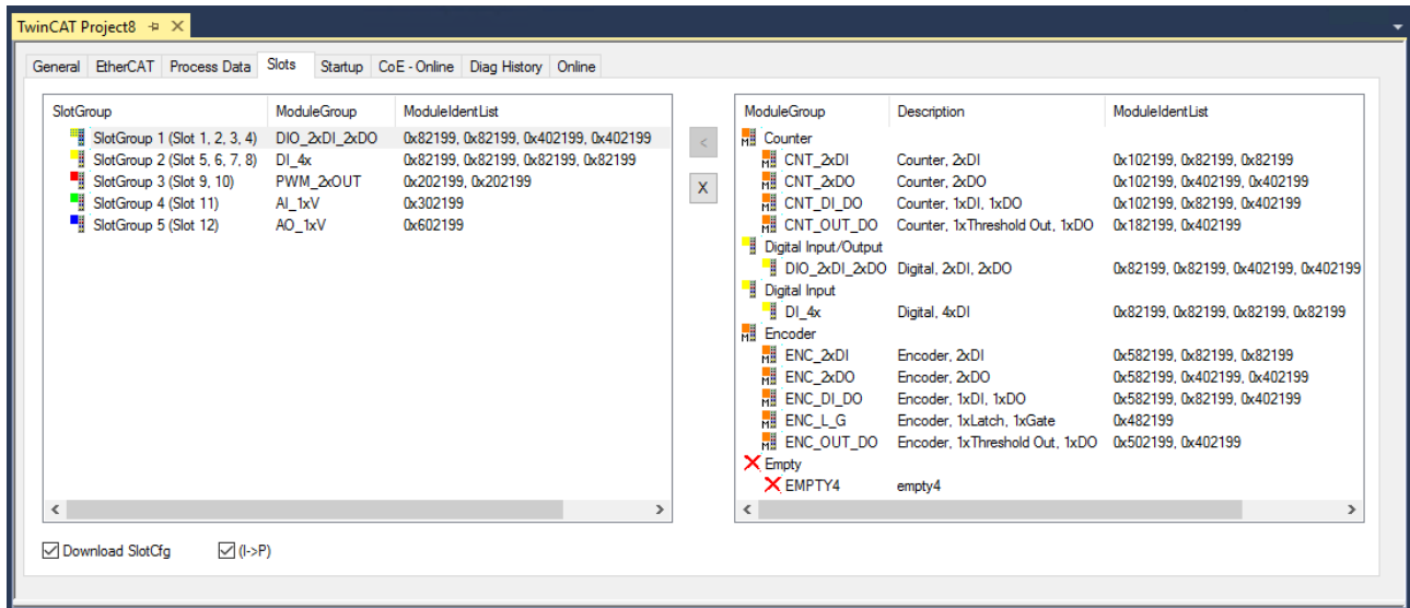
Abb. 126: Reiter „Slots“ am Beispiel EL8601-8411
