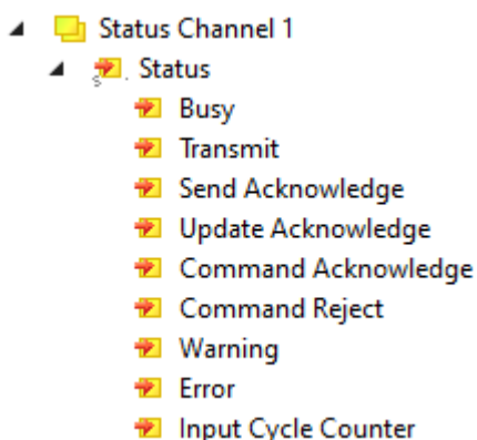
Abb. 137: EL2574 - Anzeige der Status-Informationen im TwinCAT-Baum
