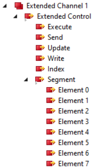
Abb. 136: EL2574 - Prozessdatenanzeige im TwinCAT-Baum „Extended Channel 1“
