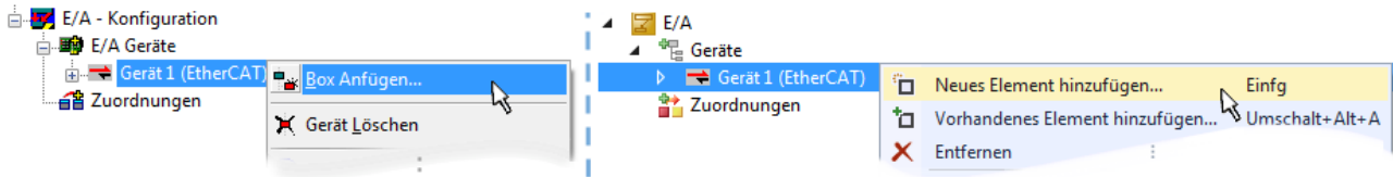
Abb. 55: Anfügen von EtherCAT-Geräten (links: TwinCAT 2; rechts: TwinCAT 3)
