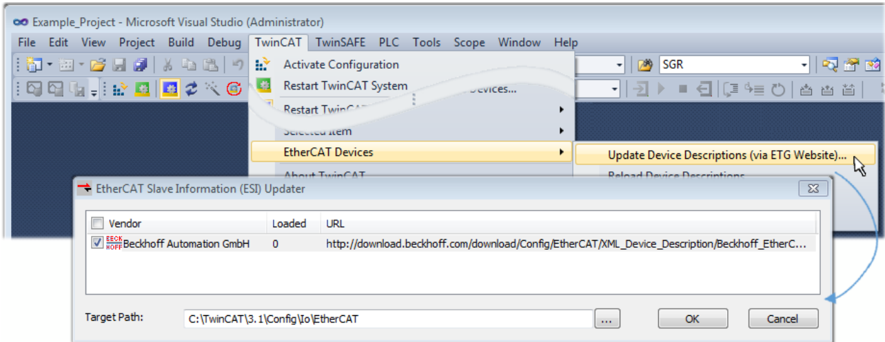
Abb. 50: Anwendung des ESI Updater (TwinCAT 3)
