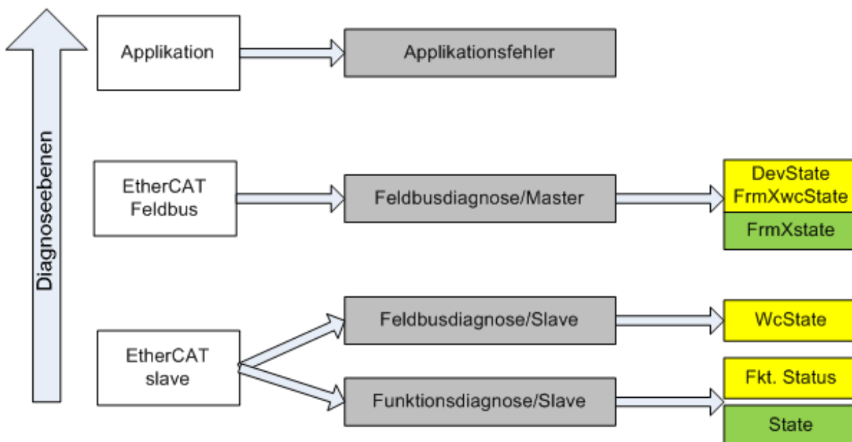
Abb. 87: Auswahl an Diagnoseinformationen eines EtherCAT-Slaves
