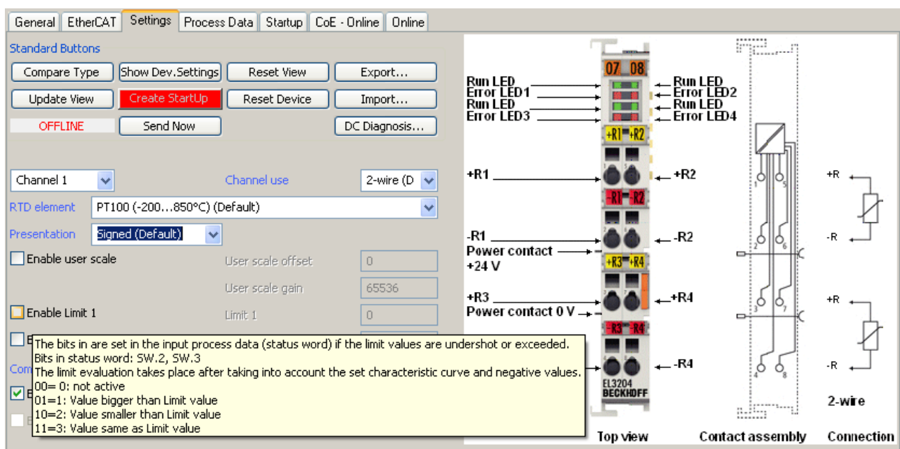
Abb. 90: Beispiel Inbetriebnahmehilfe für eine EL3204
