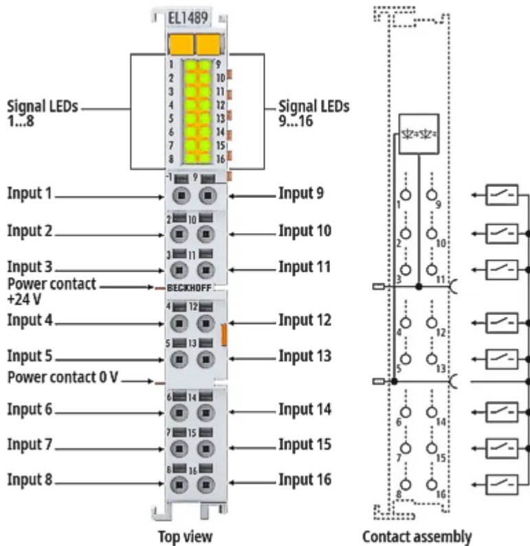
Abb. 4: EL1489
