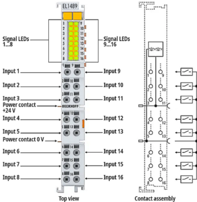
Abb. 5: EL1489
