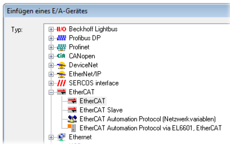
Abb. 81: Auswahl EtherCAT Anschluss (TwinCAT 2.11, TwinCAT 3)
