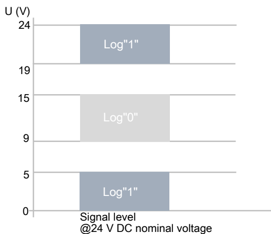
Abb. 5: Schaltcharakteristik Signalspannung „0“ und „1“:
