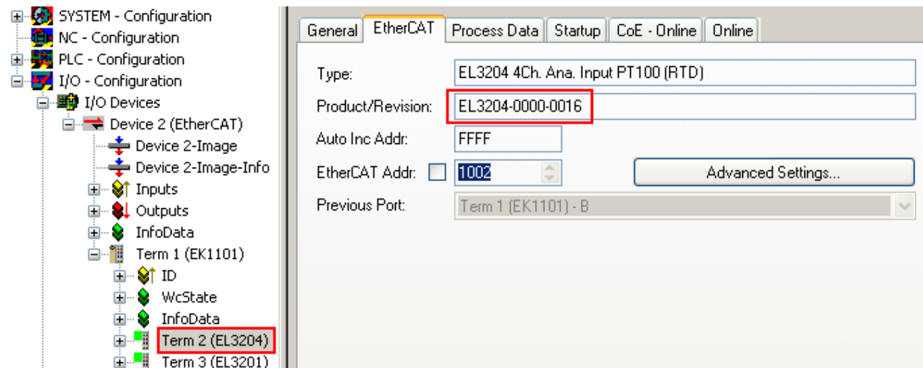
Abb. 130: Geräteerkennung aus Name EL3204-0000 und Revision -0016
