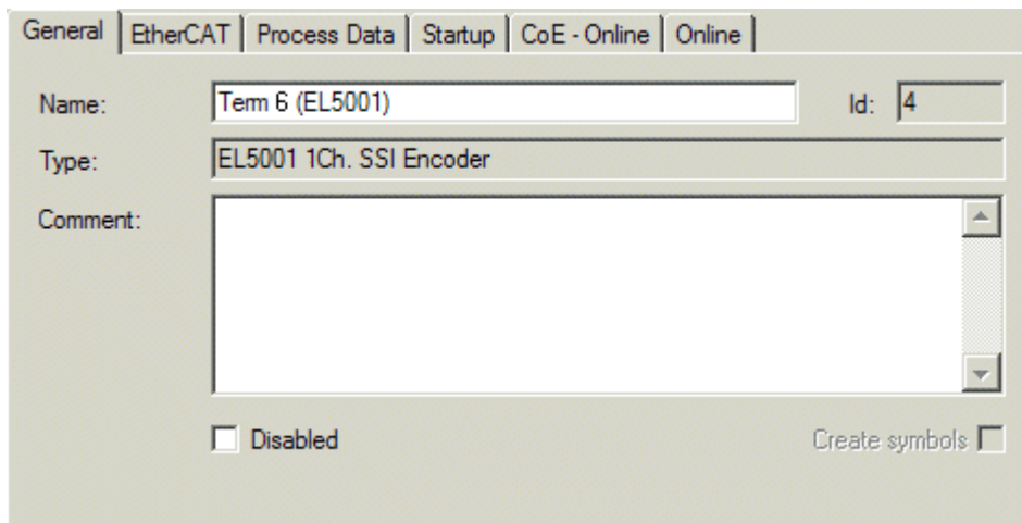
附图 113: “General(常规)” 选项卡
