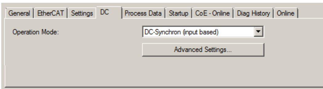
附图 121: “DC” 选项卡（分布时钟）
