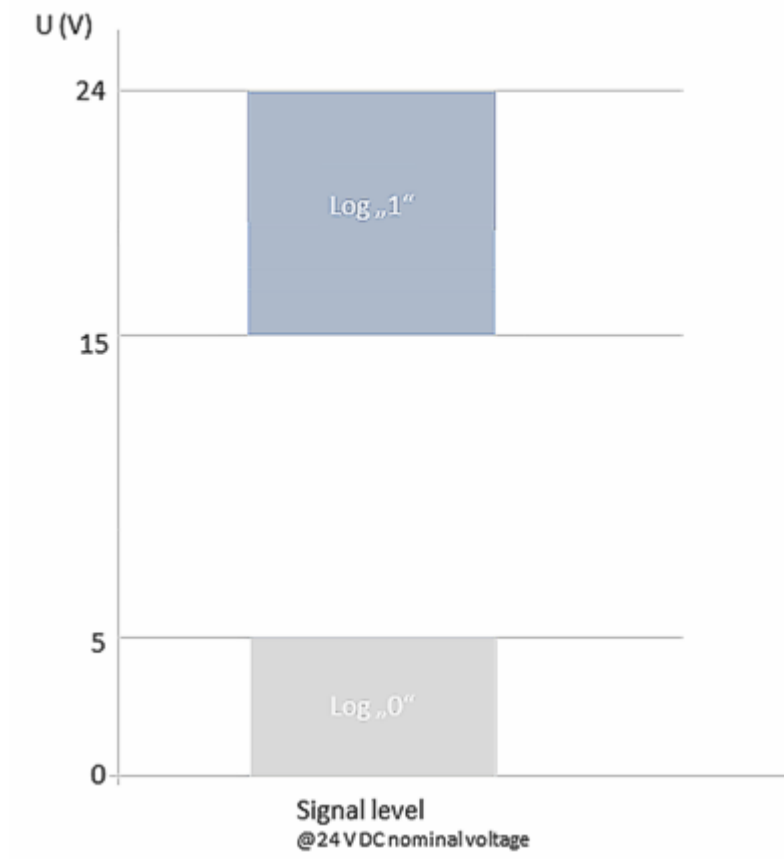
附图 5: 开关特性信号电压“0”和“1”
