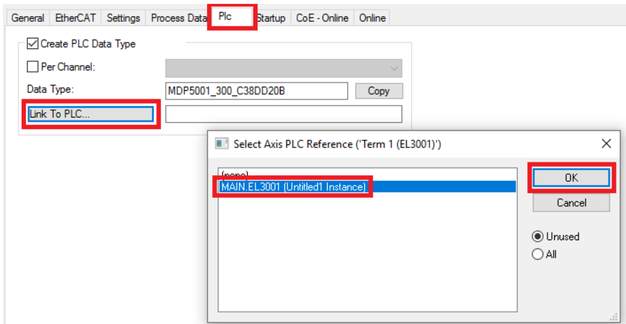
附图 61: 结构体的链接
