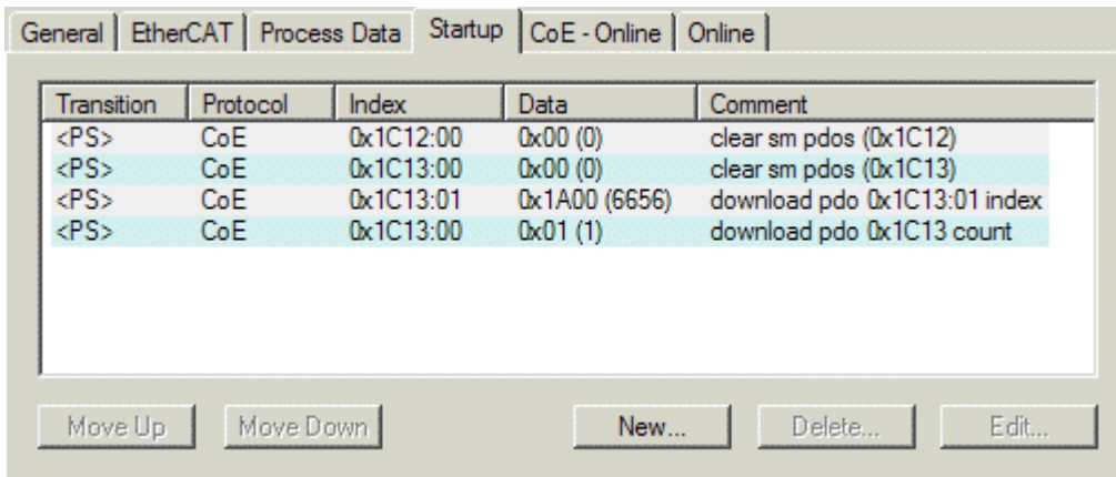
附图 117: “Startup（启动）”选项卡
