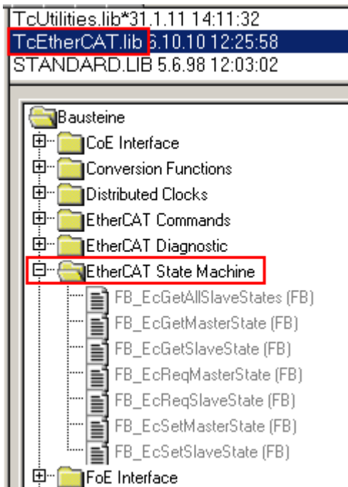
附图 128: PLC 功能块
