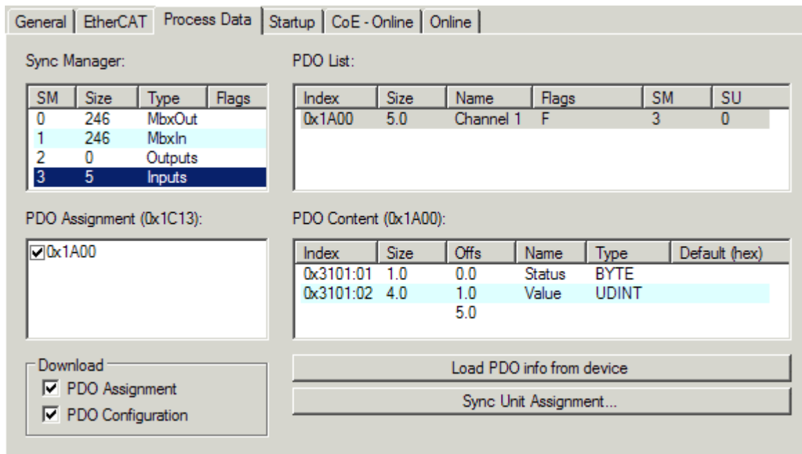
附图 115: “Process Data (过程数据)” 选项卡
