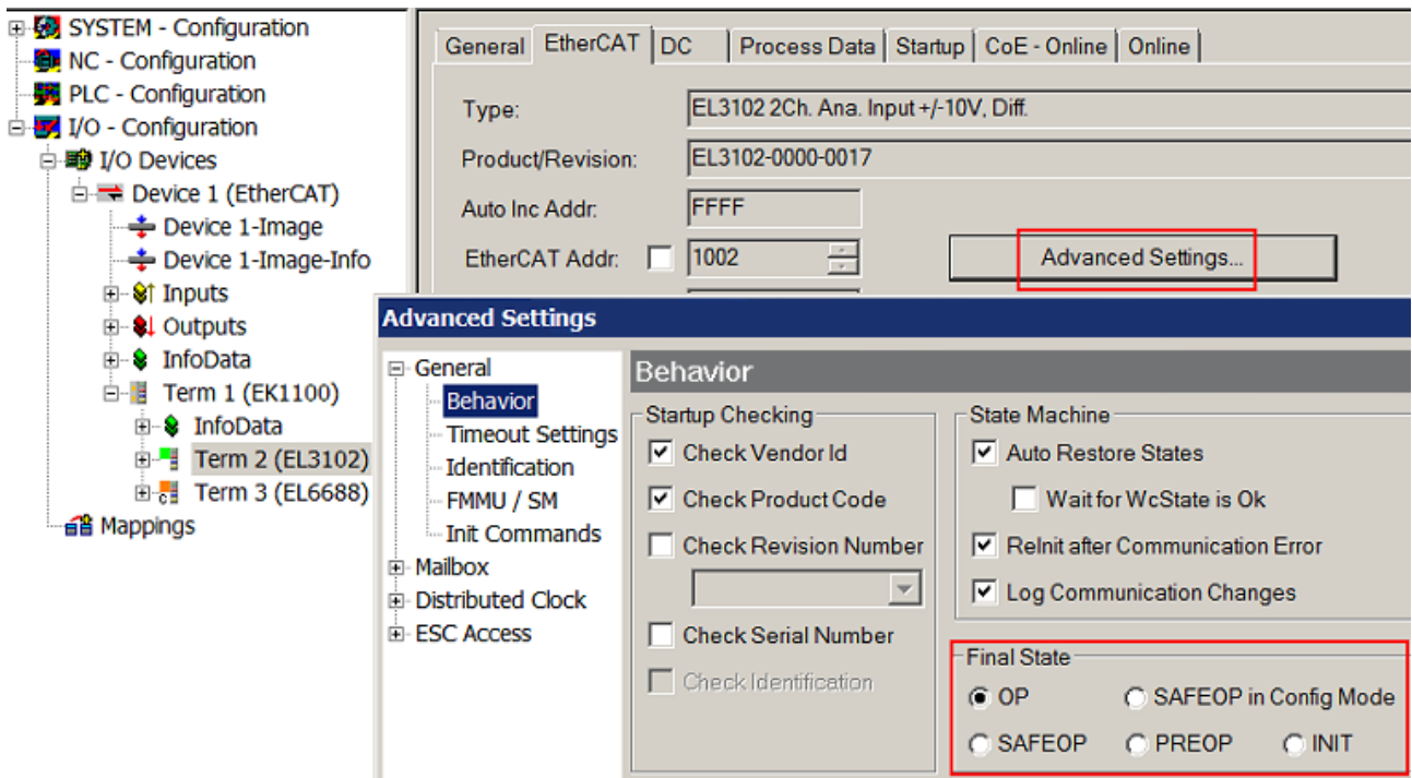
附图 127: 从站的默认目标状态
