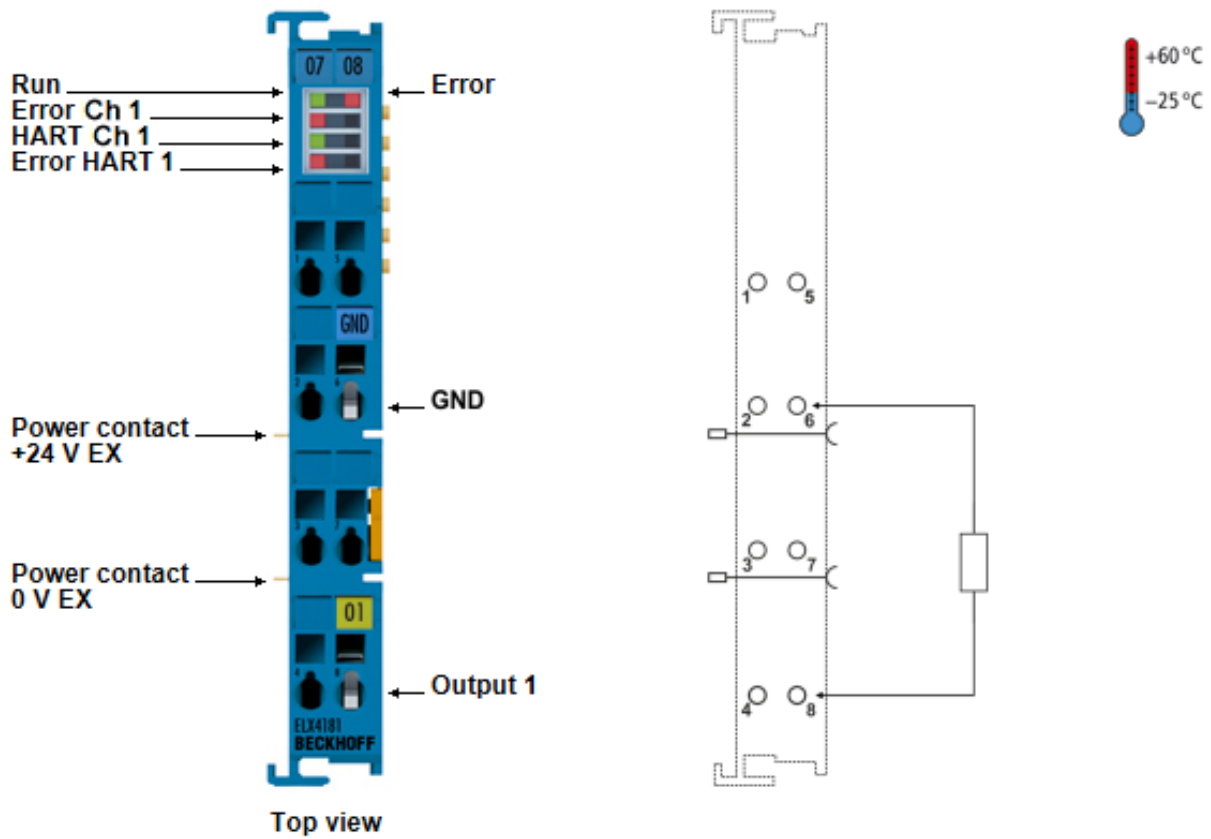
附图 20: ELX4181 - 触点分配
