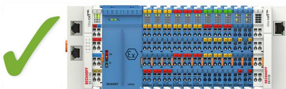
附图 7: 允许的安装 - 不属于 ELX 系列的端子模块被放置在 ELX 端子模块网段的前后。由 ELX 端子模块网段开头的 ELX9560 和 ELX 端子模块网段末端的 EK1110 隔离。
