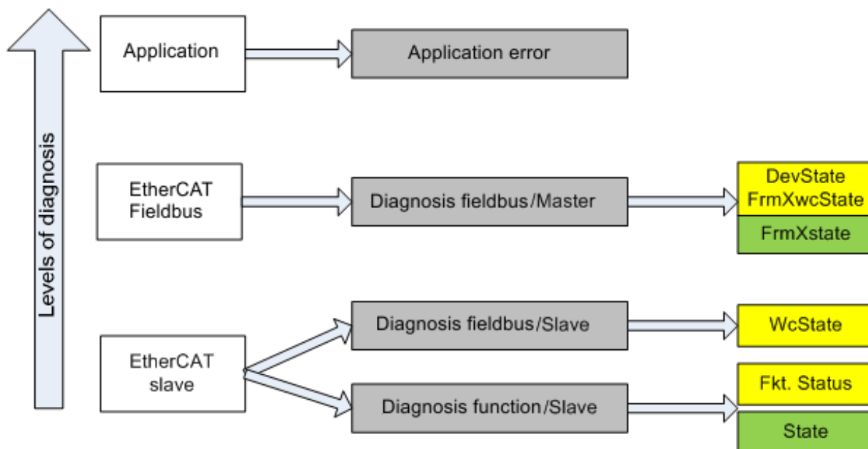
附图 131: 选择 EtherCAT 从站的诊断信息
