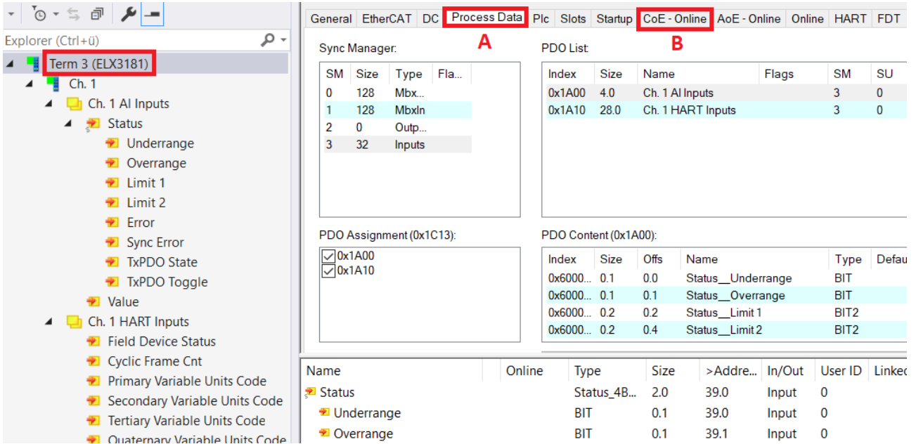
附图 140: ELX3181 - 参数化
