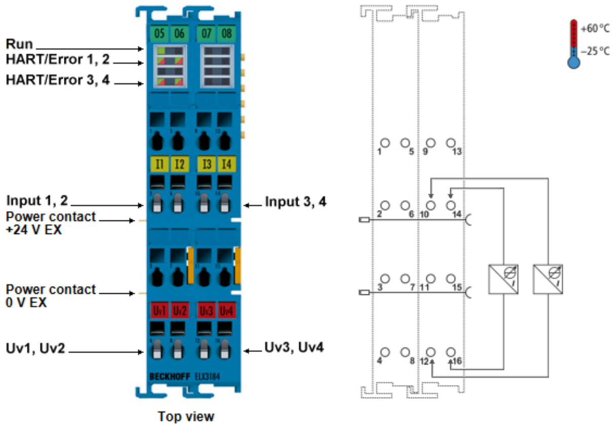
附图 22: ELX3184 - 触点分配
