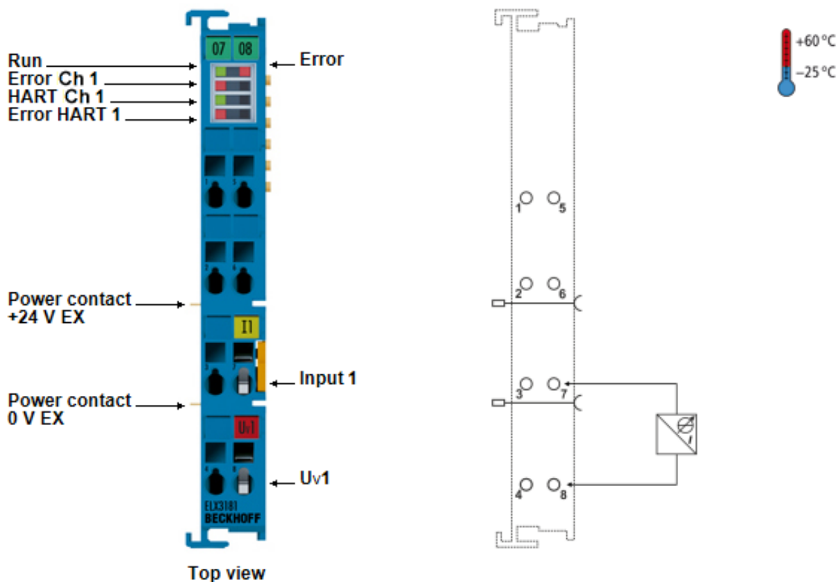
附图 4: ELX3181 - 1 通道模拟量输入端子 4...20 mA, 单端, 16 位, HART, Ex i
