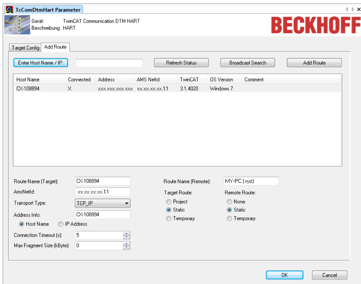
附图 163: FDT 应用程序的 Beckhoff DTM 中的 AddRoute 对话框
