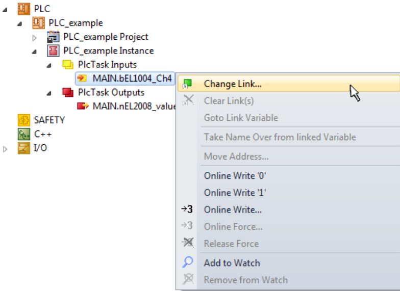
附图 65: 在PLC变量和过程对象之间建立联系
