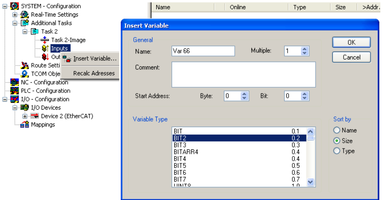
附图 142: 将 2 位变量链接至附加任务
