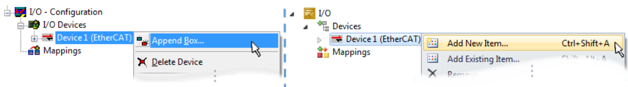
附图 94: 添加EtherCAT设备 (左: TwinCAT 2; 右: TwinCAT 3)
