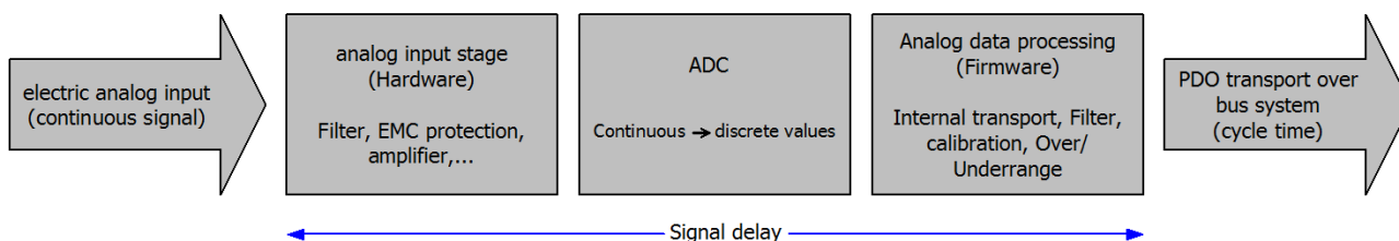
附图 28: 信号处理模拟输入
