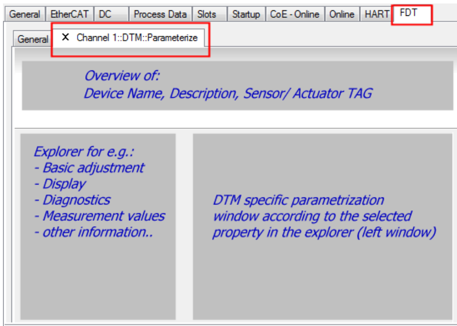
附图 158: 现场设备工具 (FDT) 中 DTM 配置窗口的一般结构
