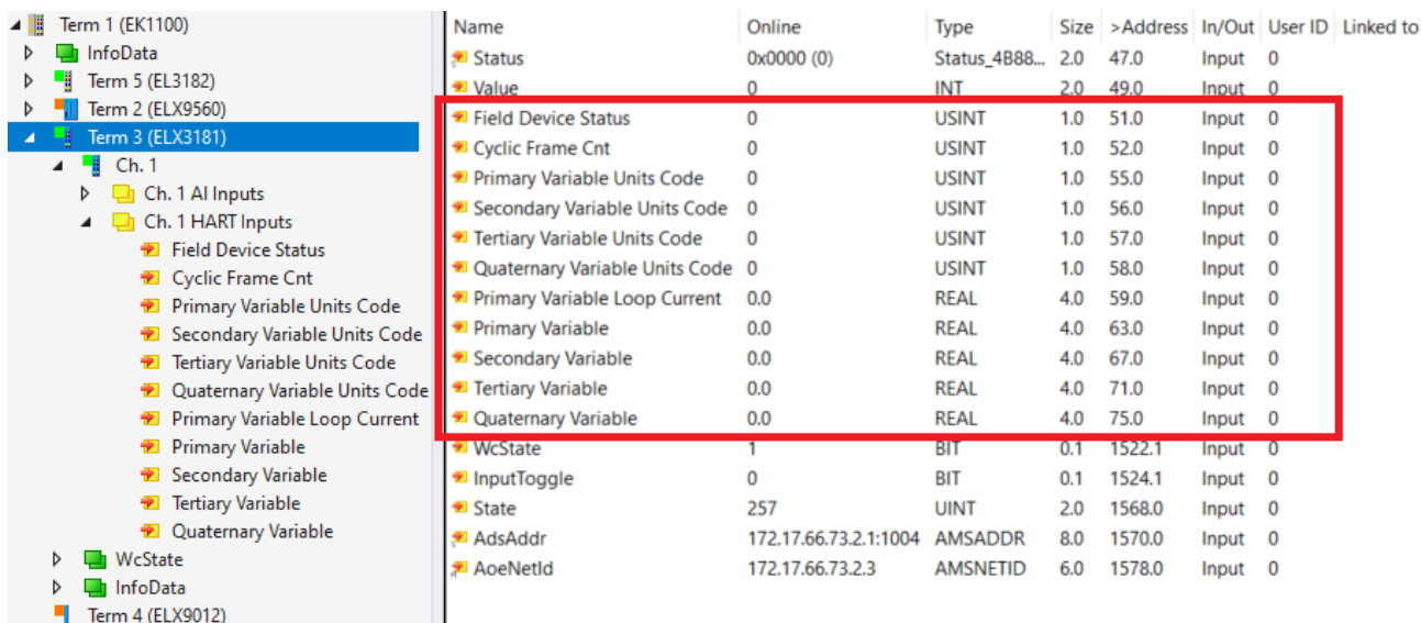
附图 155: HART 通信的附加 PDO (Cmd 3)
