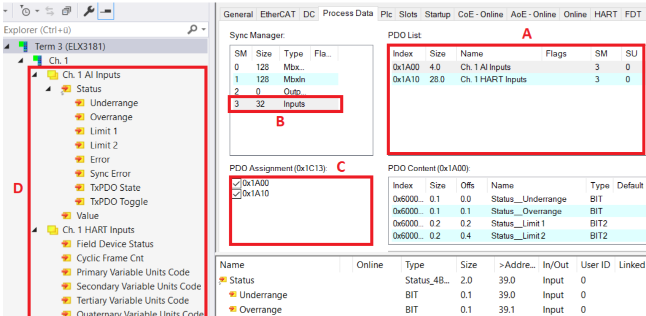
附图 148: 选择性 PDO 选择
