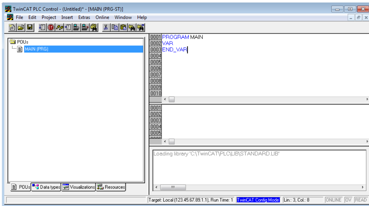
附图 41: 启动后的TwinCAT PLC控制
