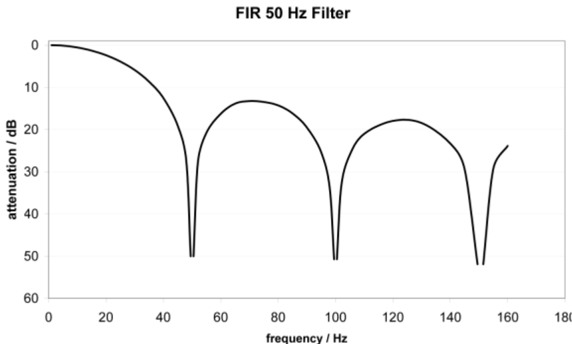
附图 144: 50 Hz 时的衰减曲线陷波滤波器
