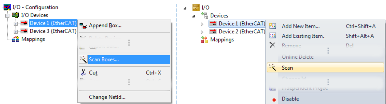
附图 108: 在一个指定的 EtherCAT 设备上手动触发设备扫描（左：TwinCAT 2；右：TwinCAT 3）
