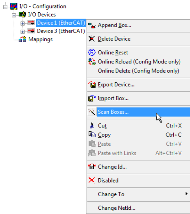
附图 40: 读取连接到设备的单个终端
