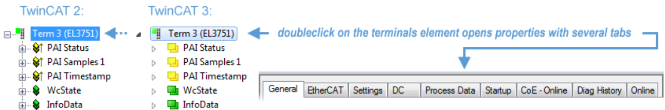
附图 121: 终端EL3751的分支元件
