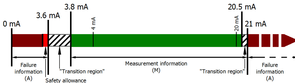
附图 31: NAMUR建议NE43中定义的表述（2003年2月3日版本）
