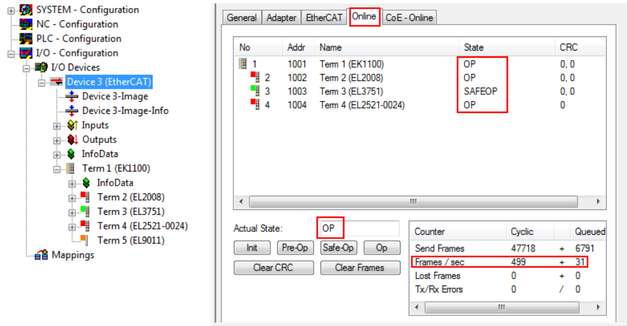
附图 113: 在线显示示例
