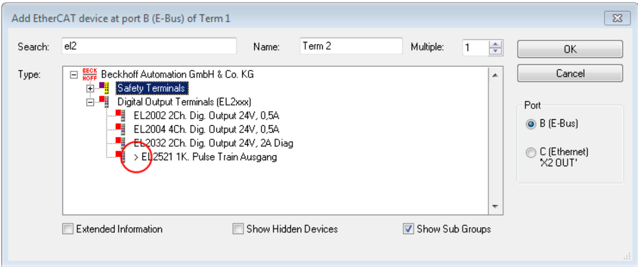
附图 86: 以EL2521在线记录ESI为例进行说明
