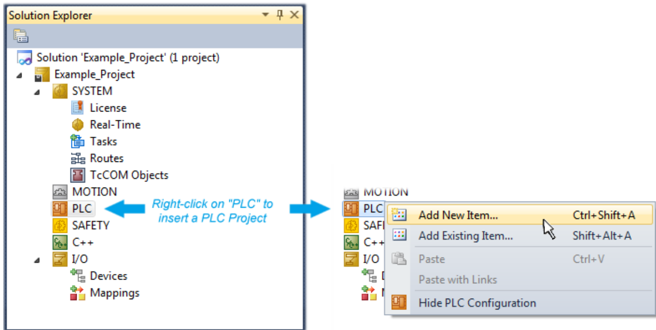
附图 60: 在“PLC”中添加编程环境
