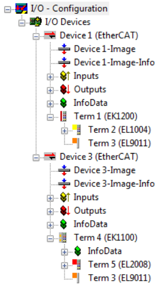
附图 39: TwinCAT 2系统管理器中的配置映射
