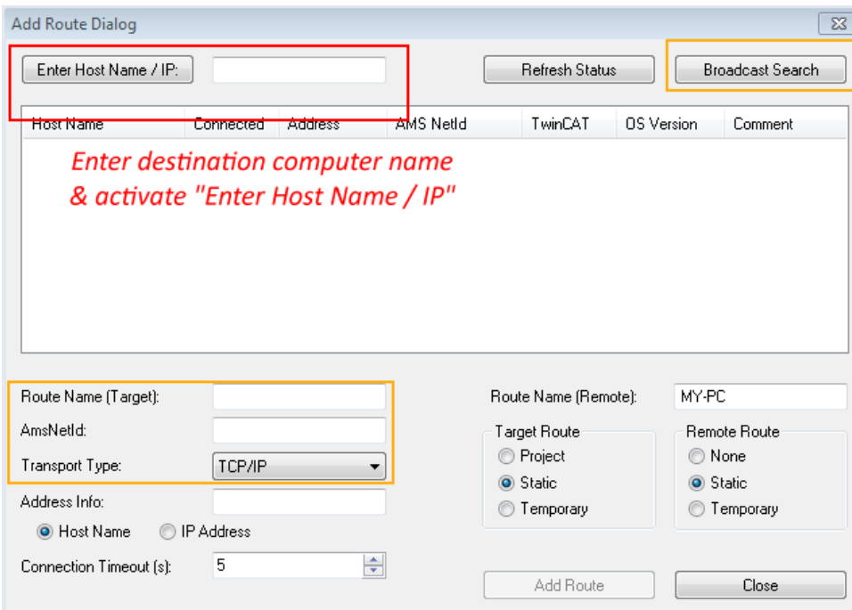
附图 55: 为TwinCAT系统管理器指定访问的PLC：选择目标系统
