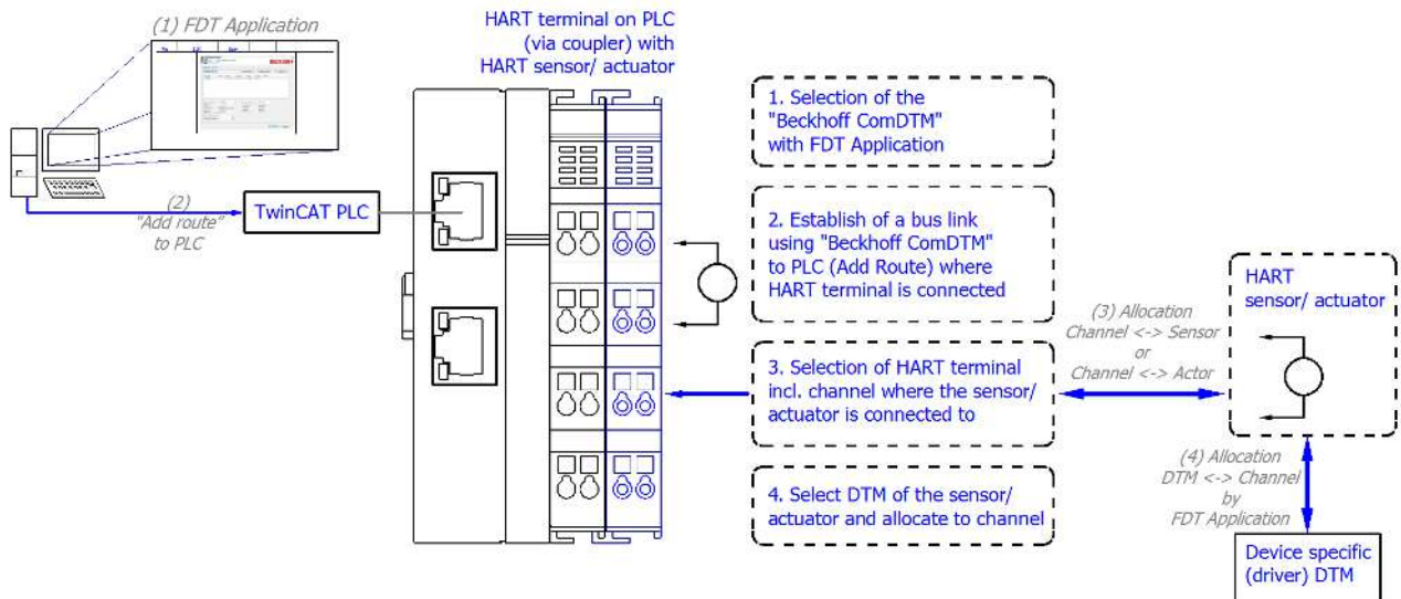
附图 166: 通过 Beckhoff_ComDTM 访问 HART DTM 的 FDT 应用的程序
