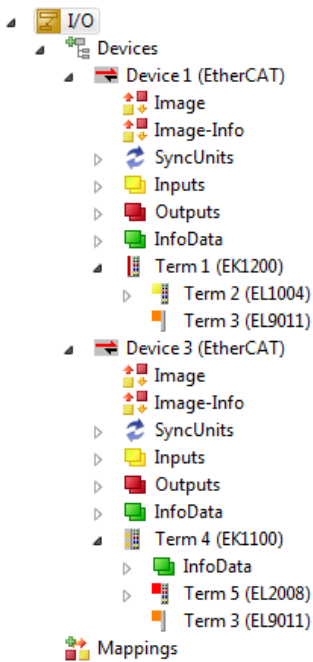
附图 58: 在TwinCAT3环境的VS shell中的配置映射
