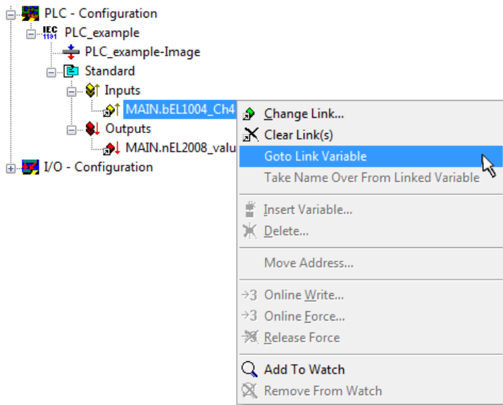
附图 48: 应用“转到链接变量”变量，以“MAIN.bEL1004_Ch4”为样本
