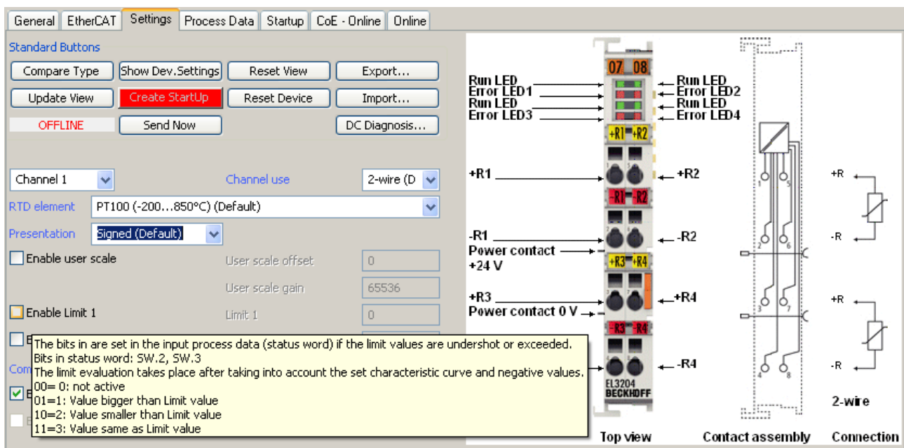
附图 134: EL3204 调试助手示例
