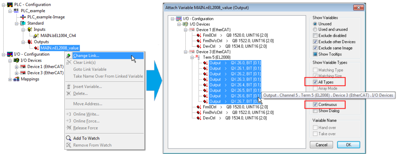
附图 47: 同时选择几个PDO: 激活“连续”和“所有类型”
