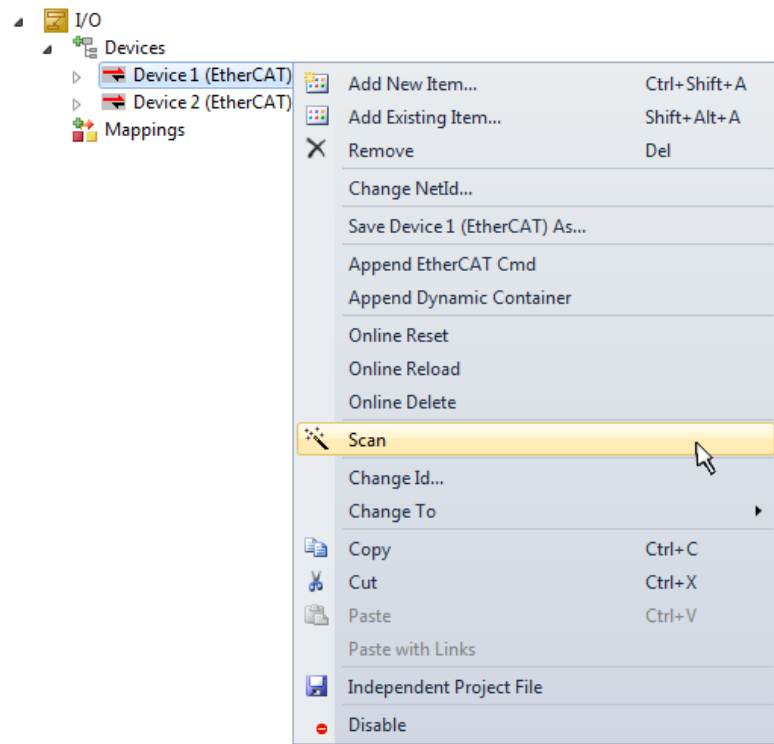
附图 59: 读取连接到设备的单个终端
