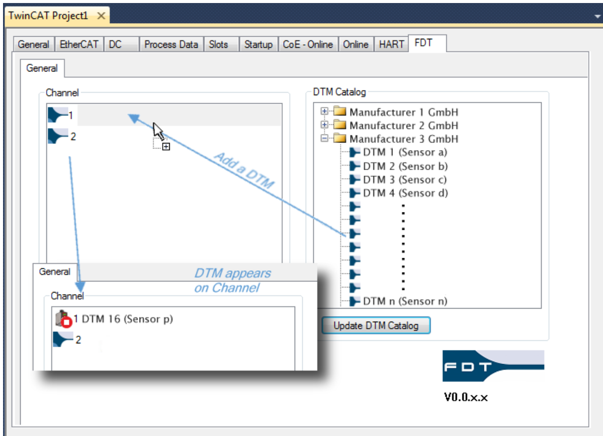
附图 157: 向端子模块/端子盒的相应通道添加传感器/执行器 DTM 设备驱动程序
