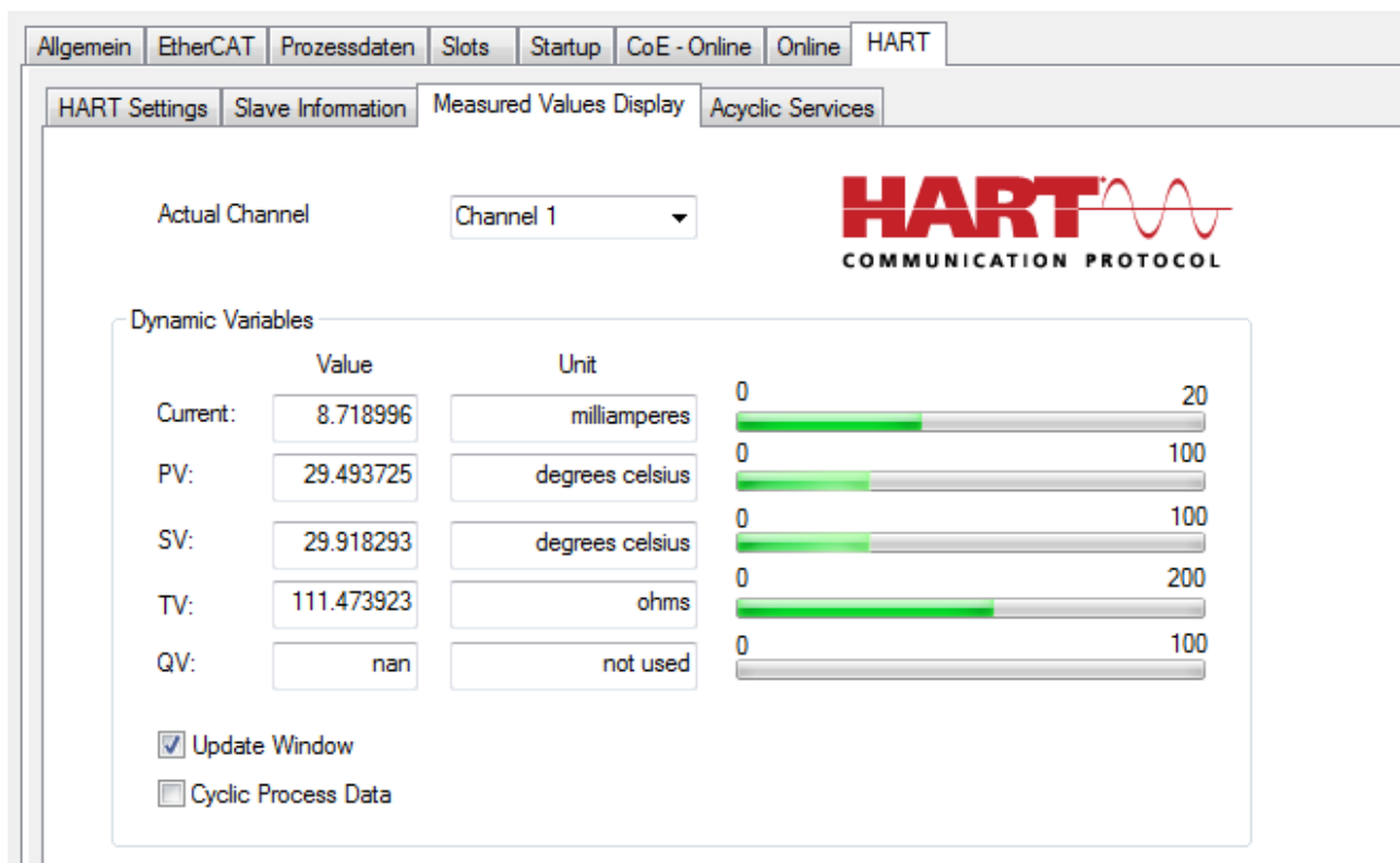
附图 154: 显示由 HART 读取的测量值
