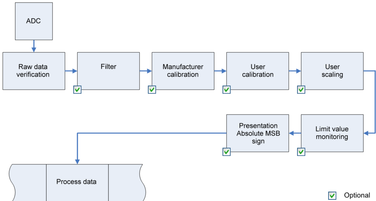
附图 151: ELX31xx/EPX31xx 的数据流
