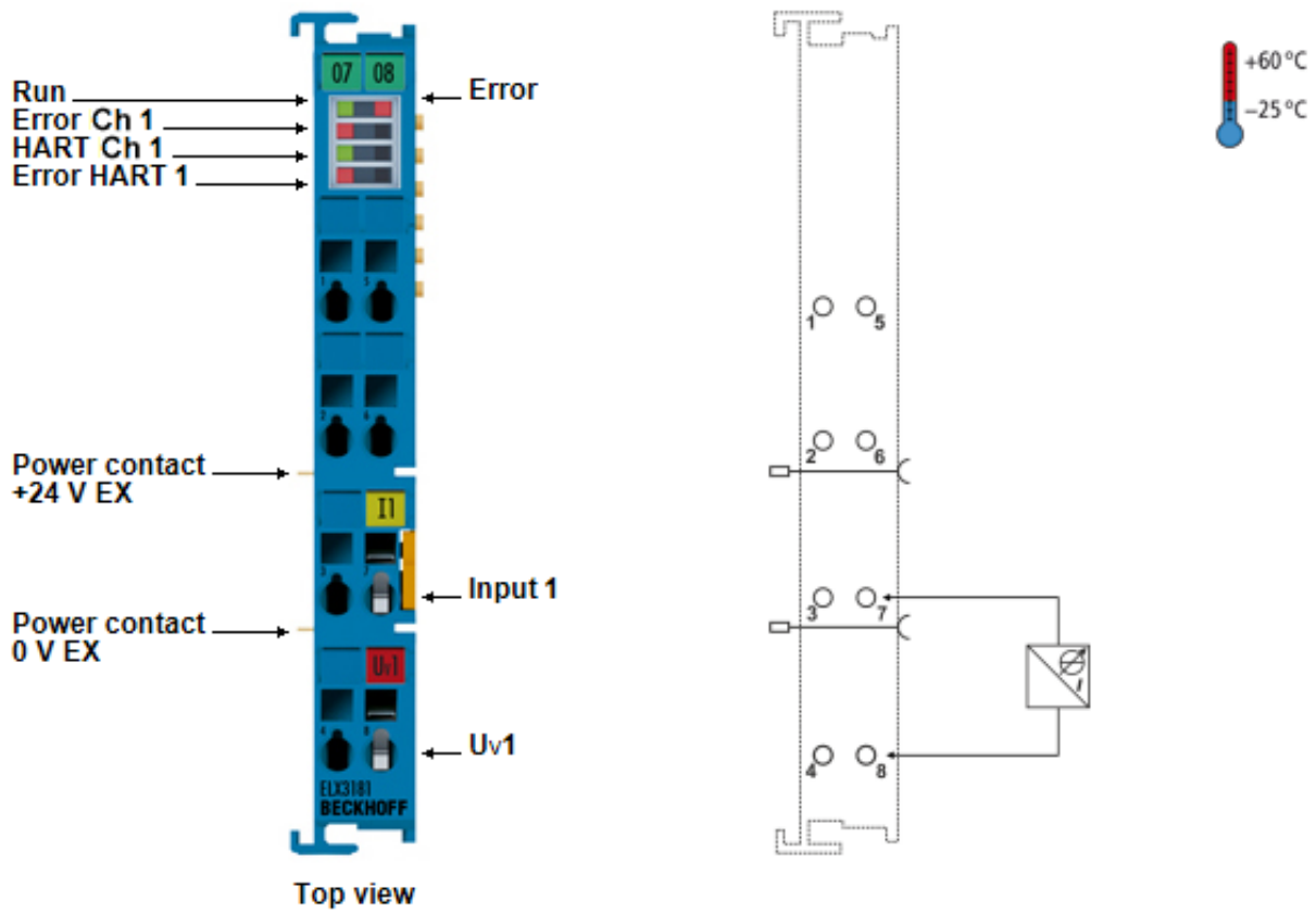
附图 21: ELX3181 - 触点分配
