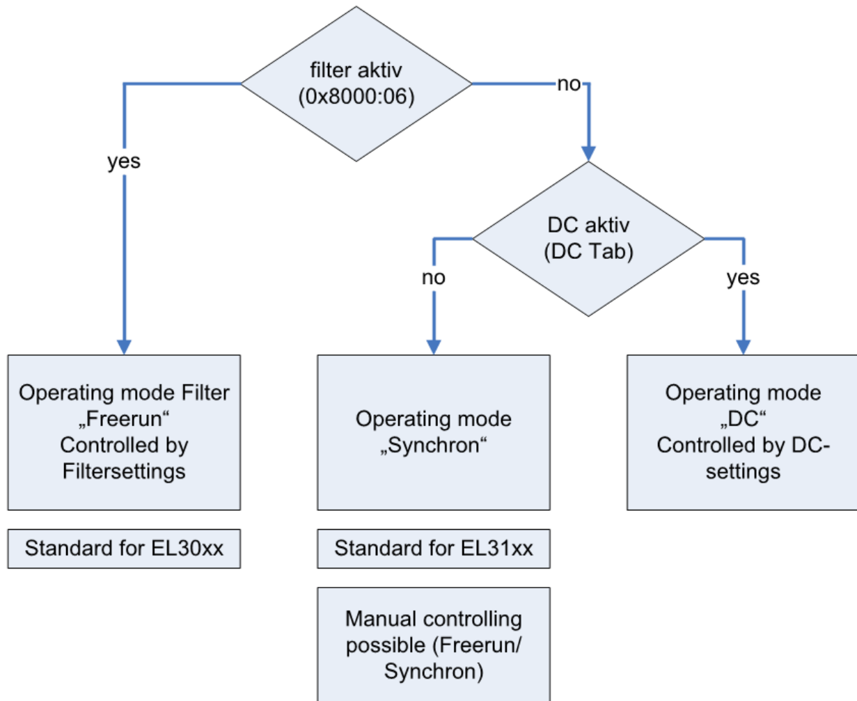
附图 143: 运行模式之间关系
