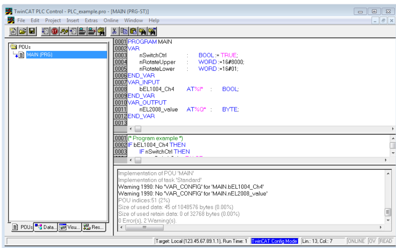
附图 42: 编译过程后带有变量的样本程序（无变量整合）
