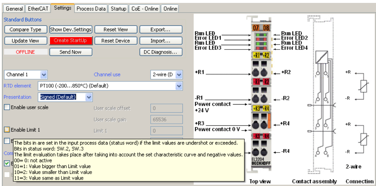
附图 130: EL3204 调试助手示例
