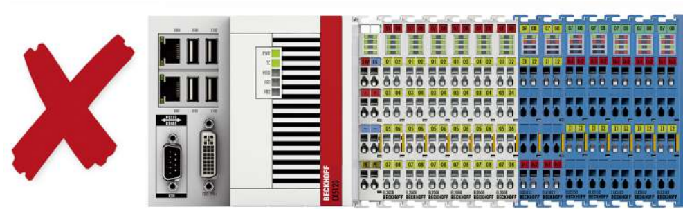
附图 12: 非法的安装 - 缺少 ELX9560 电源端子模块。
