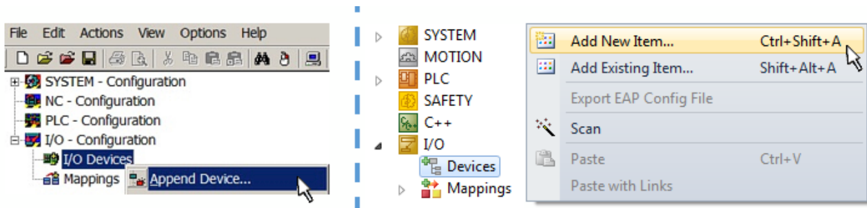
附图 86: 添加EtherCAT设备 (左: TwinCAT 2; 右: TwinCAT 3)
