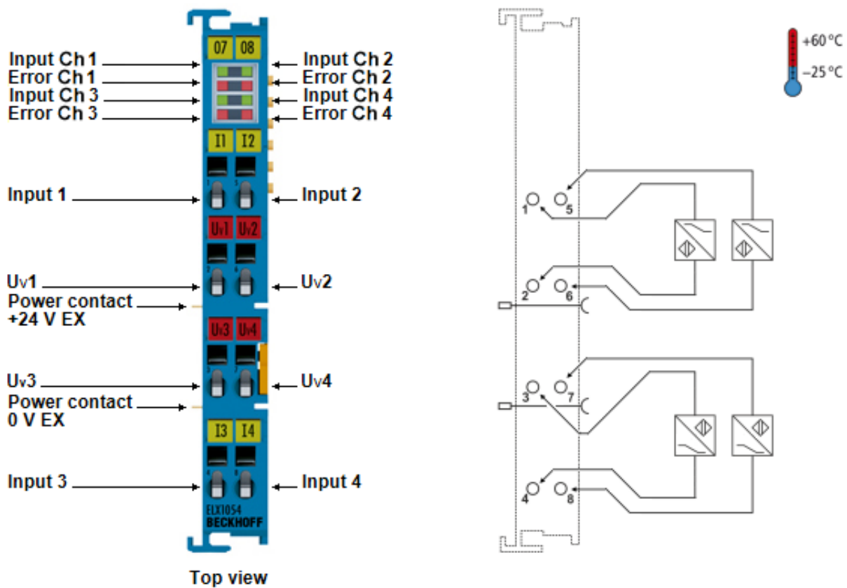
附图 23: ELX1054 - 触点分配
