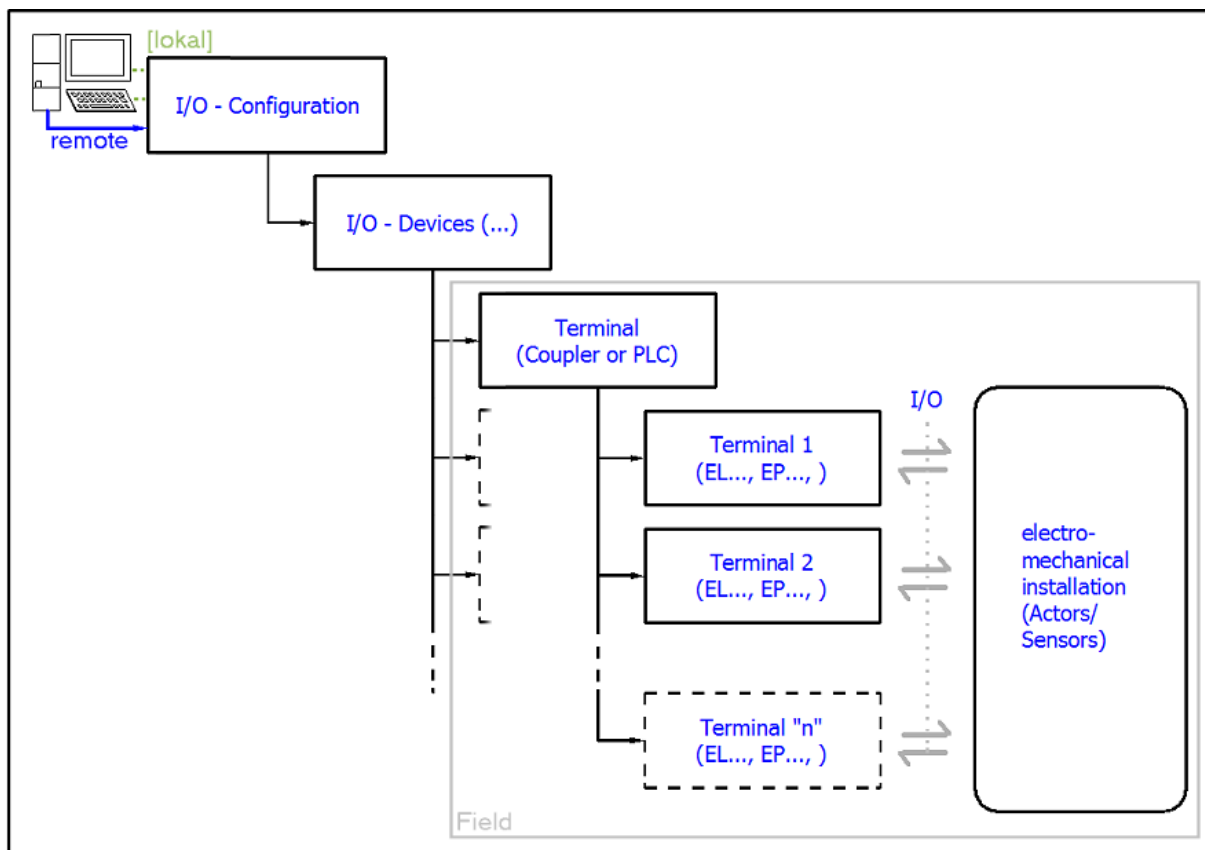
附图 28: 用户端（调试）和安装之间的关系
