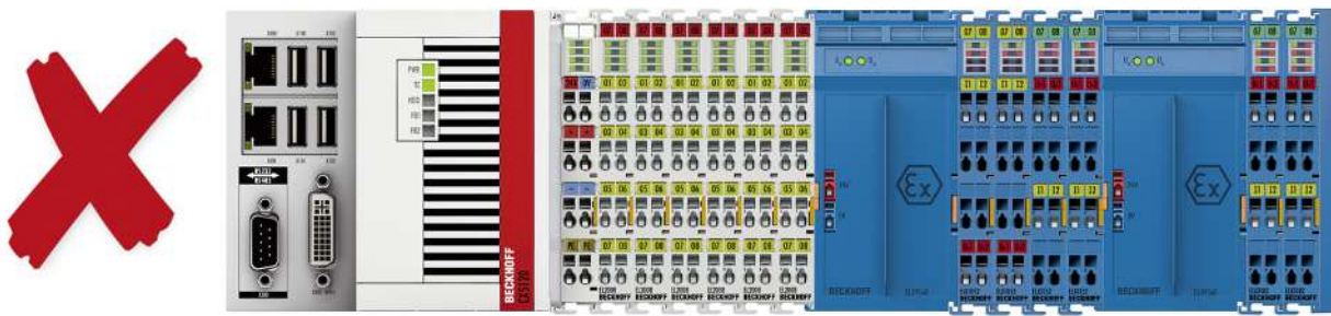
附图 14: 不允许的安装 - ELX 端子模块网段中的第二个 ELX9560 电源端子模块没有前端的 ELX9410。
