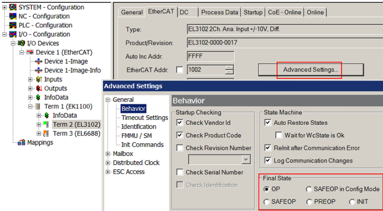
附图 132: 从站的默认目标状态
