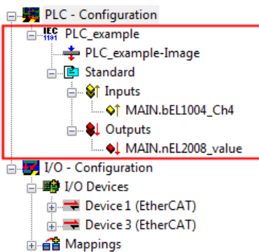
附图 40: 集成在系统管理器的PLC配置中的PLC项目
