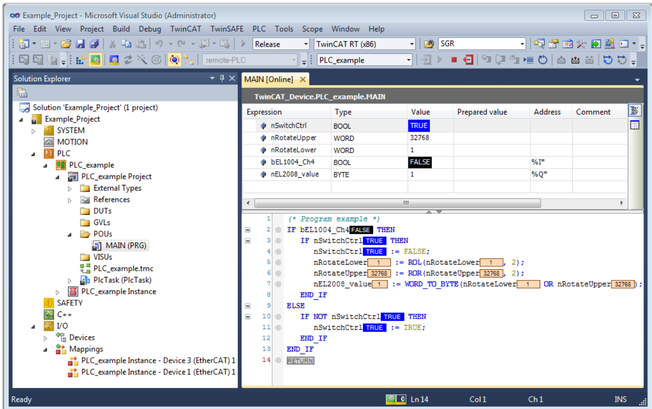
附图 69: TwinCAT开发环境（VS shell）：程序启动后登录
