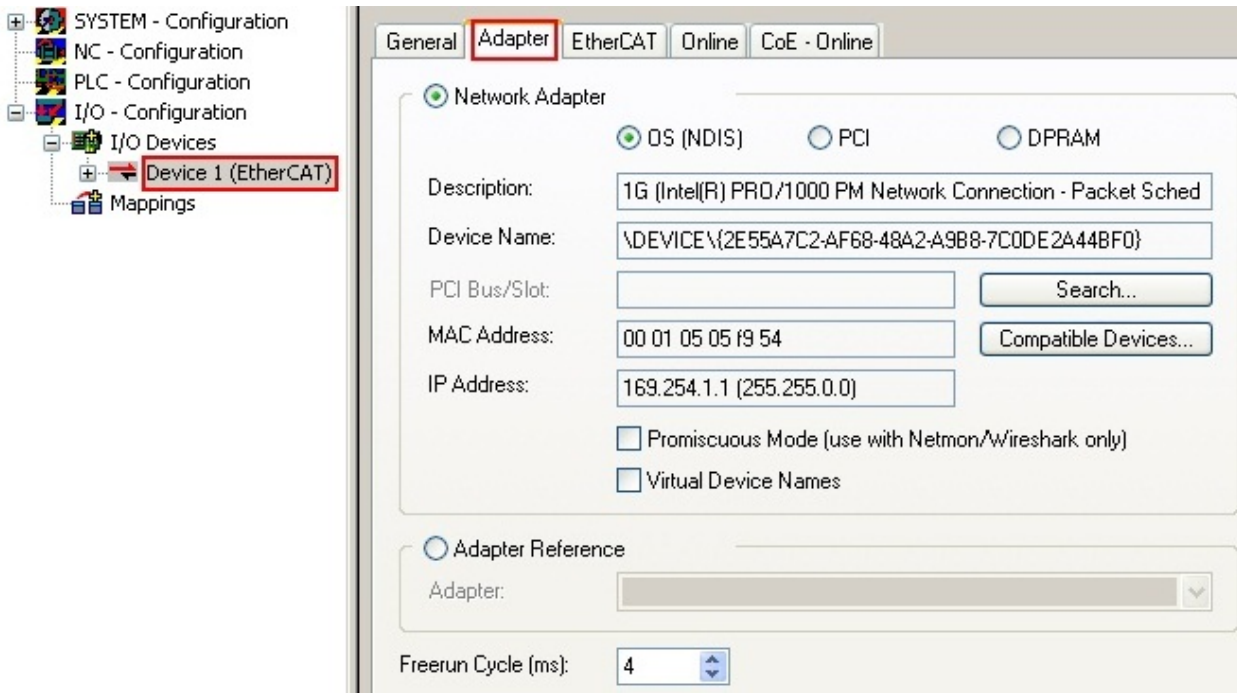
附图 89: EtherCAT设备属性 (TwinCAT 2)
