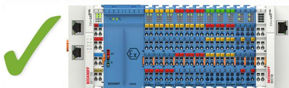
附图 9: 允许的安装 - 不属于 ELX 系列的端子模块被放置在 ELX 端子模块网段的前后。由 ELX 端子模块网段开头的 ELX9560 和 ELX 端子模块网段末端的 EK1110 隔离。
