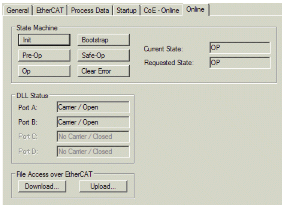
附图 125: “Online (在线)” 选项卡
