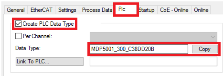
附图 65: 创建一个PLC数据类型
