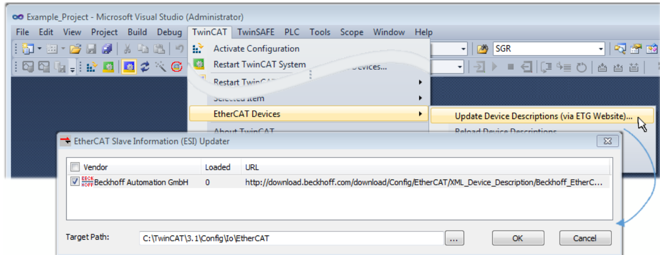
附图 85: 使用ESI Updater (TwinCAT 3)
