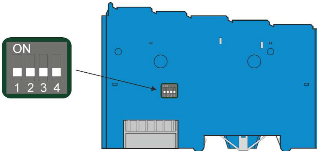
附图 24: ELX1054 - DIP 开关
