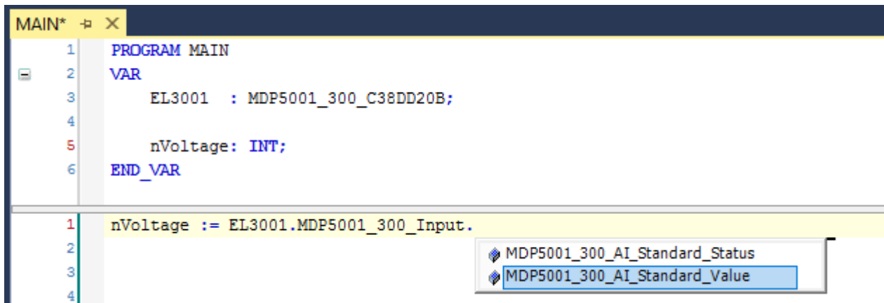
附图 68: 从过程数据的结构中读取一个变量
