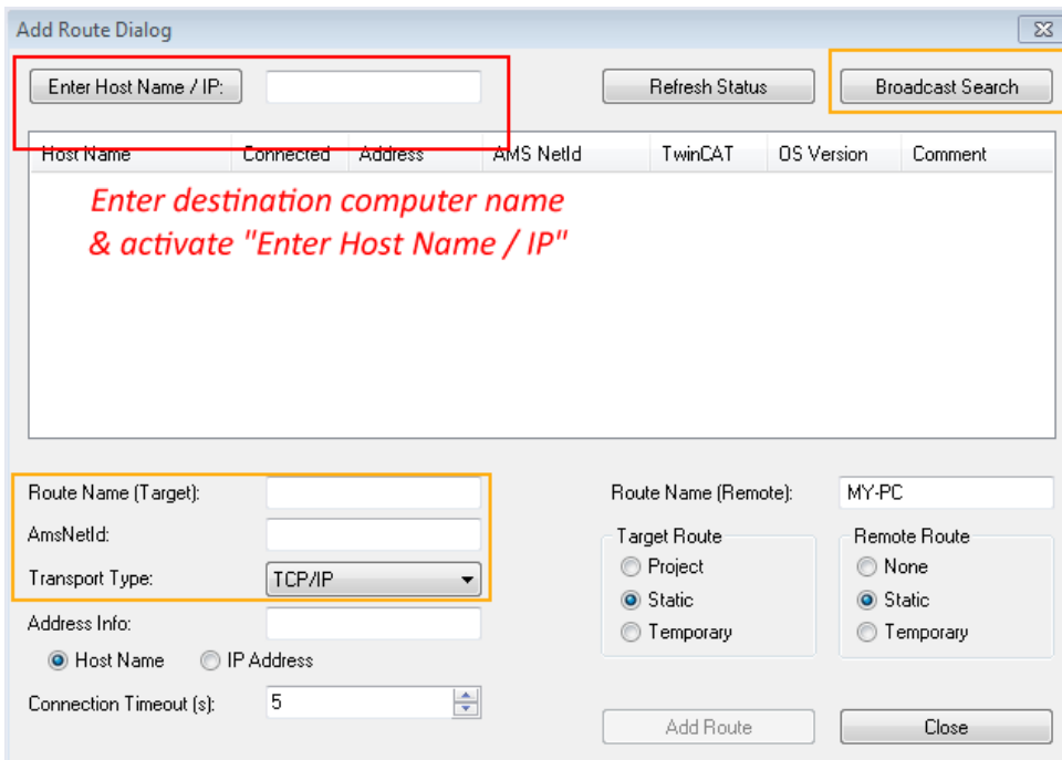
附图 51: 为TwinCAT系统管理器指定访问的PLC：选择目标系统
