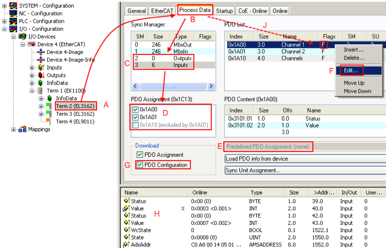
附图 121: 配置过程数据
