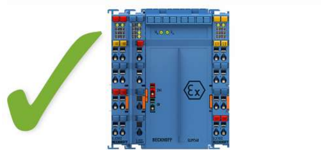
附图 11: 允许的安装 - ELX9410 在 ELX9560 电源端子模块前。
