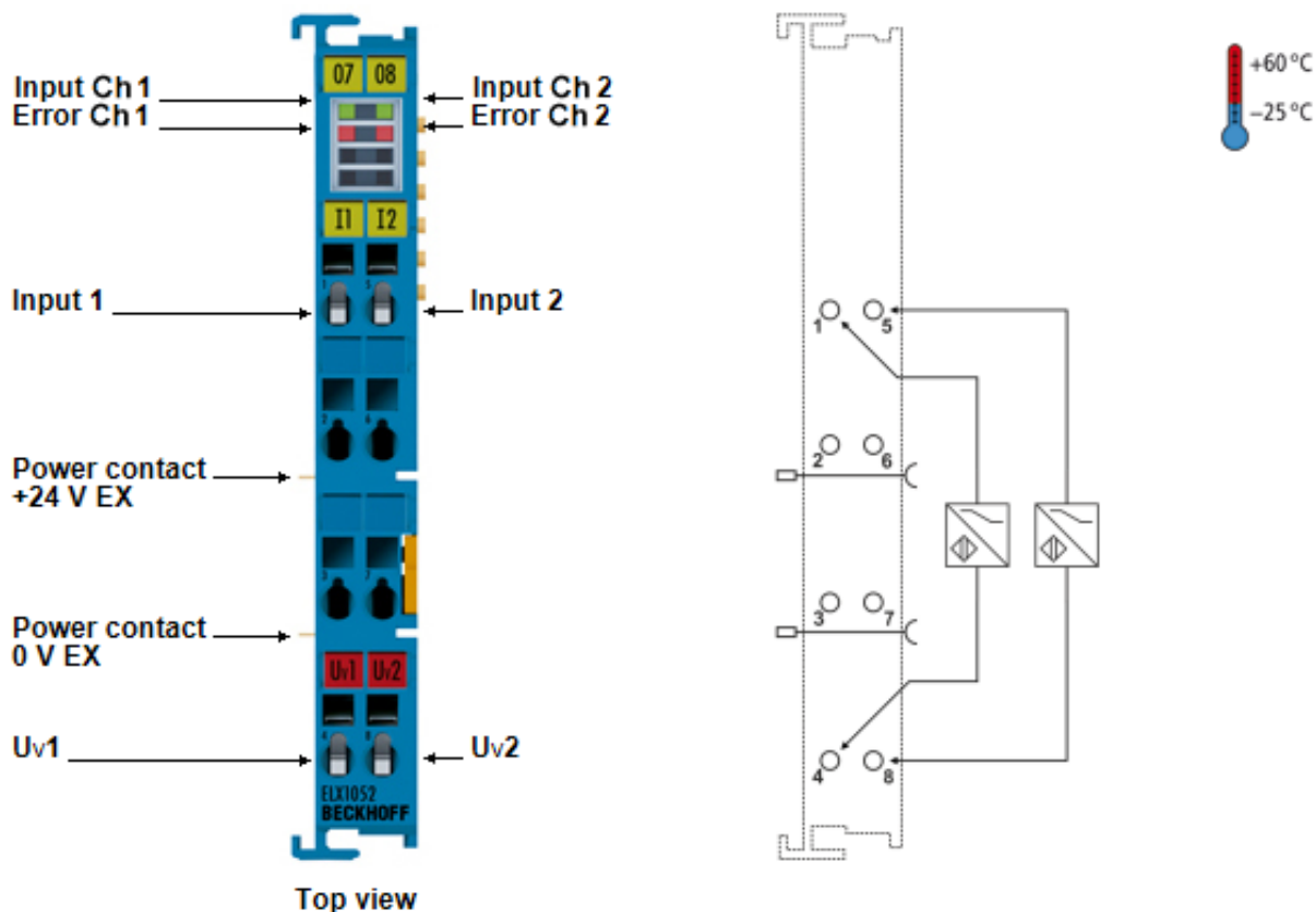
附图 22: ELX1052 - 触点分配
