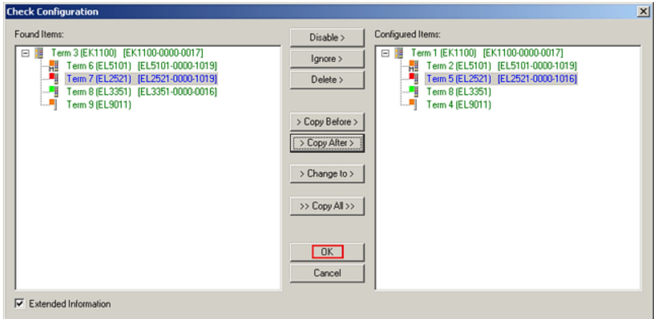
附图 114: 有修改的校正对话框
