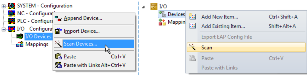
附图 97: 扫描设备（左：TwinCAT 2；右：TwinCAT 3）
