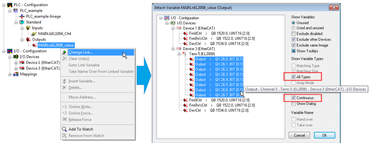
附图 43: 同时选择几个PDO: 激活“连续”和“所有类型”
