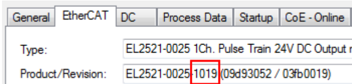
附图 102: 检测修订版本-1019 的 EtherCAT 端子
