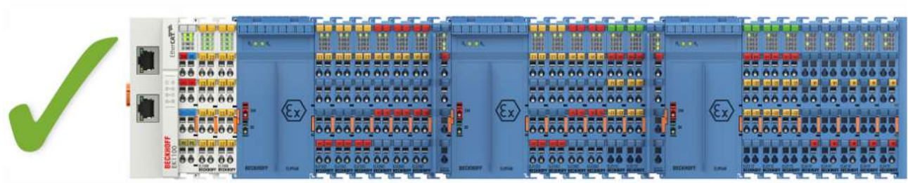
附图 10: 允许的安装 - 由 ELX9560 提供多个再次供电电源，在每种情况下都有一个前端的 ELX9410。
