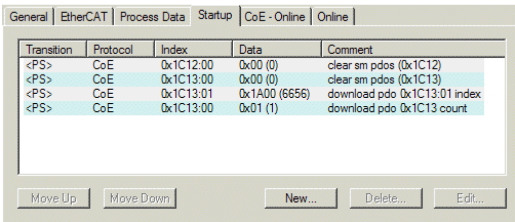
附图 122: “Startup (启动)” 选项卡
