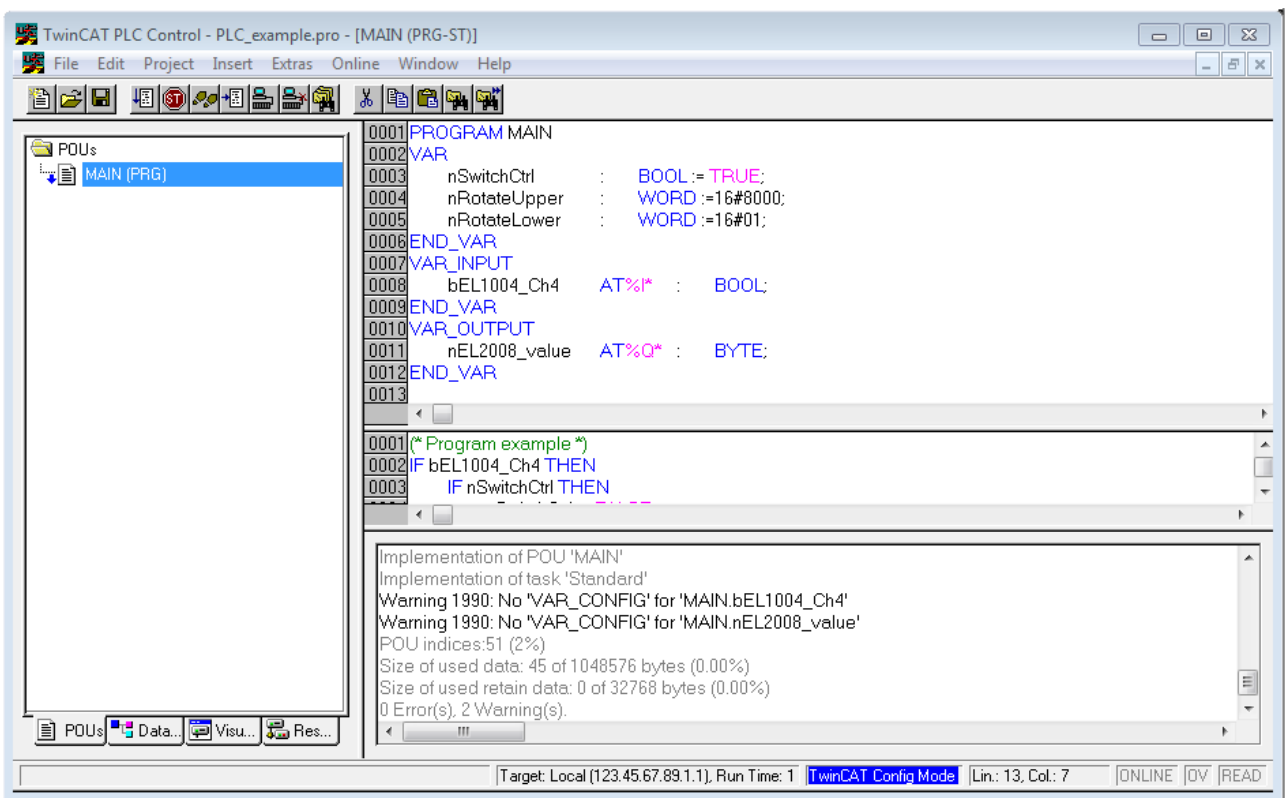
附图 38: 编译过程后带有变量的样本程序（无变量整合）
