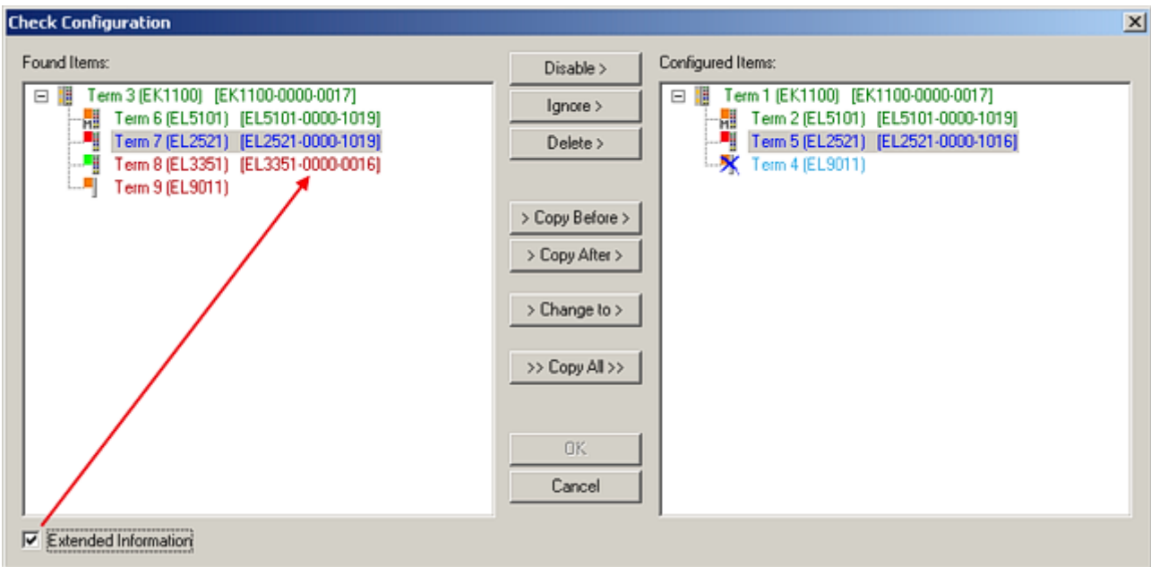
附图 112: 校正对话框
