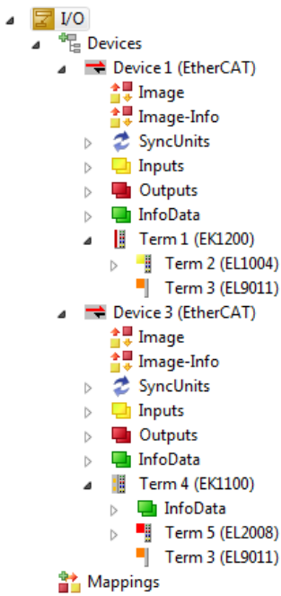
附图 54: 在TwinCAT3环境的VS shell中的配置映射
