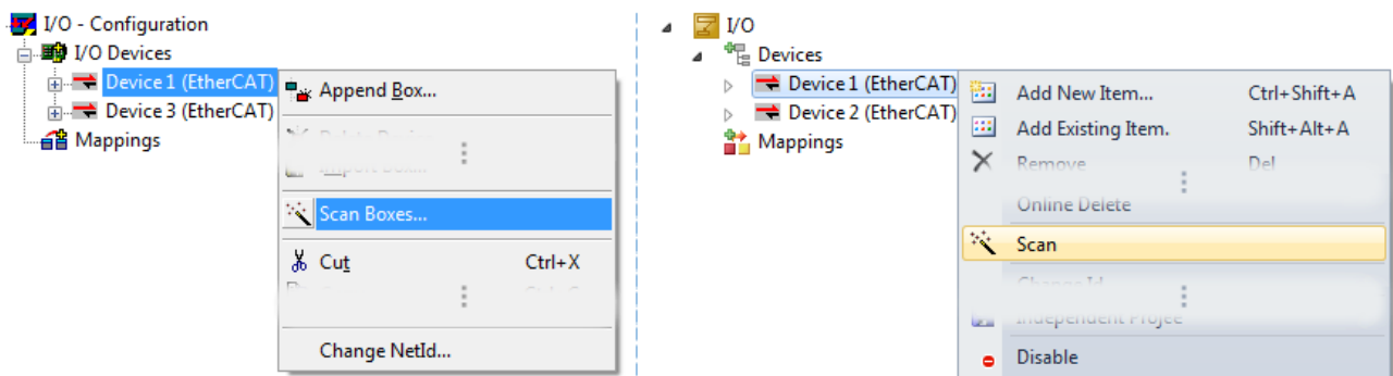
附图 104: 在一个指定的 EtherCAT 设备上手动触发设备扫描（左：TwinCAT 2；右：TwinCAT 3）
