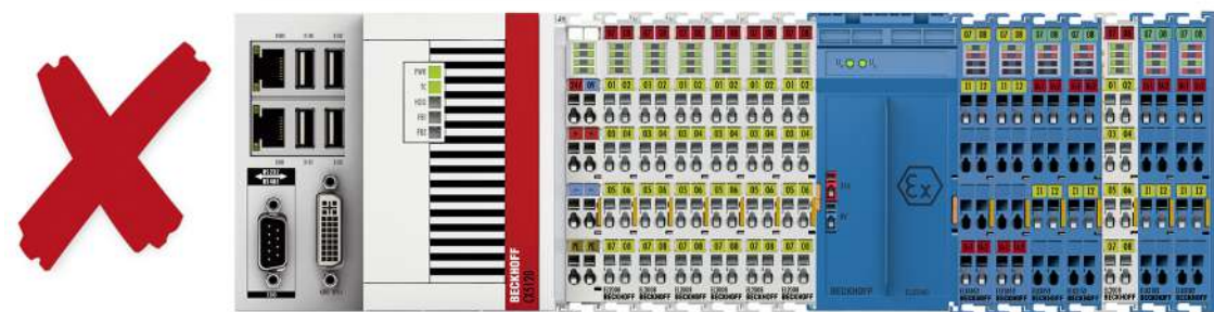
附图 13: 不允许的安装 - ELX 端子模块网段中的端子模块不属于 ELX 系列
