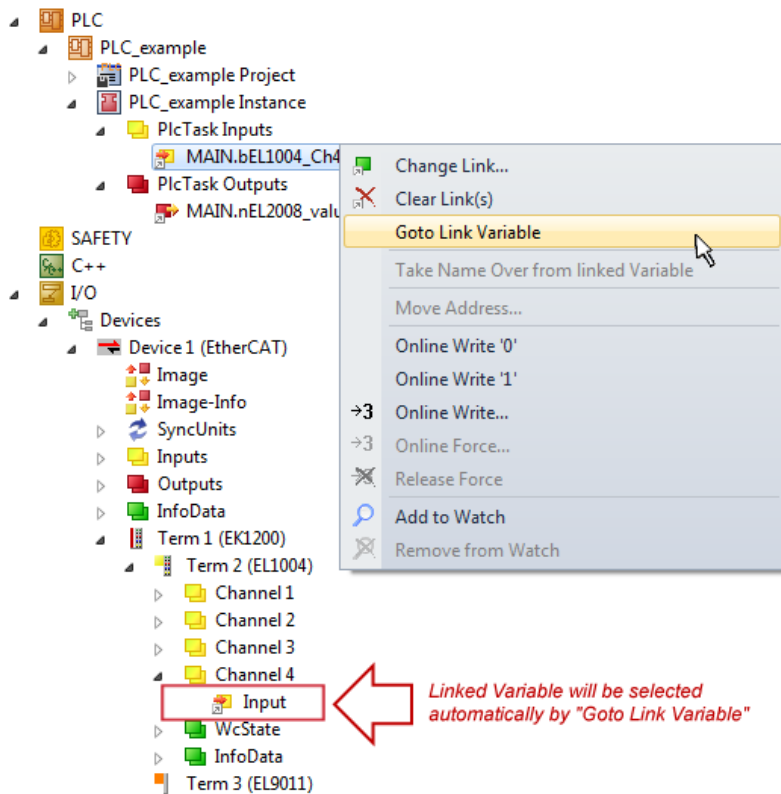
附图 64: 应用“转到链接变量”变量，以“MAIN.bEL1004_Ch4”为样本
