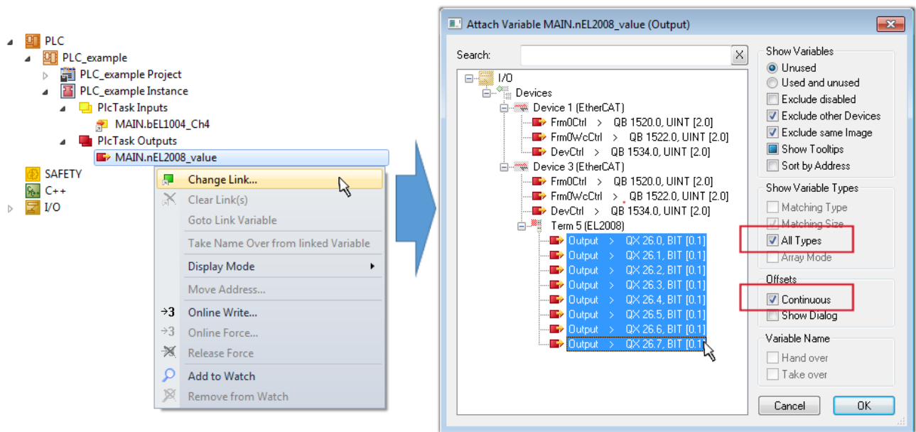
附图 63: 同时选择几个PDO: 激活“连续”和“所有类型”
