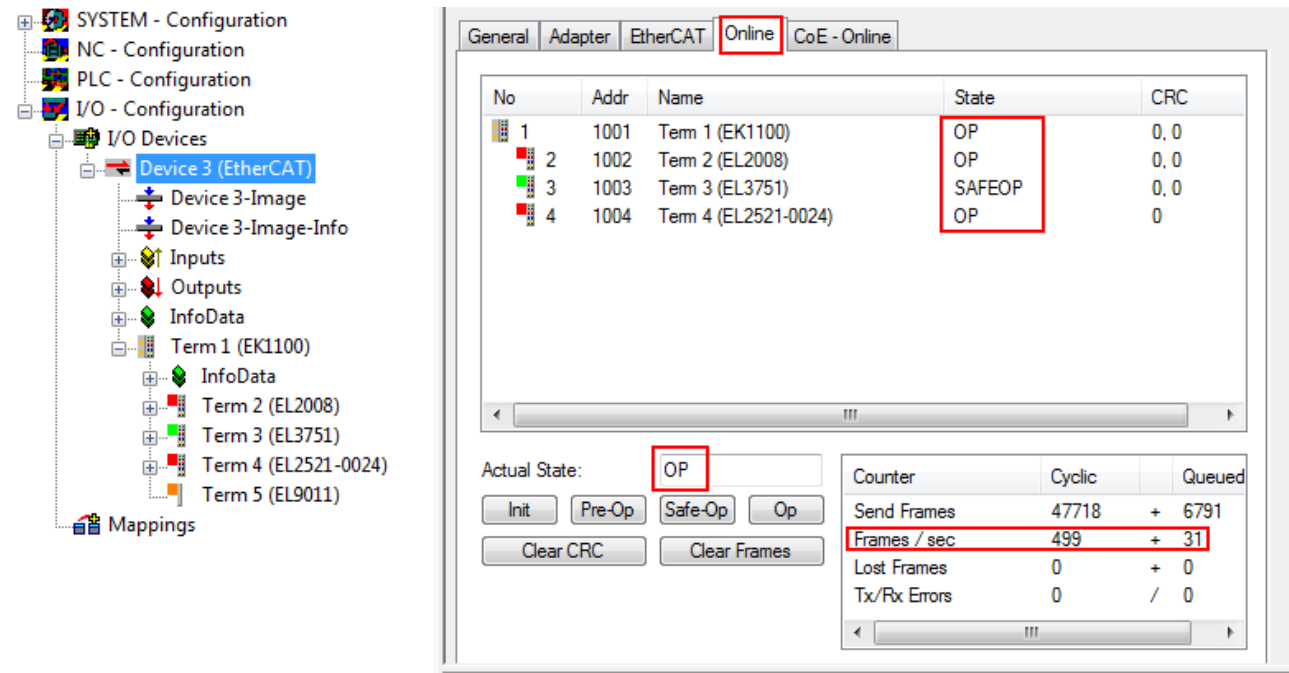
附图 109: 在线显示示例
