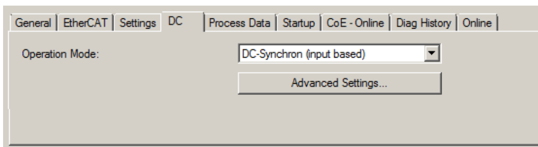
附图 126: “DC” 选项卡 (分布时钟)
