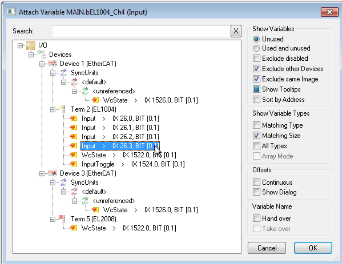
附图 62: 选择BOOL类型的PDO
