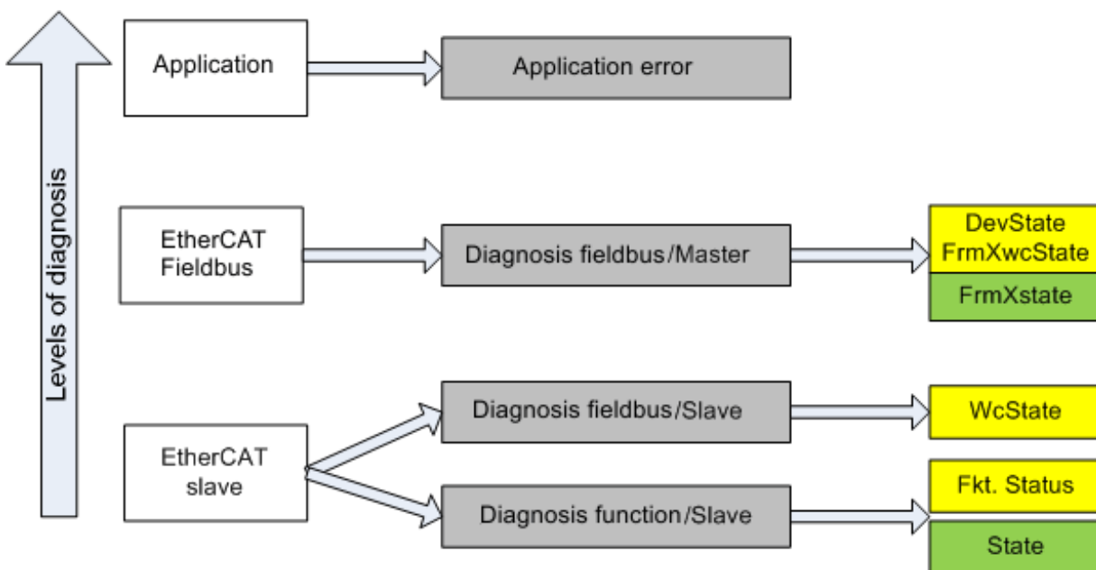
附图 127: 选择 EtherCAT 从站的诊断信息
