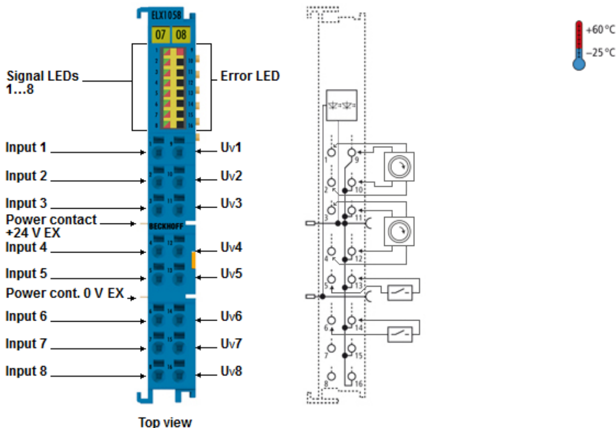
附图 27: ELX1058 - 连接增量编码器
