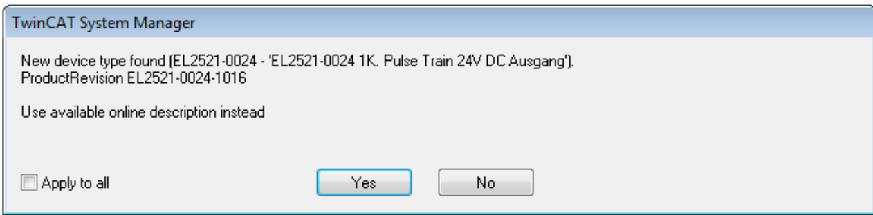
附图 79: 在线描述信息窗口 (TwinCAT 2)
