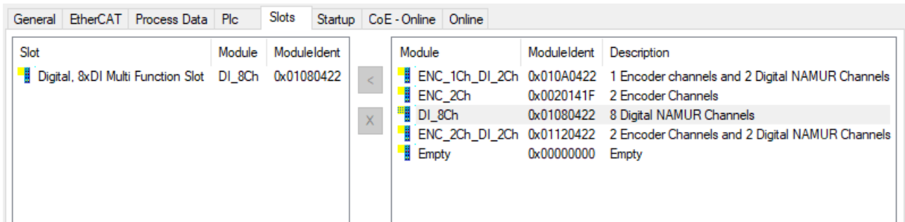
附图 25: ELX1058 - 插槽 选项卡
