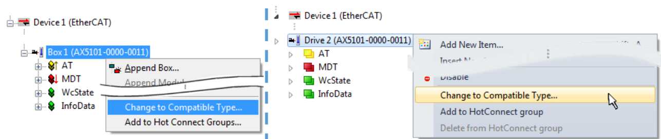
附图 115: 对话框“更改为兼容类型...” (左: TwinCAT 2; 右: TwinCAT 3)
