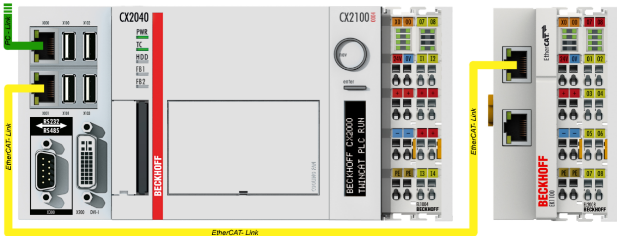
附图 29: 控制配置，带嵌入式电脑、输入（EL1004）和输出（EL2008）
