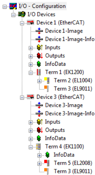
附图 35: TwinCAT 2系统管理器中的配置映射
