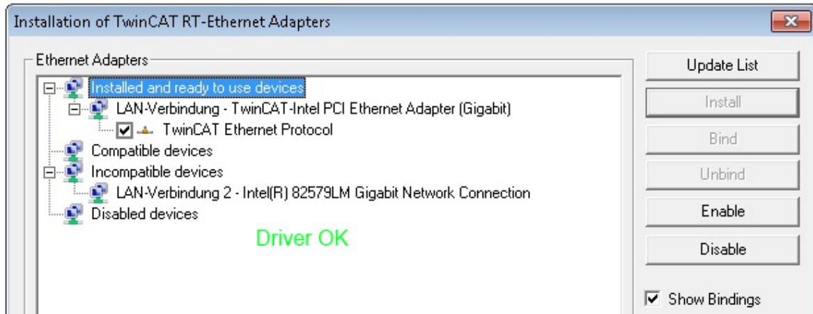
附图 75: 以太网端口的示范性正确驱动程序设置
