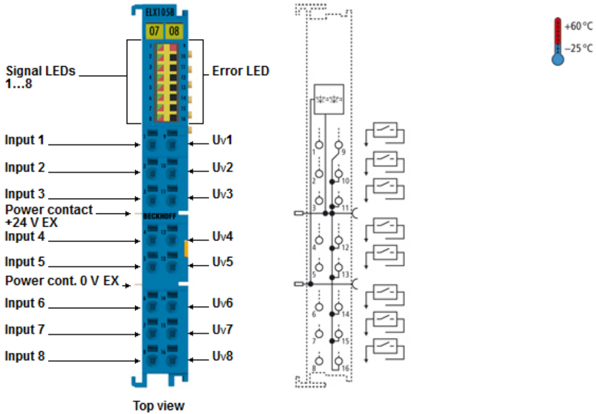
附图 26: ELX1058 - 连接数字量输入
