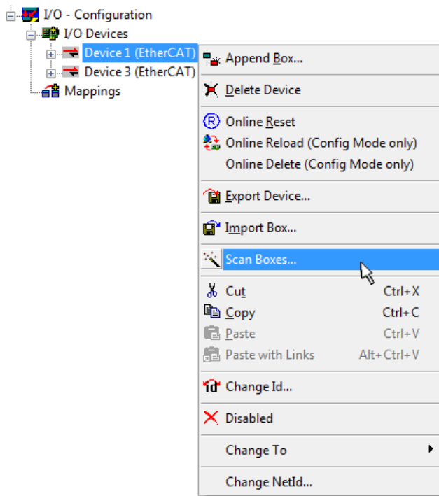
附图 36: 读取连接到设备的单个终端
