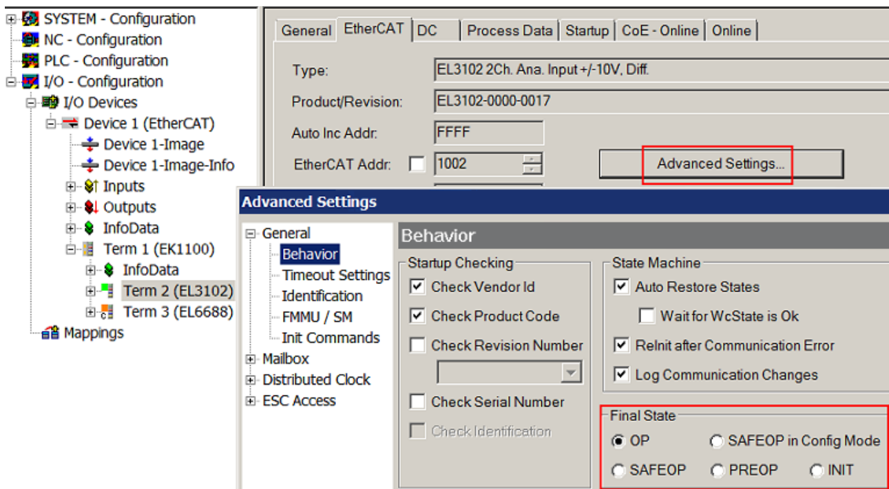
Abb. 157: Default Zielzustand im Slave
