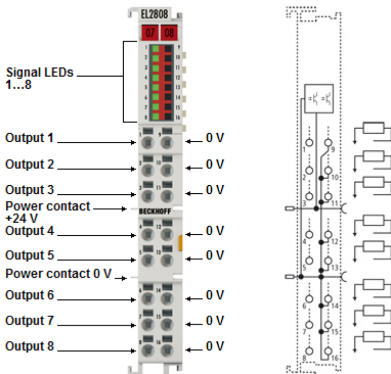
Abb. 7: EL2808
