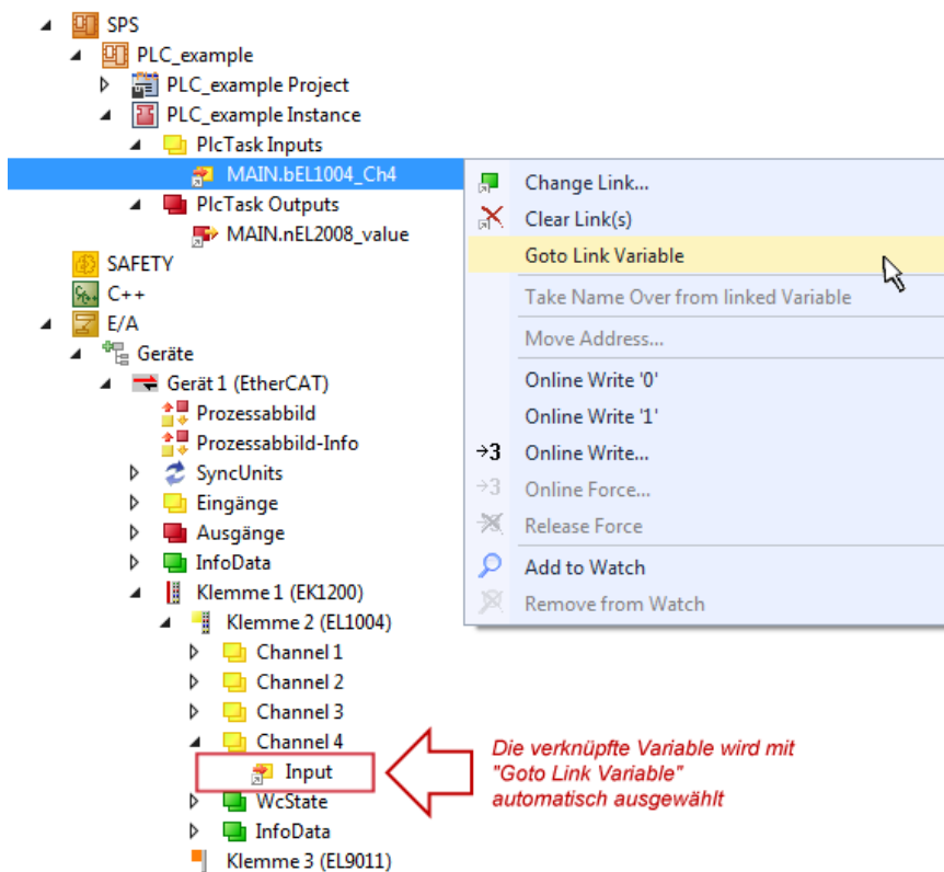
Abb. 87: Anwendung von "Goto Link Variable" am Beispiel von „MAIN.bEL1004_Ch4“
