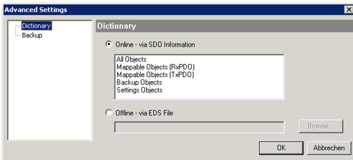
Abb. 149: Dialog „Advanced settings“
