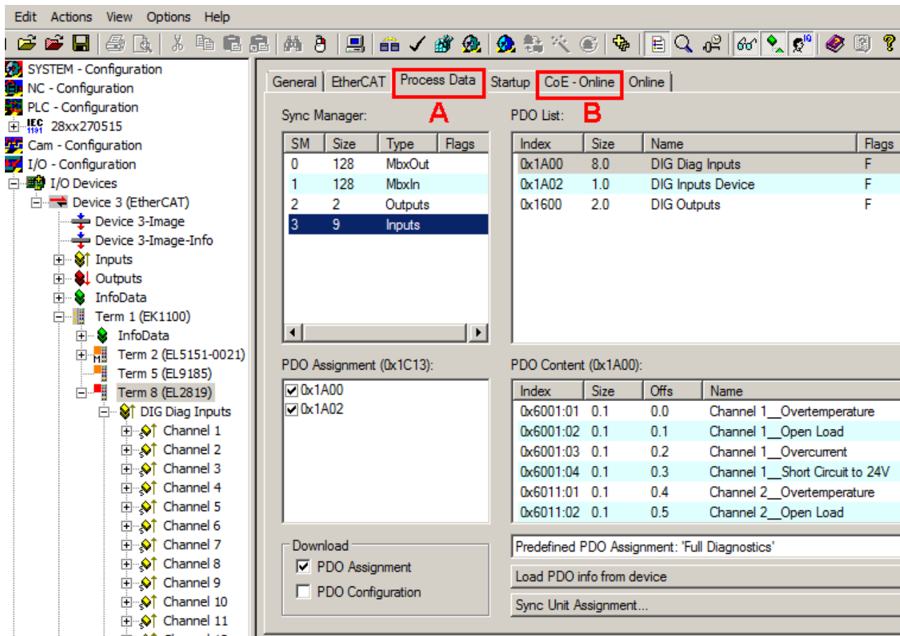
Abb. 18: EL2819 Reiter "Prozessdaten"
