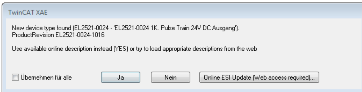
Abb. 104: Hinweisfenster OnlineDescription (TwinCAT 3)
