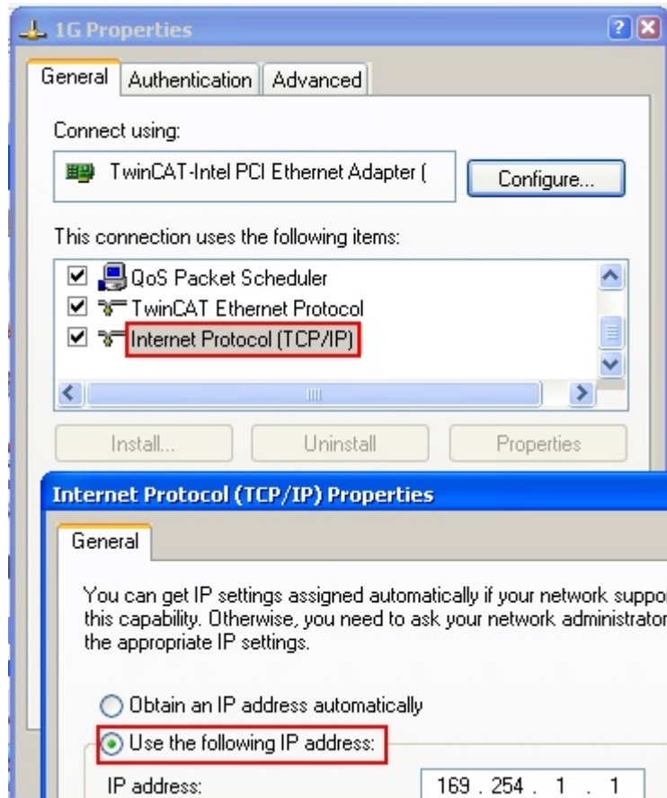
Abb. 101: TCP/IP-Einstellung des Ethernet Ports
