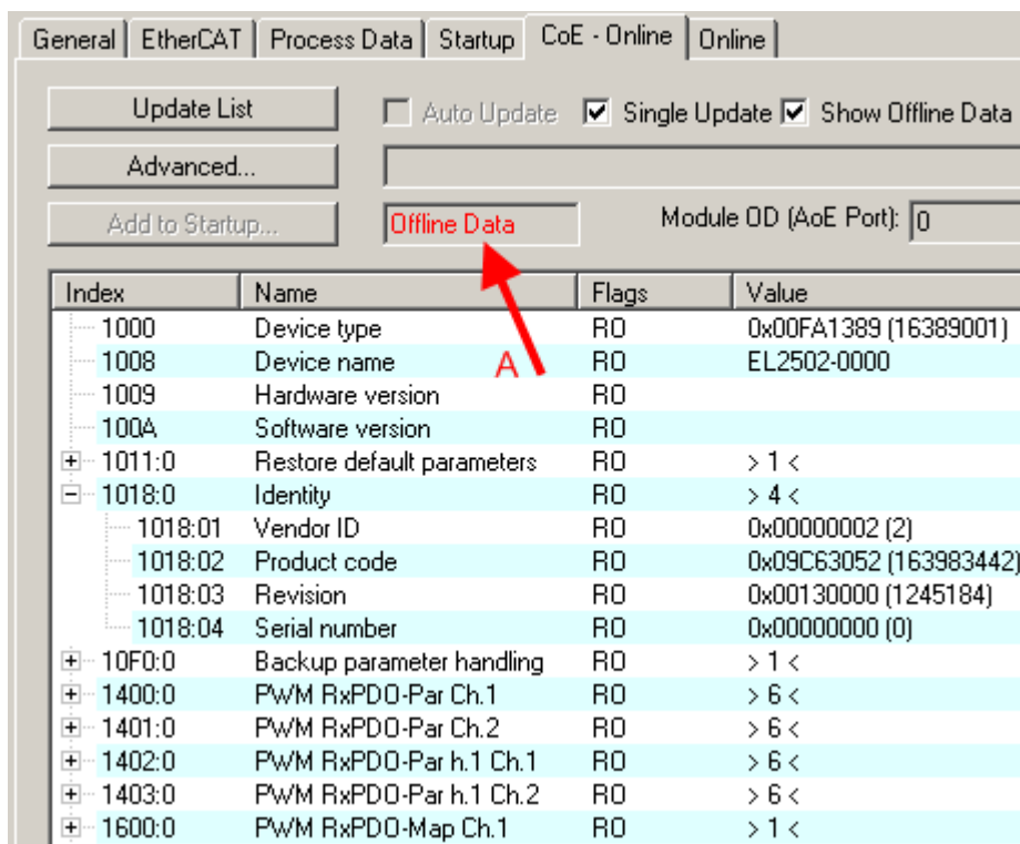
Abb. 34: Offline-Verzeichnis
