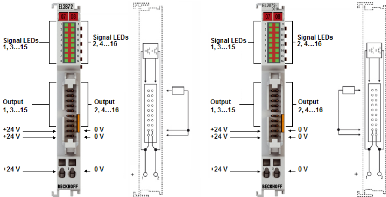
Abb. 25: EL2872, EL2872-0010
