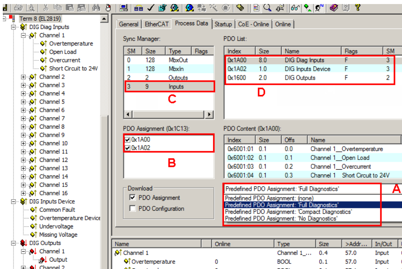
Abb. 20: EL2819 Reiter "Prozessdaten"
