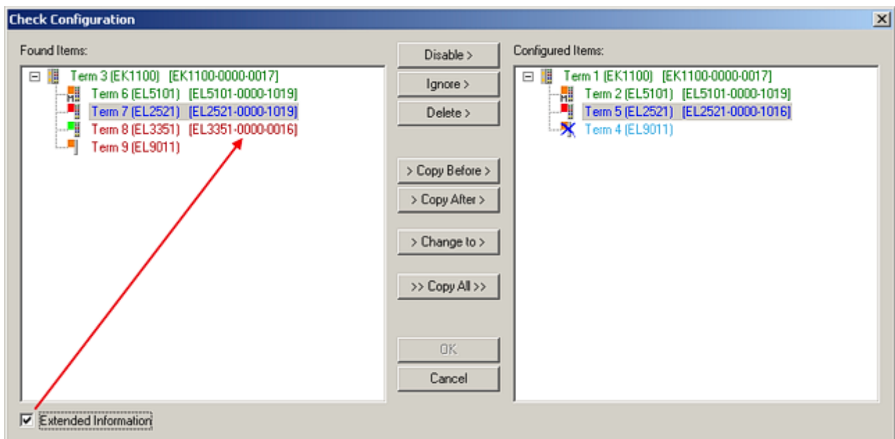
Abb. 137: Korrekturdialog
