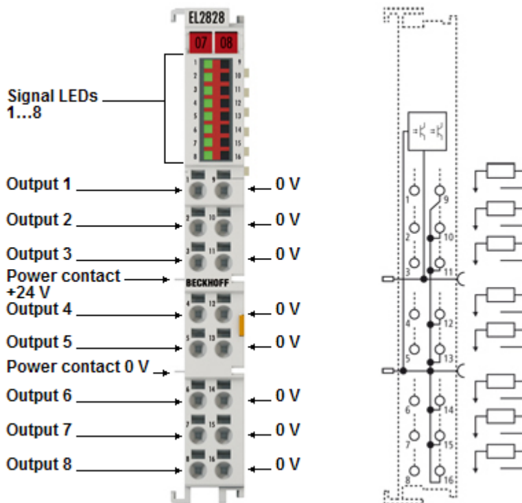
Abb. 9: EL2828
