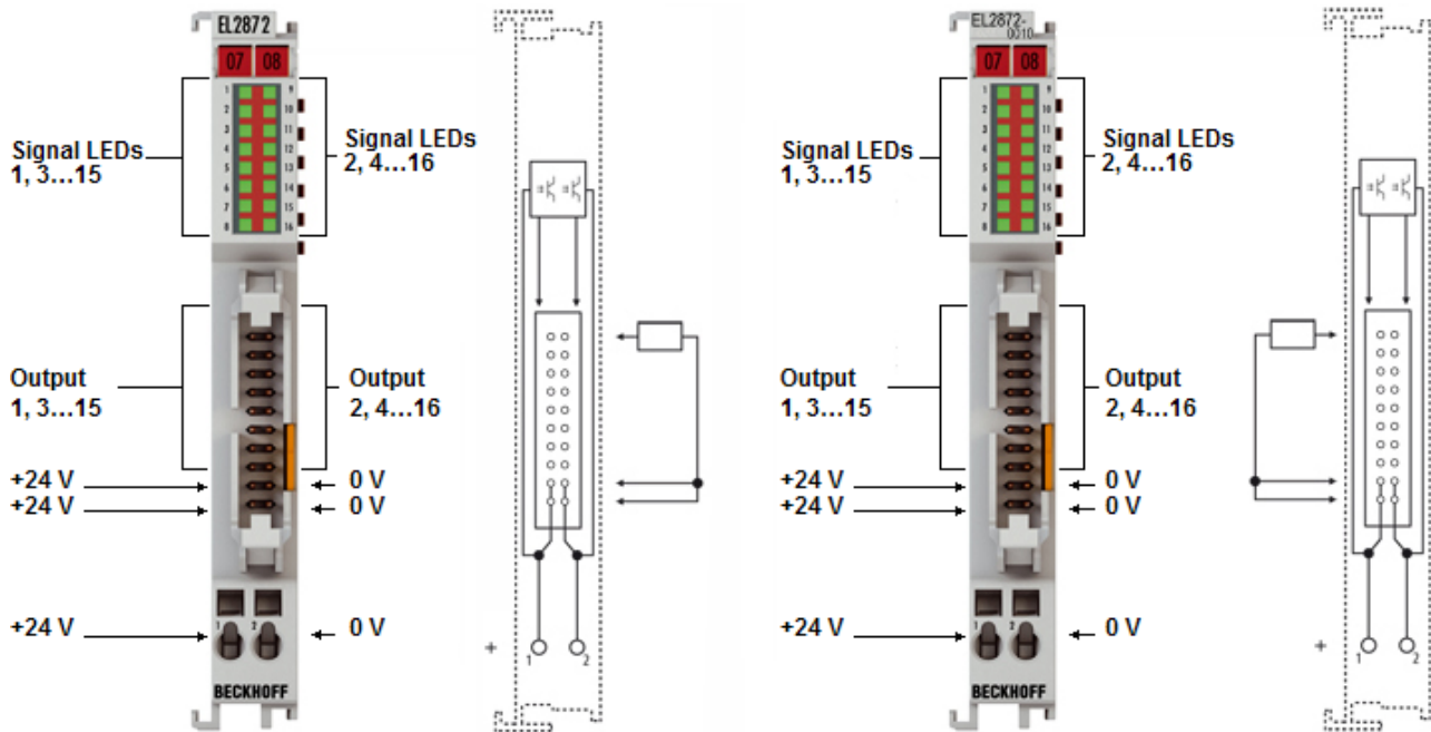
Abb. 24: EL2872, EL2872-0010
