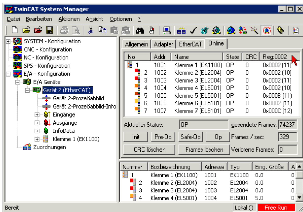
Abb. 169: Versionsbestimmung FPGA-Firmware
