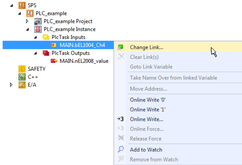
Abb. 84: Erstellen der Verknüpfungen PLC-Variablen zu Prozessobjekten
