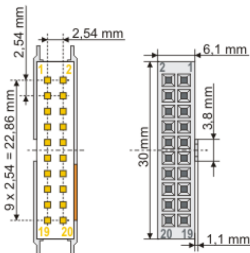
Abb. 26: Abmessungen der 20-poligen Stiftleiste der Klemme und der passenden Federleiste, Beschaltung siehe Konaktbelegung
