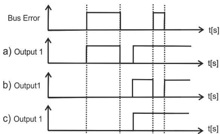
Abb. 23: graphische Darstellung des Kanalzustands bei Busstörung
