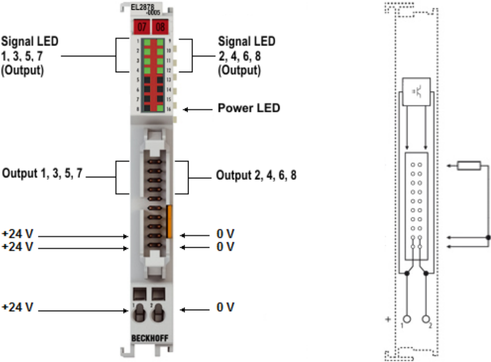
Abb. 28: EL2878-0005
