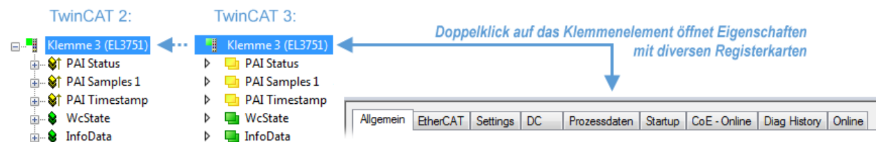
Abb. 142: „Baumzweig“ Element als Klemme EL3751
