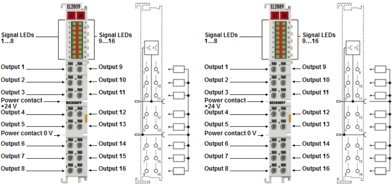
Abb. 12: EL2809, EL2889
