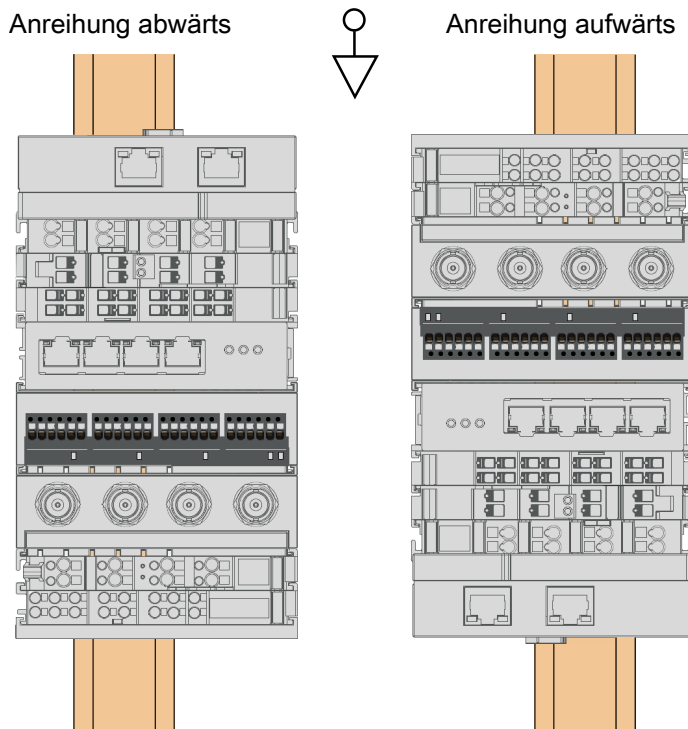
Abb. 46: Einbaulage Senkrecht, Anreihung abwärts (links) / Anreihung aufwärts (rechts)
