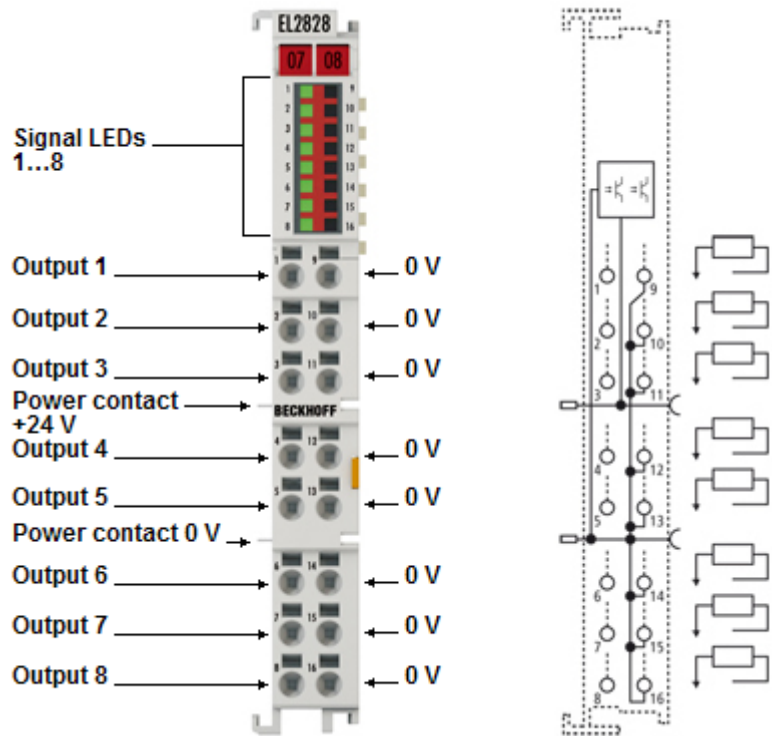
Abb. 10: EL2828
