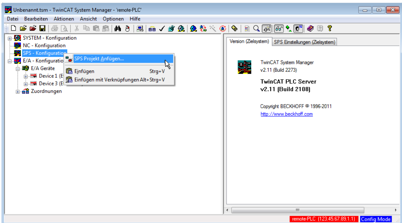
Abb. 62: Hinzufügen des Projektes des TwinCAT PLC Control
