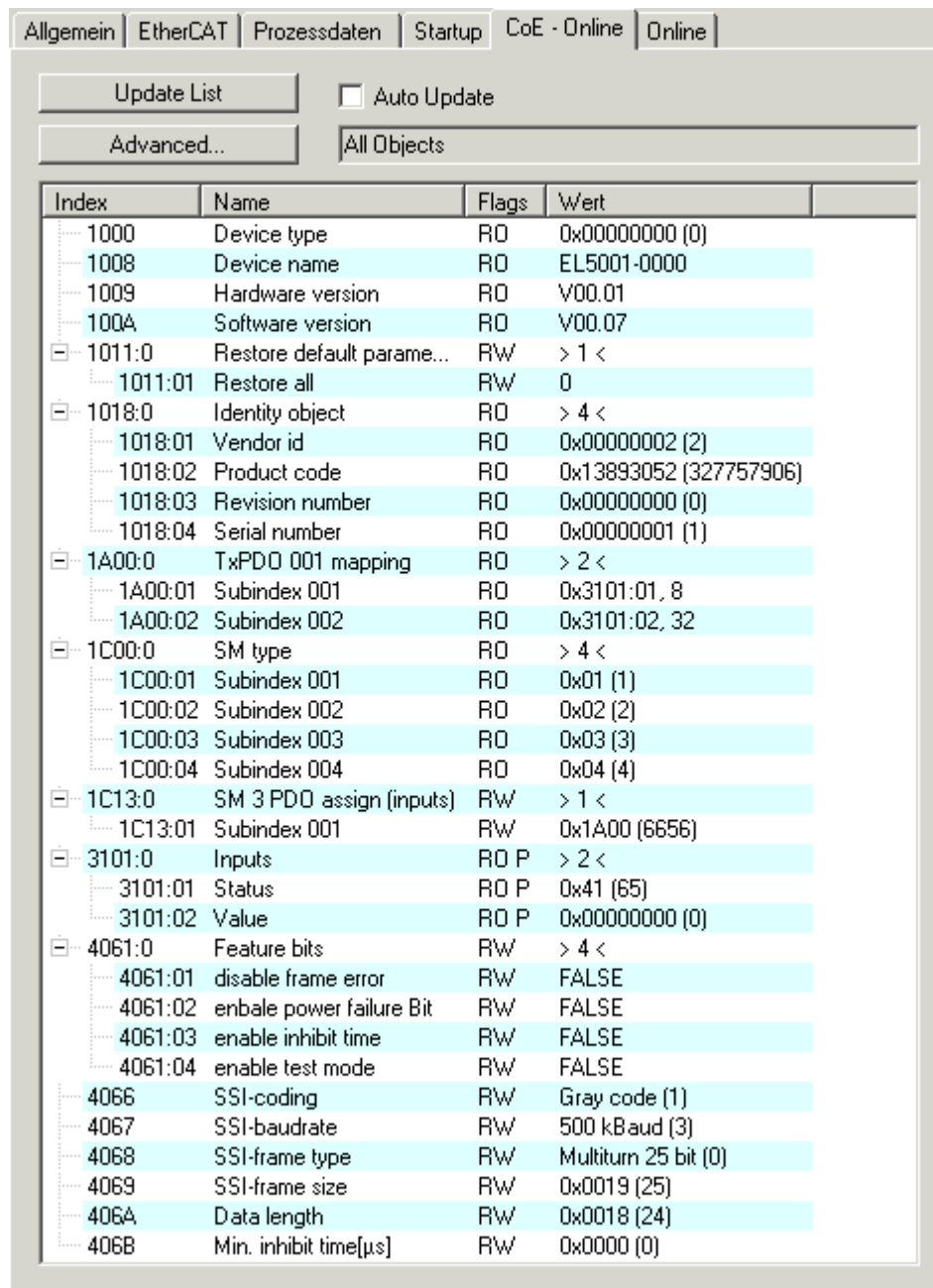
Abb. 148: Karteireiter „CoE - Online“
