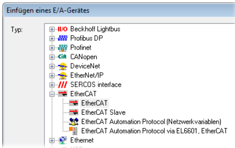
Abb. 112: Auswahl EtherCAT Anschluss (TwinCAT 2.11, TwinCAT 3)
