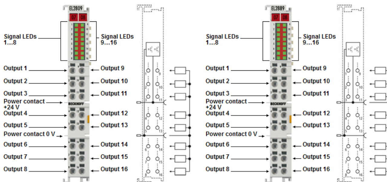
Abb. 11: EL2809, EL2889
