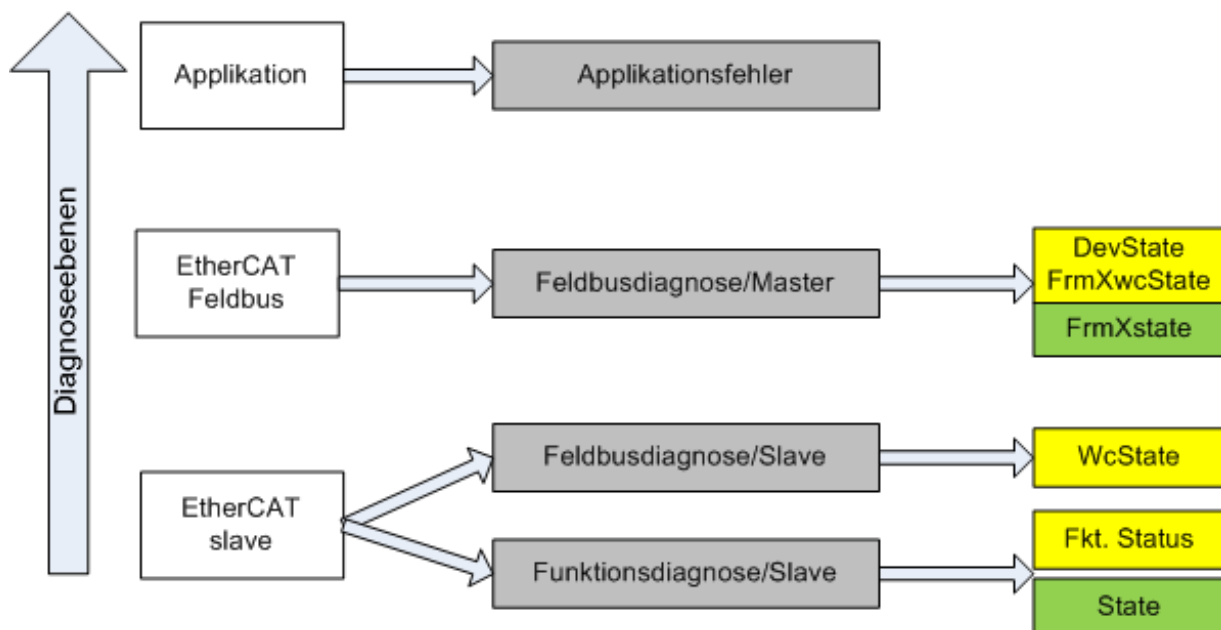
Abb. 152: Auswahl an Diagnoseinformationen eines EtherCAT-Slaves
