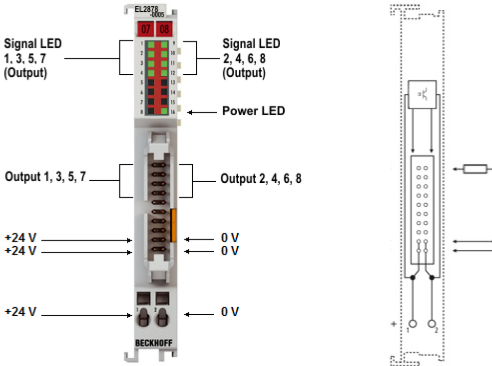
Abb. 27: EL2878-0005
