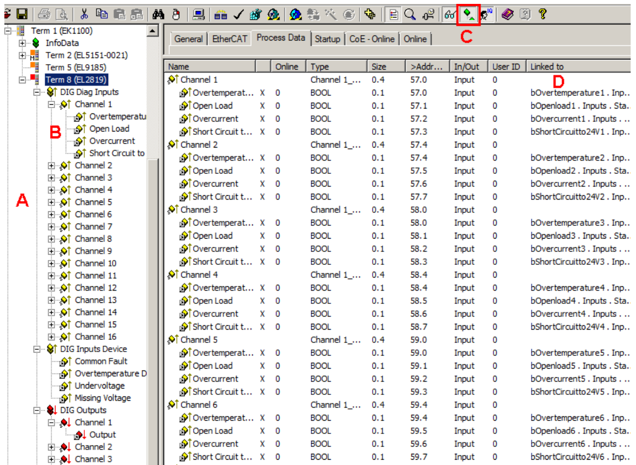
Abb. 19: EL2819 Online - Darstellung der Prozessdaten und Strukturinhalte im System Manager
