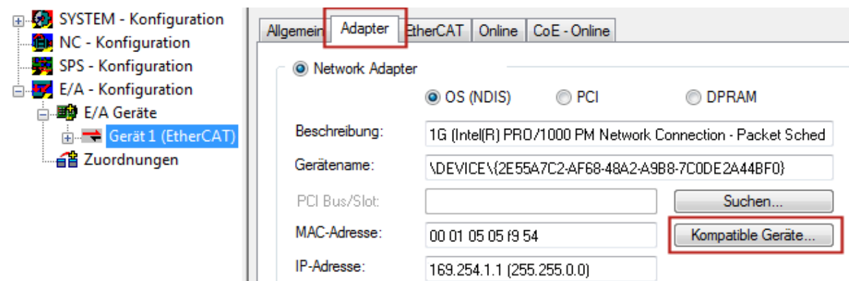
Abb. 97: Eigenschaft von EtherCAT-Gerät (TwinCAT 2): Klick auf „Kompatible Geräte...“ von „Adapter“
