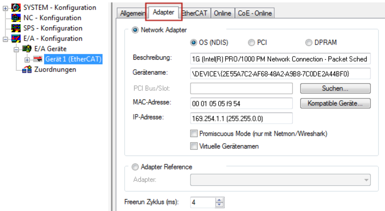
Abb. 114: Eigenschaften EtherCAT-Gerät (TwinCAT 2)
