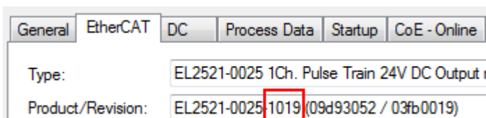
Abb. 127: Erkennen EtherCAT-Klemme mit Revision -1019
