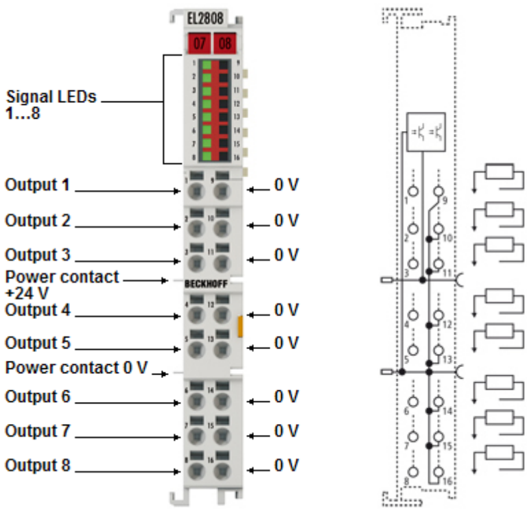
Abb. 8: EL2808
