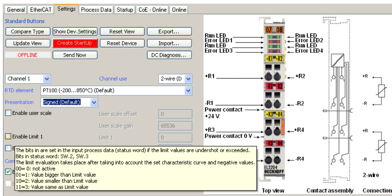
Abb. 155: Beispiel Inbetriebnahmehilfe für eine EL3204
