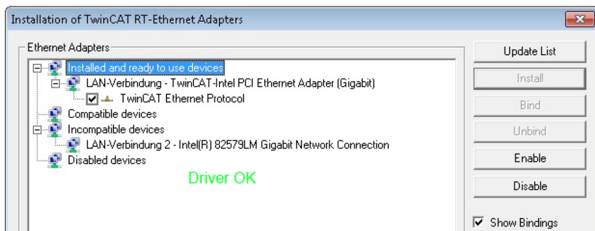
Abb. 99: Beispielhafte korrekte Treiber-Einstellung des Ethernet Ports
