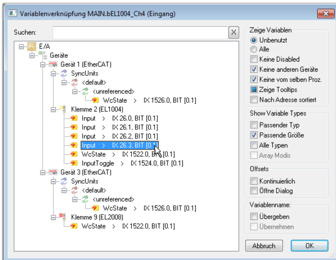
Abb. 85: Auswahl des PDO vom Typ BOOL
