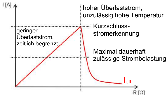
Abb. 15: Strombegrenzung bei Überlast
