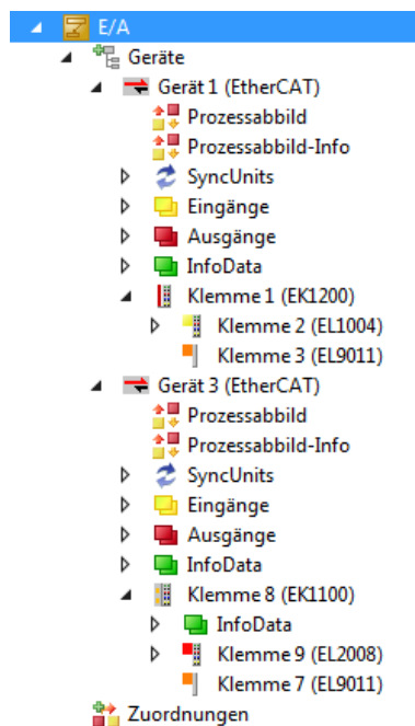
Abb. 77: Abbildung der Konfiguration in VS Shell der TwinCAT 3 Umgebung
