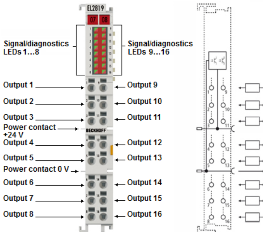
Abb. 13: EL2819
