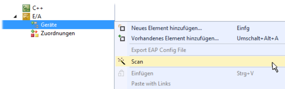
Abb. 75: Auswahl „Scan“
