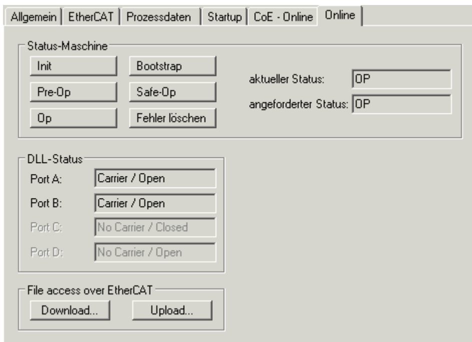
Abb. 150: Karteireiter „Online“
