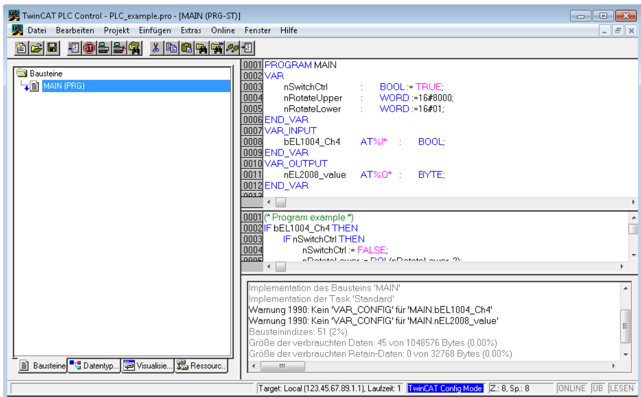
Abb. 61: Beispielprogramm mit Variablen nach einem Kompiliervorgang (ohne Variablenanbindung)
