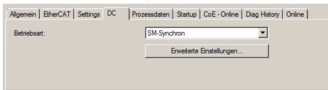
Abb. 151: Karteireiter „DC“ (Distributed Clocks)
