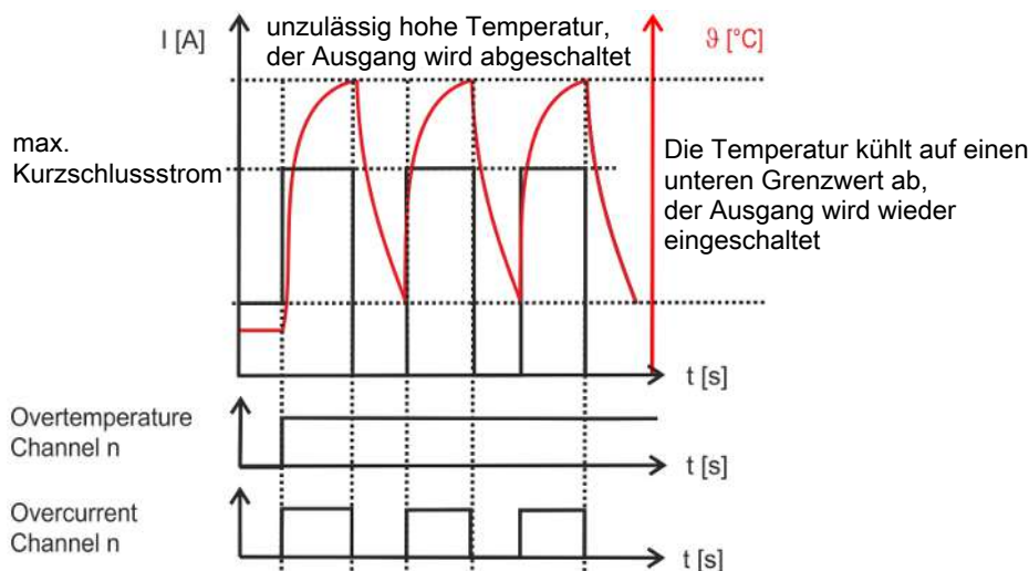
Abb. 16: Schematische Darstellung der thermischen Abschaltung bei Überlast
