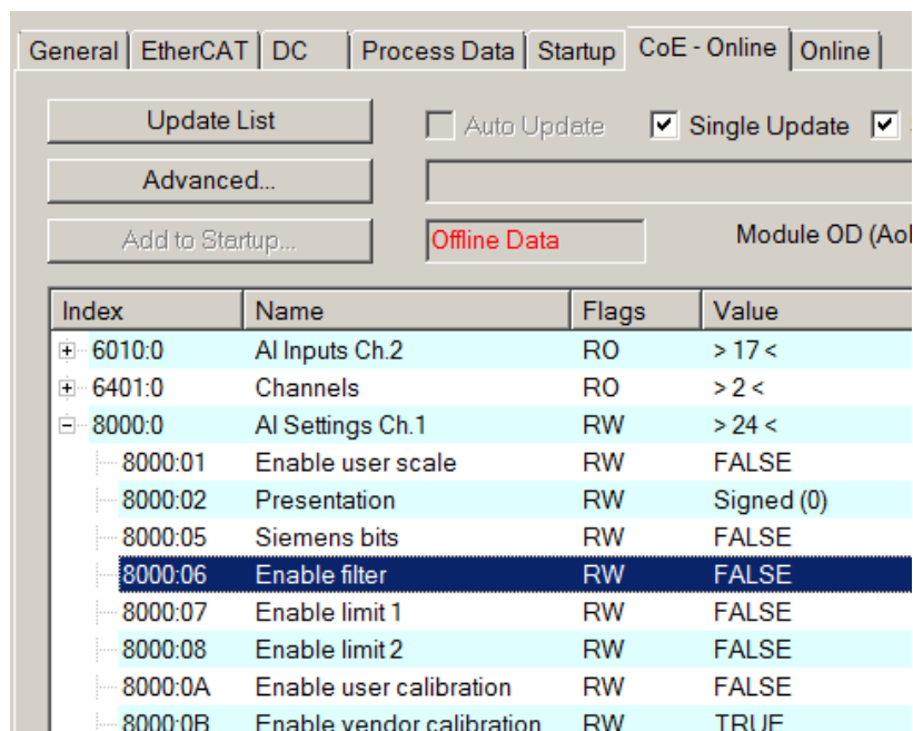
Abb. 154: EL3102, CoE-Verzeichnis
