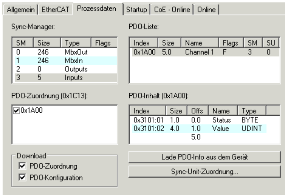
Abb. 145: Karteireiter „Prozessdaten“
