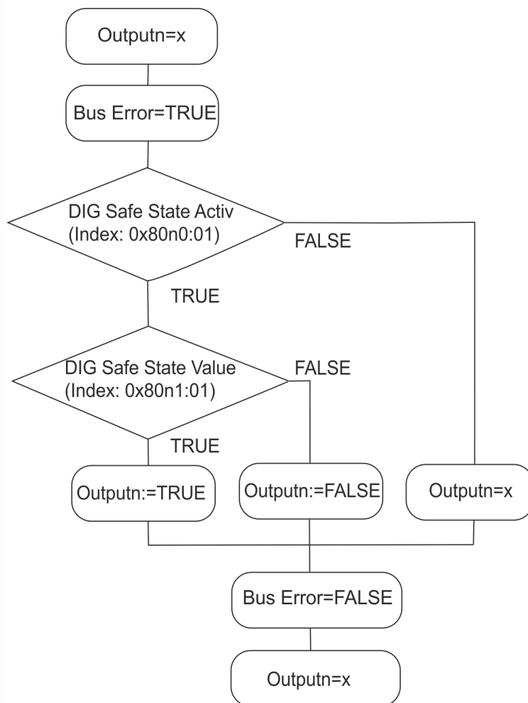
Abb. 22: Zustandsänderung der Ausgänge bei Busfehler
