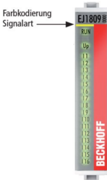
Abb. 20: EJ-Module Farbcode am Beispiel EJ1809
