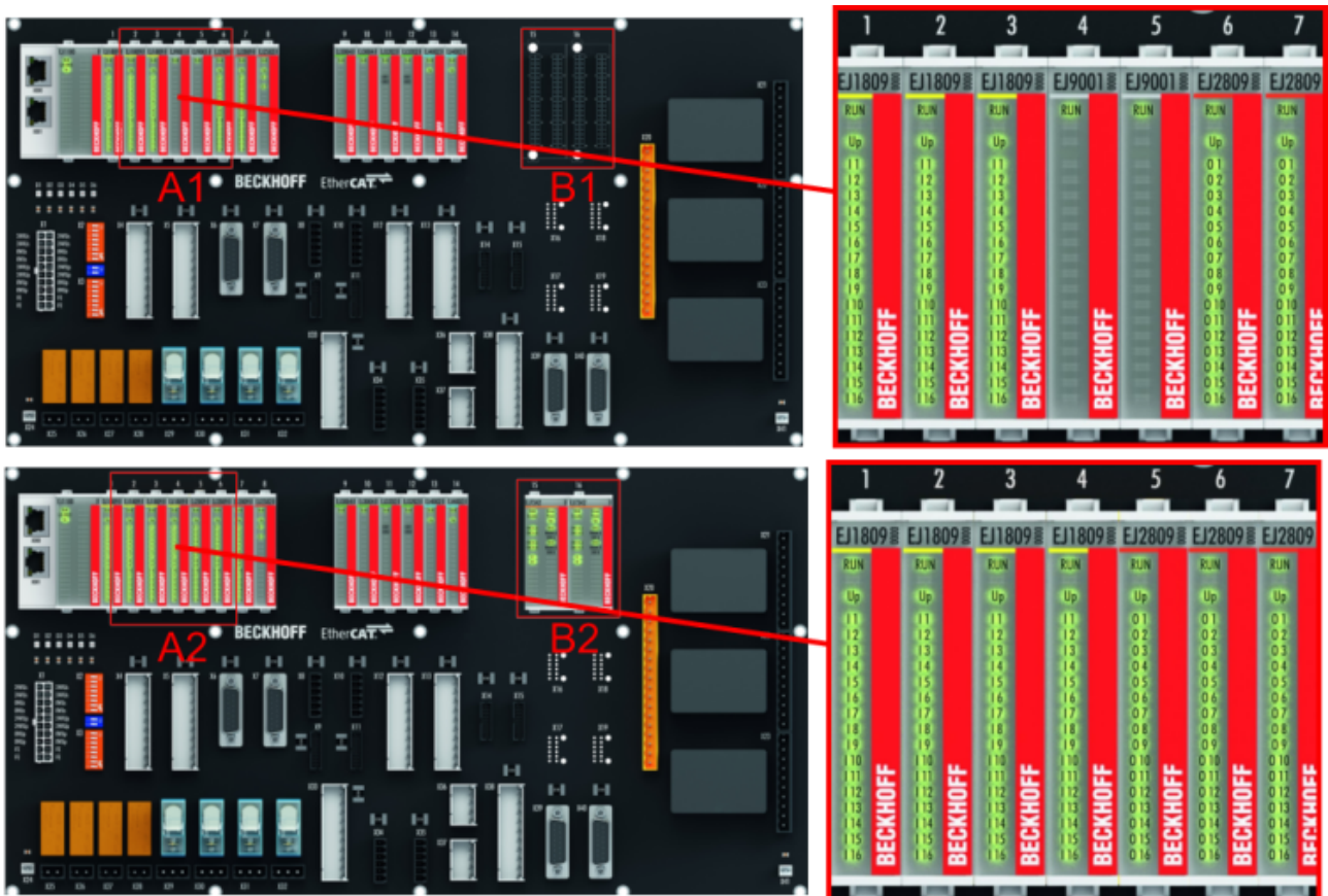
Abb. 37: Beispiel Austausch Platzhaltermodule u. Belegung Reserveslots
