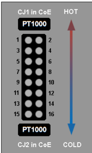
Abb. 22: Temperaturgradient über die verbundenen Anschlüsse der TCs
