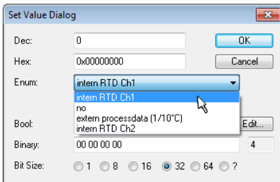
Abb. 25: CJC Auswahldialog
