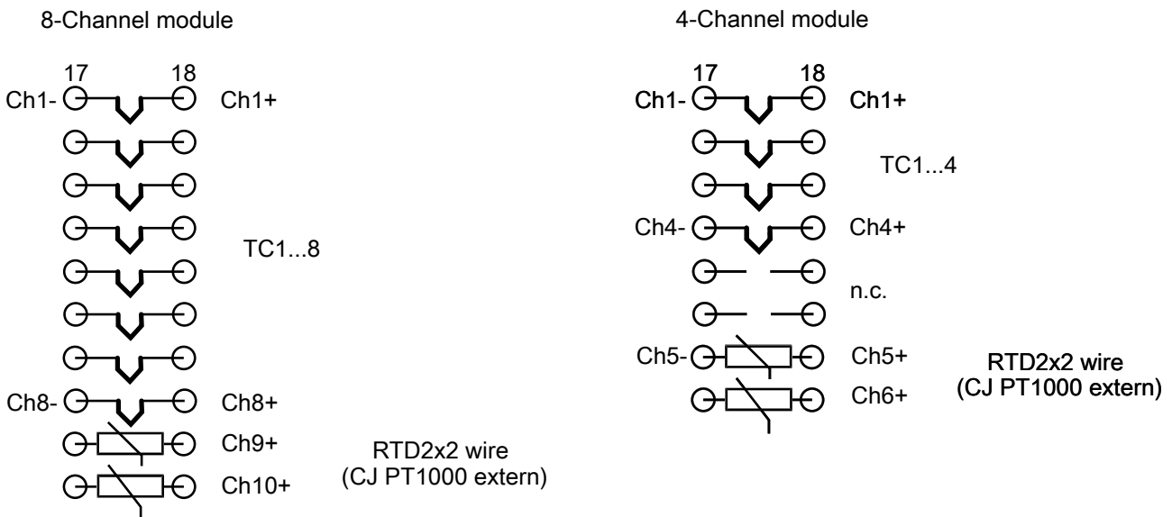
Abb. 20: TC/ RTD Anschlüsse an der „Backplane“
