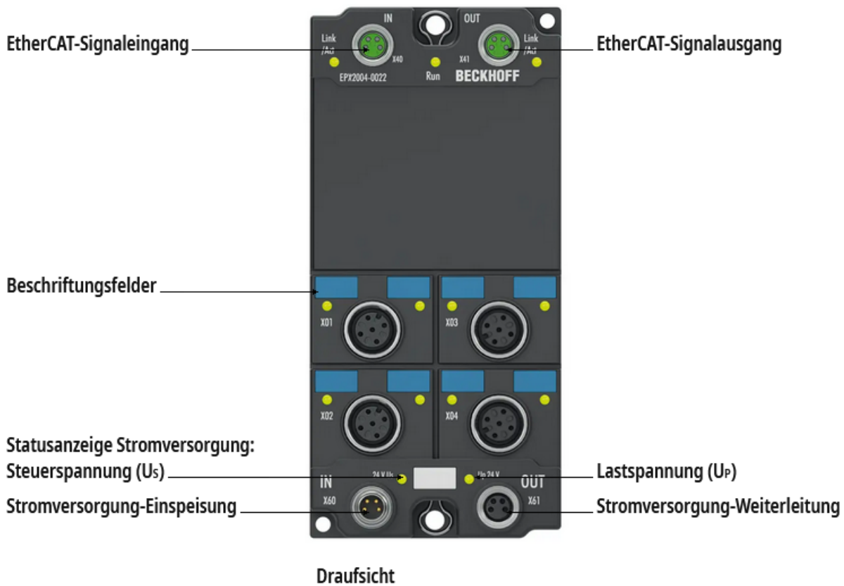
Abb. 2: EPX2004-0022 - EtherCAT Box, 4-Kanal-Digital-Ausgang, 24 V DC, 50 mA, M12, Ex i
