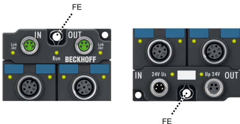
Abb. 4: EPX-EtherCAT-Box - Funktionserdung über die Befestigungslöcher
