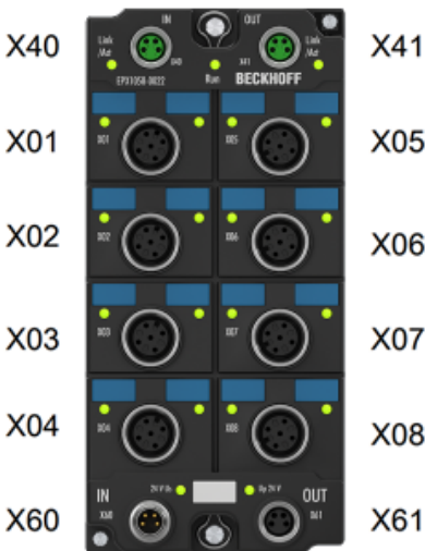
Abb. 5: Steckverbinder am Beispiel der EPX1058-0022
