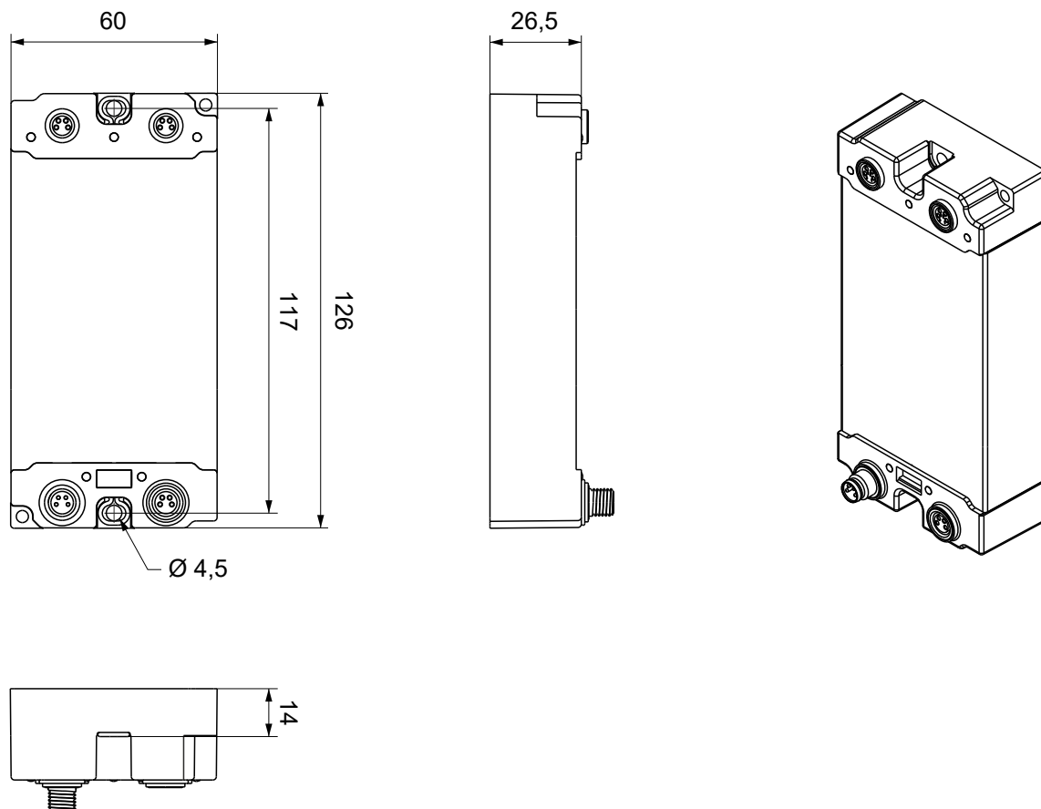
Abb. 3: EPX-EtherCAT-Box - Abmessungen
