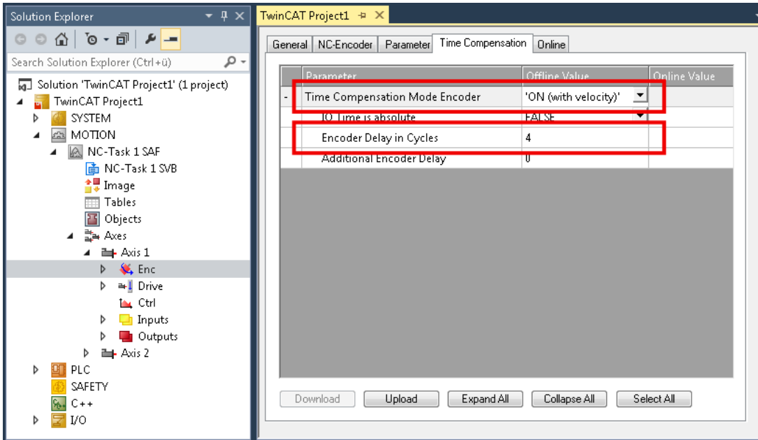
Fig. 15: Dead time compensation parameter
