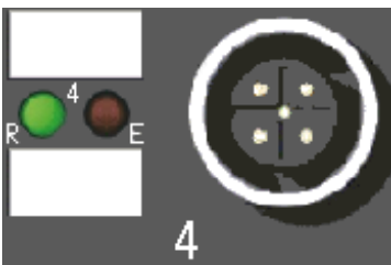
Abb. 4: Status- und Diagnose-LED am M12-Steckverbinder
