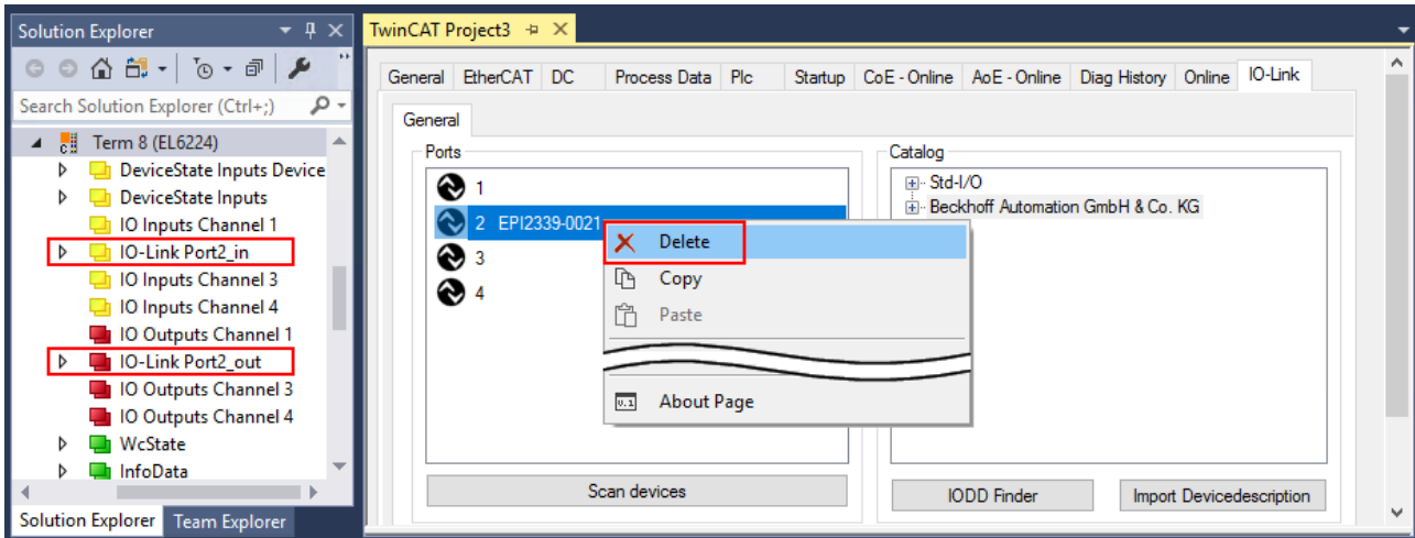
Abb. 22: Das Device an Port2 entfernen.
