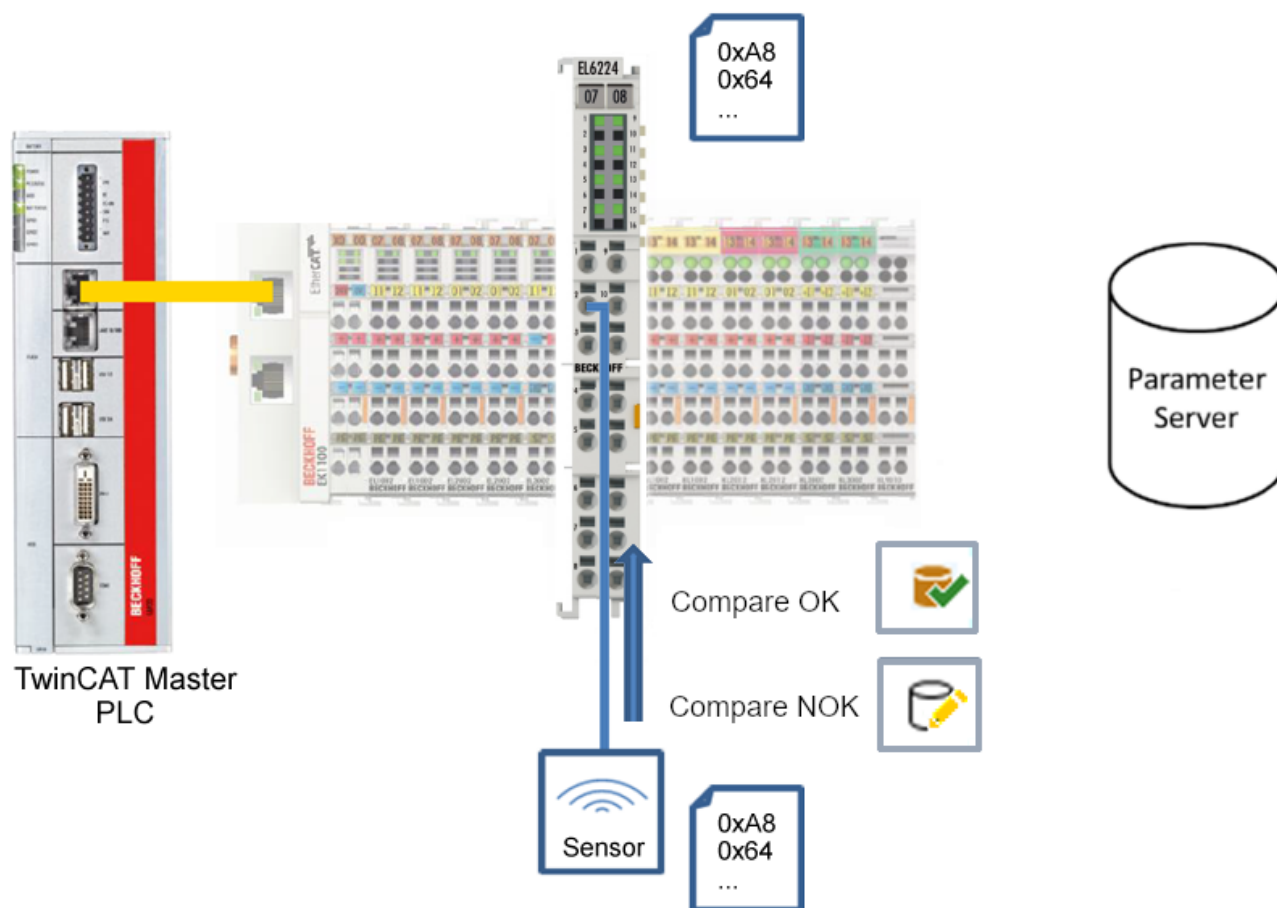
Abb. 28: Parameterdaten der Konfiguration mit Sensordaten vergleichen
