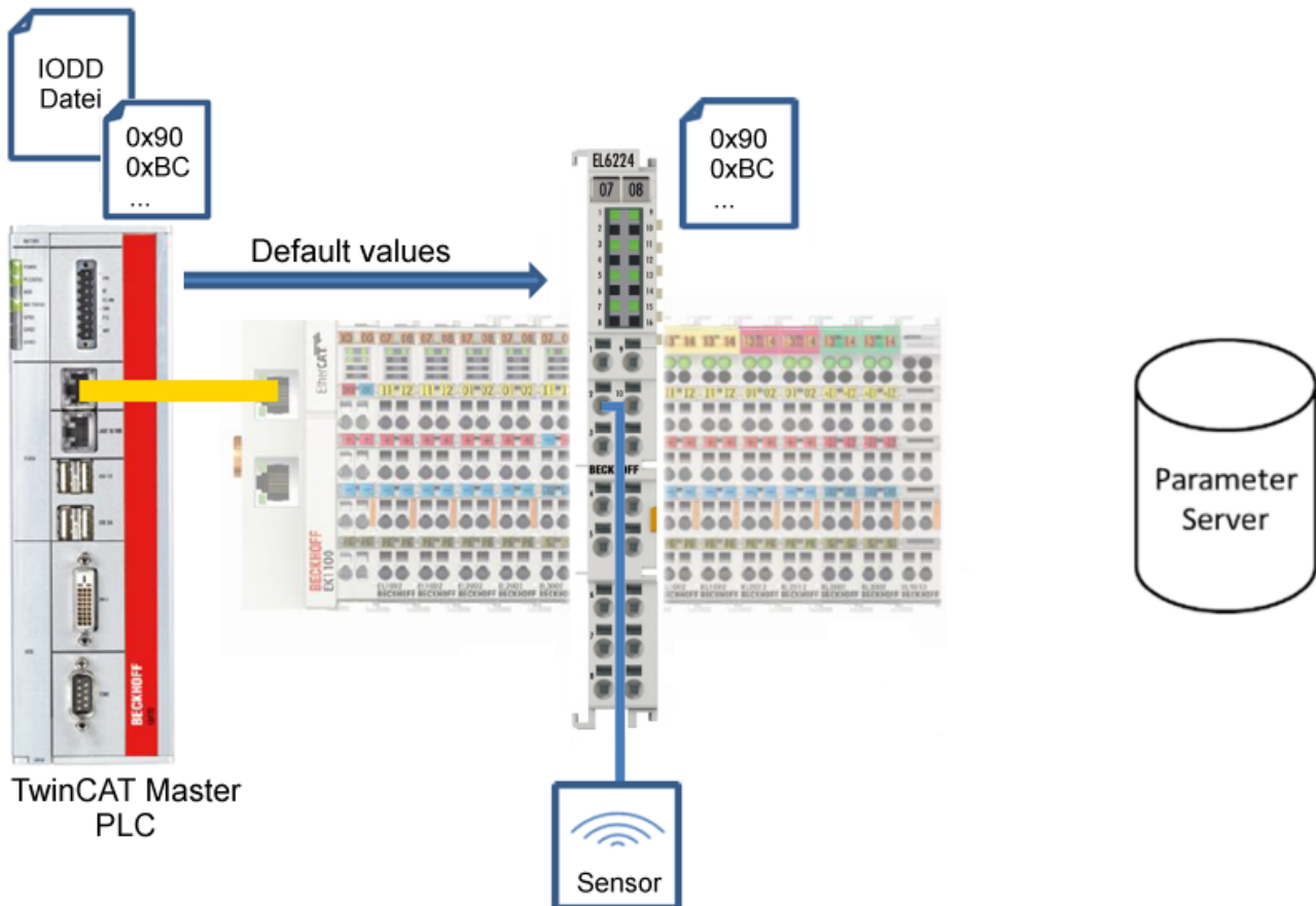
Abb. 30: Parameter auf Default-Werte zurücksetzen
