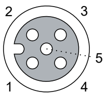
Abb. 7: M12-Buchse
