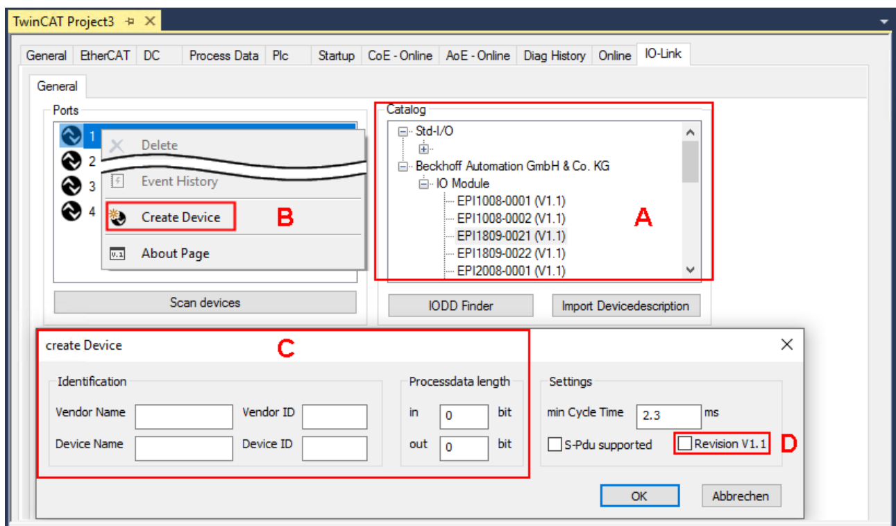
Abb. 21: Manuelles Anlegen eines IO-Link Devices über den "Create Device" Dialog (C)
