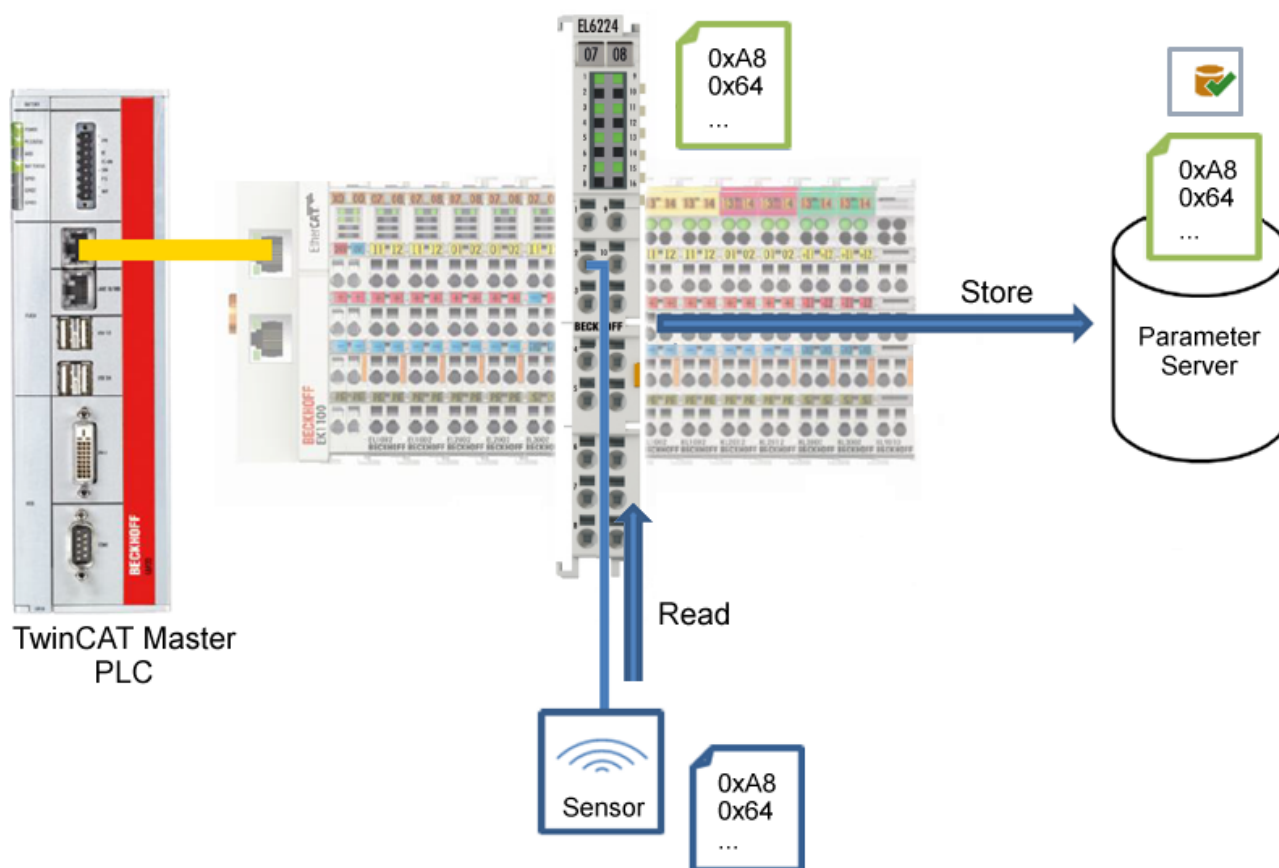
Abb. 35: Parameter speichern
