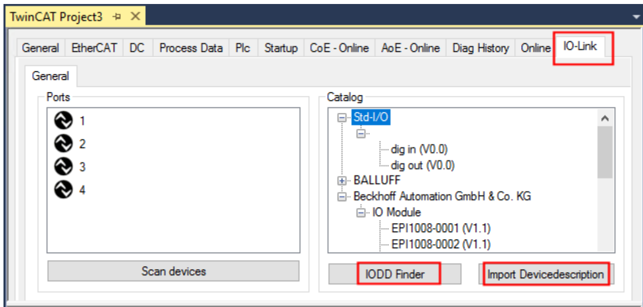
Abb. 13: Import der IODD Gerätebeschreibung über „IODD Finder“ oder „Import Devicedescription“
