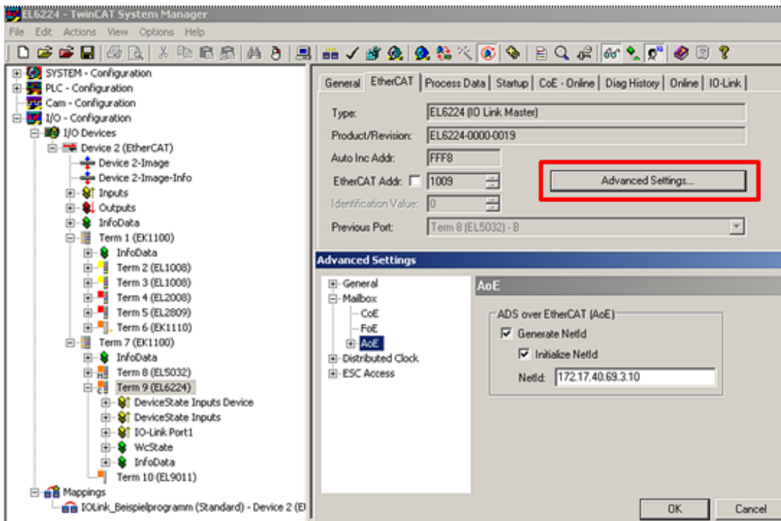
Abb. 40: Vergabe AoE-NetID
