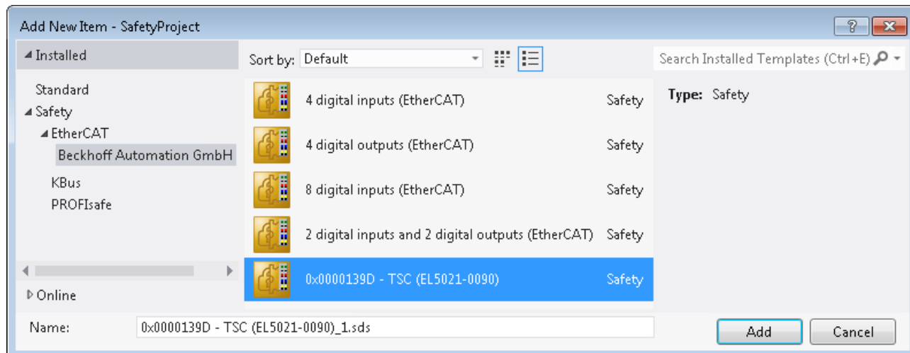
Abb. 44: Hinzufügen einer TwinSAFE-SC-Verbindung
