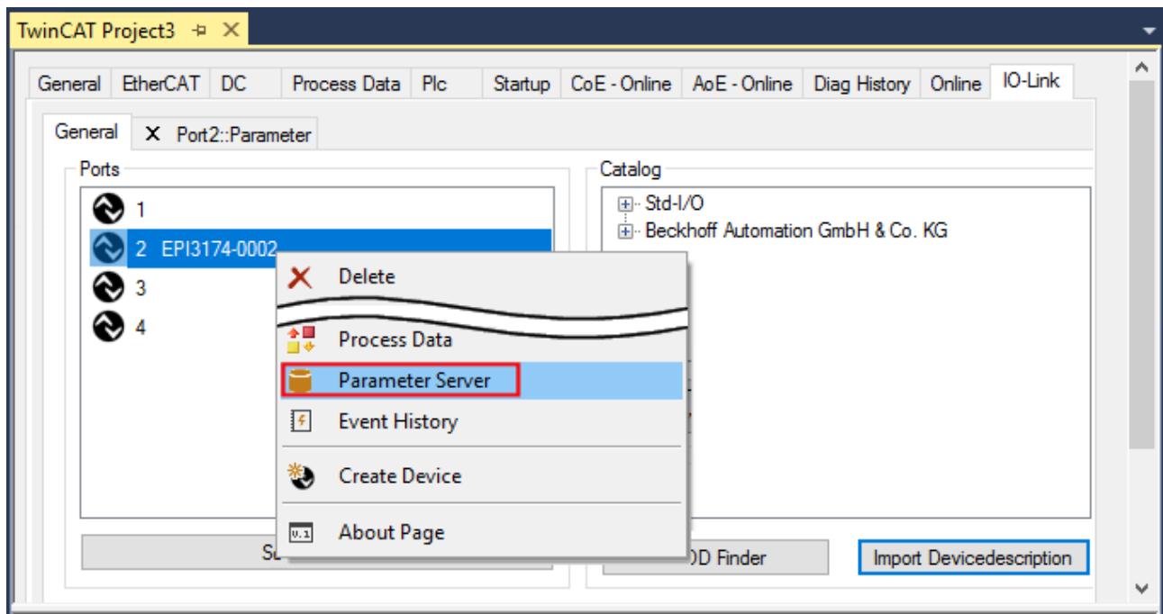
Abb. 32: Reiter „Parameter Server“ öffnen
