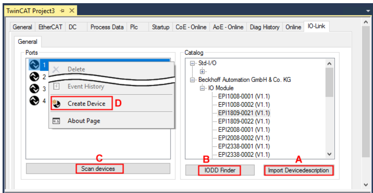
Abb. 12: Anlegen von IO-Link Devices
