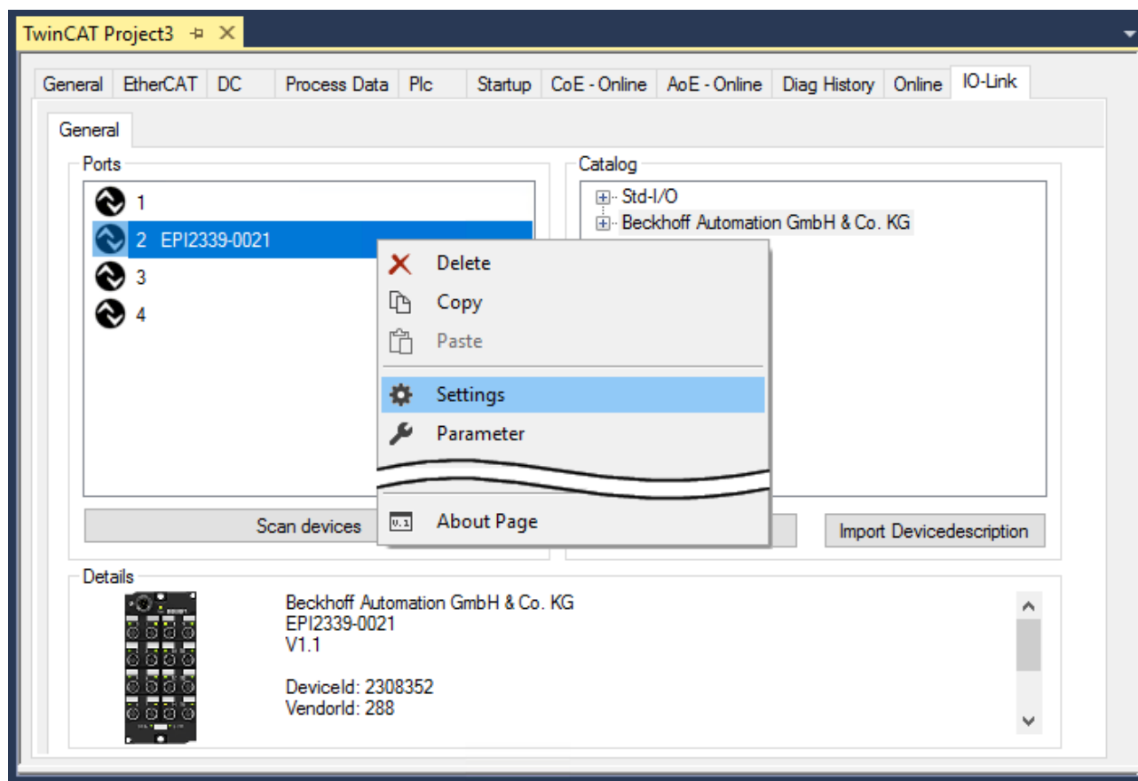
Abb. 18: Device an Port2, Anzeige „Details“, Reiter „Settings“ und „Parameter“ öffnen
