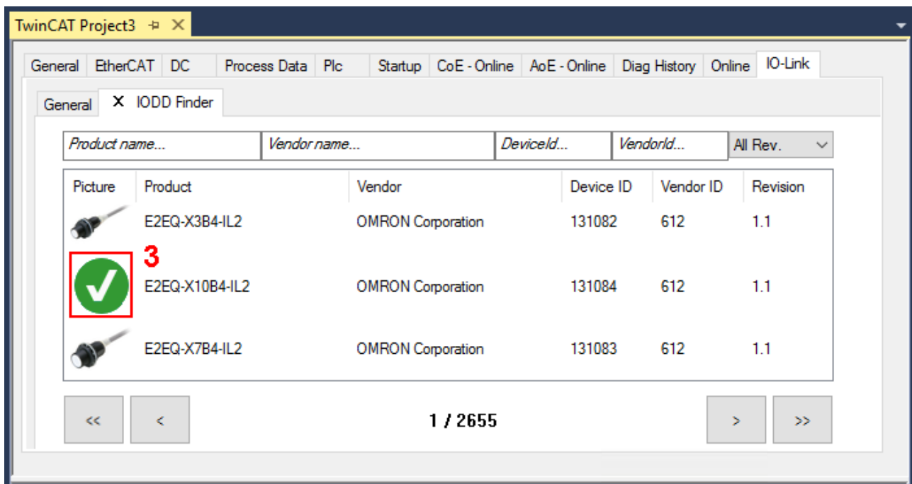
Abb. 15: IODD Finder, Anzeige einer bereits importierten Gerätebeschreibung
