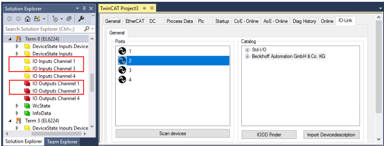
Abb. 23: Das Device an Port2 wurde entfernt, die Prozessdaten werden im Baum nicht mehr angezeigt.
