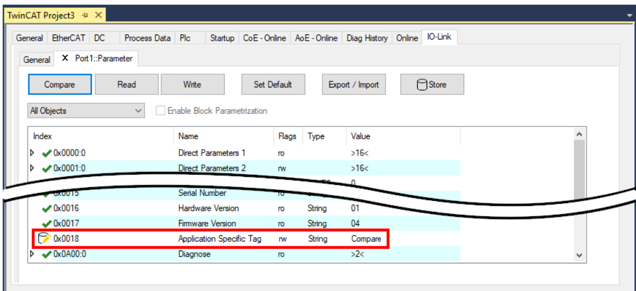
Abb. 27: Anzeige abweichender Daten im Reiter „Parameter“
