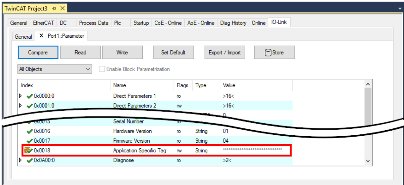
Abb. 26: Anzeige übereinstimmender Daten im Reiter „Parameter“
