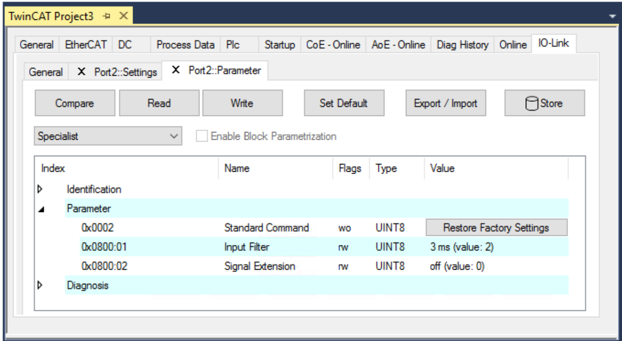
Abb. 20: Parameter Device Port2
