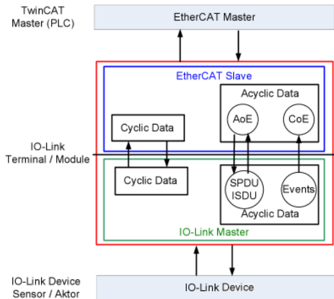
Abb. 38: Darstellung der Systemkommunikation eines EtherCAT-Masters
