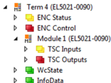
Abb. 43: Prozessdaten TwinSAFE SC Komponente, Beispiel EL5021-0090
