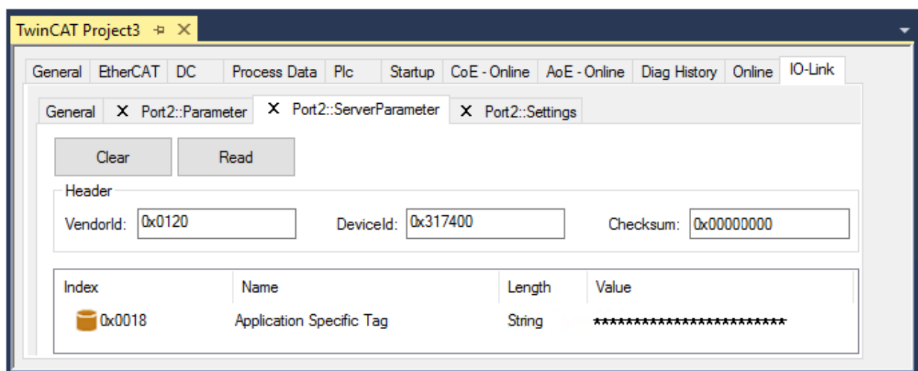
Abb. 33: Reiter „ServerParameter“
