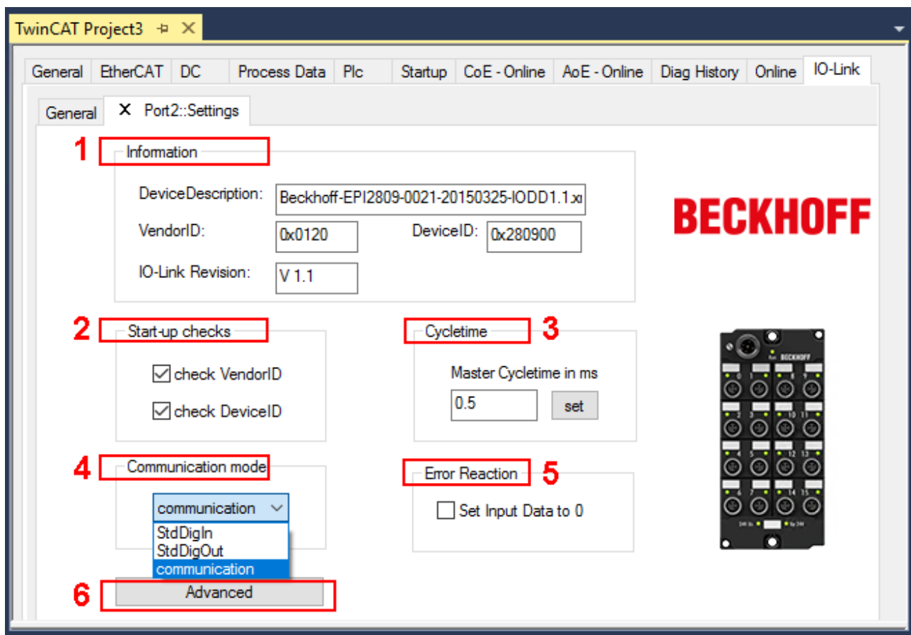
Abb. 25: Einstellungen der IO-Link Devices
