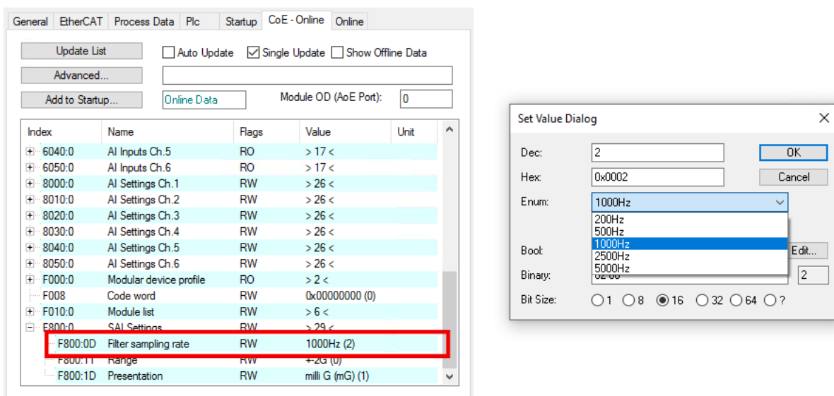
Abb. 6: Einstellung der internen Abtastfrequenz (Index 0xF800:0D)
