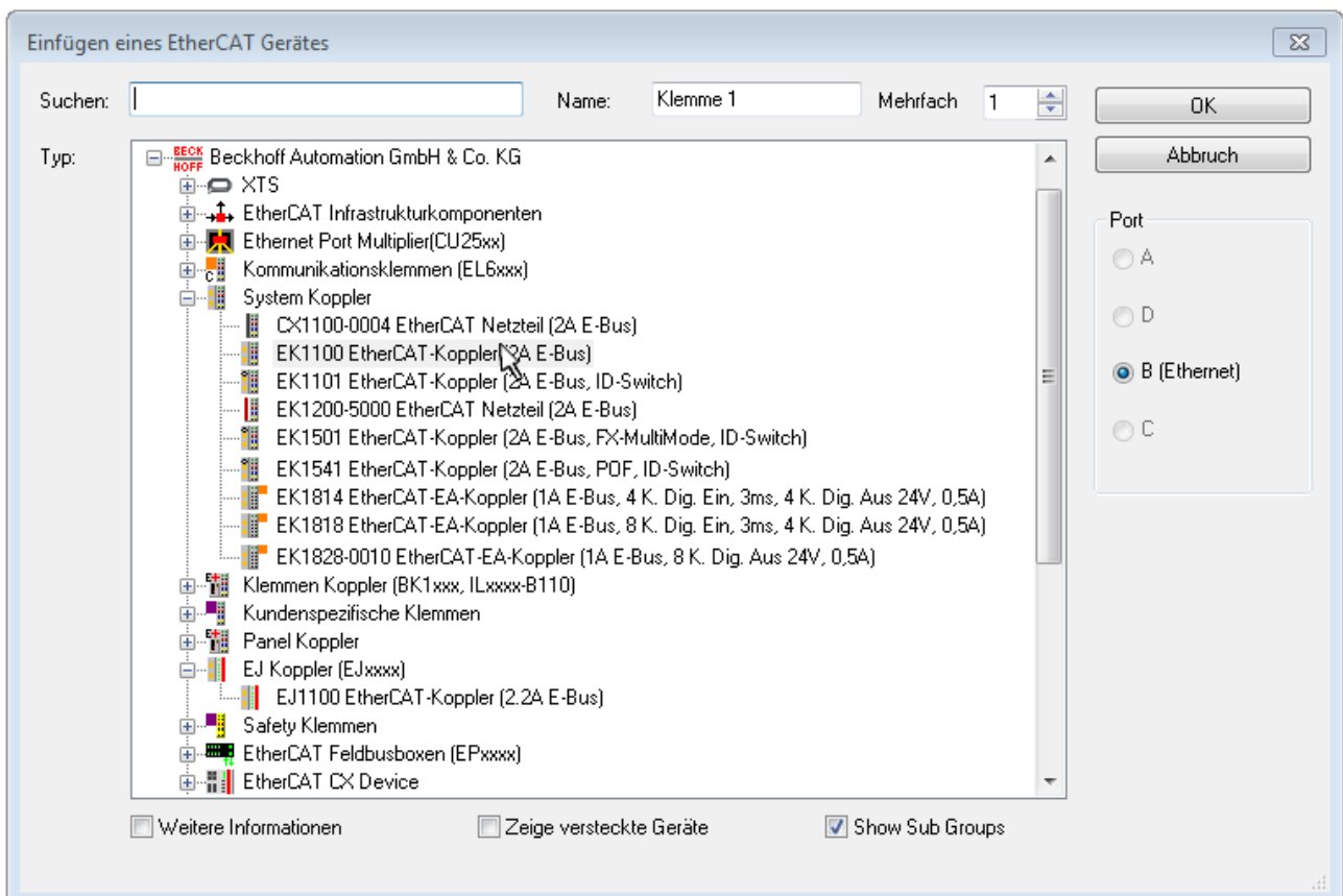
Abb. 45: Auswahldialog neues EtherCAT Gerät
