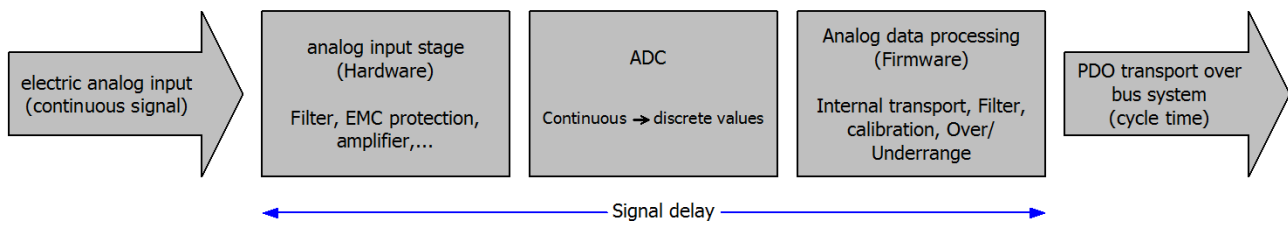
Abb. 20: Signalverarbeitung Analogeingang
