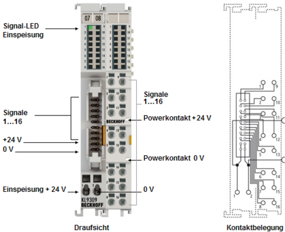
Abb. 8: KL9309
