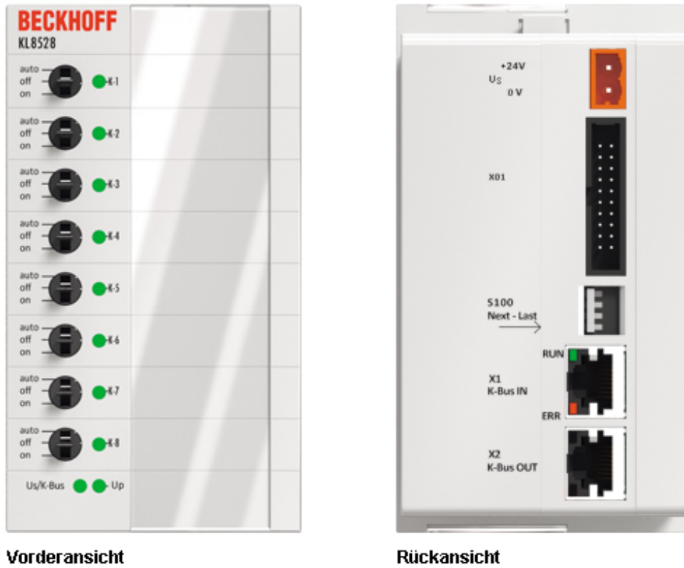
Abb. 5: KL8528
