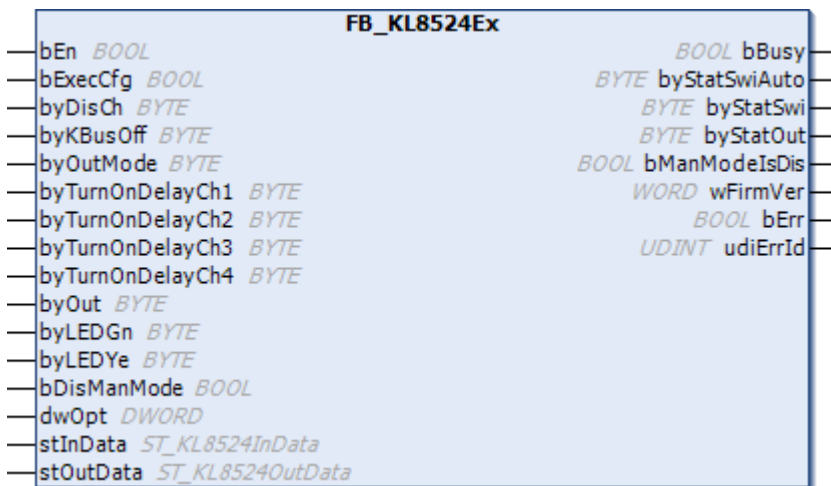
Abb. 26: Funktionsbaustein FB_KL8524Ex
