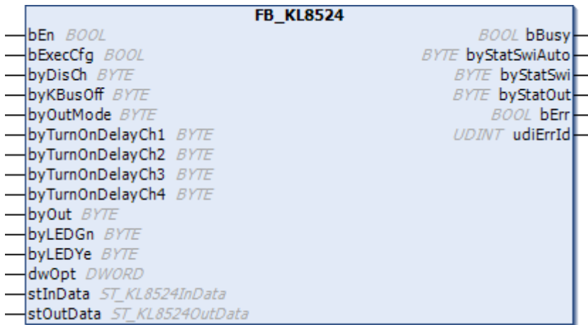
Abb. 25: Funktionsbaustein FB_KL8524
