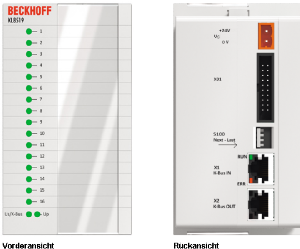
Abb. 3: KL8519
