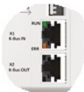
Abb. 10: Diagnose-LEDs auf der Rückseite
