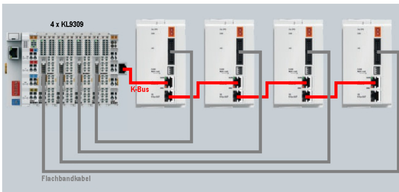
Abb. 16: Anschluss der Handbedienmodule über K-Bus-Verlängerung und Flachbandkabel
