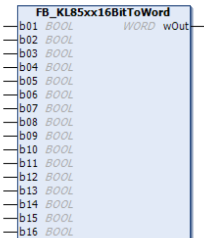
Abb. 31: Funktionsbaustein FB_KL85xx16BitToWorld
