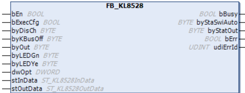
Abb. 27: Funktionsbaustein FB_KL8528
