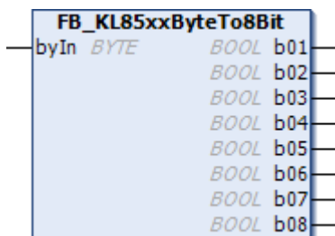
Abb. 33: Funktionsbaustein FB_KL85xxByteTo8Bit
