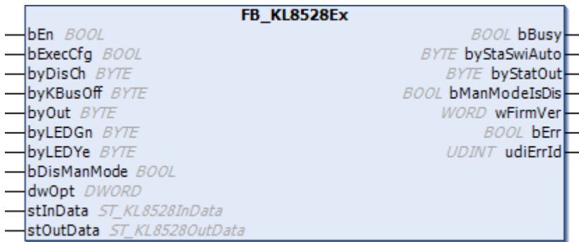
Abb. 28: Funktionsbaustein FB_KL8528Ex
