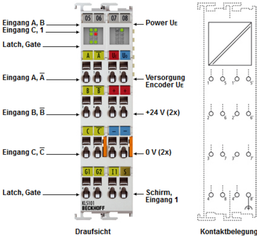
Abb. 2: Belegung der Klemmkontakte
