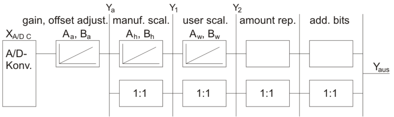
Abb. 10: Signalverarbeitung
