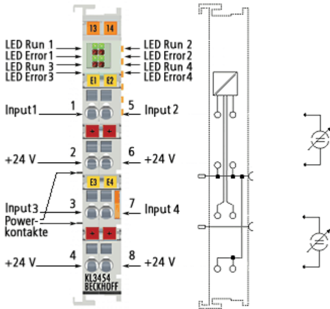
Abb. 20: KL3454 - Anschlussbelegung
