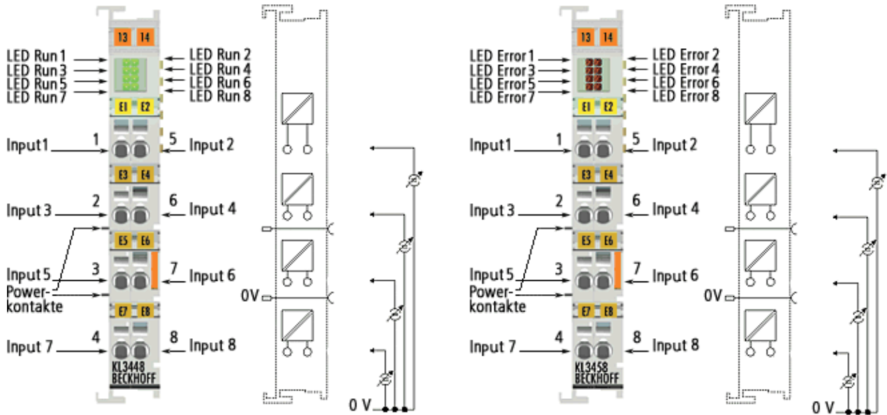
Abb. 21: KL3448, KL3458 - Anschlussbelegung
