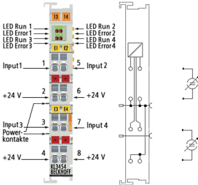
Abb. 4: KL3454
