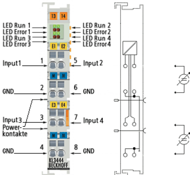
Abb. 3: KL3444
