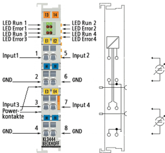
Abb. 19: KL3444 - Anschlussbelegung
