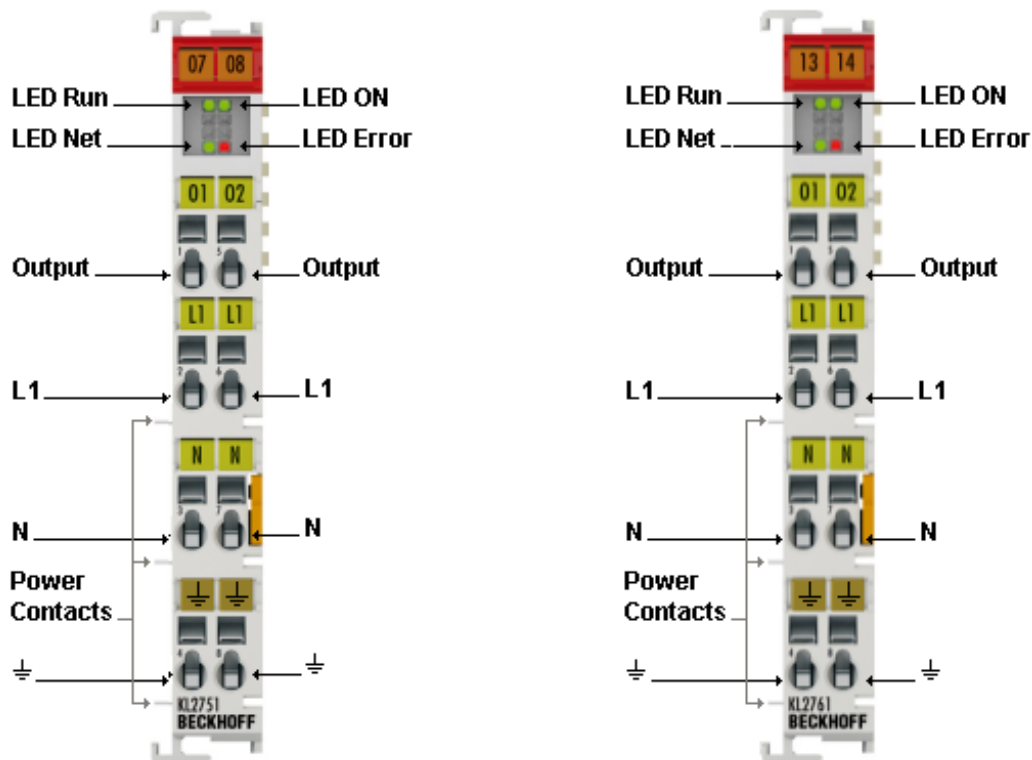
Fig. 3: KL2751, KL2761
