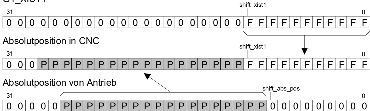
Fig. 34: Calculation mode for actual position
