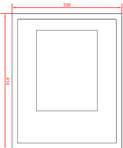
CP6921-0001 main dimensions
