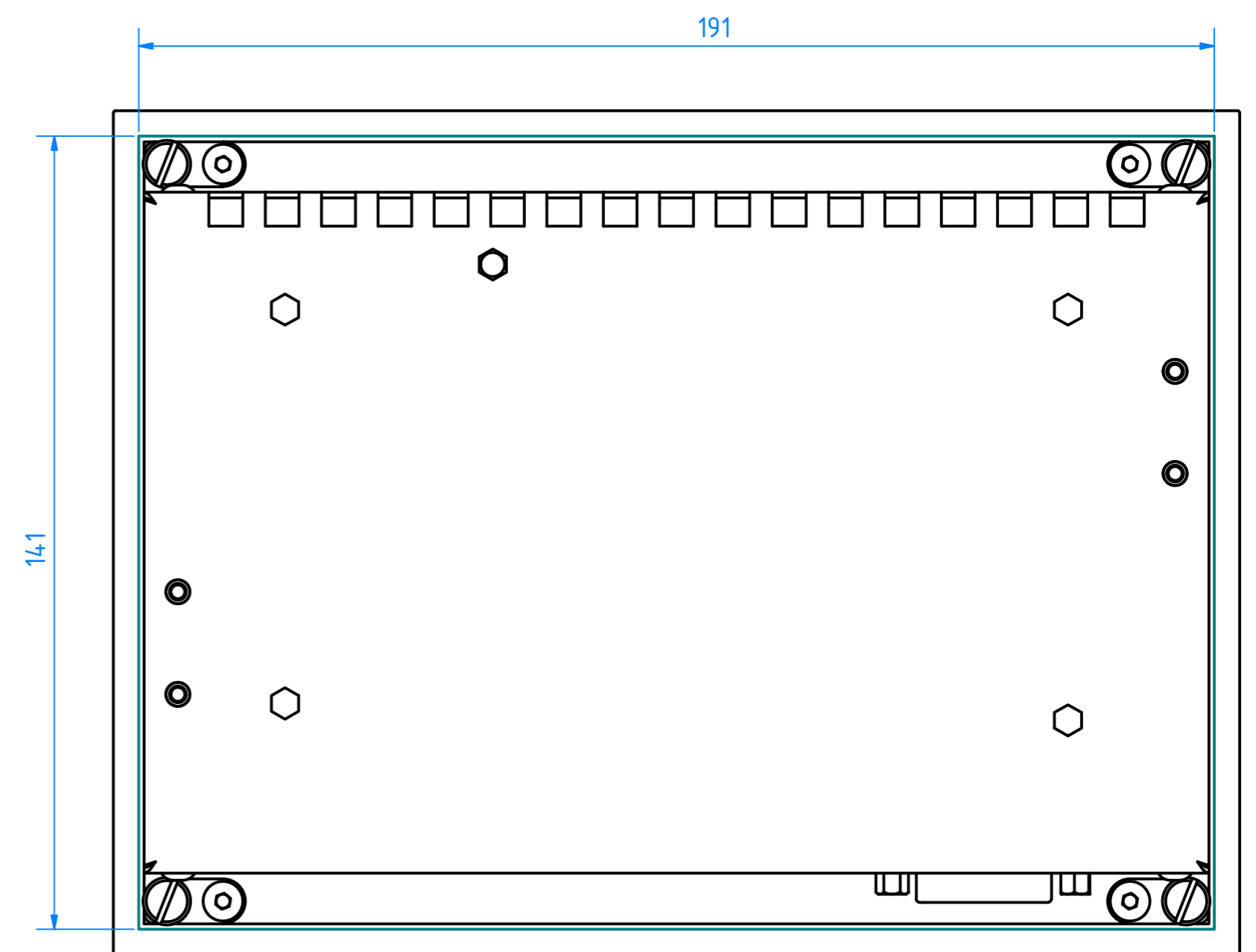
CP6906-0001-0000 main dimensions
