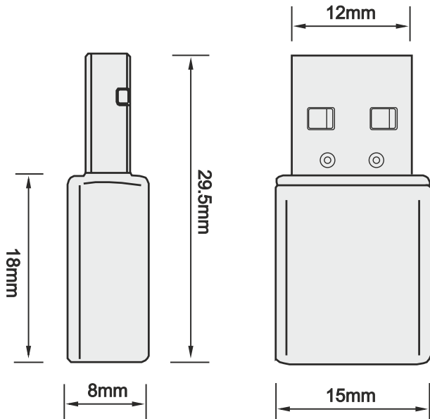
Abb. 4: CU8210-D001-0101 Abmessungen.
