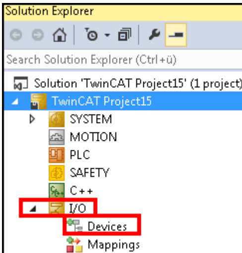
Fig. 30: XAE Project
