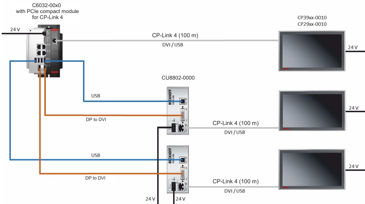
Fig. 15: CP-Link 4, CU8802-00x0
