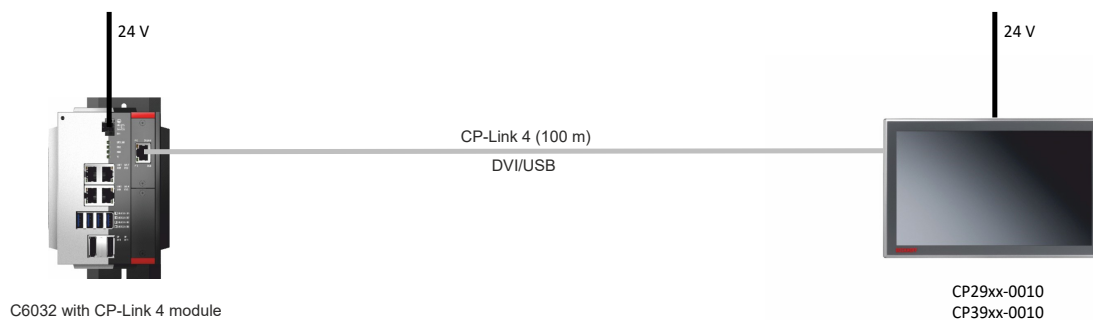
Fig. 14: CP-Link 4
