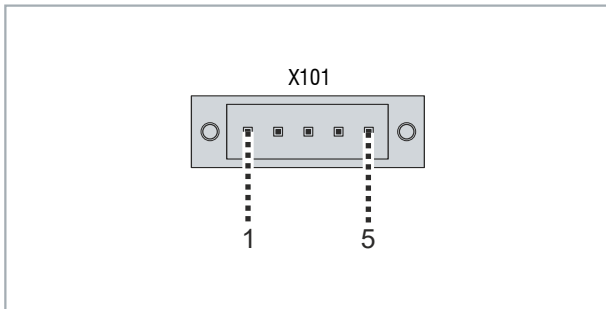
Abb. 2: Spannungsstecker Pin-Nummerierung
