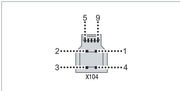
Abb. 3: USB-Schnittstelle Pin-Nummerierung
