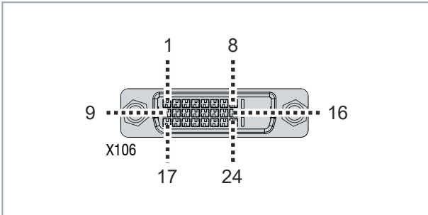
Abb. 4: DVI-Schnittstelle Pin-Nummerierung
