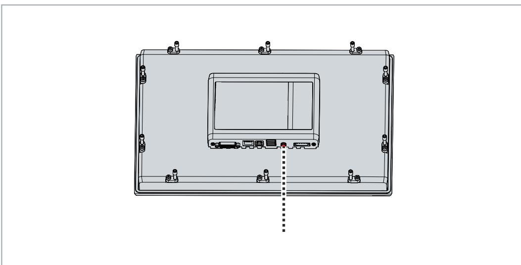
Abb. 16: Erdungsbolzen Funktionserdung
