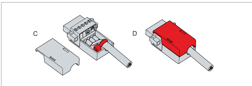
Abb. 14: Montage Oberteil Zugentlastungsgehäuse
