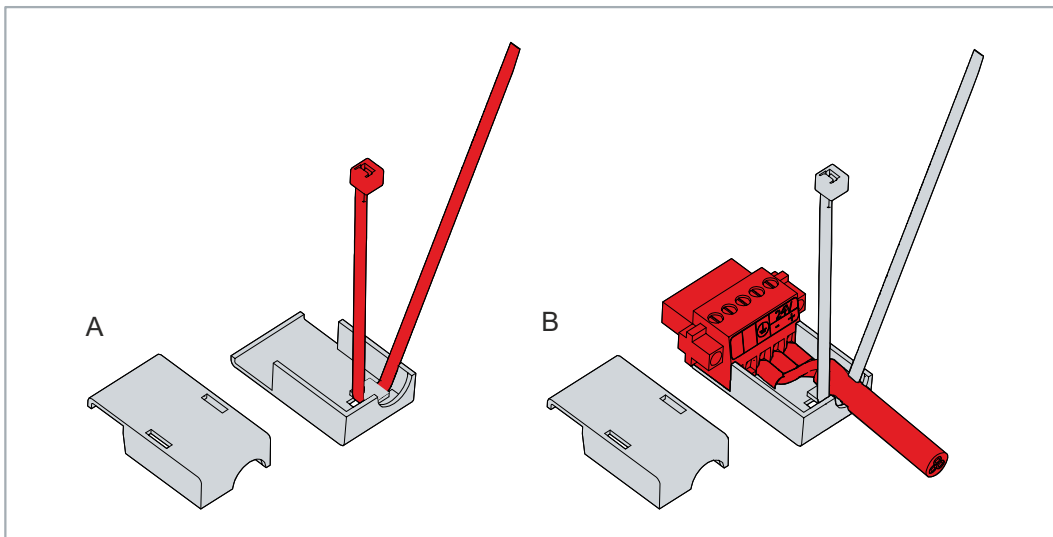
Abb. 13: Montage Unterteil Zugentlastungsgehäuse
