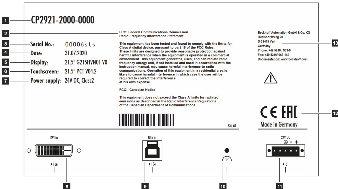
Abb. 5: Typenschild Beispiel
