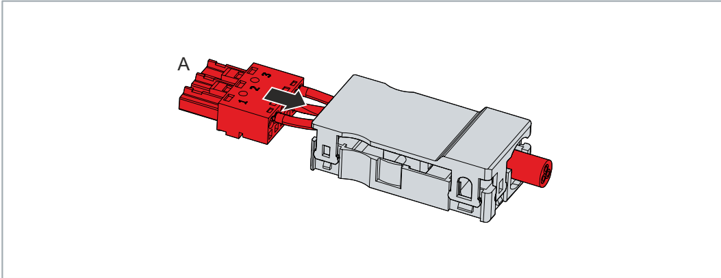
Abb. 16: Stecker einsetzen
