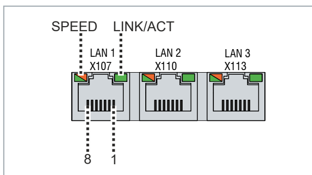
Abb. 6: Ethernet-Schnittstelle Pin-Nummerierung
