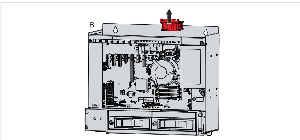
Abb. 35: Entfernen Lüfterhalter mit Lüfter
