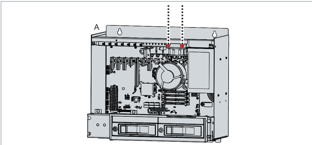
Abb. 34: Lösen Lüfterhalter
