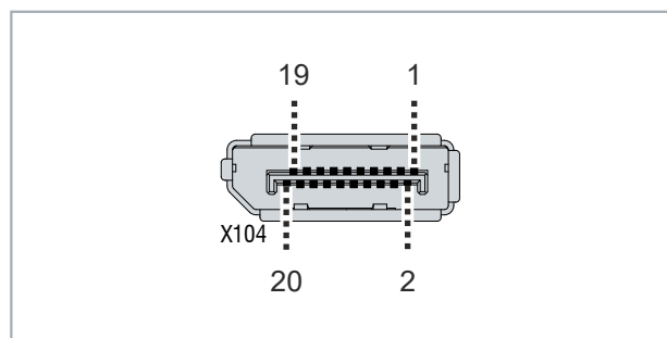
Abb. 9: DisplayPort Pin-Nummerierung
