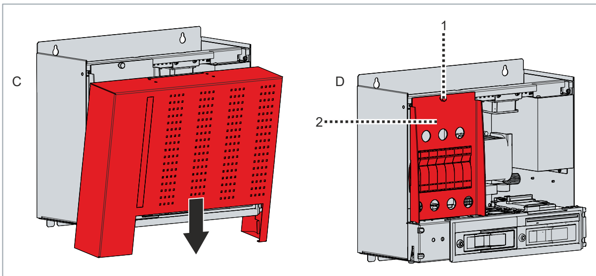
Abb. 24: Zugang Innenraum Gerät
