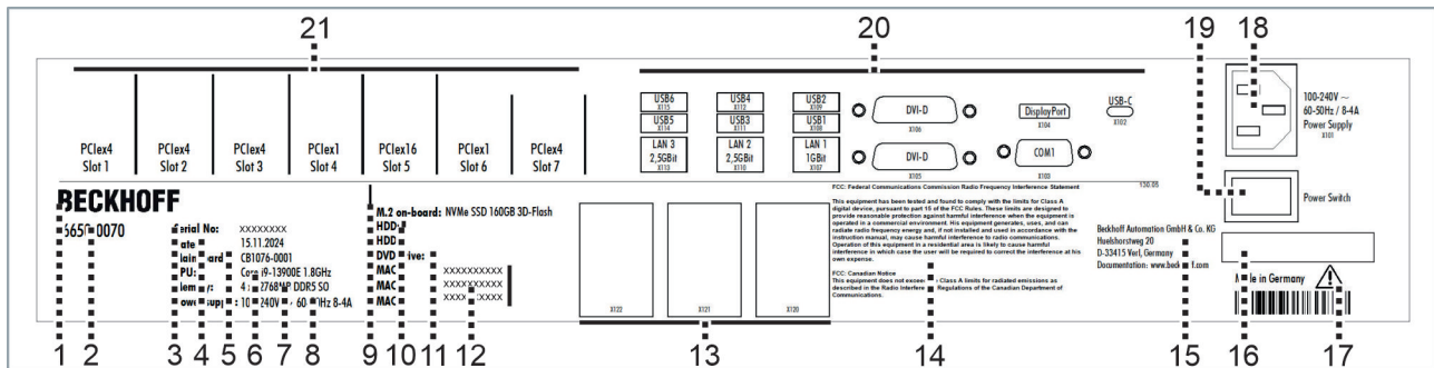
Abb. 10: Typenschild
