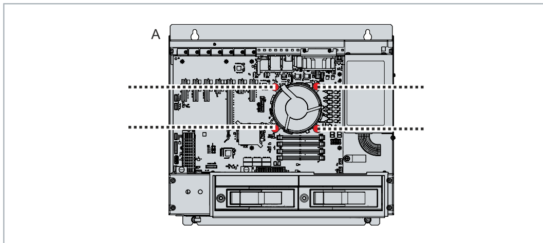
Abb. 36: Entriegelung CPU-Kühler
