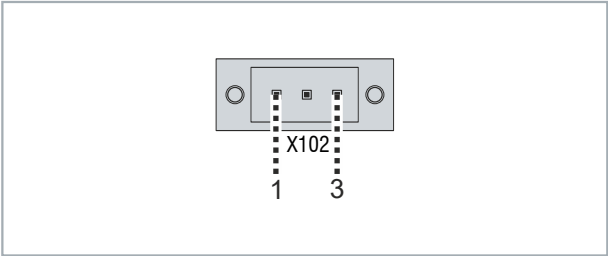
Abb. 4: Buchse externe Beschaltung Pin-Nummerierung
