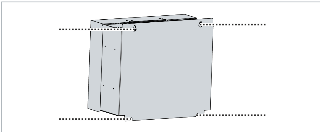
Abb. 13: Schaltschrankeinbau
