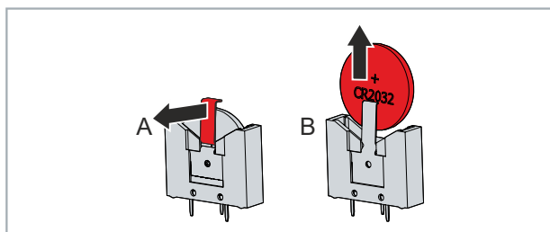
Abb. 28: Austausch Batterie
