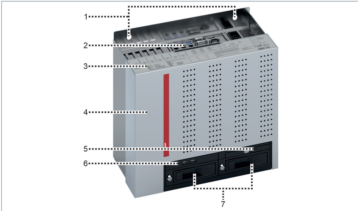
Abb. 1: Aufbau
