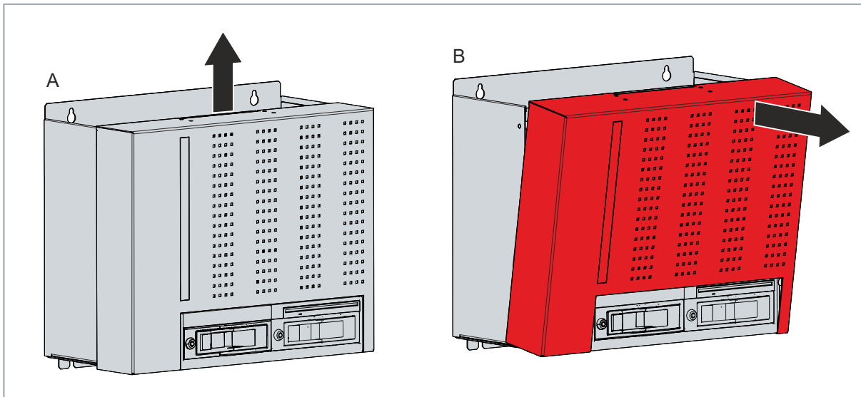
Abb. 23: Entriegelung Gehäusedeckel
