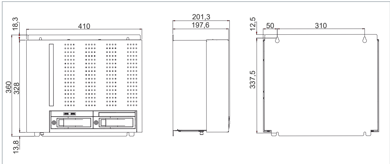
Abb. 12: Abmessungen
