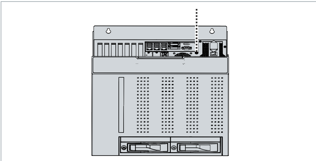
Abb. 14: Erdungsbolzen Funktionserdung
