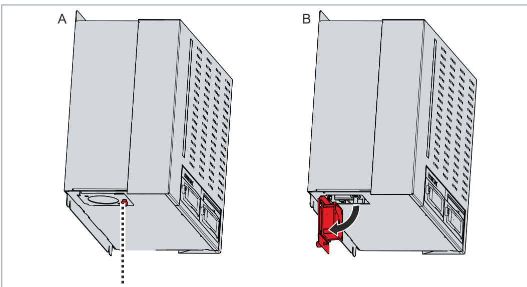
Abb. 32: Lösen Lüfterkassette
