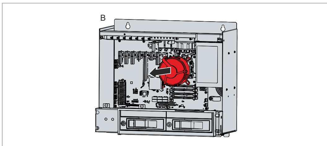
Abb. 37: Entnahme CPU-Kühler
