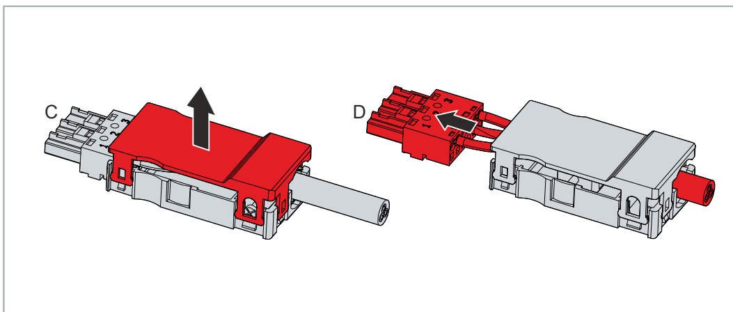
Abb. 19: Zugentlastungsgehäuse entfernen
