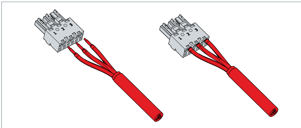
Abb. 15: Montage Versorgungsleitung
