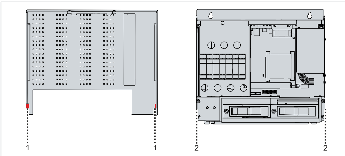
Abb. 26: Haken und Führungen
