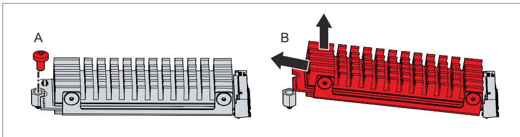
Abb. 30: Austausch NVMe™-M.2-SSD
