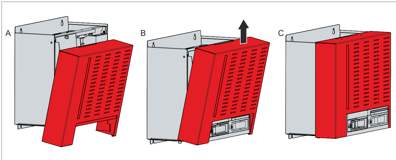
Abb. 27: Montage Gehäusedeckel
