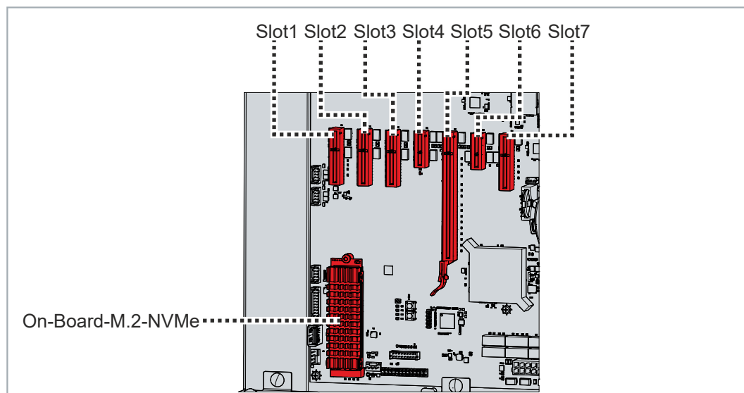
Abb. 29: Nummerierung PCIe®-Steckkartenslots
