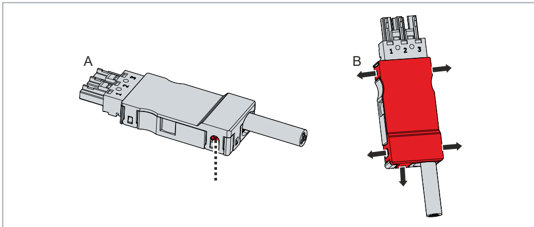
Abb. 18: Zugentlastungsgehäuse lösen
