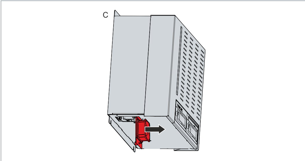
Abb. 33: Entnahme Lüfterkassette
