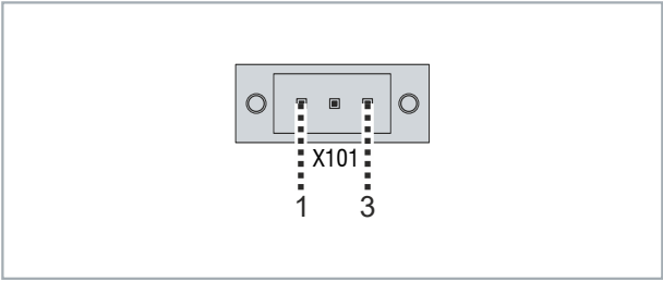
Abb. 3: Spannungsbuchse Pin-Nummerierung
