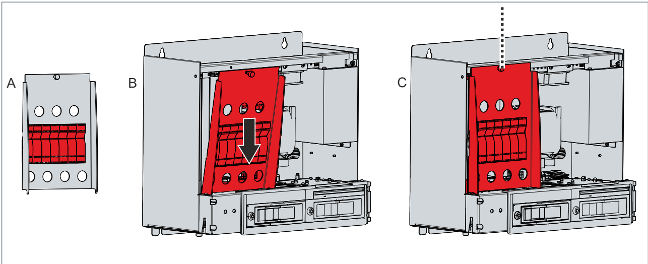
Abb. 25: Montage Kartenniederhalter
