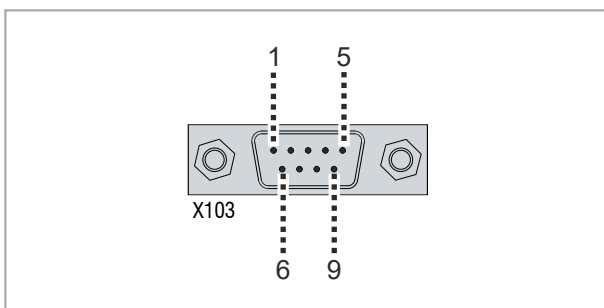
Abb. 9: RS232-Schnittstelle Pin-Nummerierung
