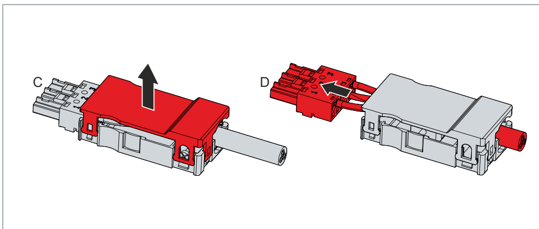
Abb. 20: Zugentlastungsgehäuse entfernen
