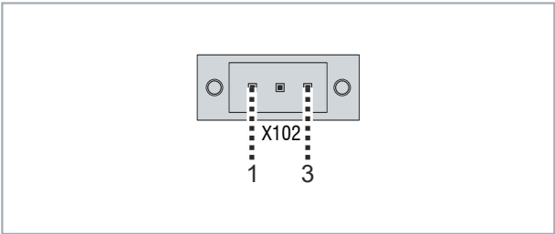
Abb. 5: Buchse externe Beschaltung Pin-Nummerierung
