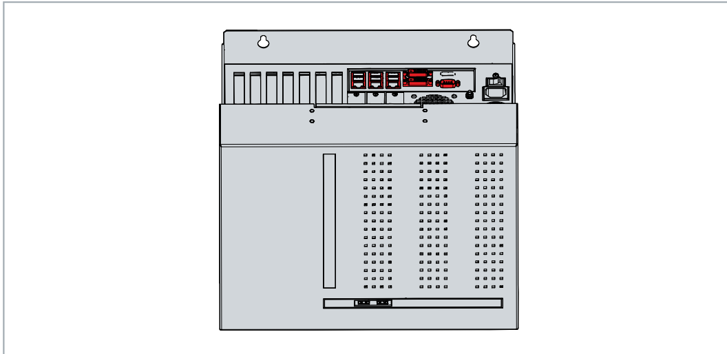
Abb. 2: Anschlussbereich
