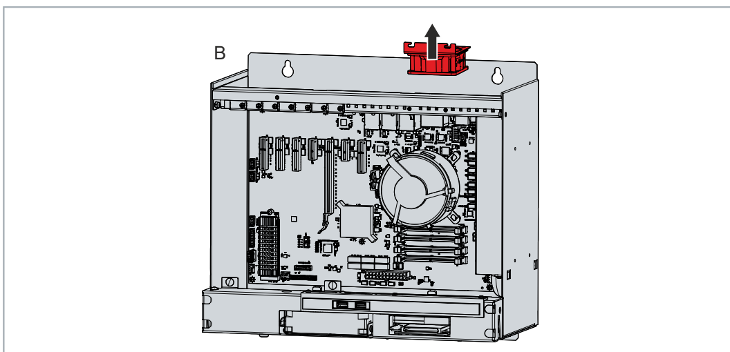
Abb. 36: Entfernen Lüfterhalter mit Lüfter
