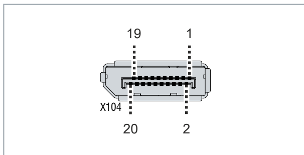
Abb. 10: DisplayPort Pin-Nummerierung
