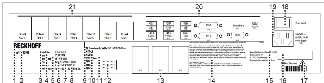
Abb. 11: Typenschild
