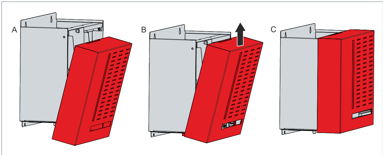
Abb. 28: Montage Gehäusedeckel
