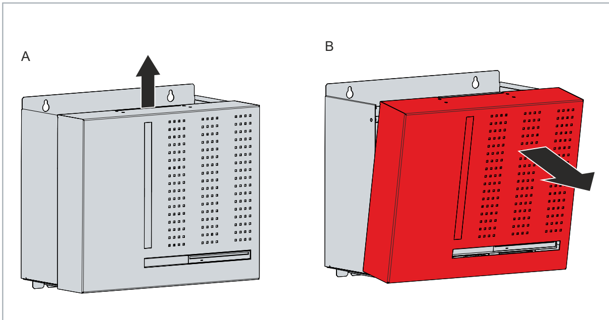
Abb. 24: Entriegelung Gehäusedeckel
