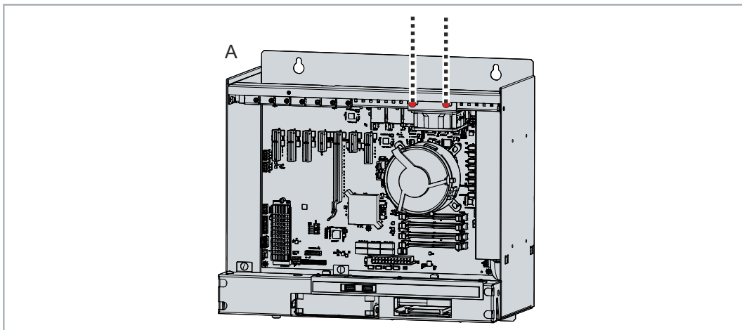
Abb. 35: Lösen Lüfterhalter
