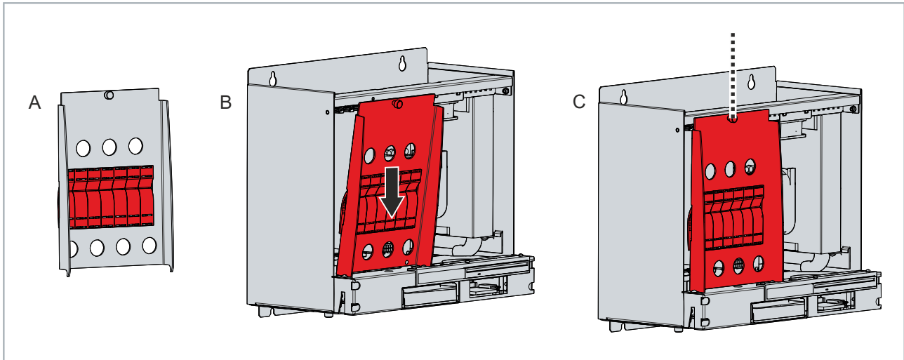
Abb. 26: Montage Kartenniederhalter
