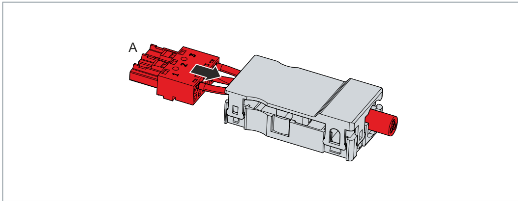
Abb. 17: Stecker einsetzen
