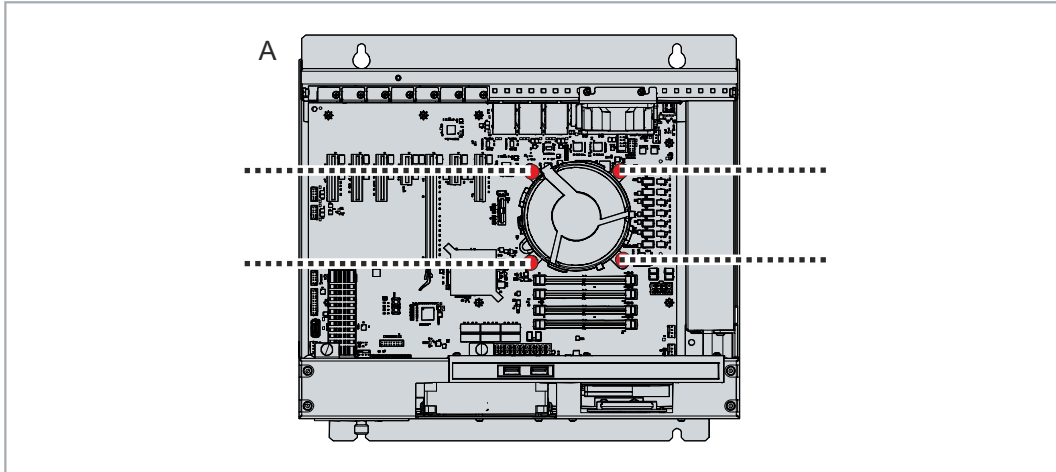
Abb. 37: Entriegelung CPU-Kühler
