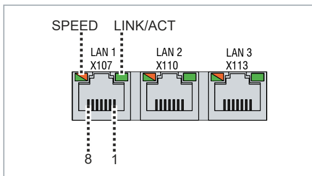
Abb. 7: Ethernet-Schnittstelle Pin-Nummerierung
