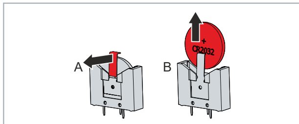
Abb. 29: Austausch Batterie
