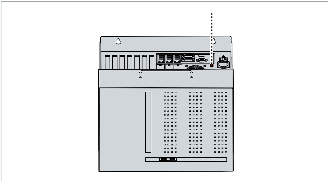
Abb. 15: Erdungsbolzen Funktionserdung
