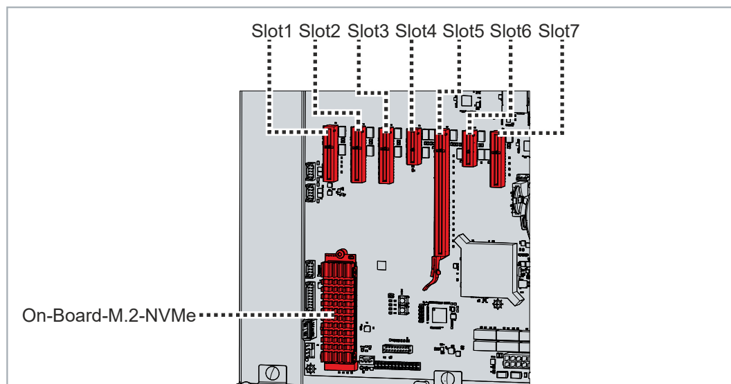
Abb. 30: Nummerierung PCIe®-Steckkartenslots
