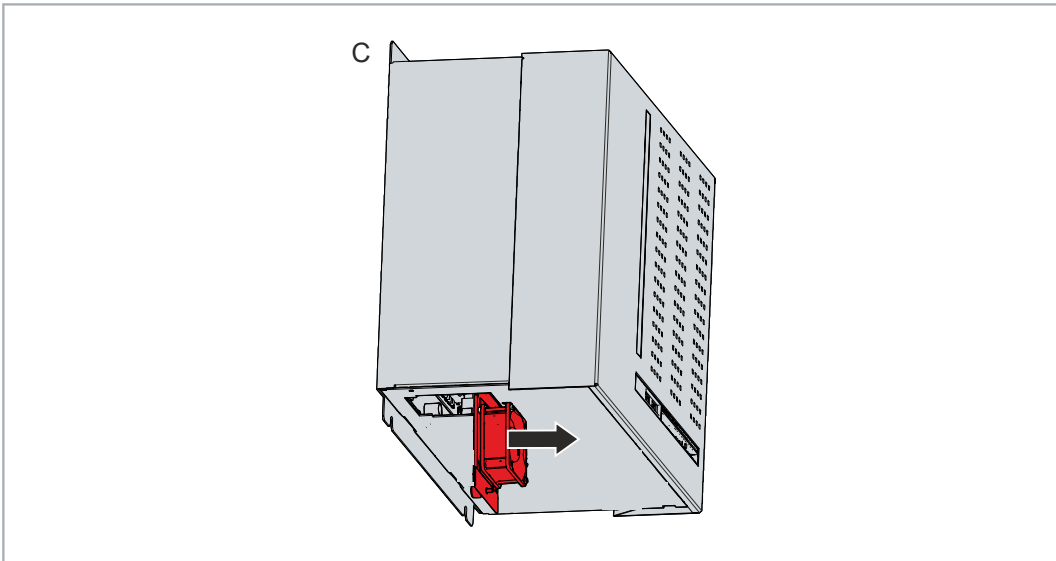
Abb. 34: Entnahme Lüfterkassette
