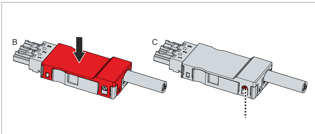
Abb. 18: Zugentlastungsgehäuse schließen
