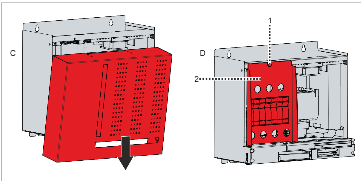
Abb. 25: Zugang Innenraum Gerät
