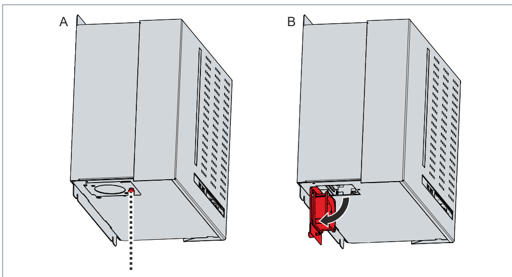
Abb. 33: Lösen Lüfterkassette
