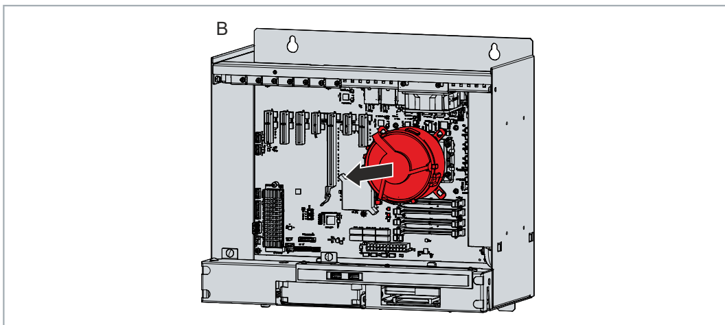
Abb. 38: Entnahme CPU-Kühler
