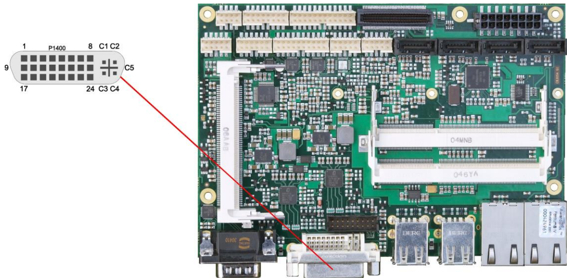
Pinbelegung DVI-I:
