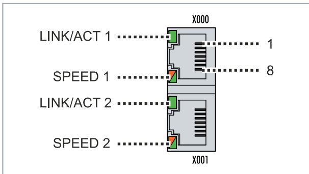
Abb. 14: EtherCAT-Master-Schnittstelle X300.
